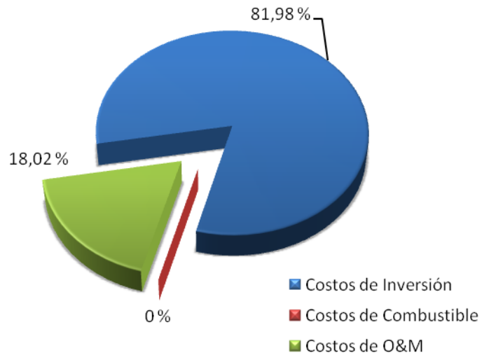
Figura I.12 Distribución de los Costos de Generación en Centrales Eólicas
