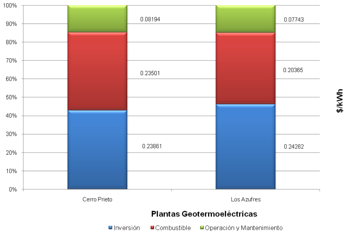
Figura I.8 Costo del kWh en Centrales Geotérmicas
