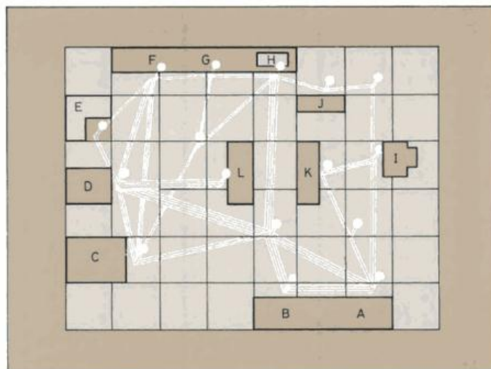
Diagrama de hilos. Valhonrat J (1991). Localización, distribución en planta y mantenimiento.
