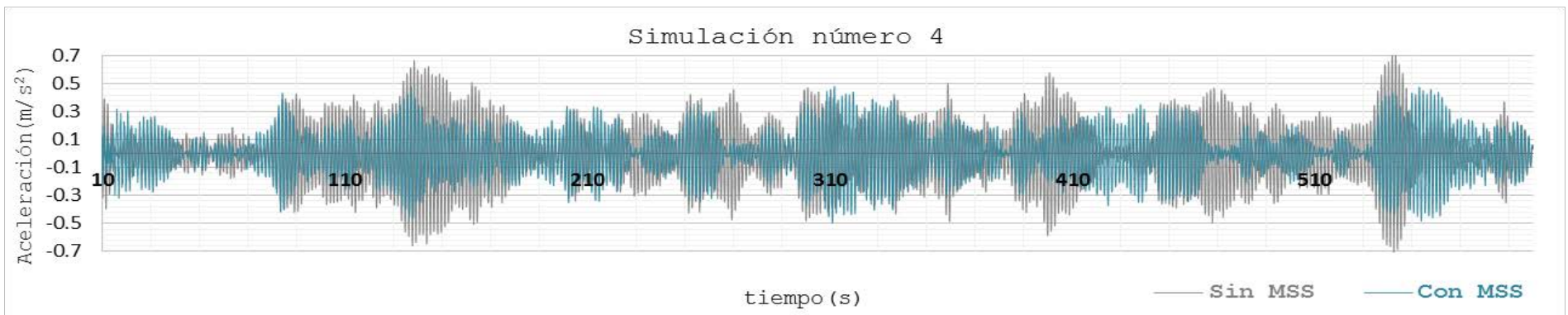
Figura 24. Historia en el tiempo de la aceleración en el nodo 392, debida a la cuarta simulación.
