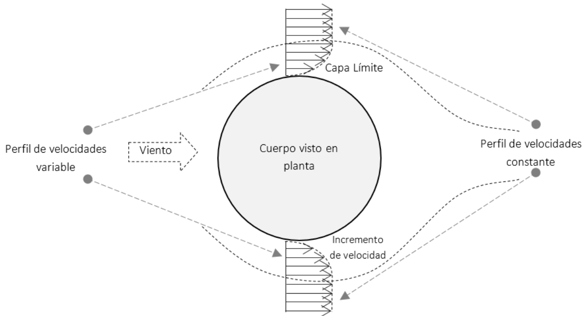
Figura 3. Capa límite.
