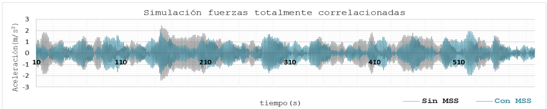
Figura 33. Historia en el tiempo de la aceleración en el nodo 392, debida a la simulación de fuerzas totalmente correlacionadas.
