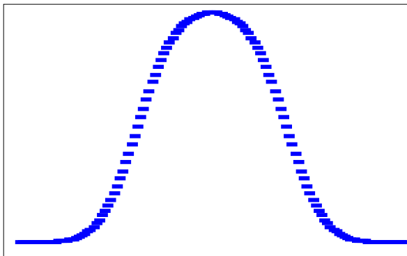
Figura 2.4 \phi(x, \sigma\sqrt{t})
