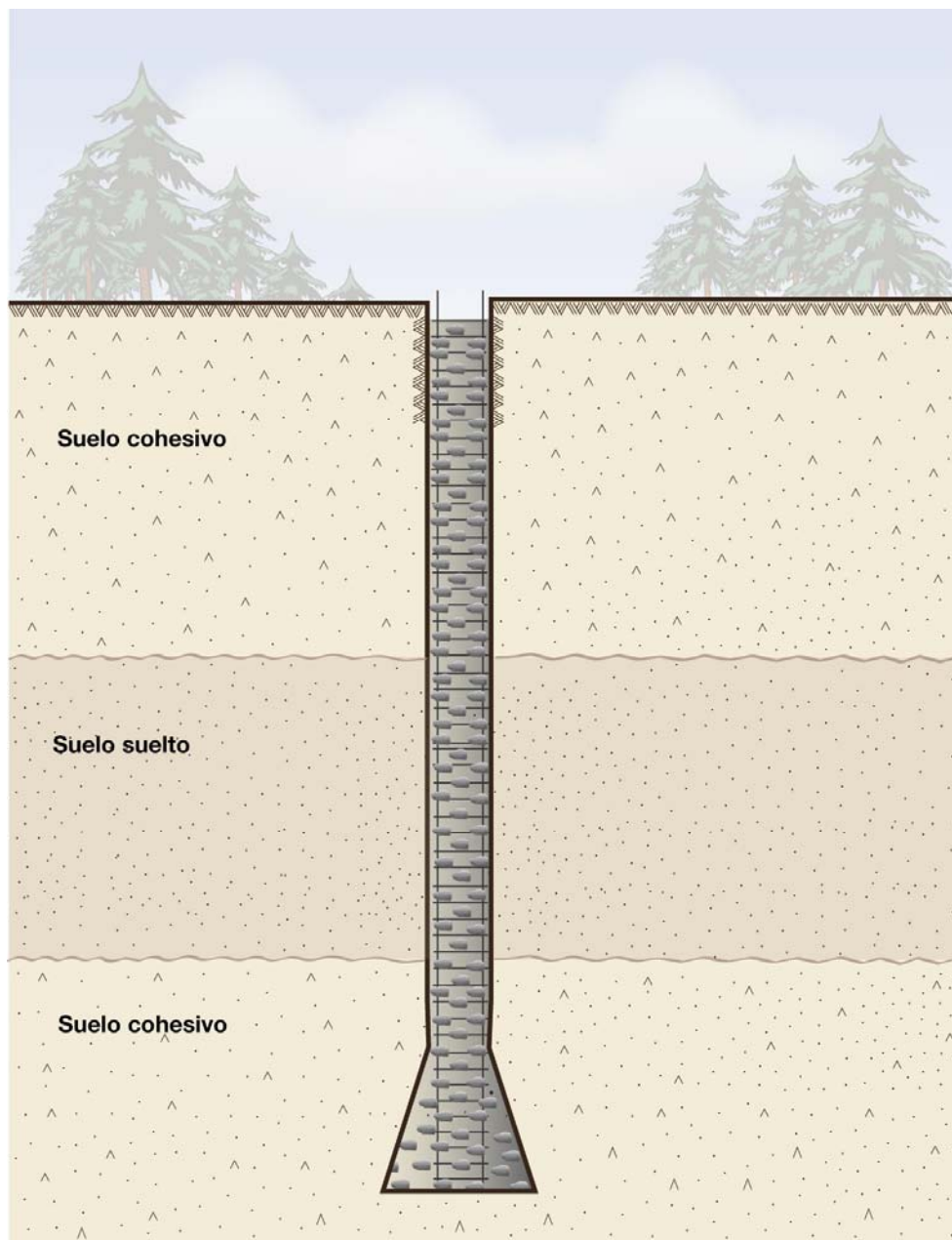
Fig. 1.17 Método de ademe, cimiento terminado
