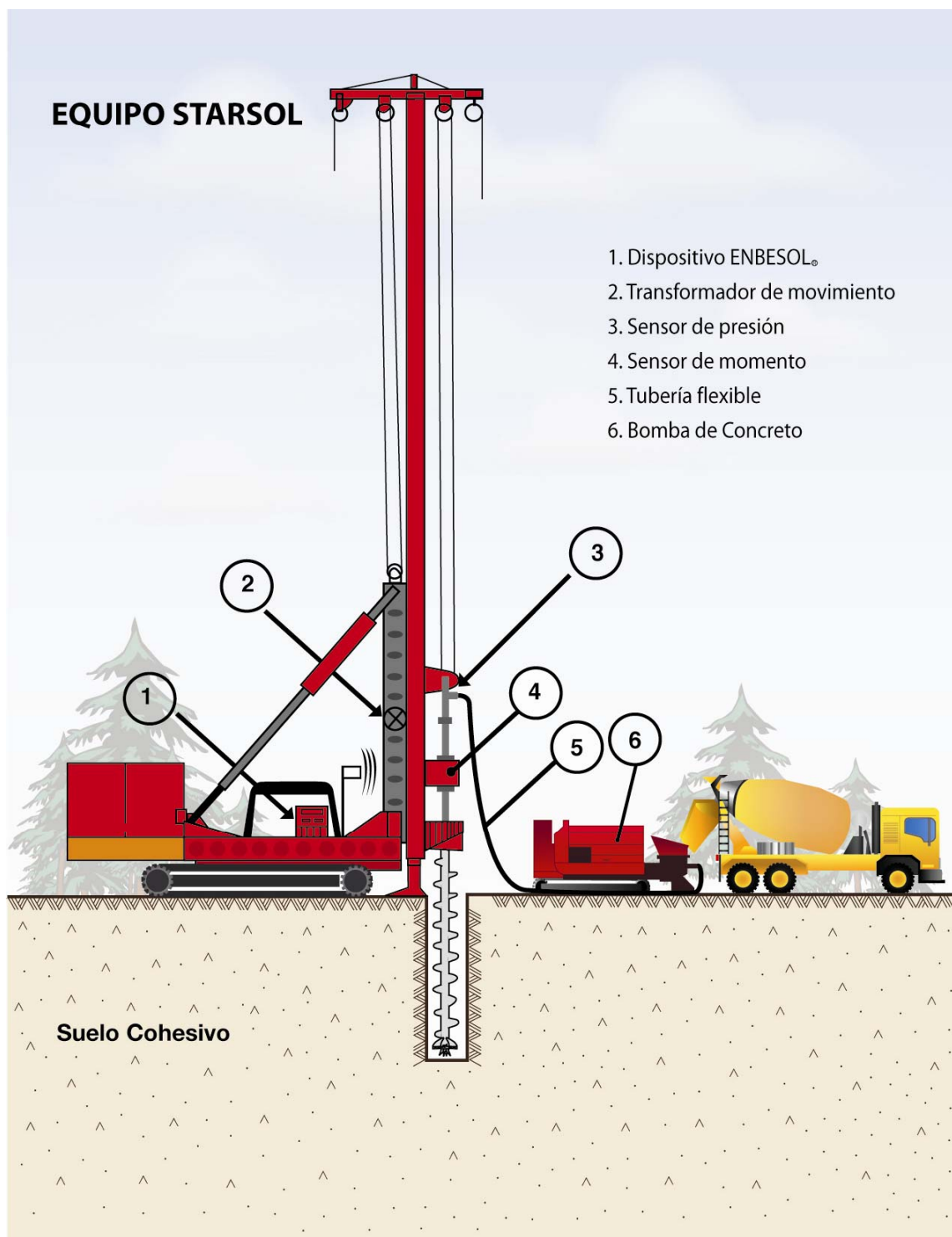
Fig. 2.15 Dispositivos que componen el equipo STARSOL®
