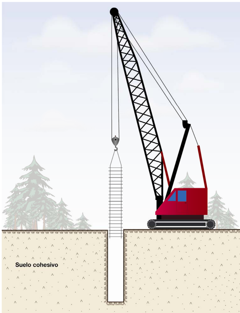
Fig. 1.4 Método seco, colocación del refuerzo de acero
