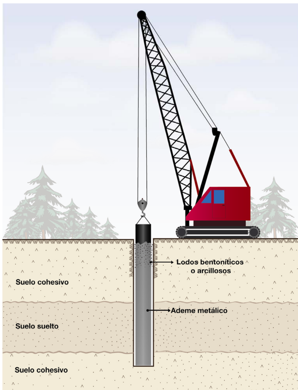
Fig. 1.11 Método de ademe, colocación del mismo
