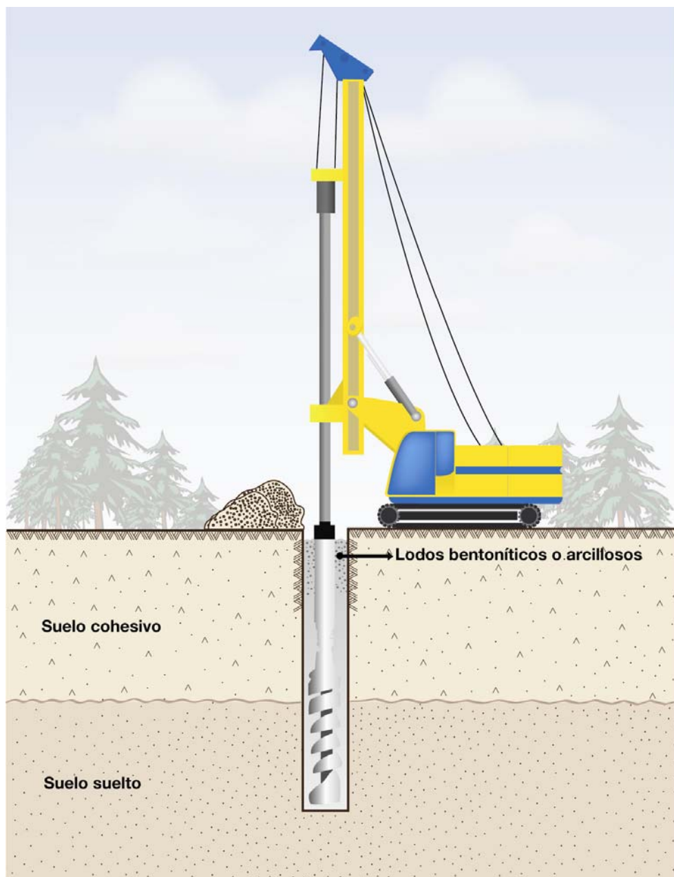
Fig. 1.19 Método de lodo, perforación empleando lodos
