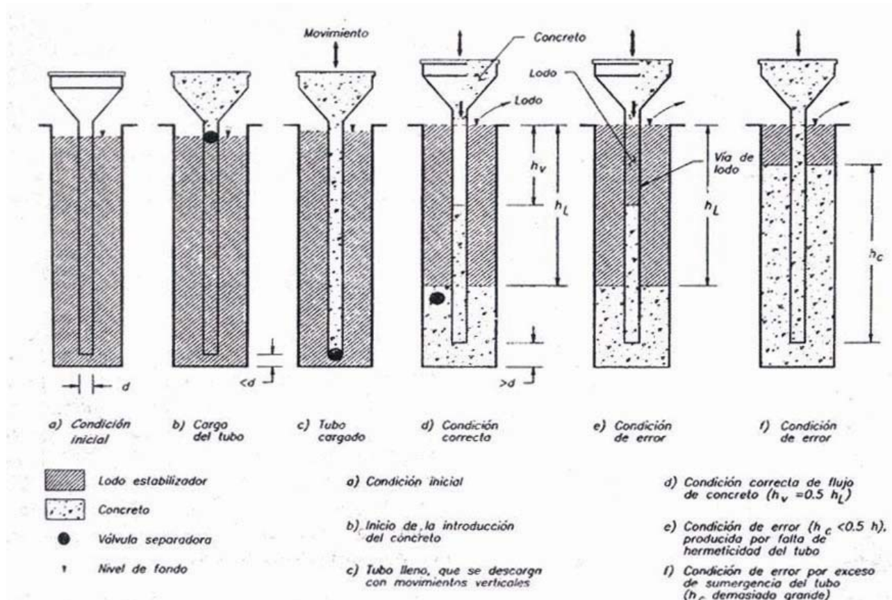
Fig. 1.7 Operación de tubo Tremie Ref. (4)
