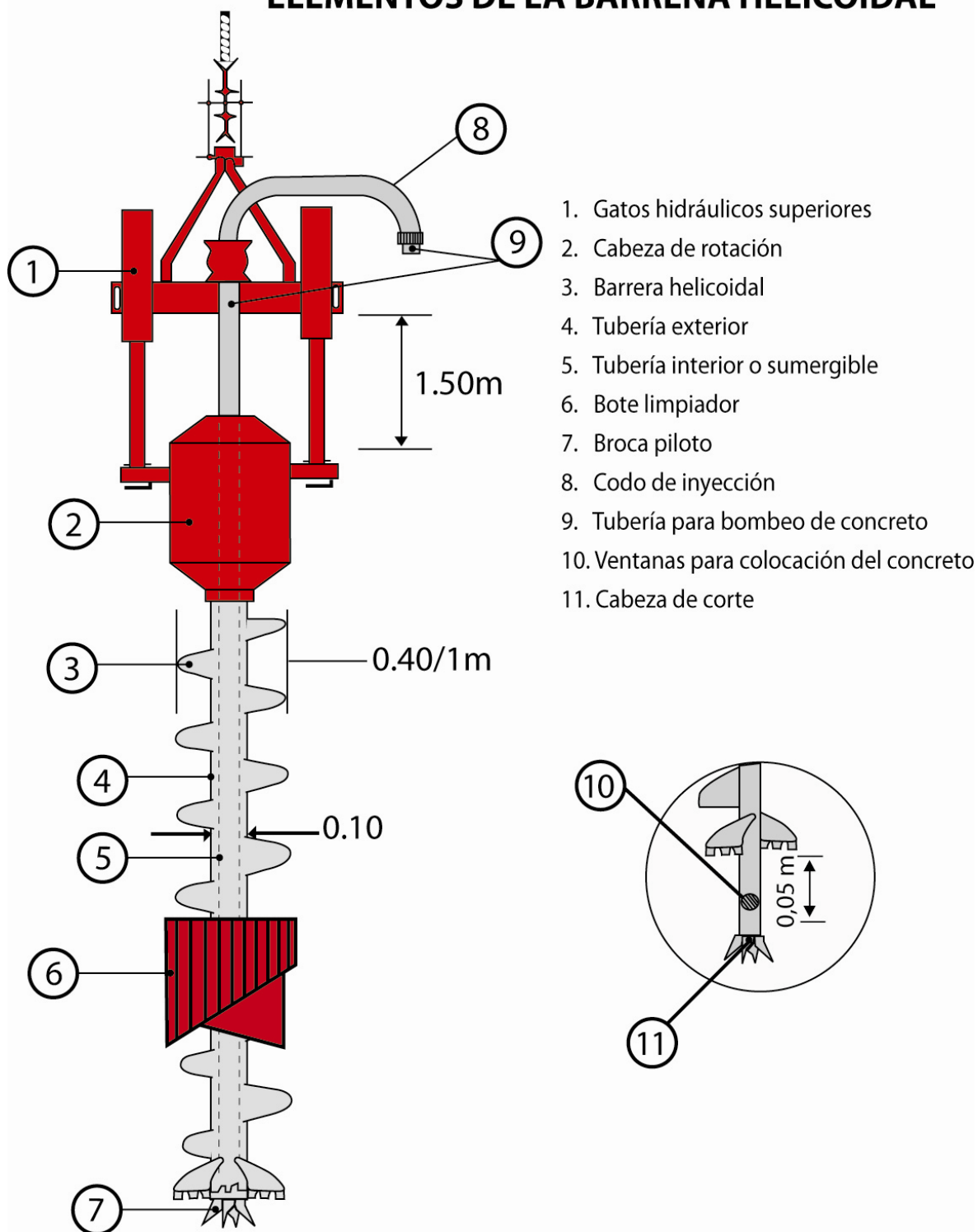
Fig. 2.9 Principales elementos de la barrena continua
