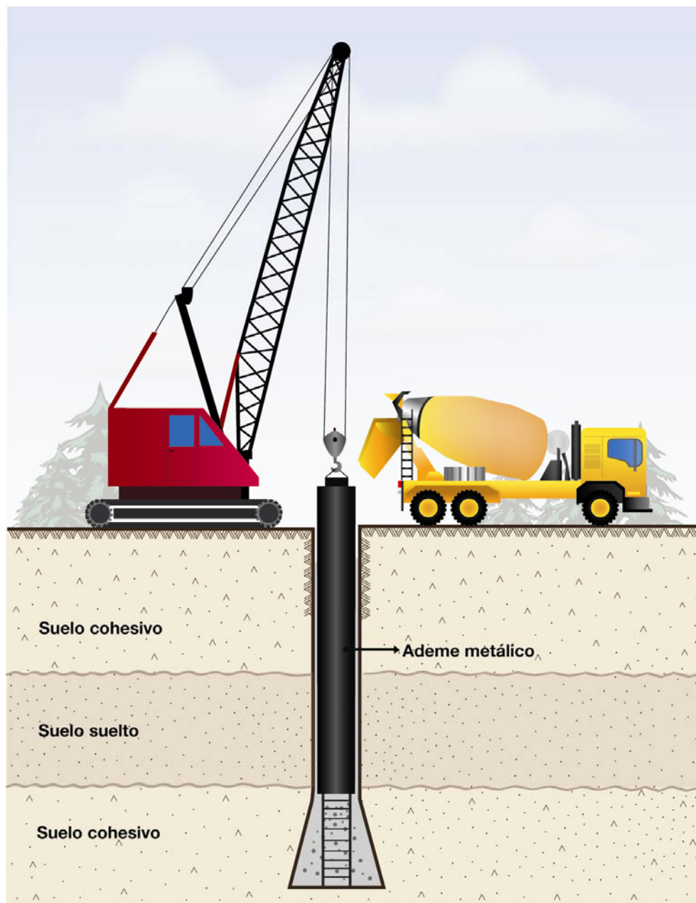
Fig. 1.15 Método de ademe, inicio del colado
