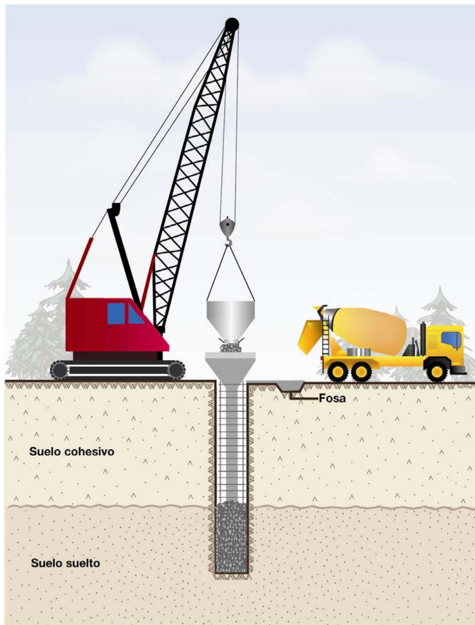
Fig. 1.21 Método de lodos, colado
