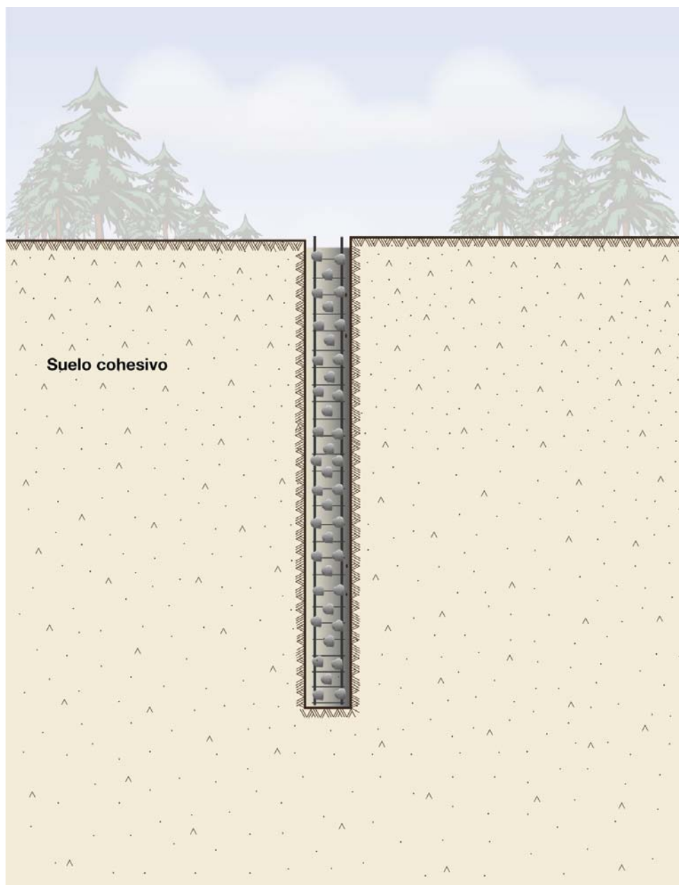
Fig. 1.8 Método seco, cemento terminado
