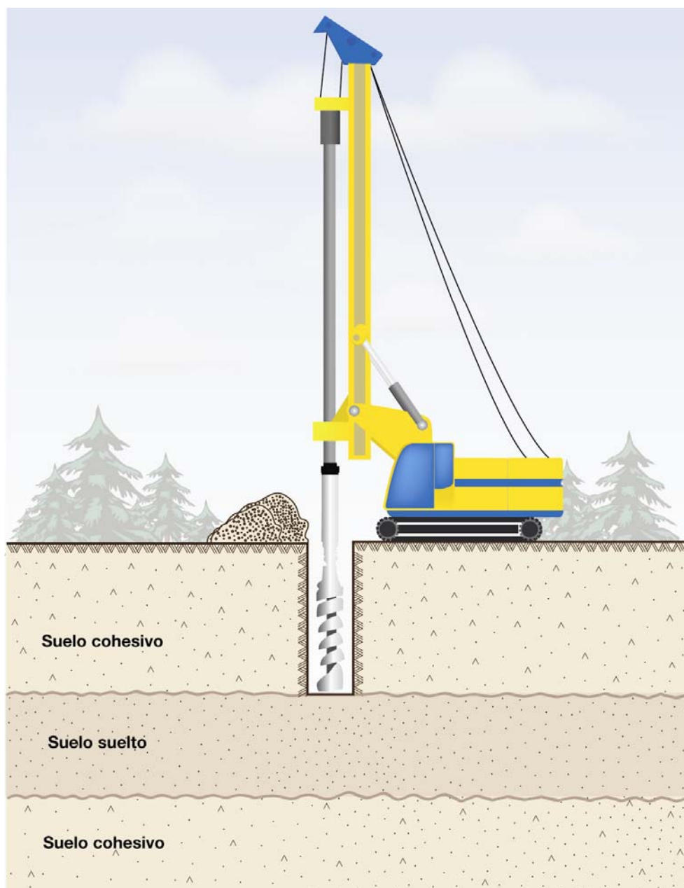
Fig. 1.9 Método de ademe, inicio de la perforación
