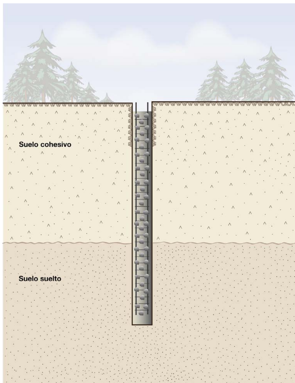
Fig. 1.22 Método de lodos, cemento terminado
