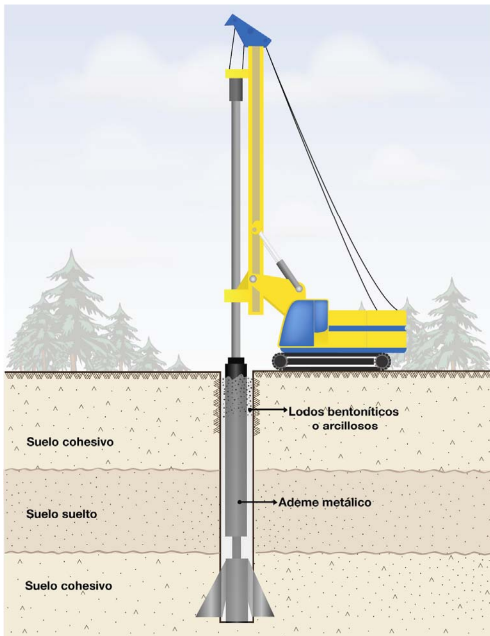
Fig. 1.14 Método de ademe, uso del amplificador
