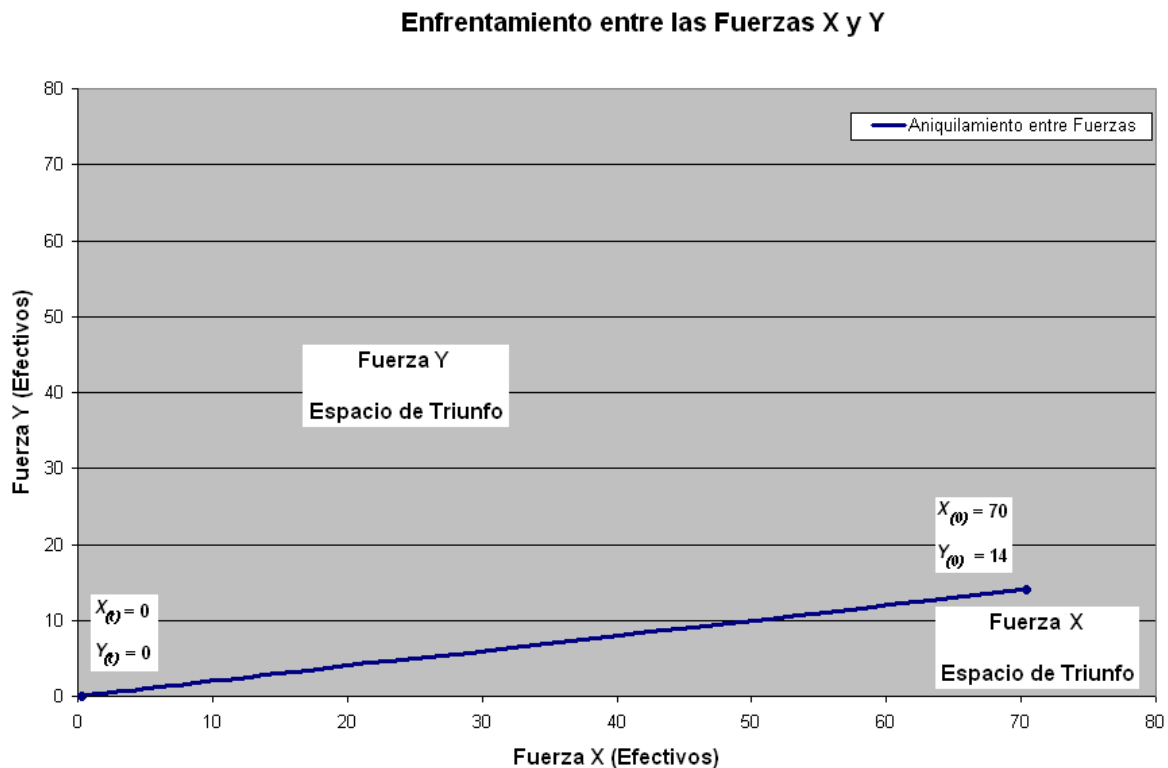
Figura 4.7. Enfrentamiento entre las fuerzas X y Y . El resultado es un empate.
