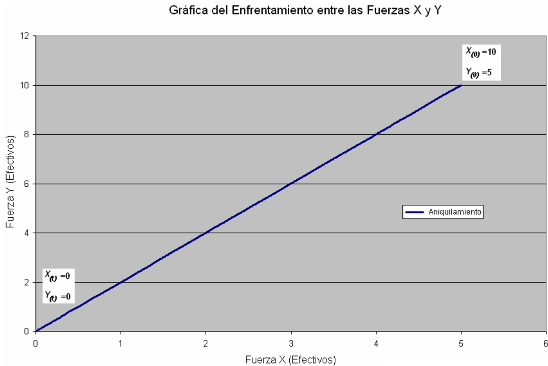
Figura 4.2. Enfrentamiento entre las fuerzas X y Y
