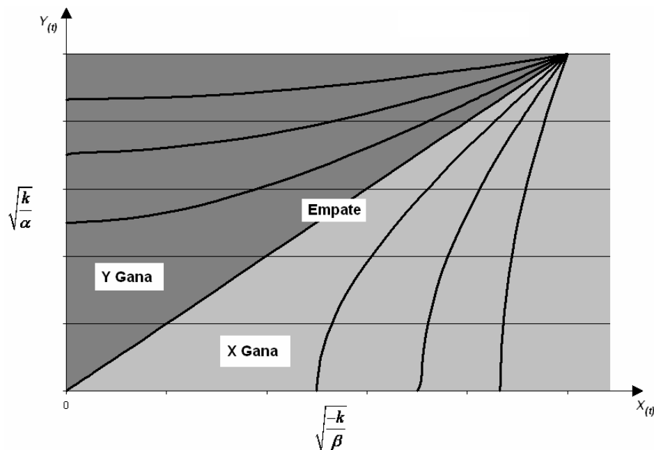
Figura 4.1. Hipérbolas para distintos valores de \alpha y \beta , considerando X_{(0)} y Y_{(0)} igual a 10
