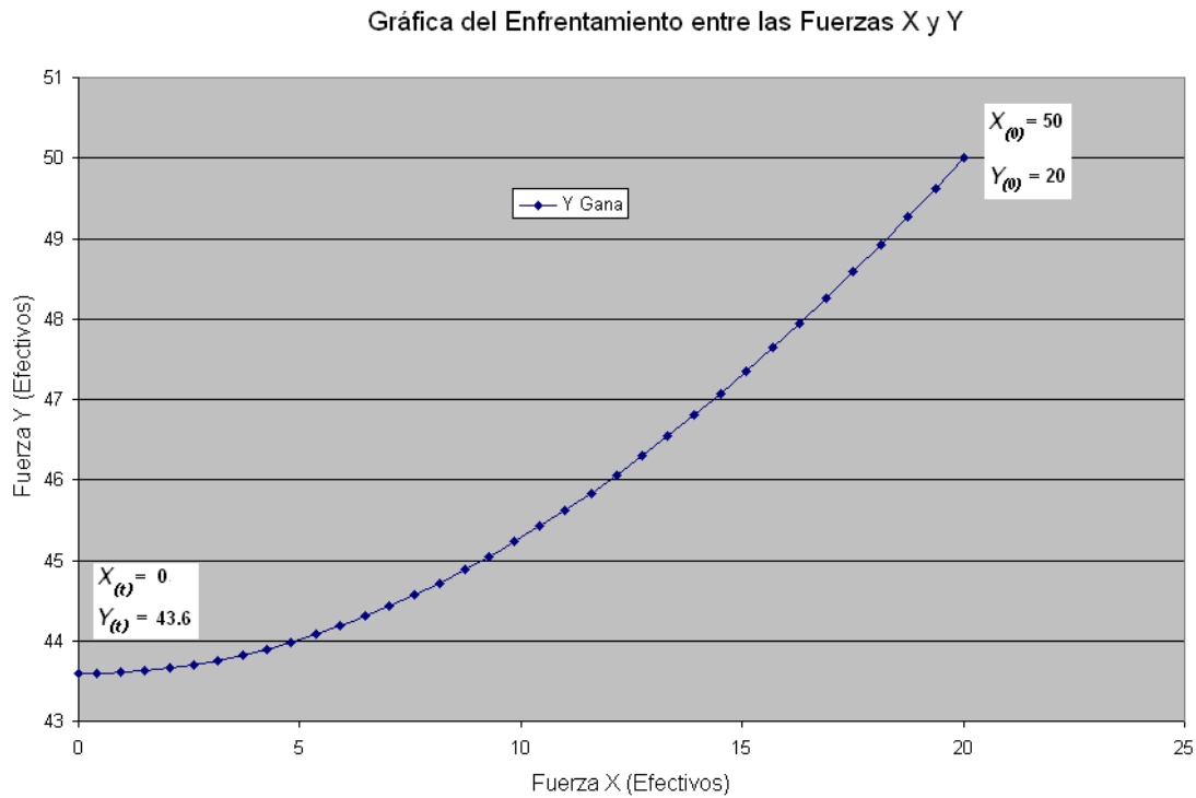
Figura 4.3. Enfrentamiento entre las fuerzas X y Y
