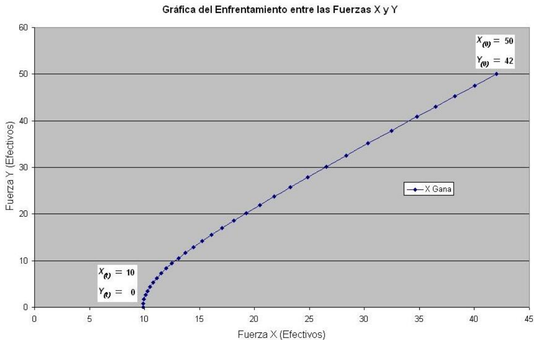
Figura 4.4. Enfrentamiento entre las fuerzas X y Y
