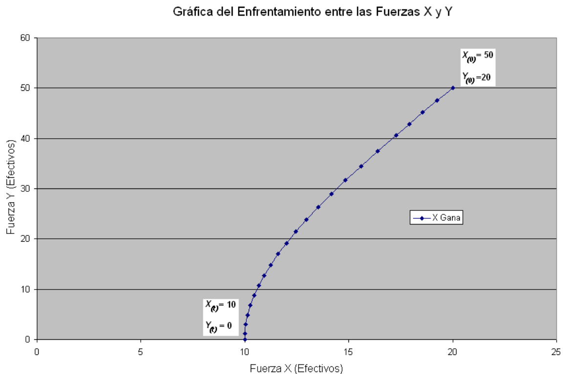
Figura 4.5. Enfrentamiento entre las fuerzas X y Y . La fuerza X aniquila a la fuerza Y
