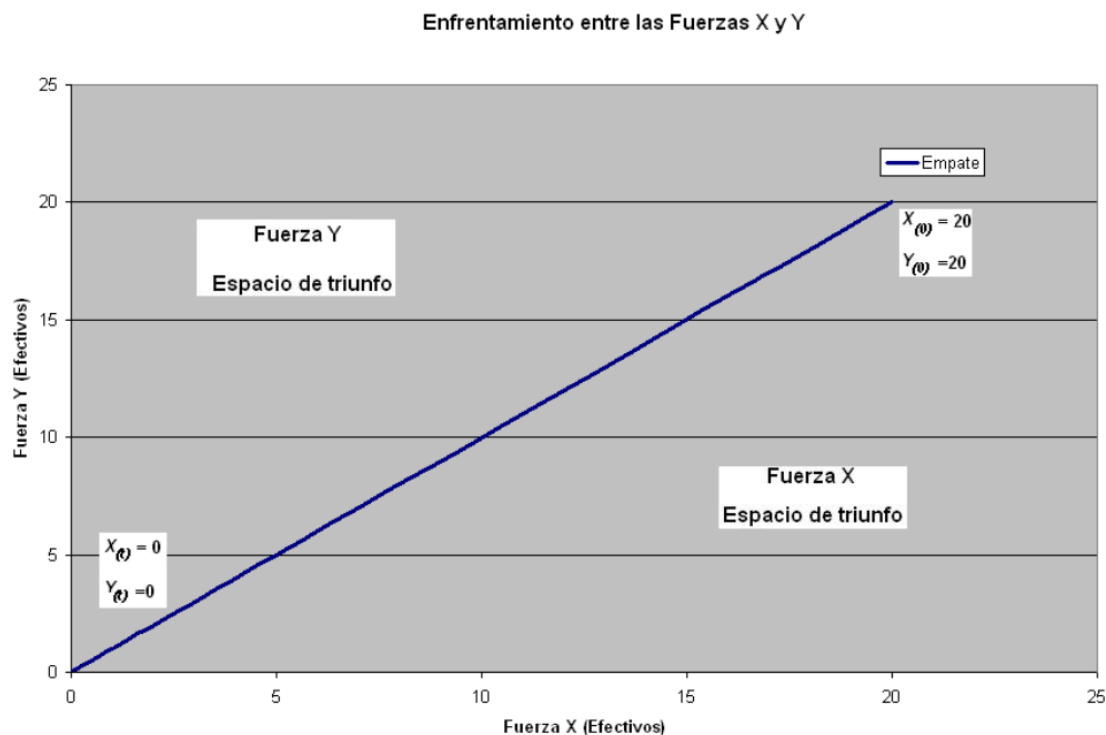
Figura 4.6. Enfrentamiento entre las fuerzas X y Y. Hay empate.
