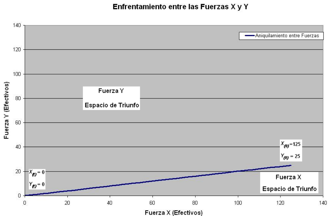
Figura 4.8. Enfrentamiento entre las fuerzas X y Y. El resultado es un empate.
