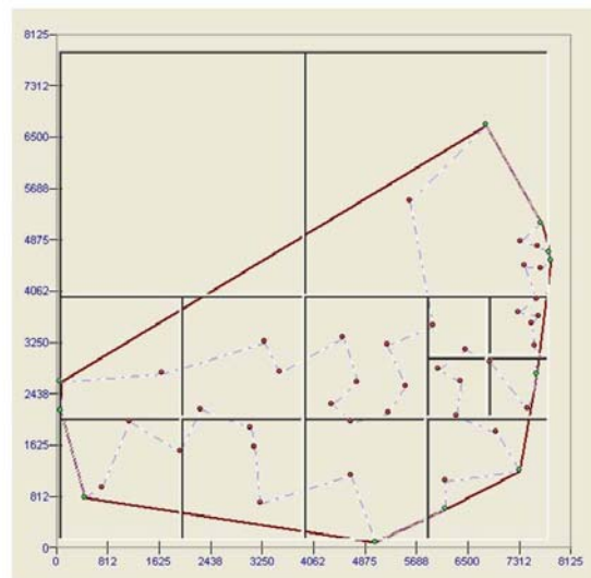
Figura 25. Ilustración de Quadrees
