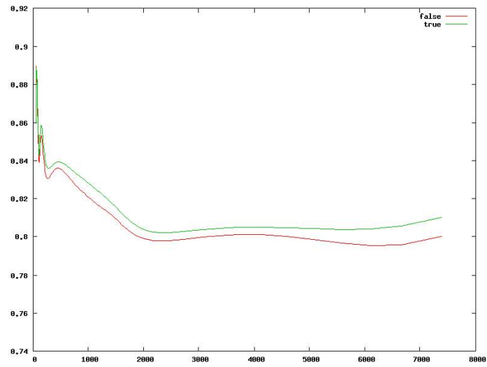
Gráfica 5.13 Porcentaje de mejora en la calidad del tour final con y sin recálculo.
