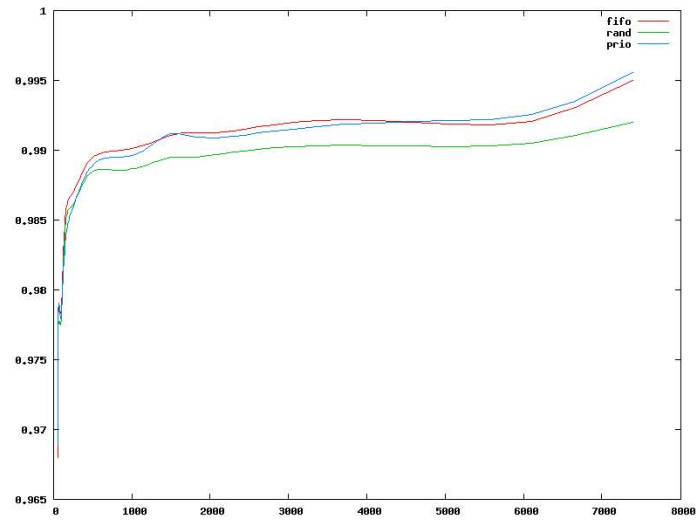
Gráfica 5.7 Radio de mejora en cada iteración en los tres criterios de destrucción.
