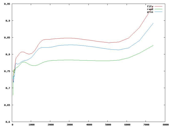
Gráfica 5.6 Porcentaje de desruces en cada iteración
