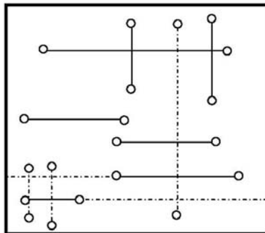
Figura 4.3 Estado del algoritmo de intersección de barrido del plano
