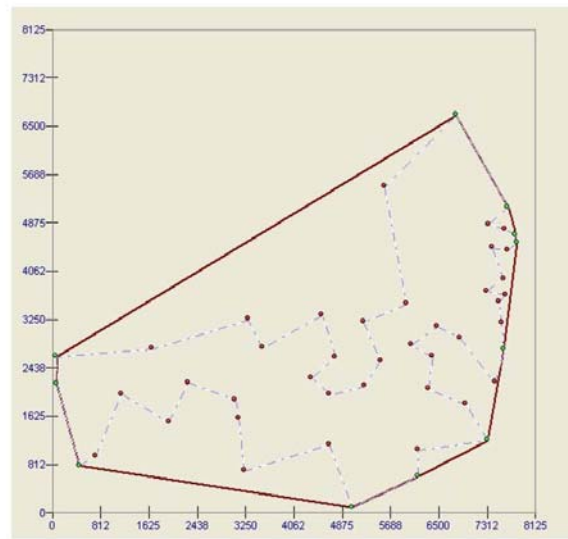
Figura 24. Ilustración de casco convexo.
