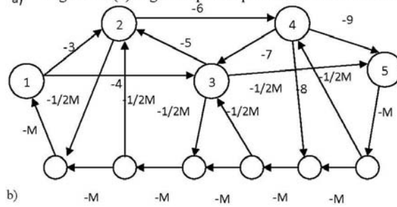
Figura 2.2 (b) Transformación de la digráfica al TSP
