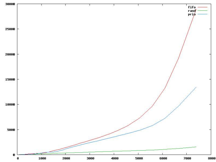
Gráfica 5.5 Iteraciones requeridas por los tres criterios de desruce.
