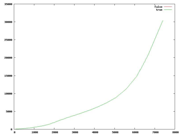
Gráfica 5.10 Tiempo de procesamiento con y sin recalcu de la lista L.
