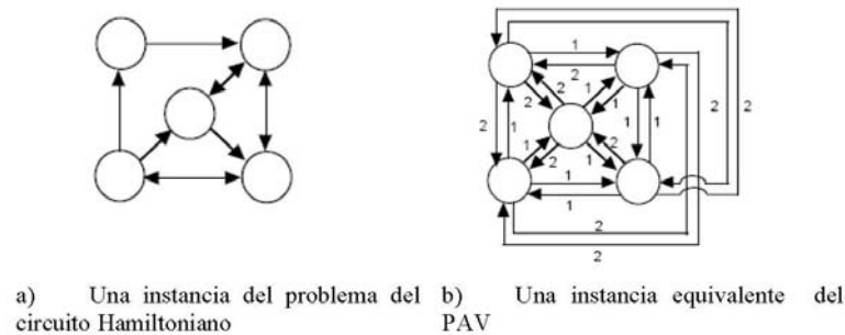
Figura 2.4 Reducción polinomial del problema del circuito hamiltoniano al problema del agente viajero (PAV)
