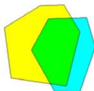
Figura 4.6 Intersección de polígonos convexos
