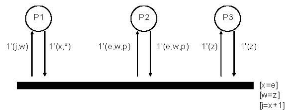
Figura 10-1: Modelo en RdPC del Taller de trabajo 3x3
