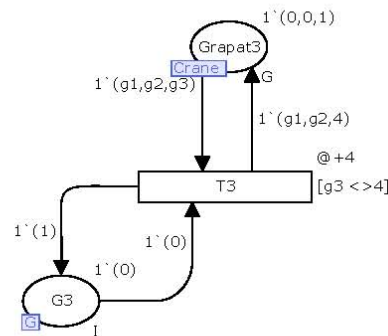
Figura 4-20: Movimiento de grúa
