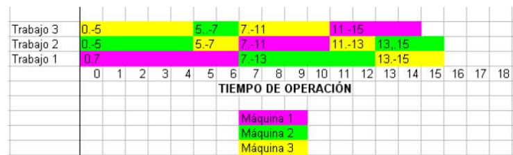
Figura 4-12: Diagrama de Gantt de la secuencia óptima para el T-T 3x3
