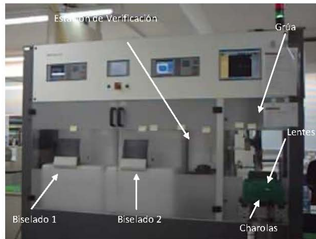
Figura 4-16: Esquema de la máquina de control numérico
