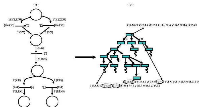
Figura 2-7: Información de un árbol de alcance típico
