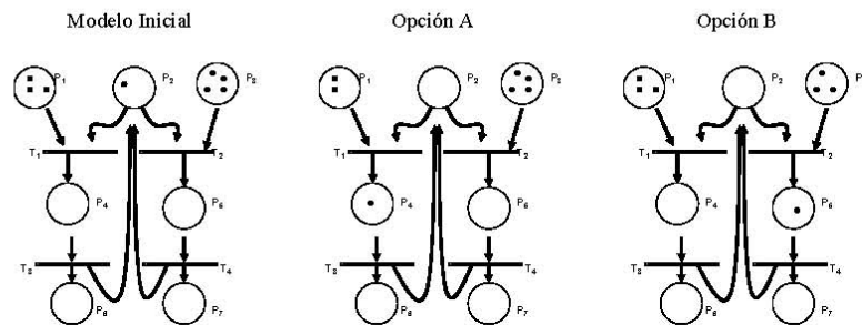
Figura 1-7: Modelo de RdP con recursos compartidos
