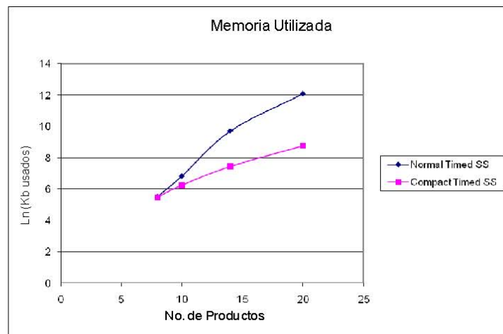
Figura 2-13: Uso de memoria para el modelo de manufactura en RdPC
