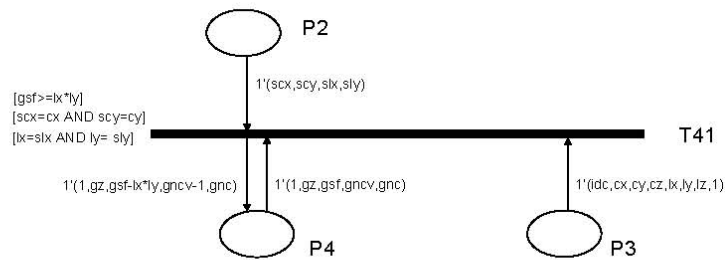
Figura 9-4: Posicionado de caja virtual en espacio disponible de la misma dimensión
