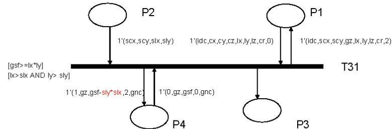
Figura 9-3: Posicionado de caja excediendo dimensiones de superficie libre
