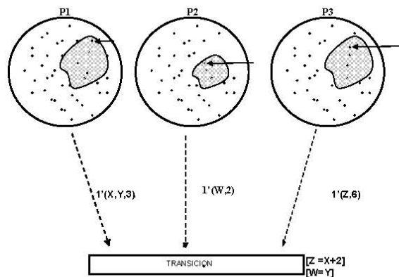
Figura 3-3: Transición lista para disparo
