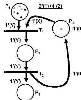
Figura 1-11: RdPC de un sistema con recursos compartidos
