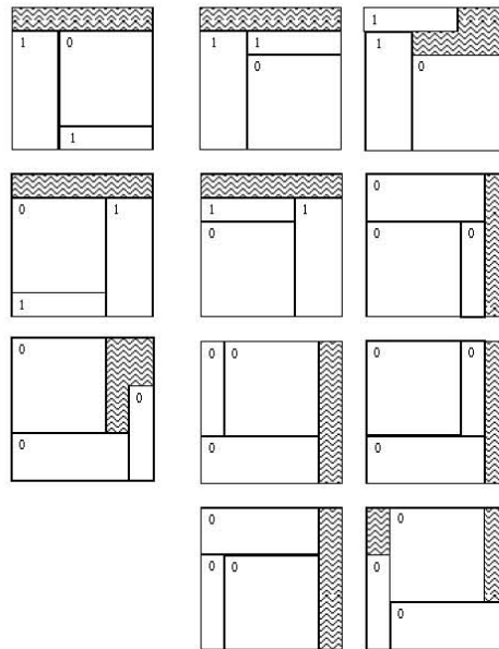
Figura 4-7: Soluciones al problema del Paletizado 3 cajas diferentes dimensiones.
