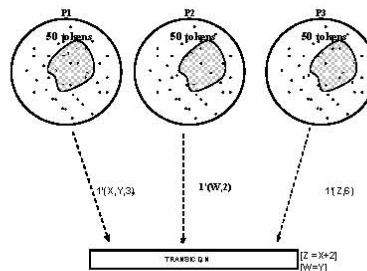
Figura 2-6: Evaluación de una transición
