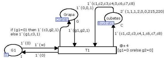
Figura 4-19: Las transiciones de recogida de lentes
