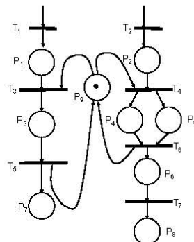
Figura 1-6: Compartición de recursos
