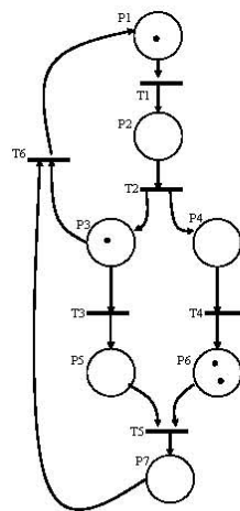
Figura 1-1: Marcado en las RdP
