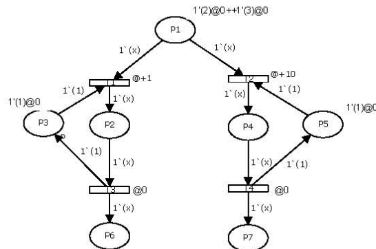
Figura 2-16: Modelo en RdPCT con transiciones en conflicto
