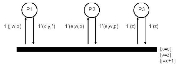
Figura 4-13: Modelo en RdPC del taller de trabajo 6x6
