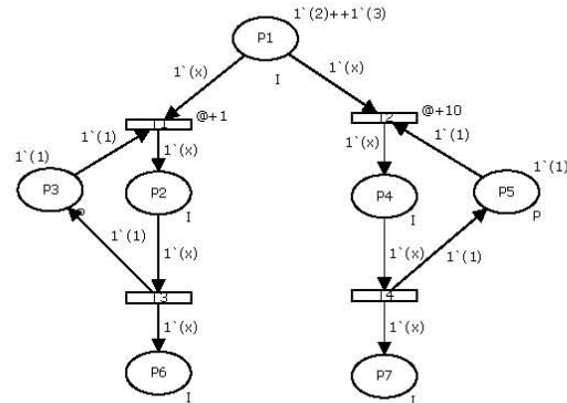
Figura 2-12: Modelo en RdPC temporales de un sistema de manufactura
