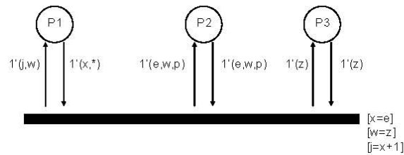
Figura 4-8: Modelo en RdPC del taller de trabajo 3x3
