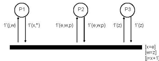
Figura 8-1: Modelo RdPC de Taller de trabajo 3x3
