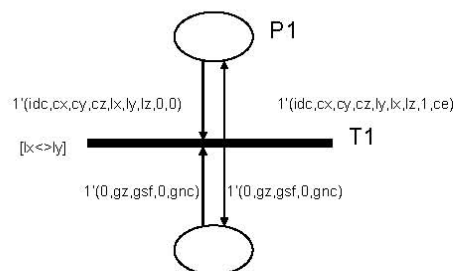
Figura 9-1: Rotación de una caja
