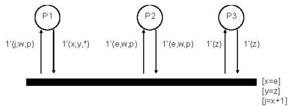
Figura 10-5: Modelo en RdPC del Taller de trabajo 6x6
