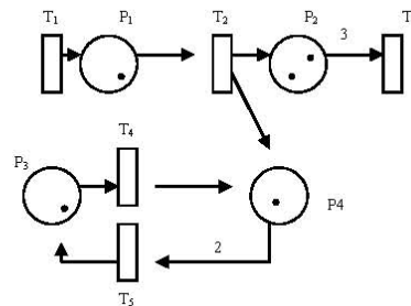
Figura 1-3: Red de Petri ordinaria
