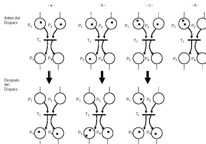
Figura 1-2: El disparo de una transición
