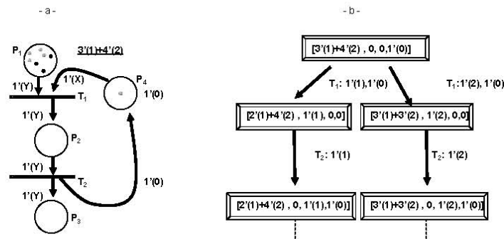
Figura 1-9: El árbol de alcance
