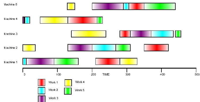
Figura 10-4: Diagrama de Gantt de la secuencia Óptima del T-T 5x5
