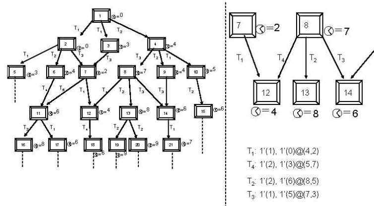
Figura 1-10: Árbol de alcance con extensión temporal
