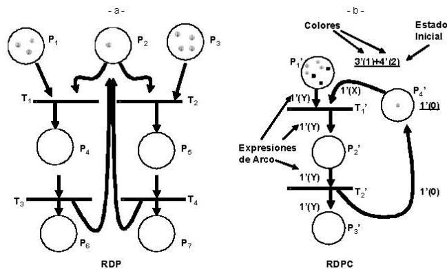
Figura 1-8: Modelado en RdP y RdPC
