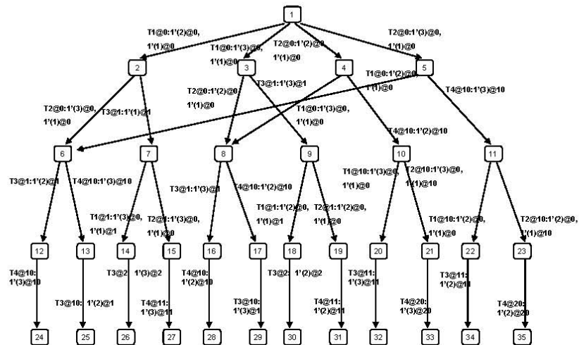
Figura 2-18: Espacio de estados del modelo en RDPCT
