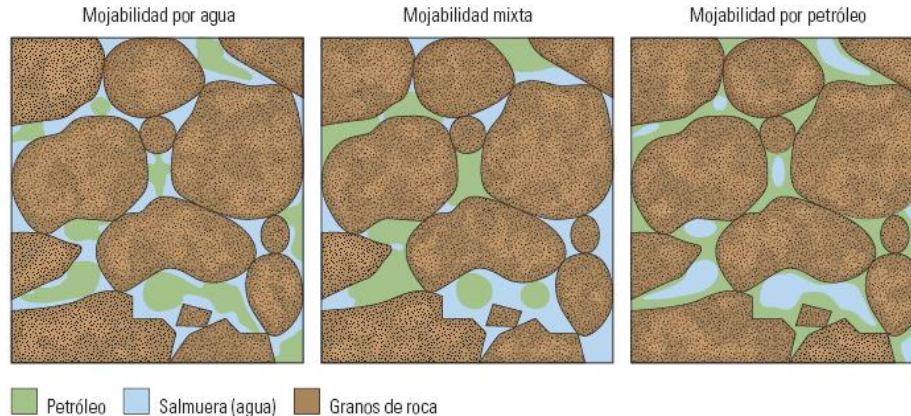
Figura 1.15 Escenarios de mojabilidad en un medio poroso
