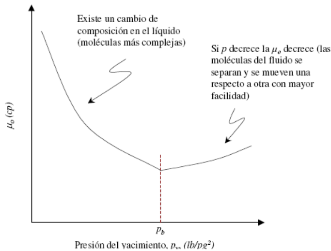
Figura 1.13 Variación de la viscosidad del aceite en función de la presión y temperatura en el yacimiento.
