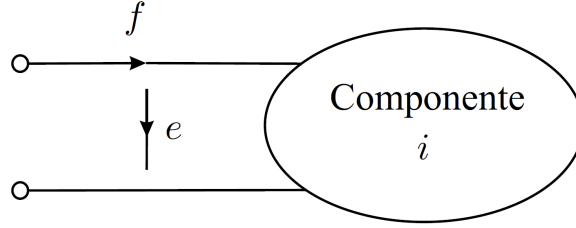
Figura 2.3: Sentidos definidos como positivos para las variables de esfuerzo y flujo
