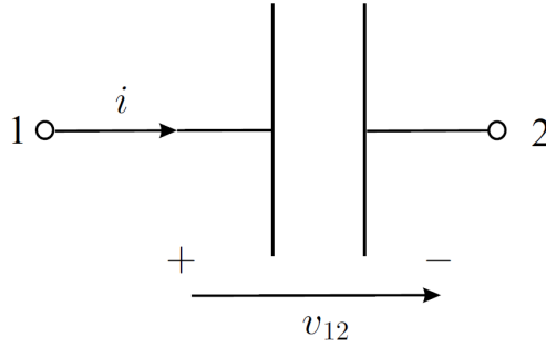
Figura 2.5: Un capacitor como almacenador de flujo
