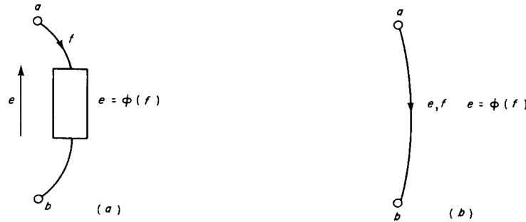
Figura 2.6: Segmento de linea que puede representar a cualquier elemento del sistema.
