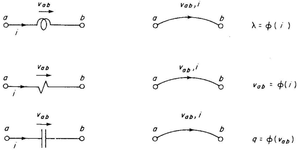
Figura 2.7: Elementos del sistema representados como segmentos de linea orientados.
