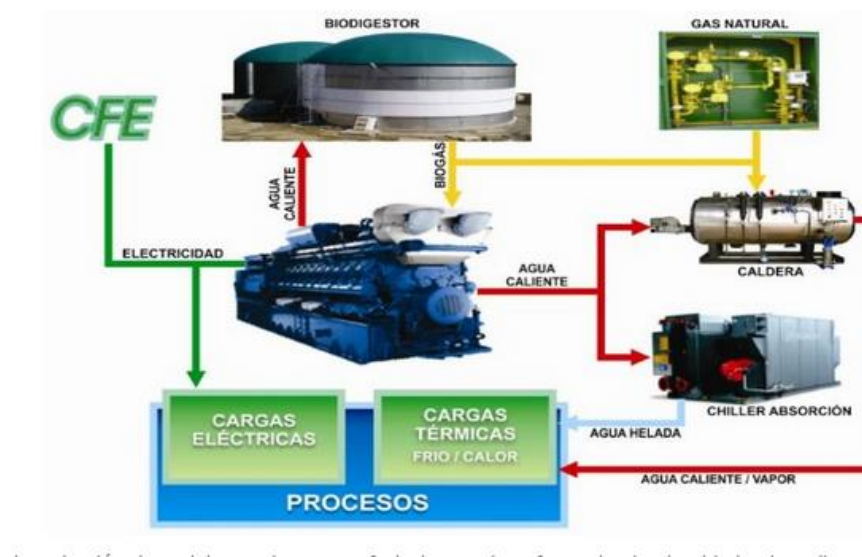
Figura 5 Esquema de la empresa Electríz de un sistema de cogeneración
