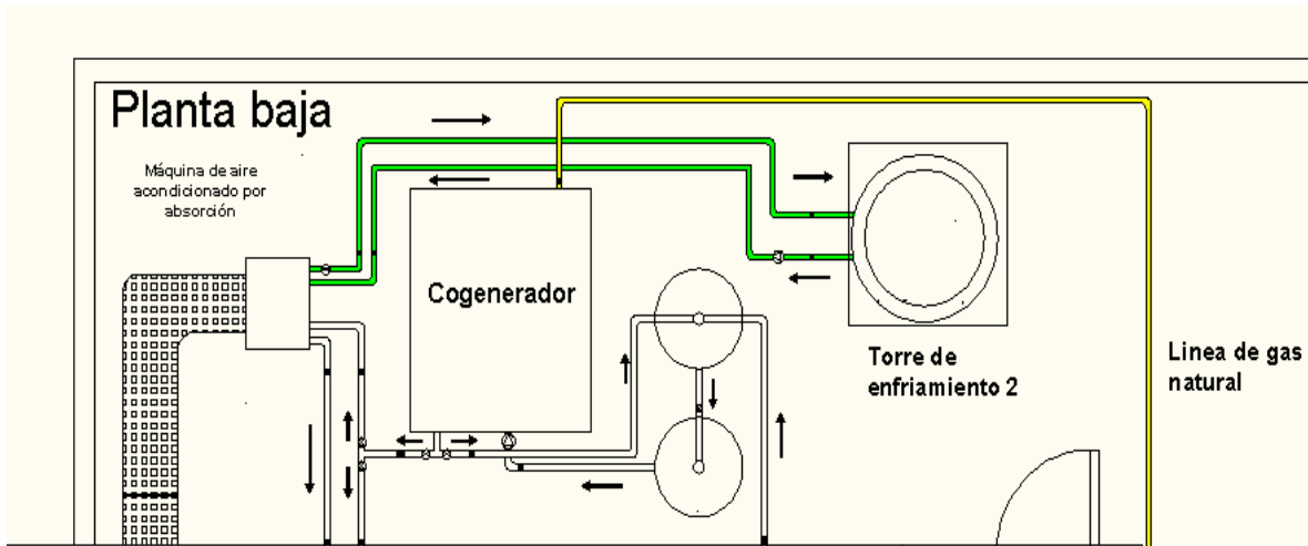
Figura 50; Circuito de enfriamiento de la máquina de absorción.
