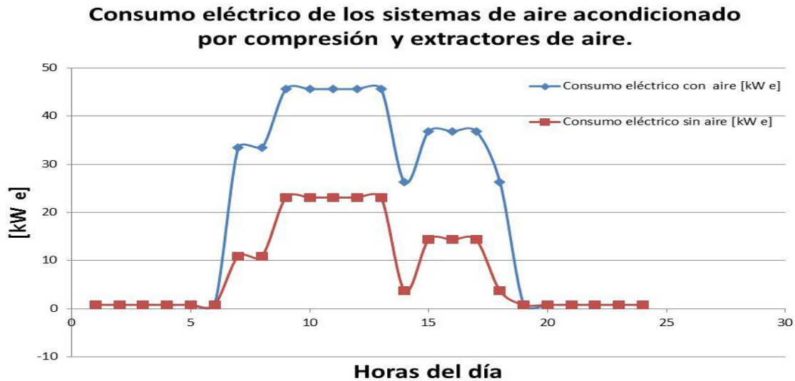
Figura 32; comparación del consumo eléctrico del aire acondicionado, con respecto al consumo actual.
