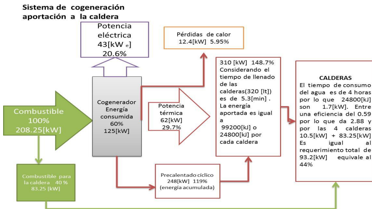
Figura 57; Diagrama de energía aprovechada por el sistema de cogeneración.
