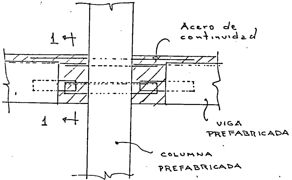
ELEVACION
