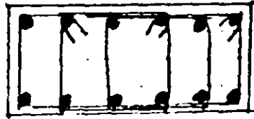
Fig 10.12 Arreglos admisibles de refuerzo en columnas de marcos dúctiles de concreto
