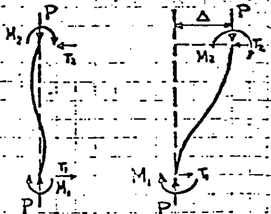
COLUMNAS
