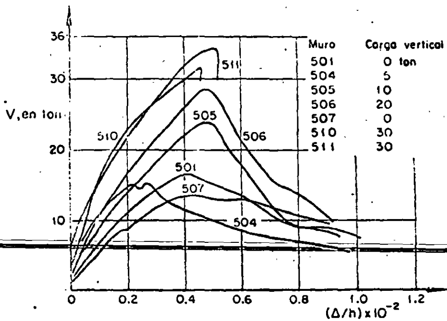
Muros de bloque de concreto. Fallo en tensión diagonal. Efecto de la carga vertical
