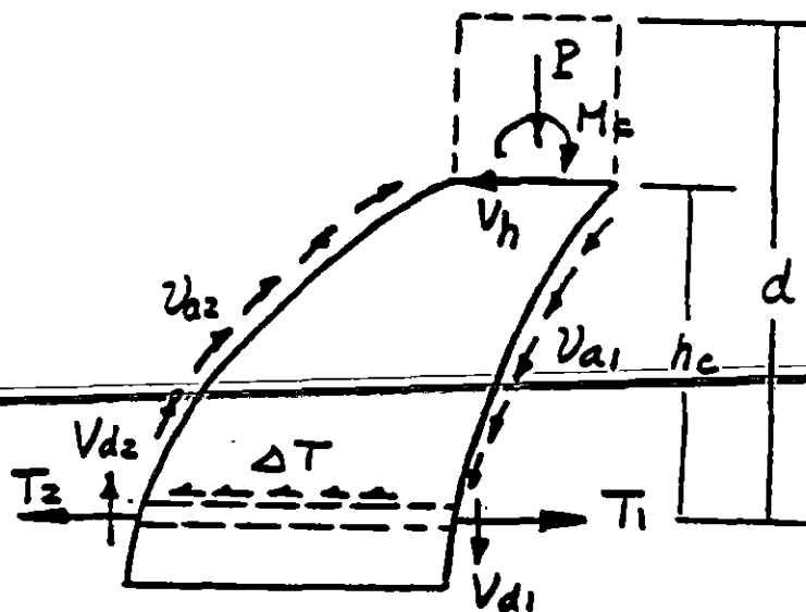
Fig. 15 Acciones en el "cantil ver" formado por grietas de flexo-cortante
