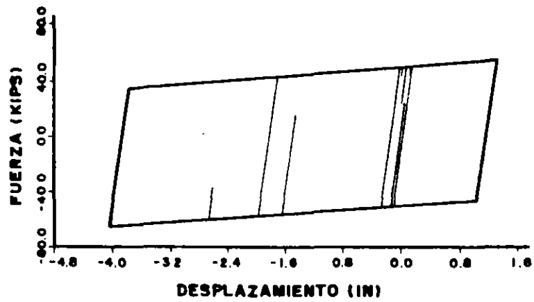
Fig. 39 Comportamiento histerético
