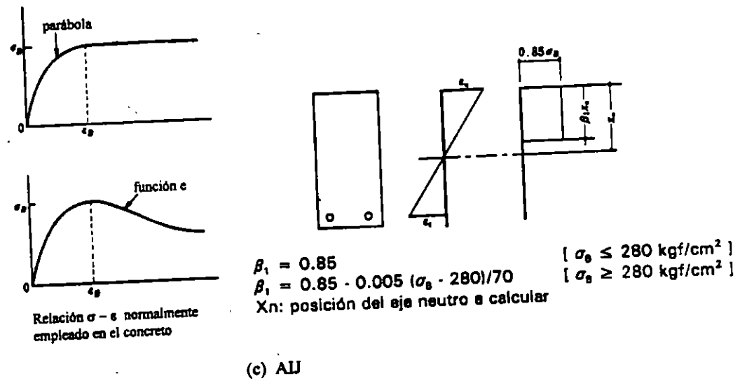
Fig. 7 Hipótesis simplificadoras para el análisis por flexión según los reglamentos RDF, AIC y AIJ
