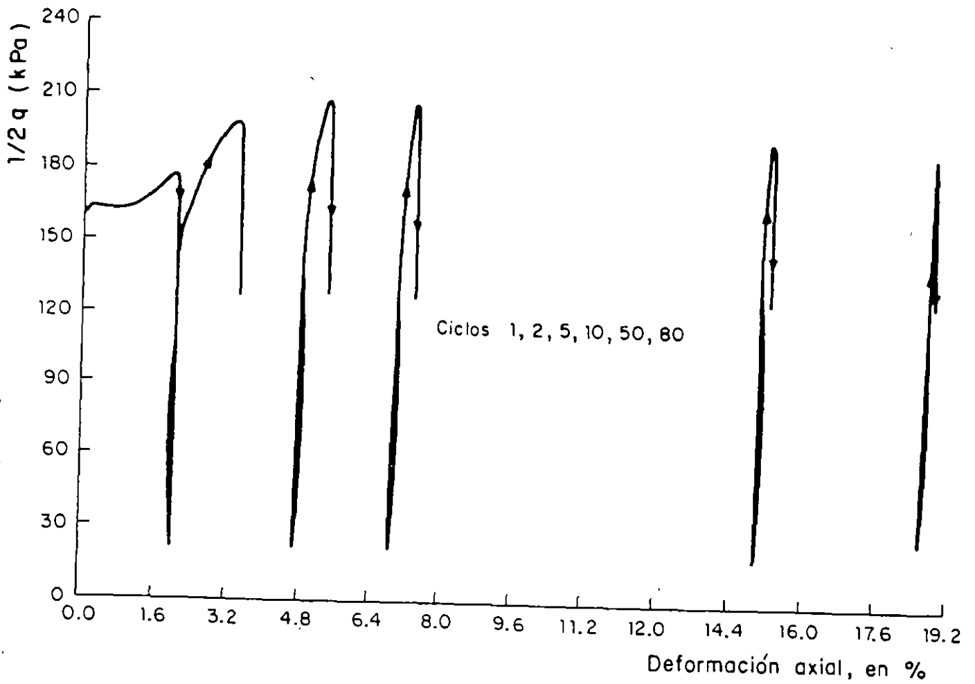
Fig 10.A Ejemplo de una curva esfuerzo-deformación con endurecimiento progresivo.
