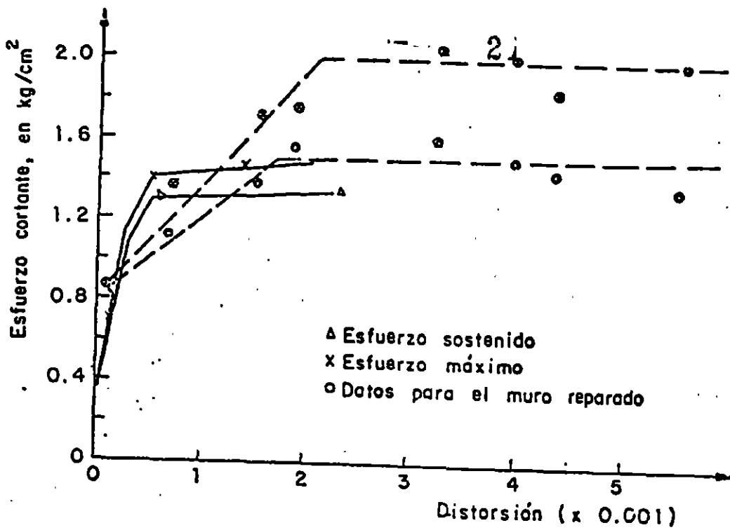
Fig 12. Envolventes de esfuerzos del muro 7
