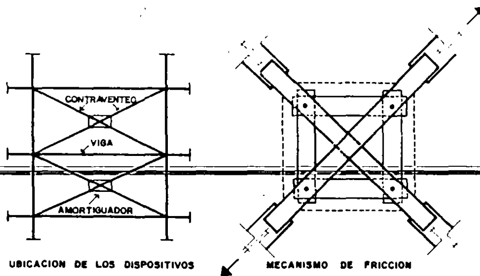
Fig. 24 Dissipador de energia por fricción
