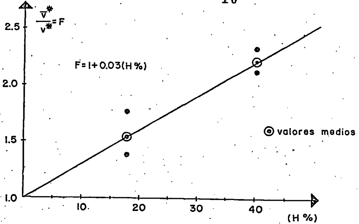
Fig.2 Aumento de la resistencia con el llenado de huecos y aplanado en las caras laterales.
