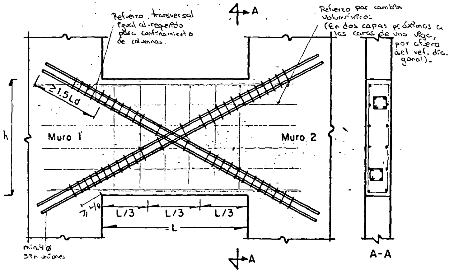
Fig. 10.21 Refuerzo de viga de acoplamiento que une muros de concreto (para l/h < 4 )
