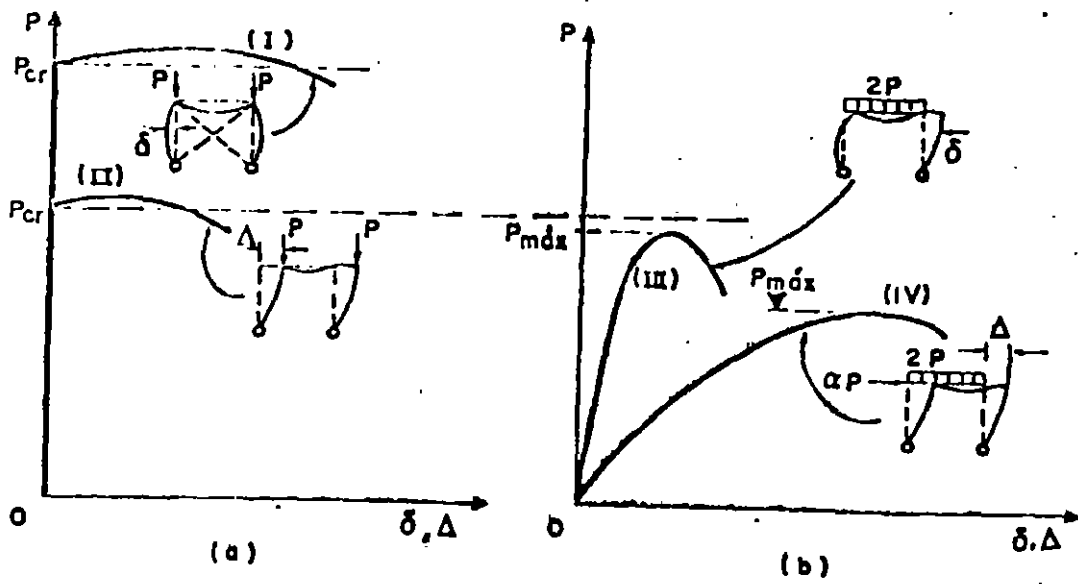
FIG. 5 Curvas carga-desplazamiento de marcos que fallan por pandeo y por inestabilidad
