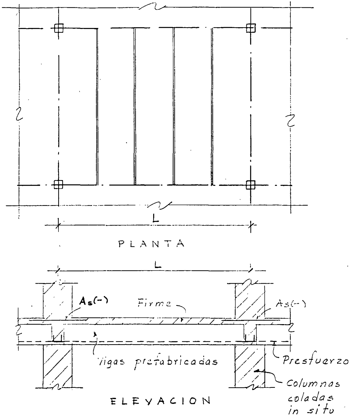
ESTRUCTURACION PRETENSADA
