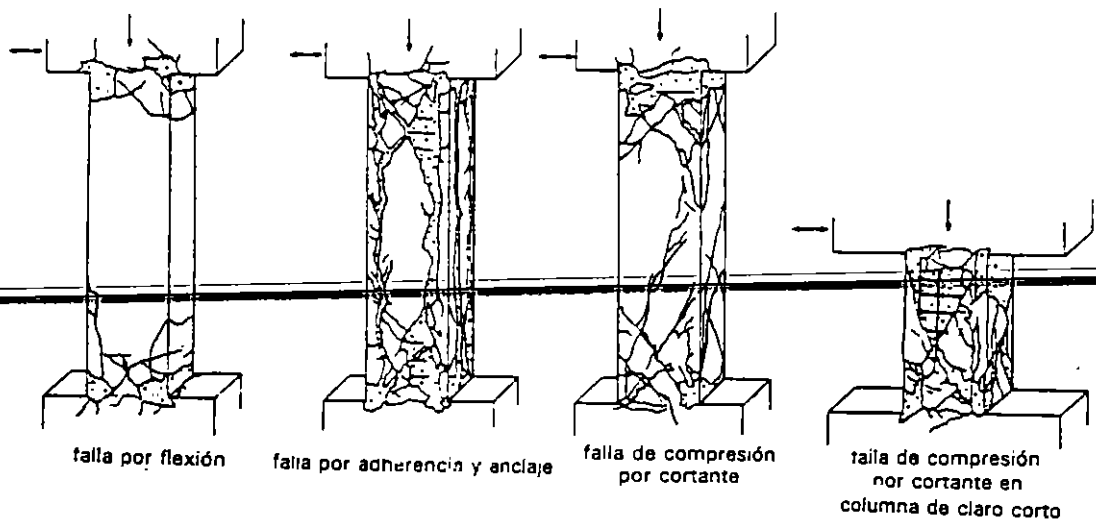
Fig. 24 Modos de falla en columnas
