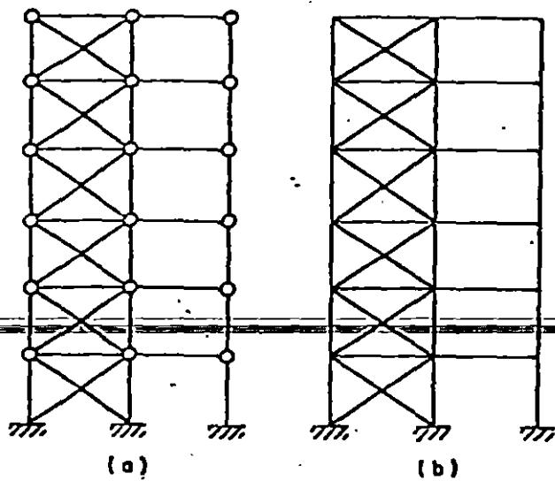
FIG. 3 Marcos contraventados
