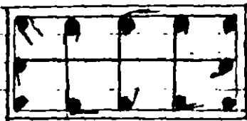
Fig 10.12 Arreglos admisibles de refuerzo en columnas de marcos dúctiles de concreto
