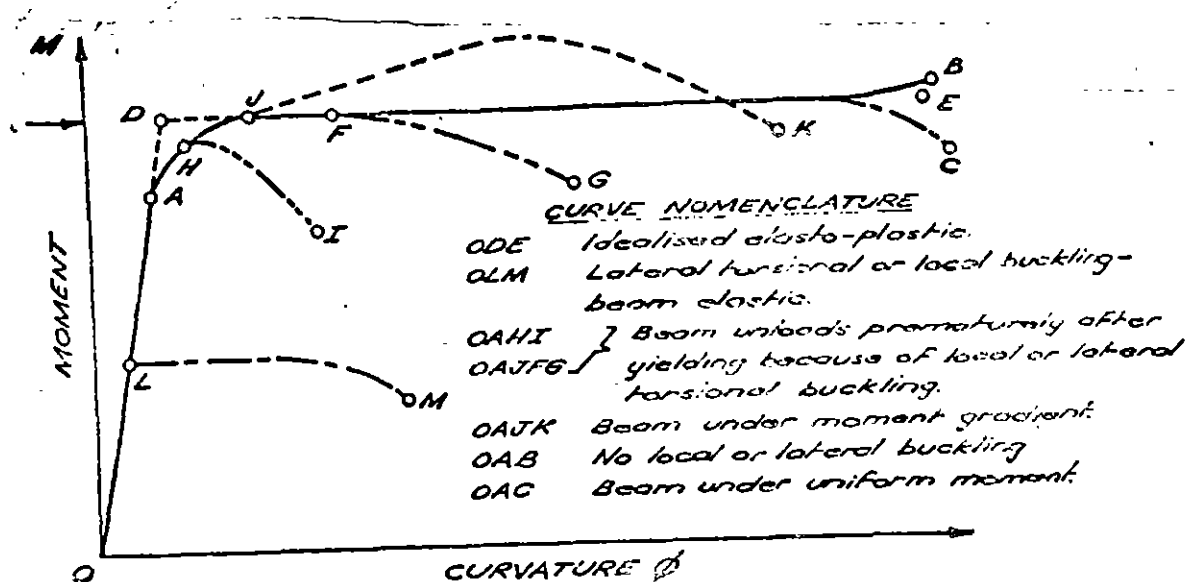
a) Vigas
