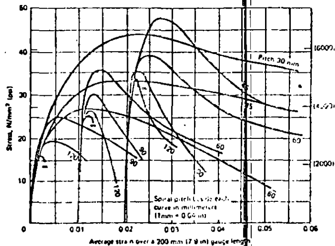
c) Curvas esfuerzo deformación de cilindros de concreto reforzados con hélices 6.5 mm de diámetro, de acero grado estructural y distintos espaciamentos
