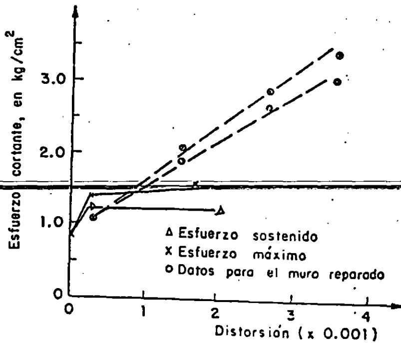
Fig 13. Envolventes de esfuerzos del muro 8.
