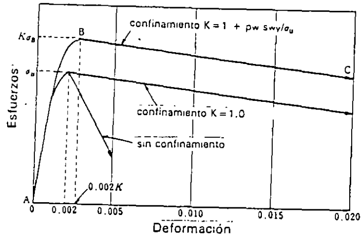
Fig. 5 Relación esfuerzo-deformación del concreto confinado [3]
