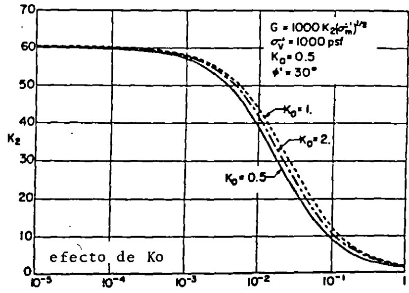
FIG. 23 INFLUENCIA DE VARIOS FACTORES SOBRE EL MODULO DE RIGIDEZ AL CORTANTE DE ARENAS. (SEED E IDRISSE, 1970)
