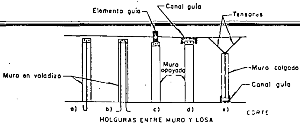
Fig 38. Posibles soluciones a muros que no forman parte integrante de la estructura
