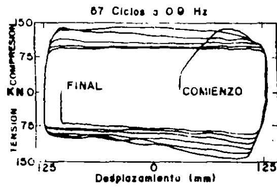
Fig. 23 Comportamiento histerético del dissipador por extrusión
