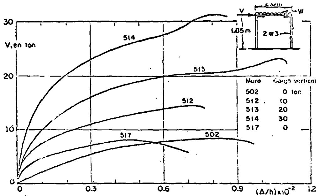
Muros de bloque de concreto. Fallo en flexión. Efecto de la carga vertical
