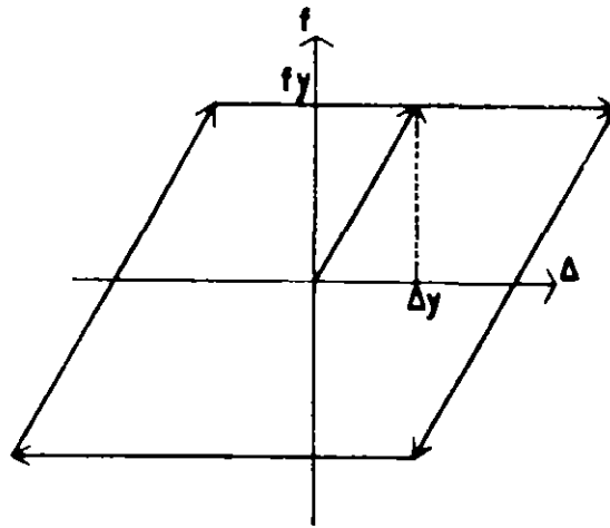
Fig. 1 Comportamiento elastoplástico
