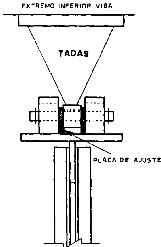
-Fig 16 Dispositivo Tadas
