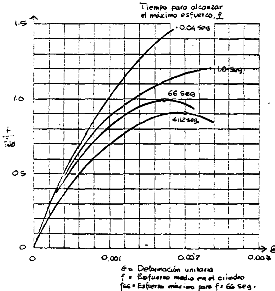
Fig 6 EFECTO DE LA VELOCIDAD DE CARGA (Hatakeyama 21 )
