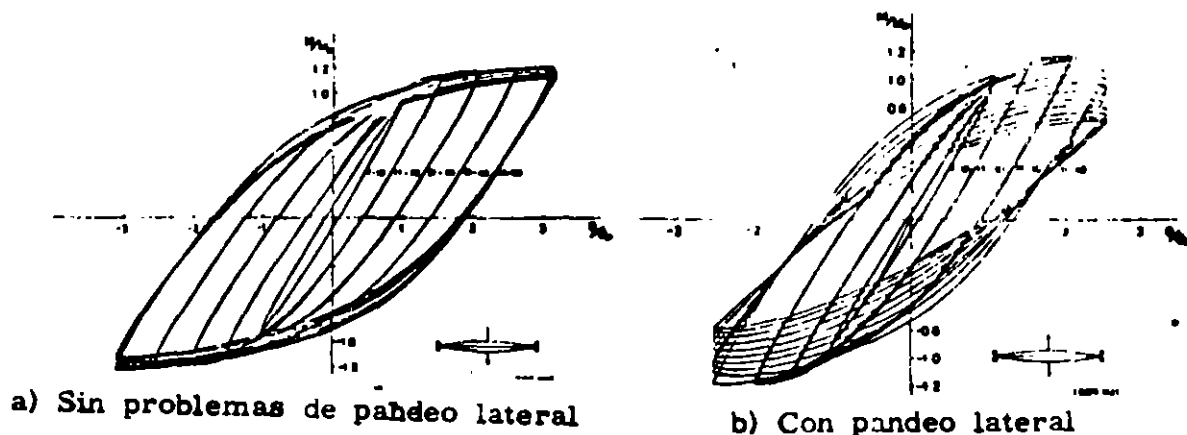
Fig 21 Comportamiento histerético de elementos de acero estructural
