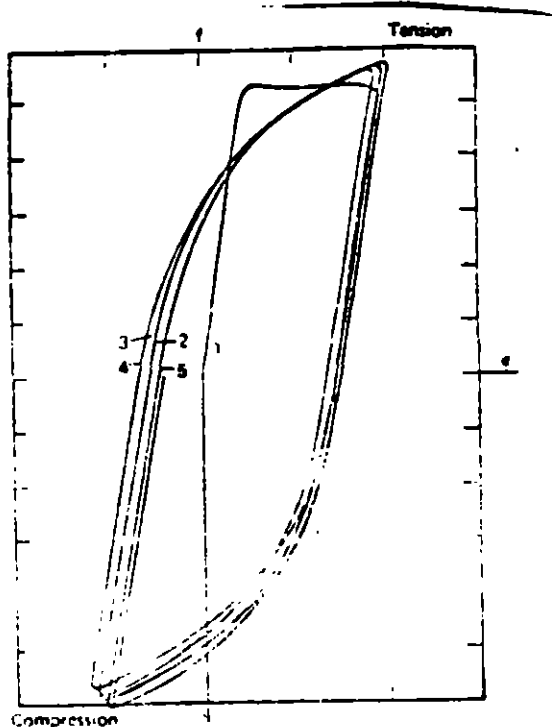
Fig 10 Ciclos histéricos en una barra de refuerzo
