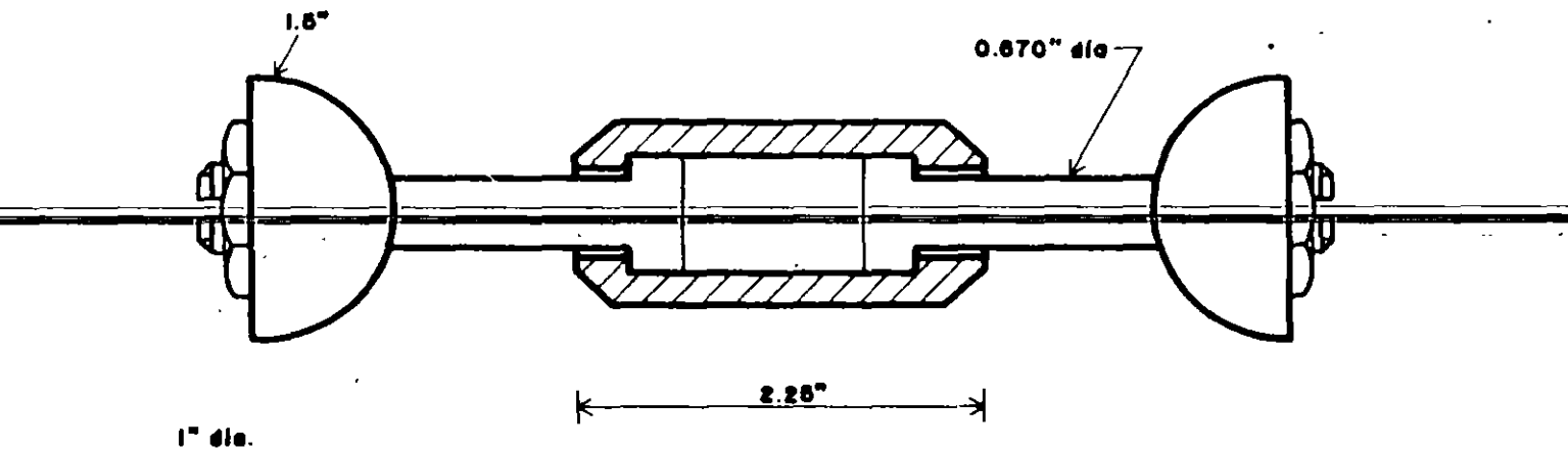
Fig. 34 Aislador de base con dispositivo para tomar tensiones
