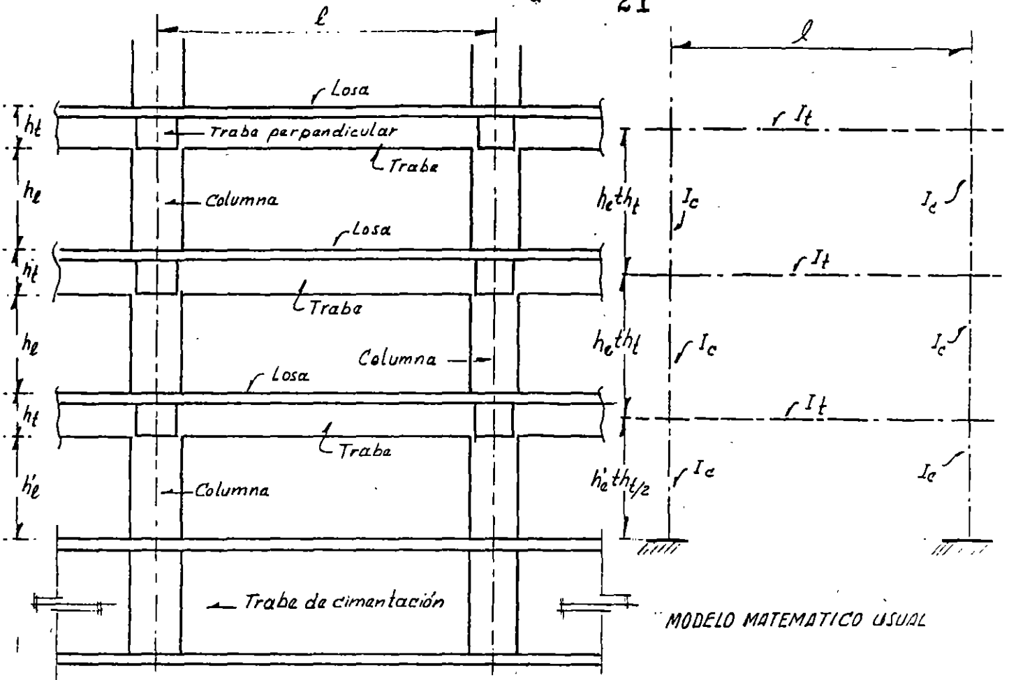
ESTRUCTURA REAL
