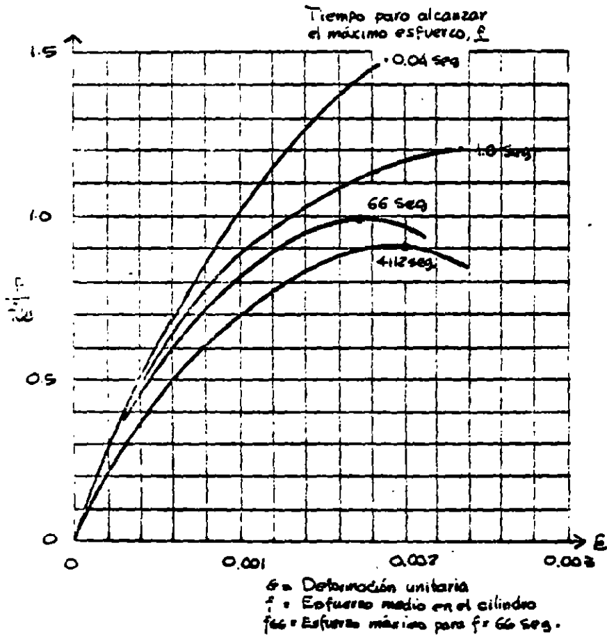
Fig 6 EFECTO DE LA VELOCIDAD DE CARGA (Hatchuo 71 )
