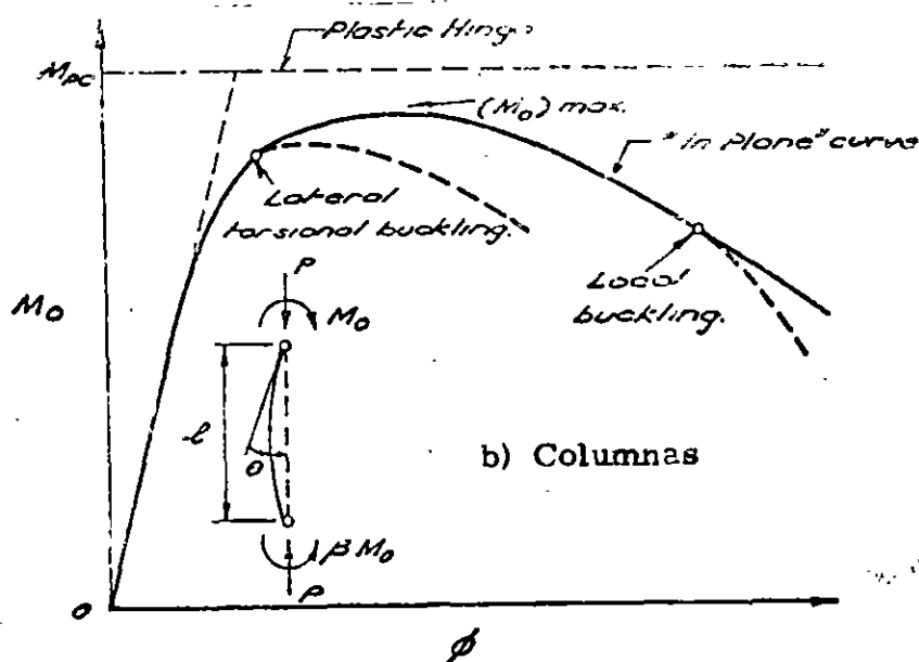
Fig 20 Relaciones momento-curvatura idealizadas en elementos de acero estructural
