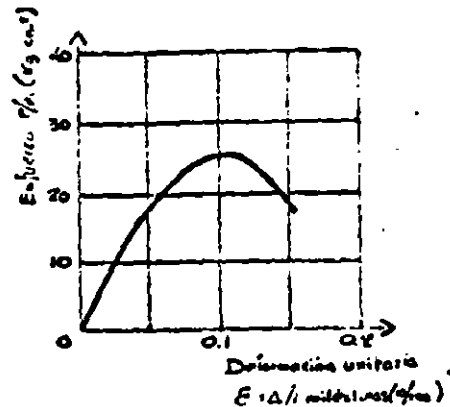
CURVA ESFUERZO-DEFORMACION DEL CONCRETO EN TENSION
