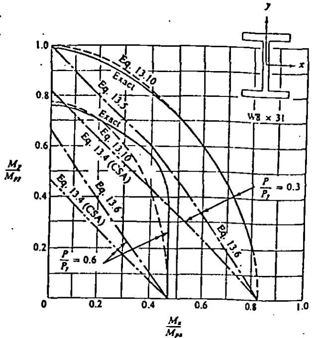
CURVAS DE INTERACCIÓN PARA COLUMNAS DE LONGITUD NULA.
