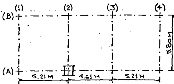
PLANTA, EJES Y ORIENTACIÓN COLUMNAS
