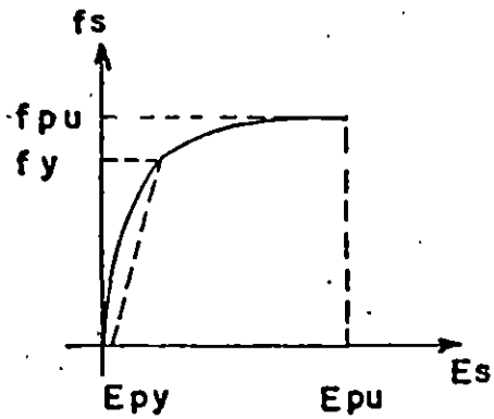
Acero de presfuerzo
