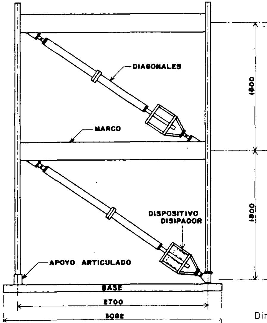
Elevación longitudinal
