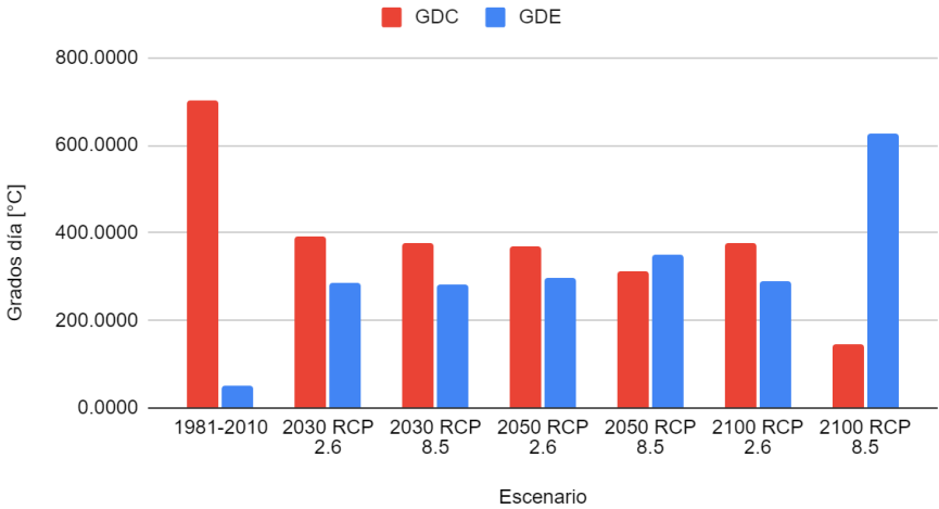
Grados Día Cuernavaca
