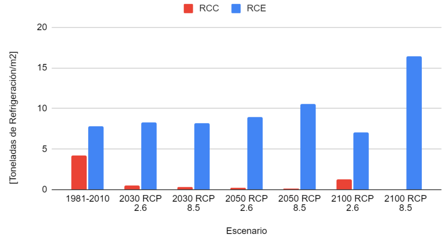
Requerimientos de Climatización Villahermosa
