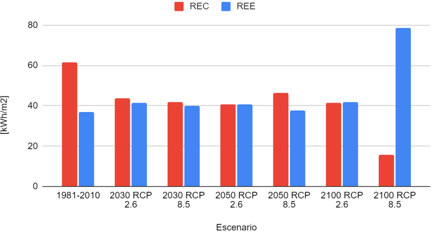
Gráfico 30 - Comparativo de los requerimientos energéticos en Hermosillo
