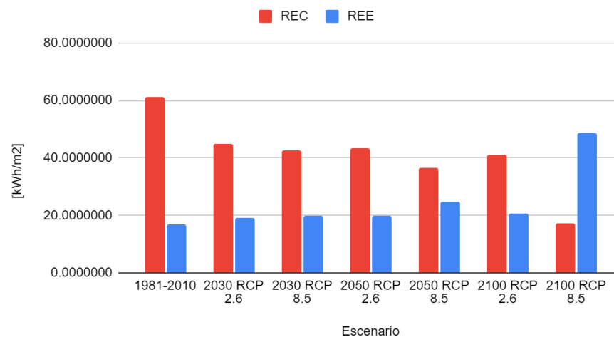
Gráfico 34 - Comparativo de los requerimientos energéticos en Monterrey
