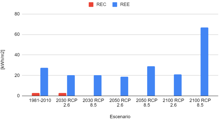
Gráfico 22 - Comparativo de los requerimientos energéticos en Acapulco
