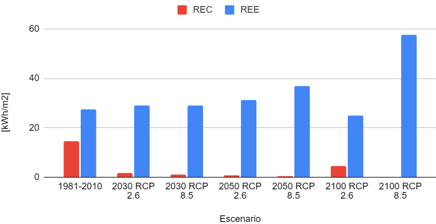
Requerimientos Energéticos para la Climatización Villahermosa
