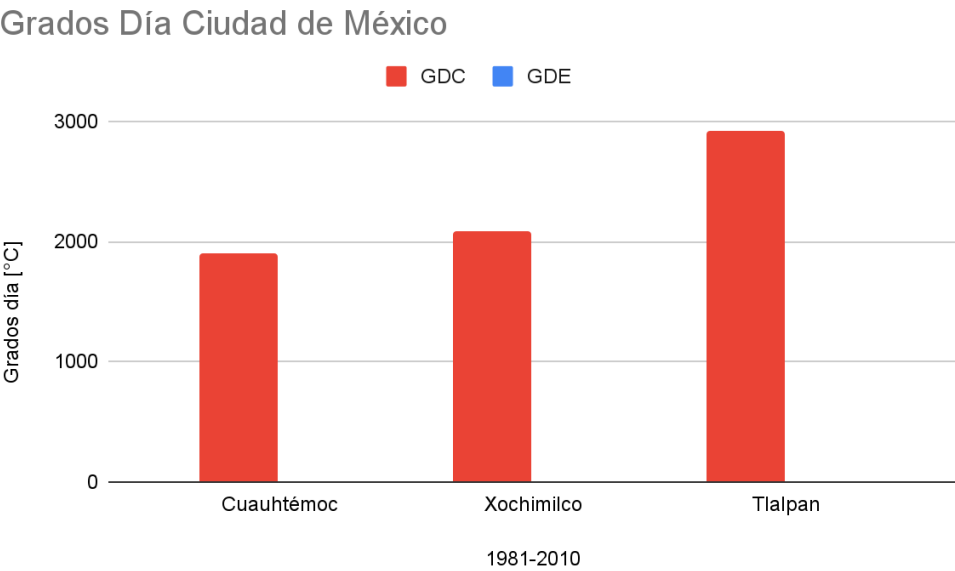
Figura 14 - Comparativo de los grados día anuales en [°C] de la Ciudad de México en la época actual (1980-2010). Fuente: Elaboración propia
