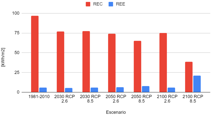
Gráfico 6 - Comparativo de los requerimientos energéticos en Guadalajara
