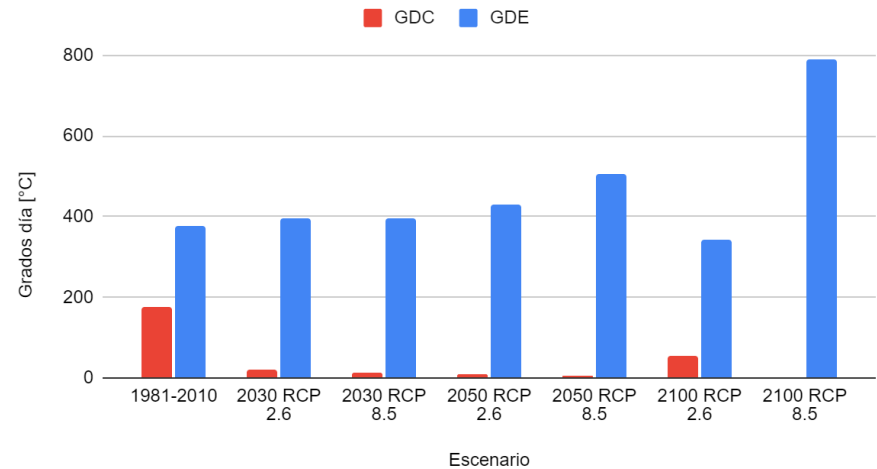
Grados Día Villahermosa
