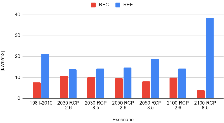
Gráfico 10 - Comparativo de los requerimientos energéticos en Cancún
