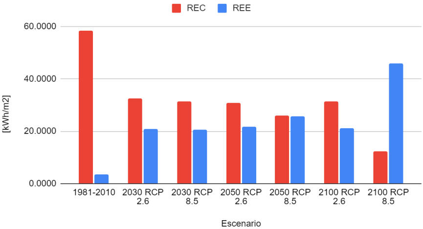
Requerimientos Energéticos para la Climatización Cuernavaca
