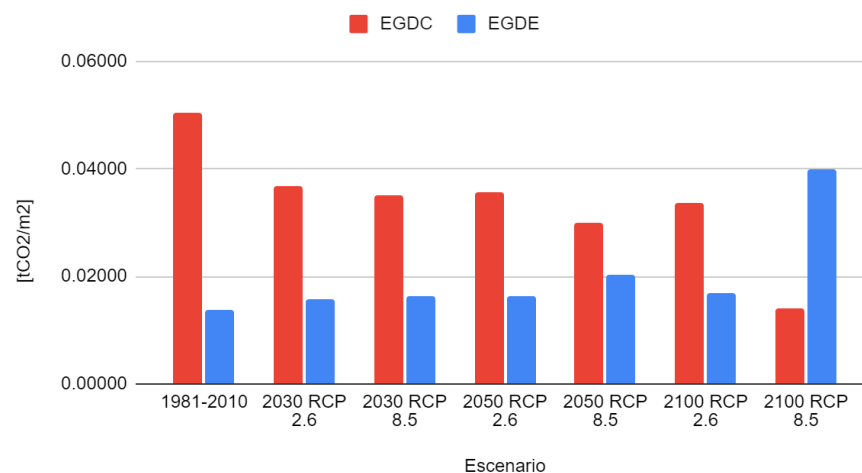
Gráfico 35 - Comparativo de las emisiones de CO 2 relacionadas con el uso de la energía en Monterrey
