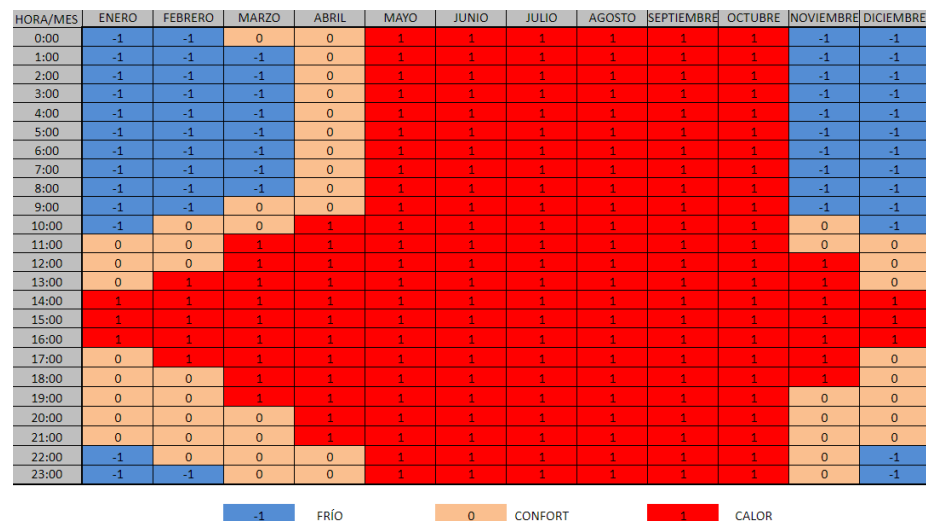
Figura 95 - Estudio del bioclima de Monterrey. 2100 - RCP 8.5
