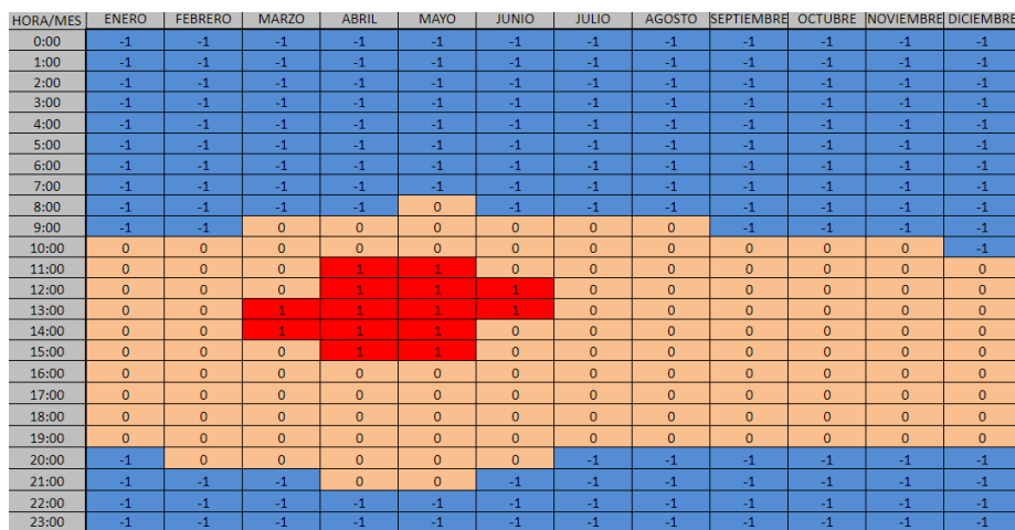
Figura 47 - Estudio del bioclima de Cuernavaca. Época actual (1980-2010)
