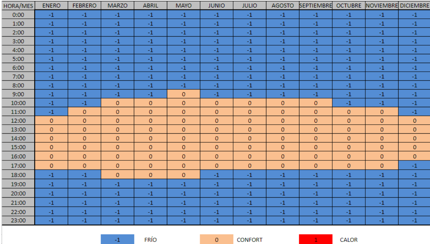
Figura 7 - Diagrama del estudio del bioclima de la Ciudad de México (1980-2010). Fuente: Biosol (2013)
