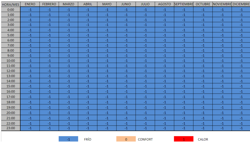
Figura 31 - Estudio del bioclima de la alcaldía Tlalpan. Época actual (1980-2010)
