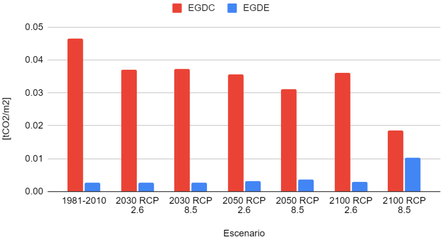
Gráfico 7 - Comparativo de las emisiones de CO 2 relacionadas con el uso de la energía en Guadalajara
