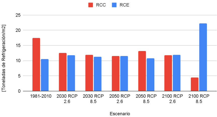
Gráfico 29 - Comparativo de los requerimientos de climatización en Hermosillo
