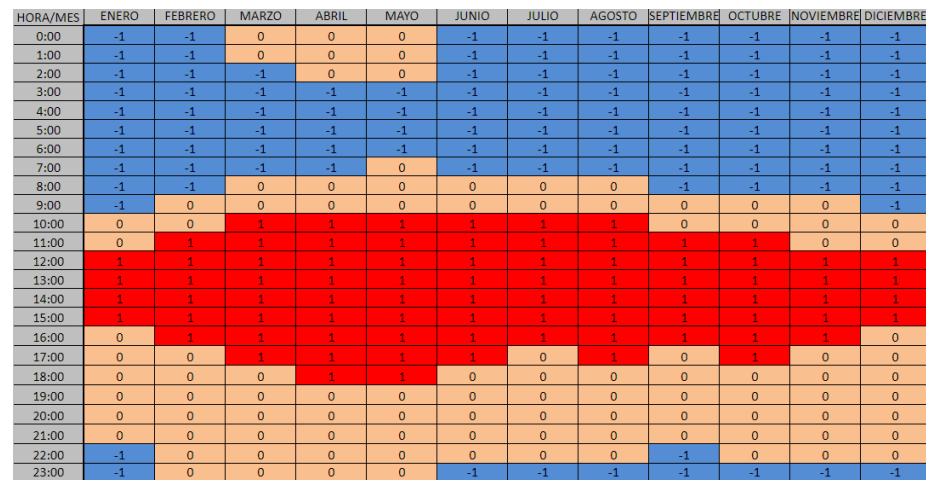
Figura 49 - Estudio del bioclima de Cuernavaca. 2030 - RCP 8.5
