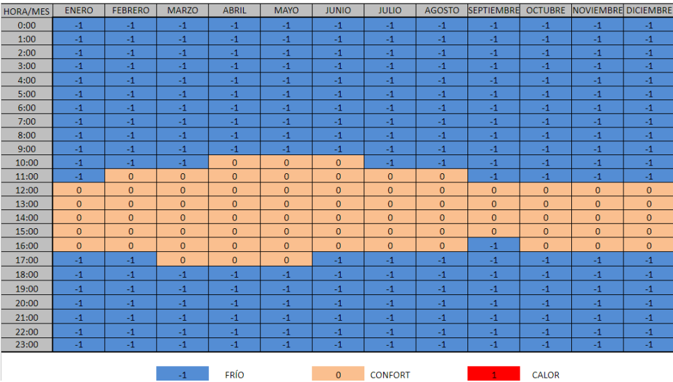
Figura 32 - Estudio del bioclima de la alcaldía Xochimilco. Época actual (1980-2010)
