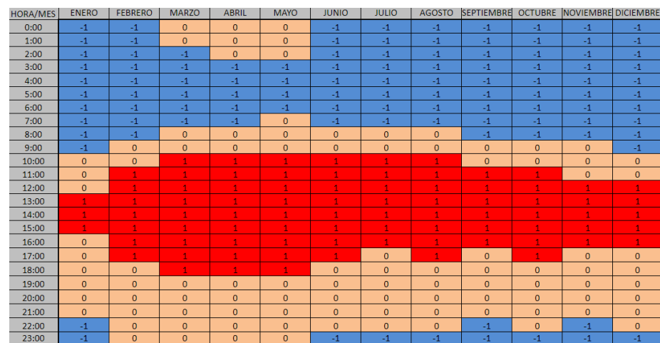
Figura 50 - Estudio del bioclima de Cuernavaca. 2050 - RCP 2.6
