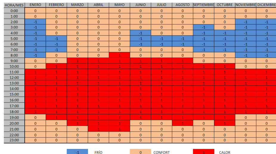
Figura 53 - Estudio del bioclima de Cuernavaca. 2100 - RCP 8.5
