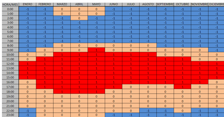
Figura 48 - Estudio del bioclima de Cuernavaca. 2030 - RCP 2.6
