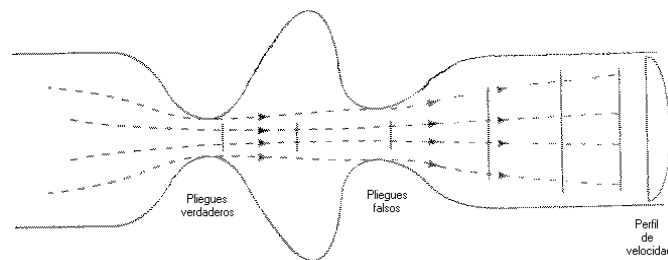
Figura 25: Modelo clásico de propagación uniforme
