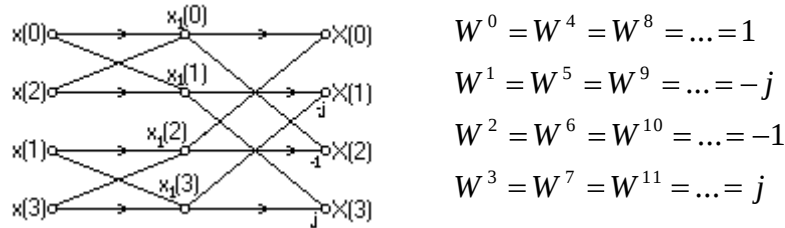
Figura 58: Mariposa para FFT con N = 4
