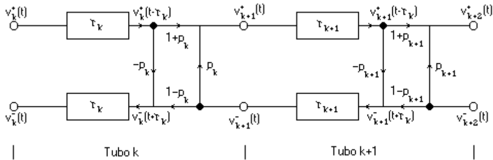
Figura 32: Diagrama de flujo de dos tubos sin pérdidas
