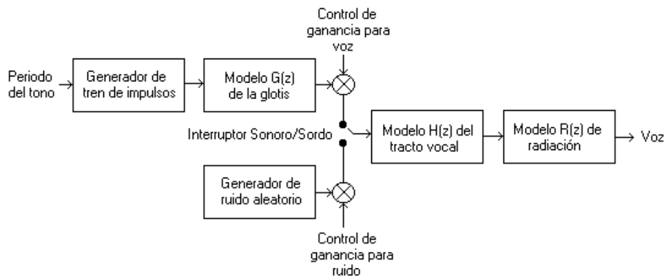
Figura 36: Modelo general discreto para producción de voz
