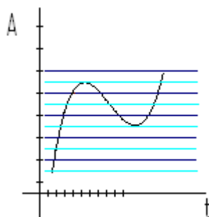
Figura 23: Cuantificación mejorada
