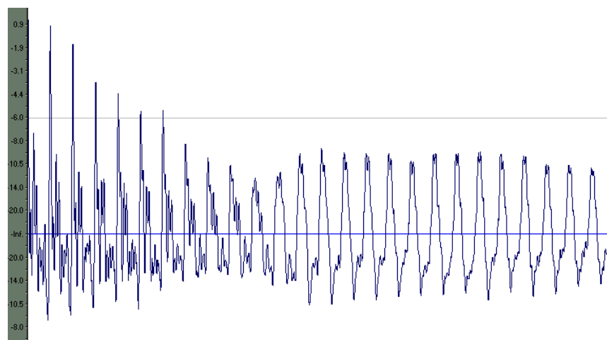
Figura 2: Sonido complejo
