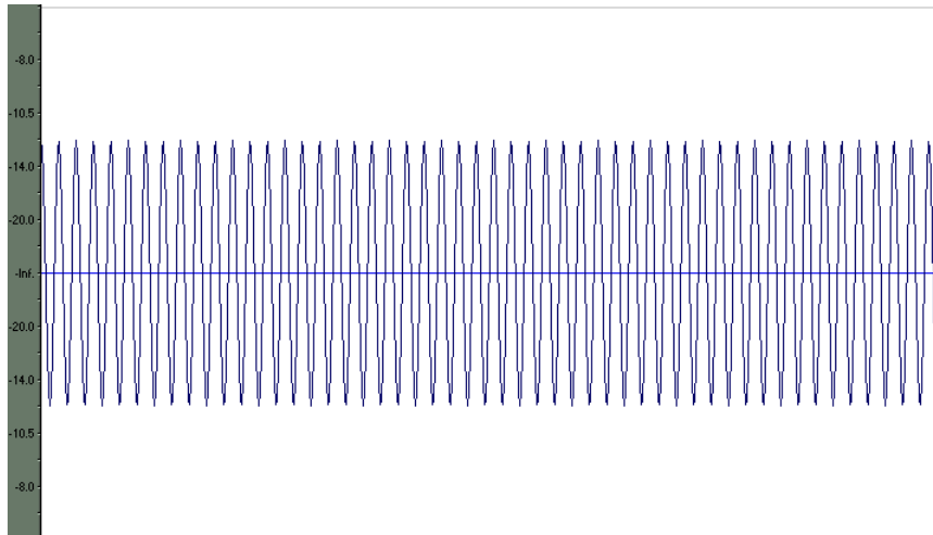
Figura 1: Sonido simple
