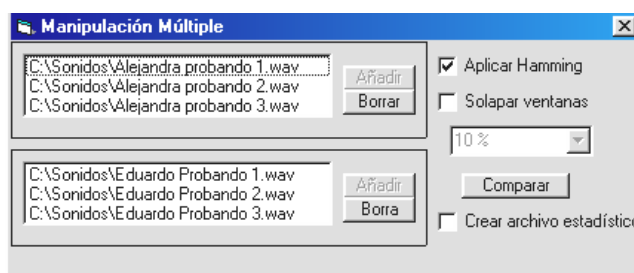
Figura 83: Manipulación Múltiple
