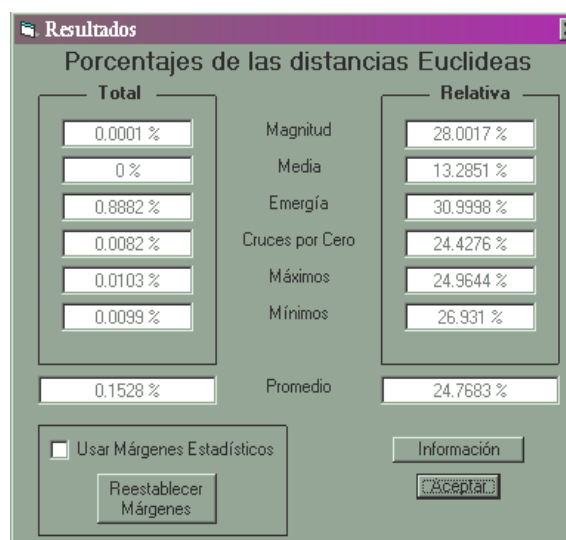
Figura 78: Comparación Analítica
