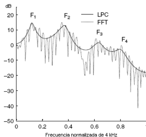
Figura 61: Envolvente
