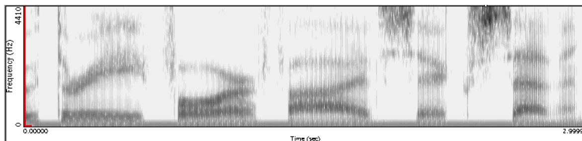
Figura 65: Sonograma
