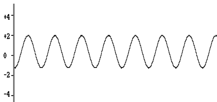
Figura 6: Señal senoidal de 100 Hz
