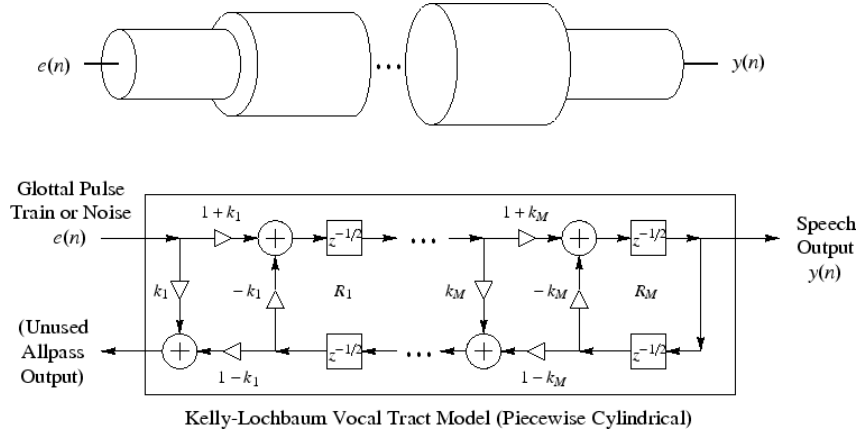
Figura 33: Modelo de 'n' tubos
