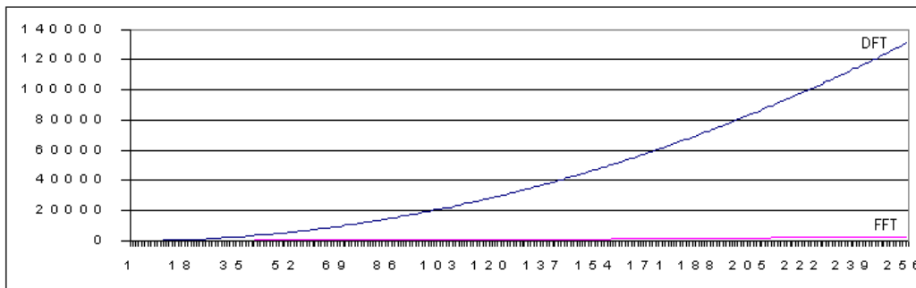
Figura 59: Número de operaciones en la DFT y FFT cuando varía ‘N’
