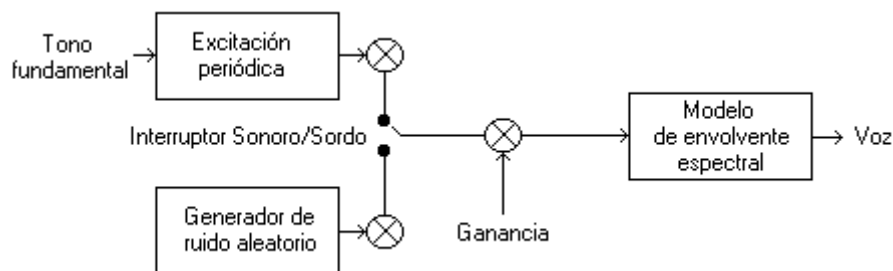
Figura 37: Modelo de un vocoder
