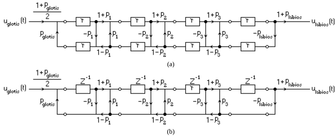
Figura 35: Modelo simplificado y modelo en tiempo discreto
