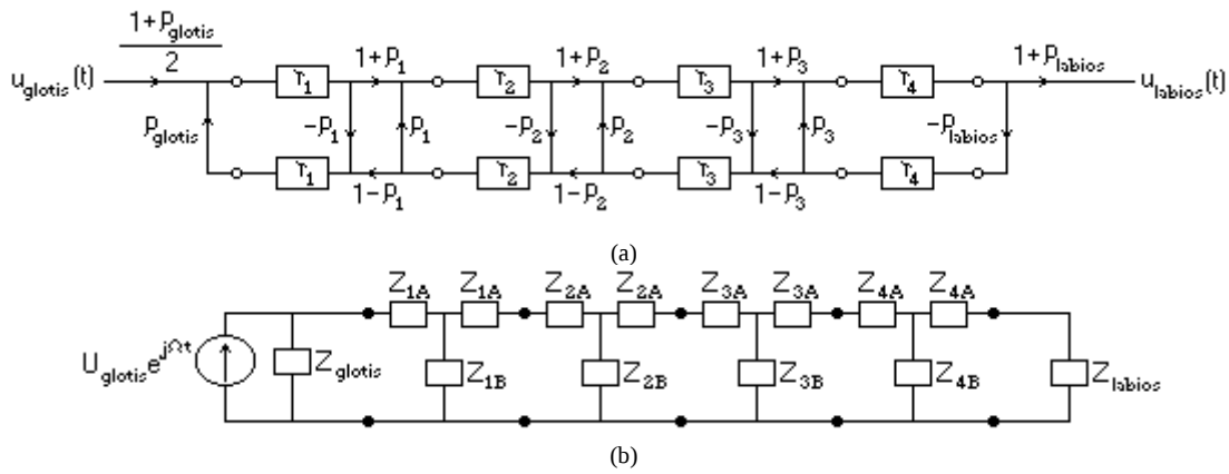
Figura 34: Diagrama de flujo de un modelo de cuatro tubos y su equivalente en una línea de transmisión
