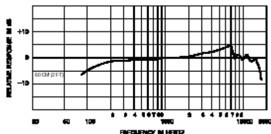
Patrón de captación y respuesta en frecuencia
