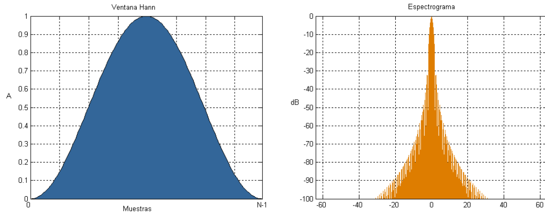
Figura 50: Ventana Hann
