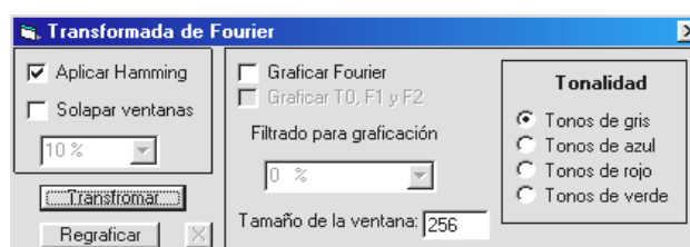
Figura 87: Transformada de Fourier
