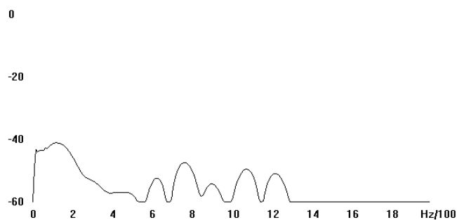
Figura 62: Espectrograma
