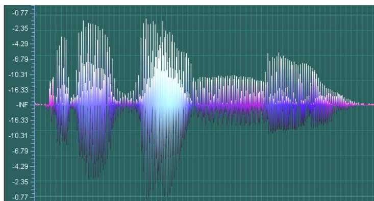
Figura 98: Sonógrama de la palabra “probando”
