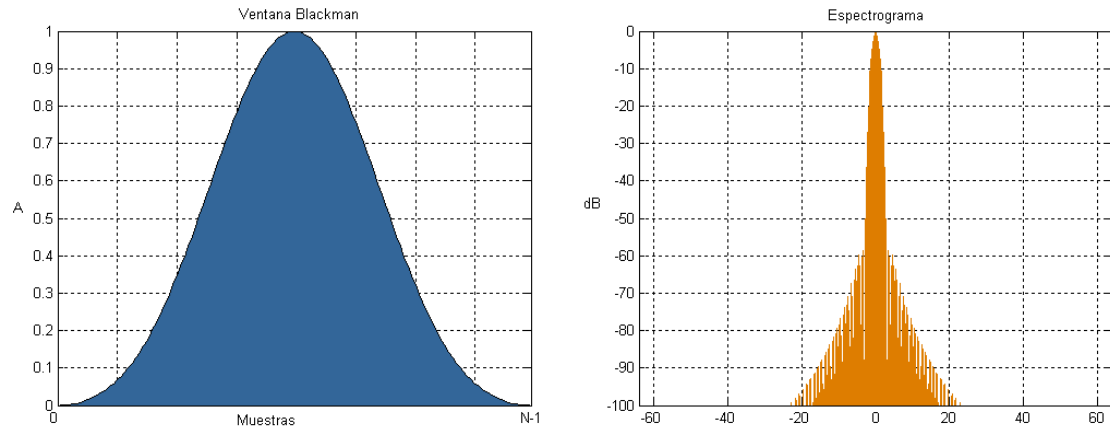
Figura 51: Ventana Blackman
