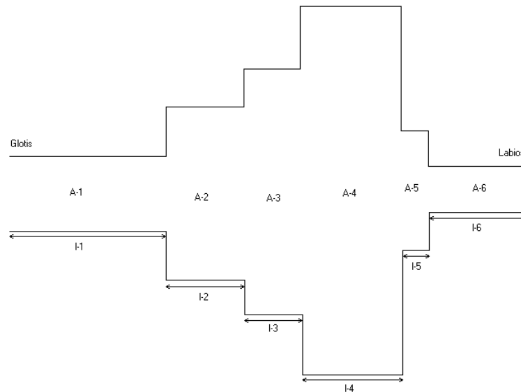
Figura 29: Modelo de seis tubos
