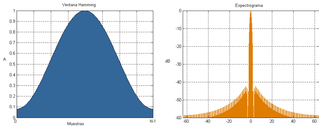
Figura 49: Ventana Hamming
