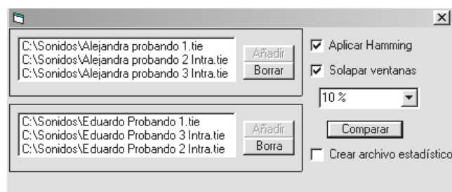
Figura 84: Archivos procesados
