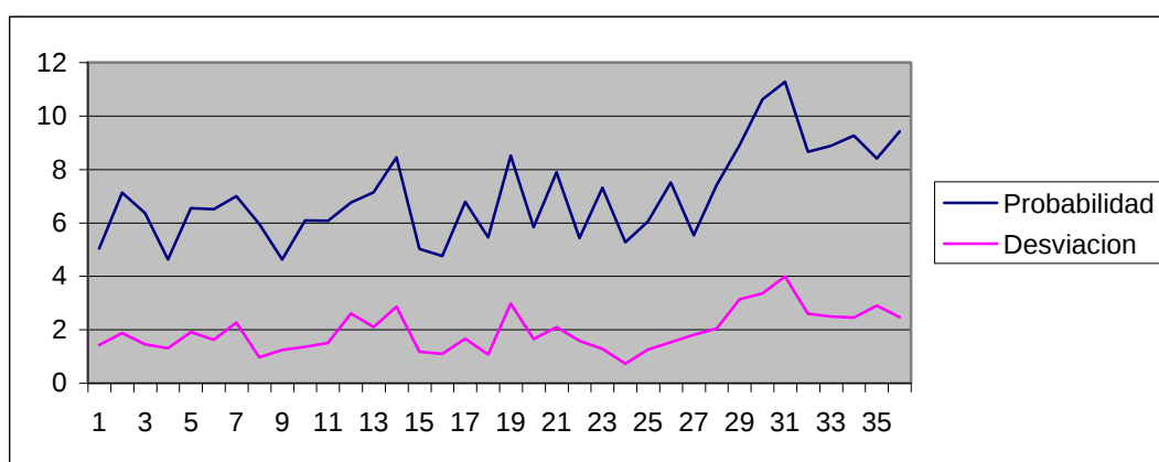
Figura 108: Grafica de las diversas configuraciones
