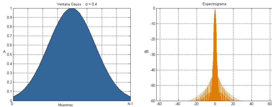
Figura 52: Ventana Gauss
