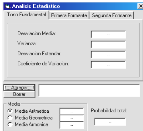
Figura 91: Análisis Estadístico
