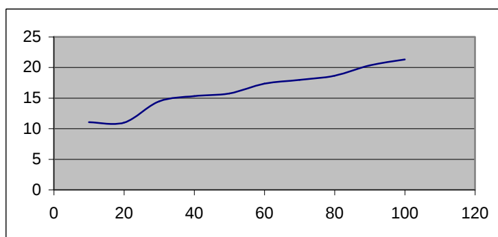
Figura 107: Aumento de la distancia por desplazamiento
