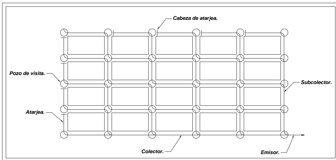
Figura 2.5 Trazo en Bayoneta.
