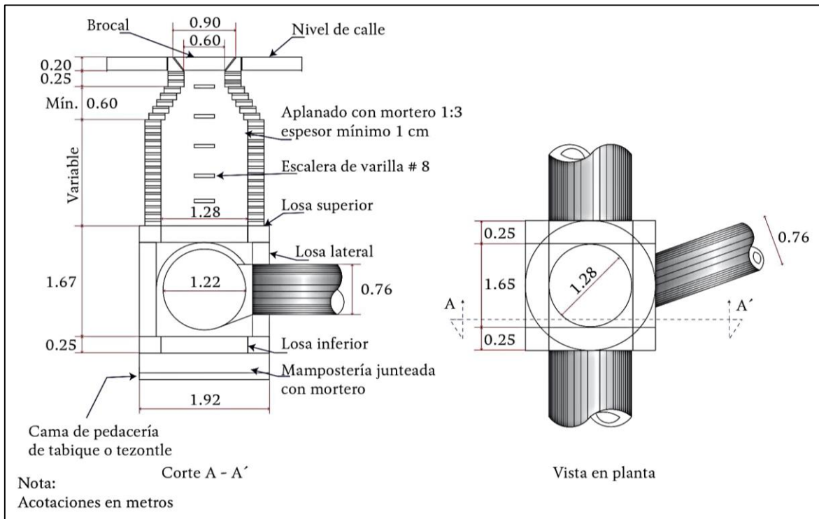
Imagen 3.4 Pozo caja.
