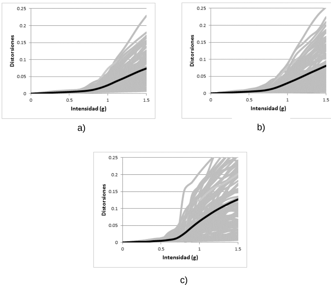
Figura A2.1. a) IDA 2004, b) IDA 1987, c) IDA 1977.
