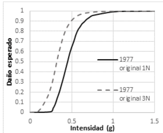
Figura 5.4.Comparación estructura RCDF-1977 uno y tres niveles.
