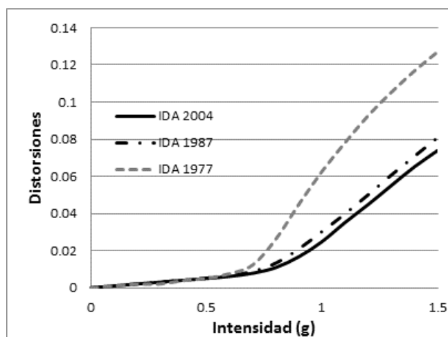
Figura A2.2. Comparación de las curvas IDA para las estructuras rigidizadas.
