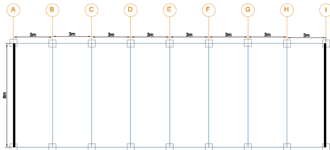
Figura 3.3. Vista en planta de la colocación de tensores tipo L.
