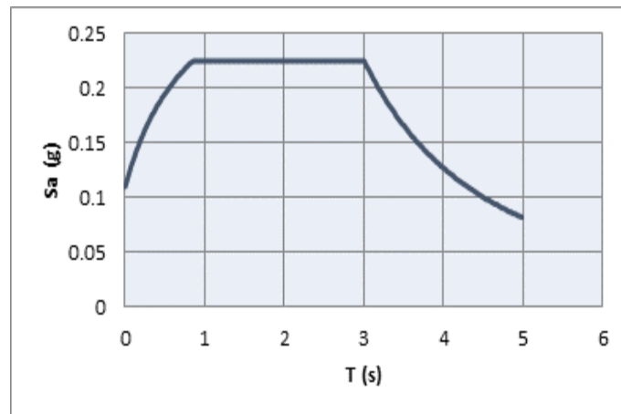
Figura 2.3 Espectro inelástico para diseño sísmico RCDF-2004.
