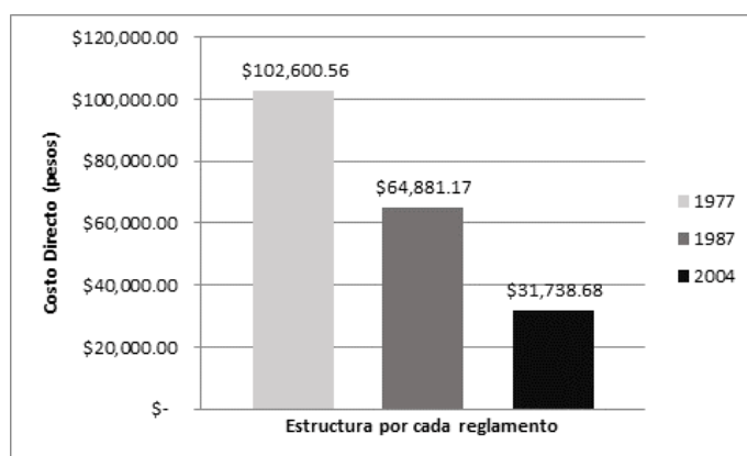
Figura 5.2.Costo directo de los tensores
