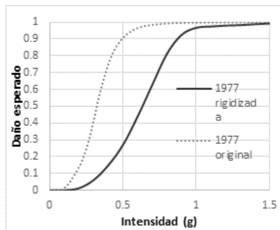
Figura 5.3.Comparación estructura RCDF-1977 original y rigidizada.
