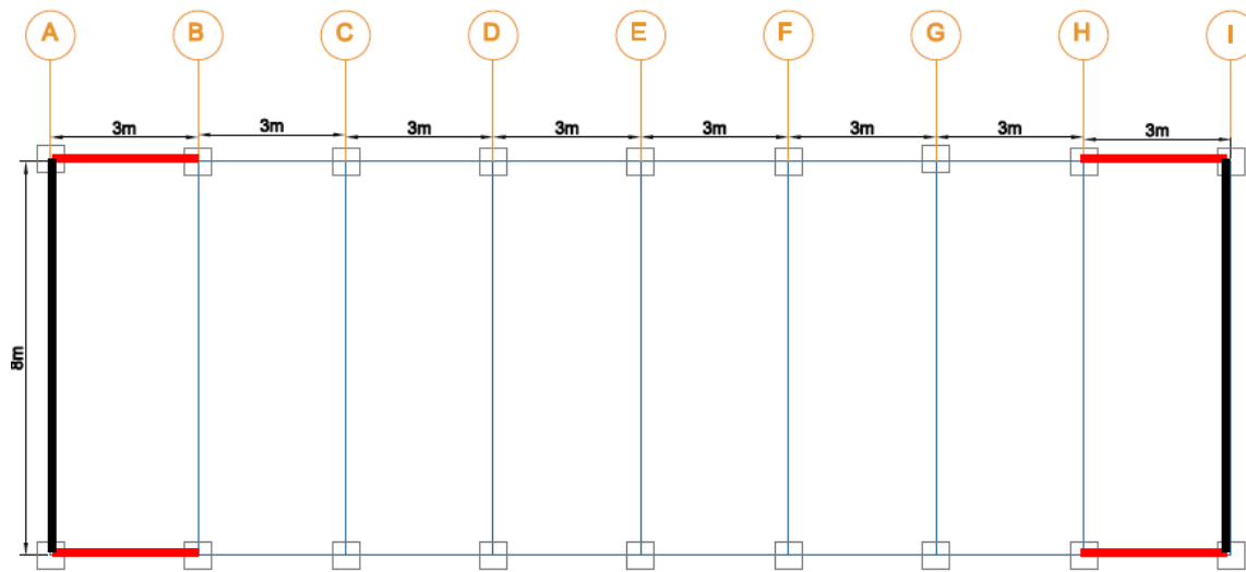
Figura 3.1 Vista en planta de la colocación de sensores tipo L.
