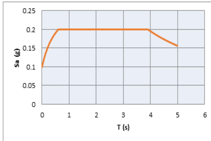
Figura 2.4 Espectro inelástico para diseño sísmico RCDF-1987
