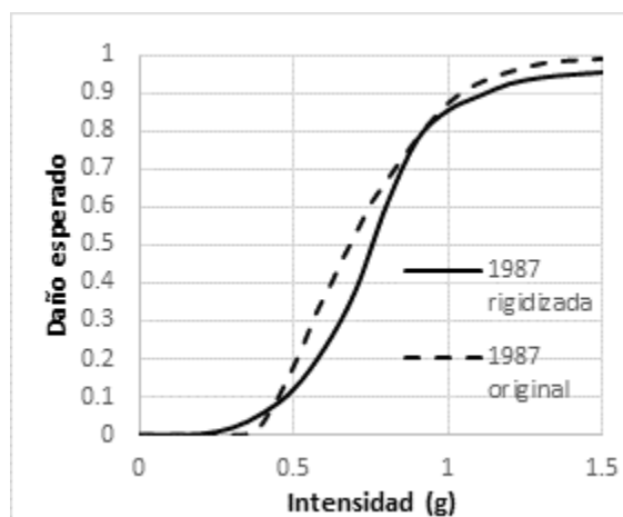
Figura 5.5.Comparación estructura RCDF-1987 original y rigidizada.
