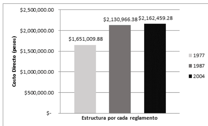
Figura 5.1.Costo directo de la estructuras RCDF-1977, RCDF-1987 y RCDF-2004.
