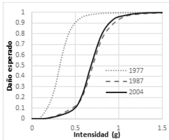
Figura 4.4 Comparación de curvas de vulnerabilidad obtenidas.
