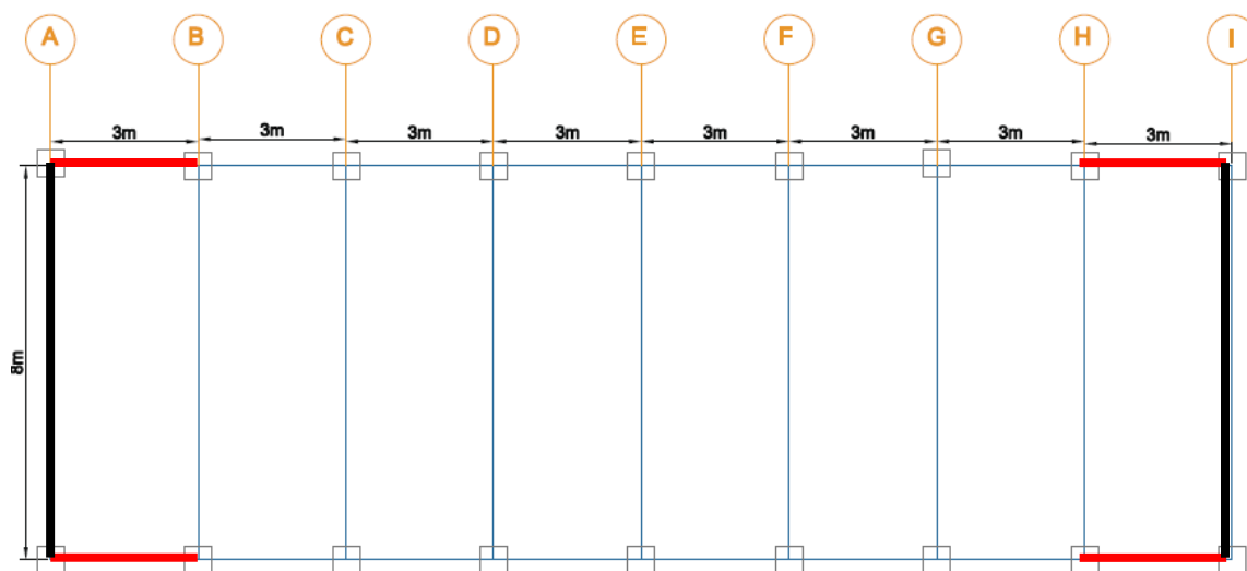
Figura 3.2. Vista en planta de la colocación de tensores tipo L.
