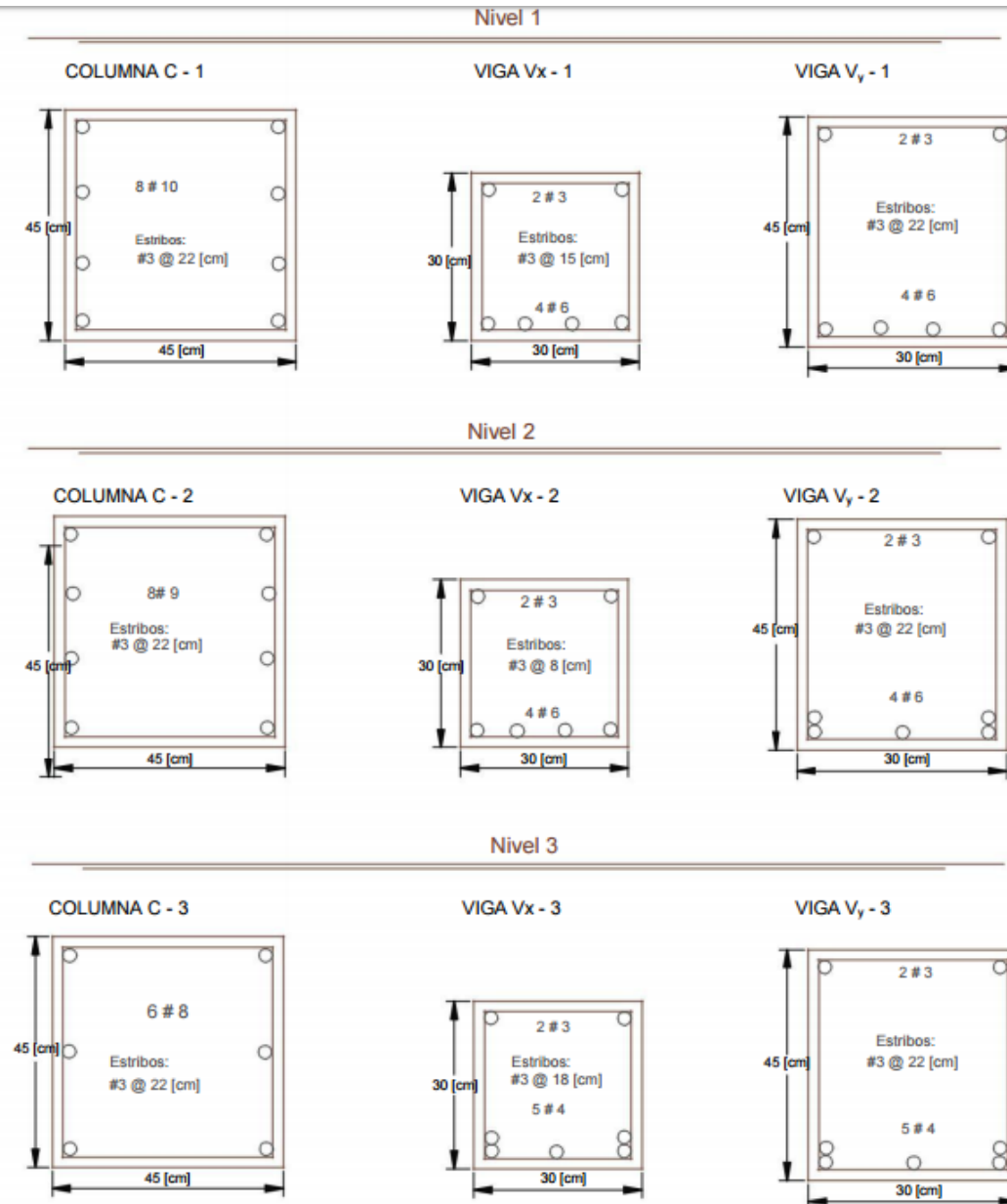
Figura 2.8 armados propuestos
