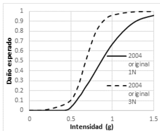
Figura 5.8.Comparación estructura RCDF-2004 uno y tres niveles.
