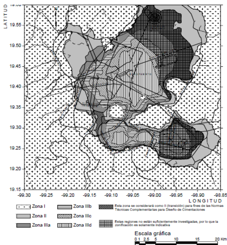
Figura 2.2 Zonificación Sísmica del Distrito Federal (GDF, 2004)
