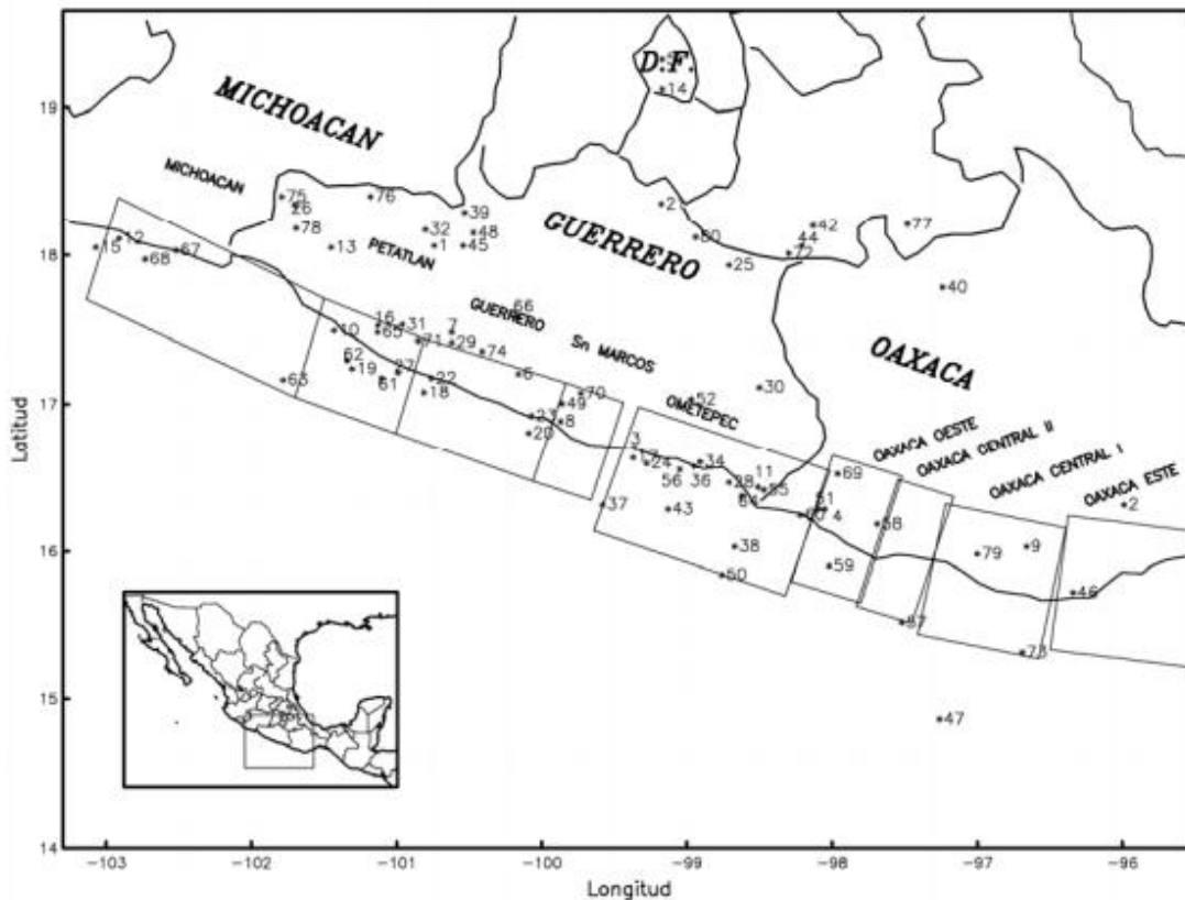
Figura 1.2. Epicentro de sismos que han afectado a la ciudad de México desde 1985, en la región de Michoacán, Guerrero y Oaxaca (Reinoso, 1994)
