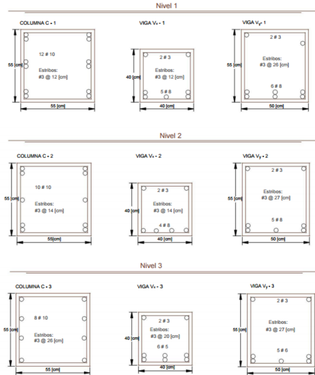
Figura 2.6 Armados propuestos.
