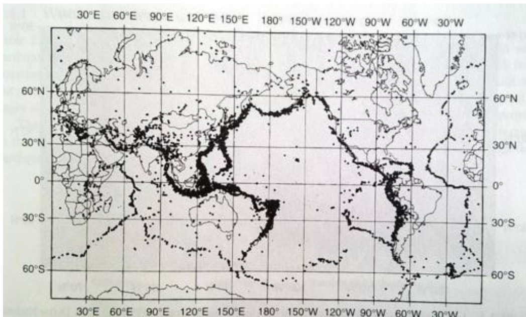
Figura 1.1 Ocurrencia de sismos obtenidos por Villaverde entre 1963 y 1988 (Villaverde, 2009).
