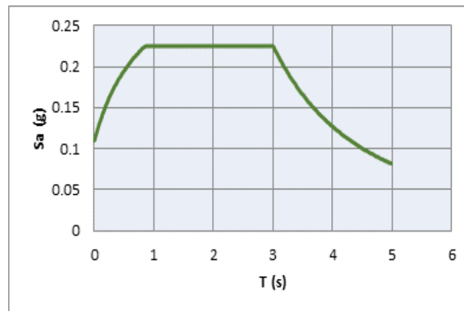
Figura 2.5 Espectro inelástico para diseño sísmico RCDF-1977
