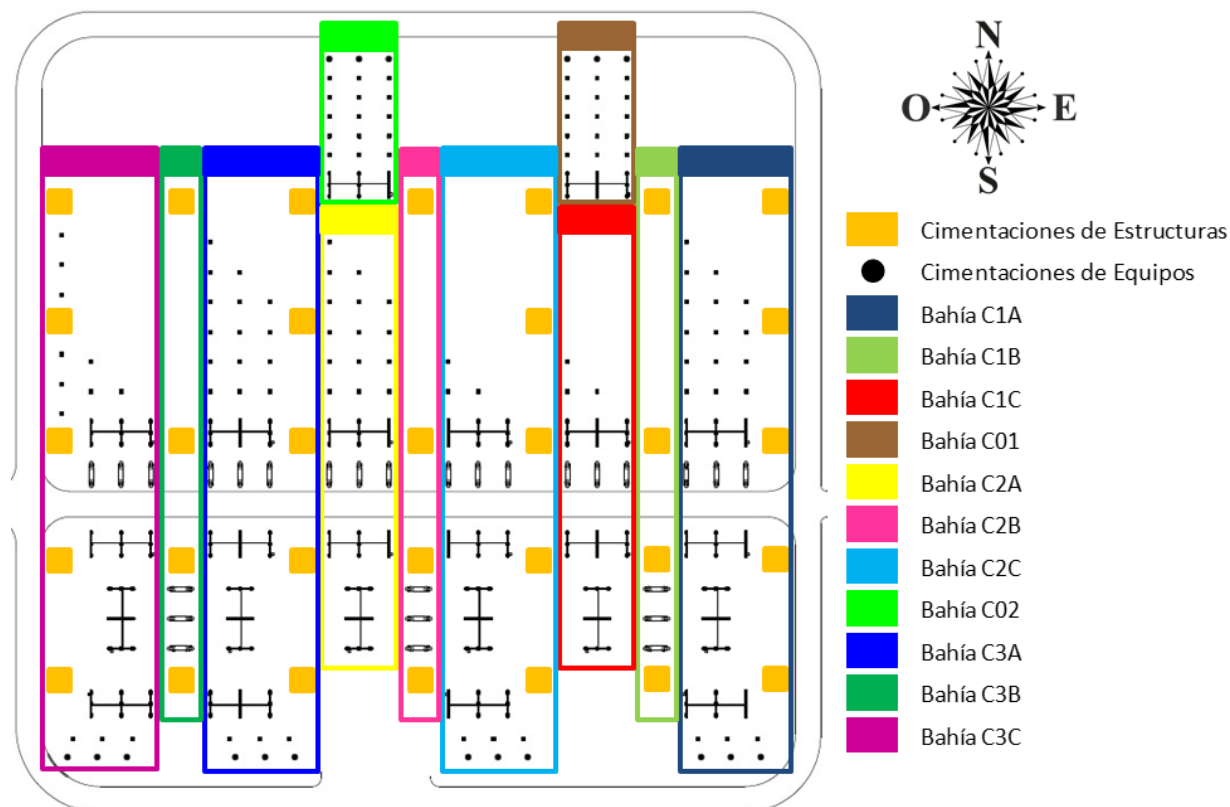
Figura 31 Plano de Cimentaciones de Bahías SE 39
