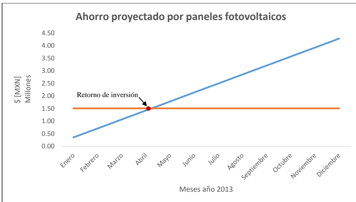
Figura 33. Ahorro proyectado por instalación de paneles fotovoltaicos para dar suministro al 11% del consumo.
