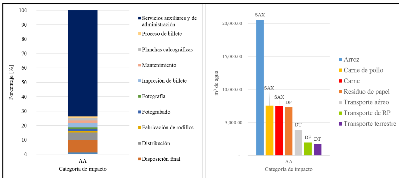
Figura 27. Resultados de impacto ambiental para la categoría de agotamiento de agua.
