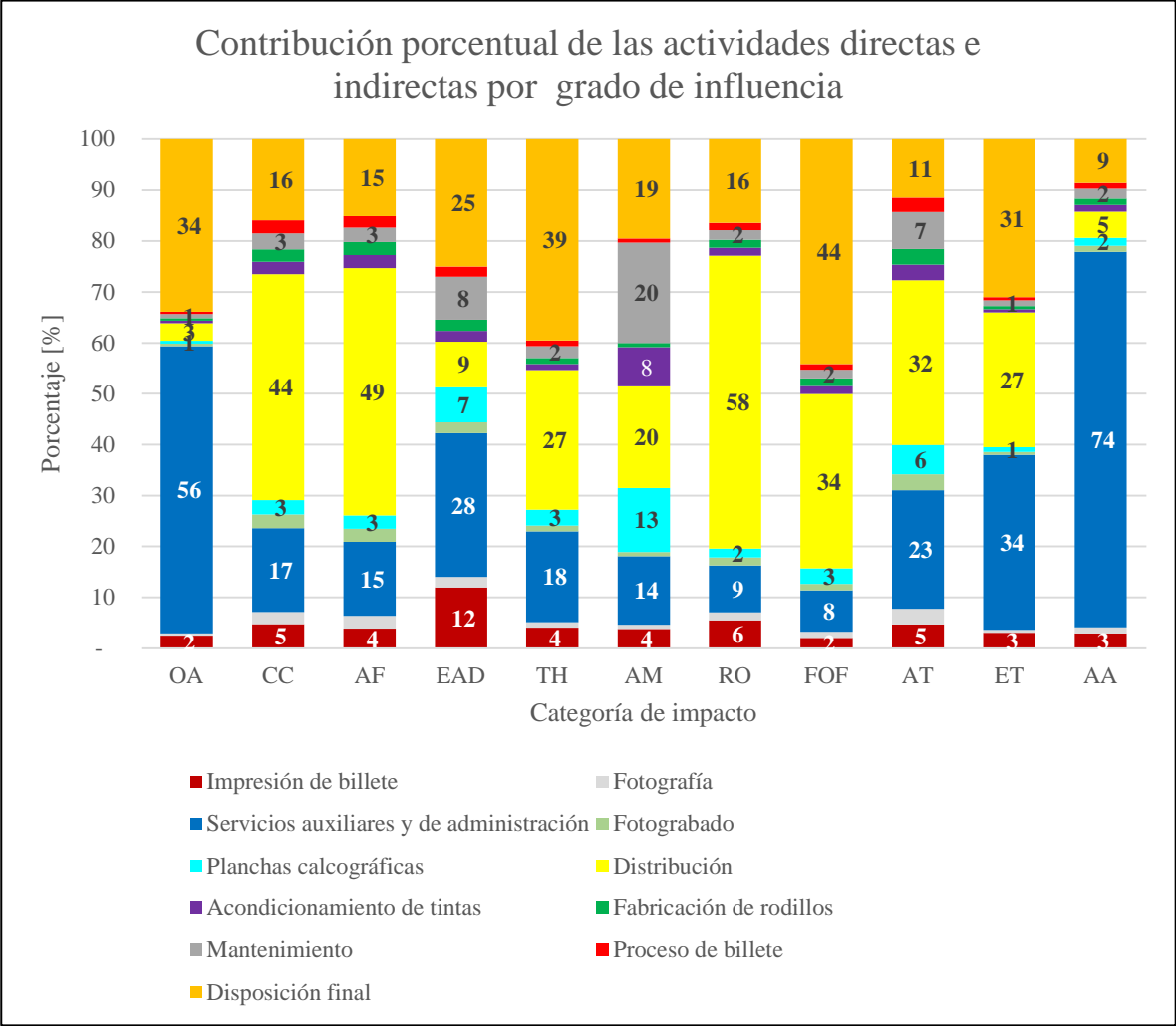
Figura 16. Impactos ambientales por áreas del Complejo Legaria.
