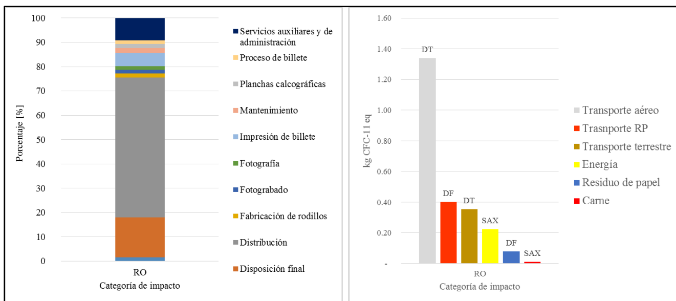
Figura 23. Resultados de impacto ambiental para la categoría de agotamiento de la capa de ozono. DT: distribución; DF: disposición final; SAX: servicios auxiliares y de administración.
