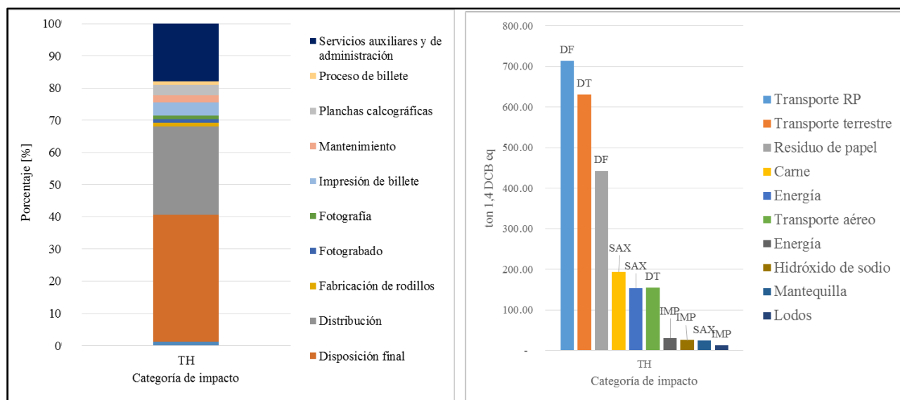
Figura 21. Resultados de impacto ambiental para la categoría de toxicidad humana. *DF: disposición final; DT: distribución; SAX: servicios auxiliares y de administración.
