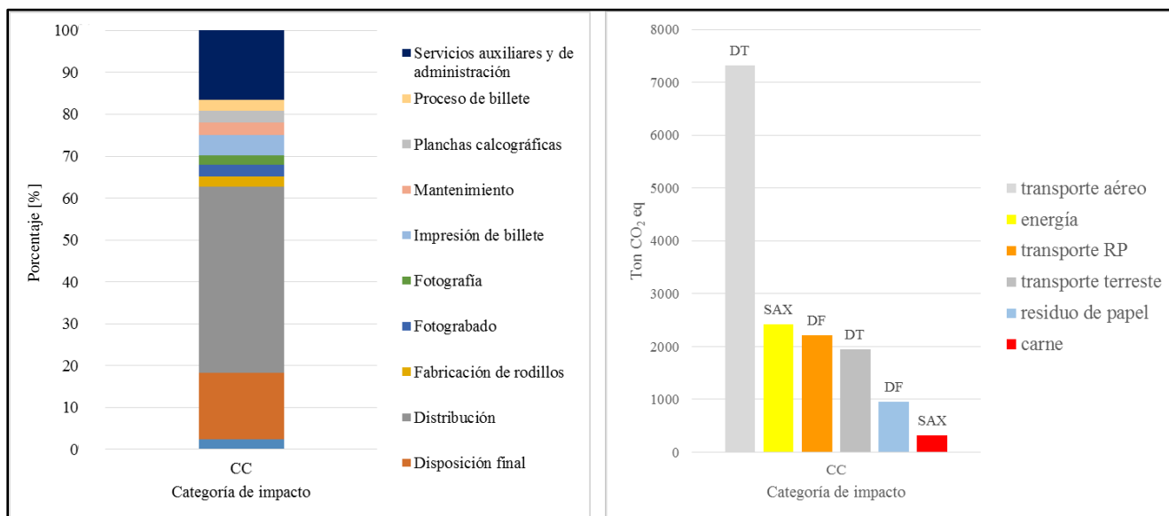
Figura 18. Resultados de impacto ambiental para la categoría de cambio climático
