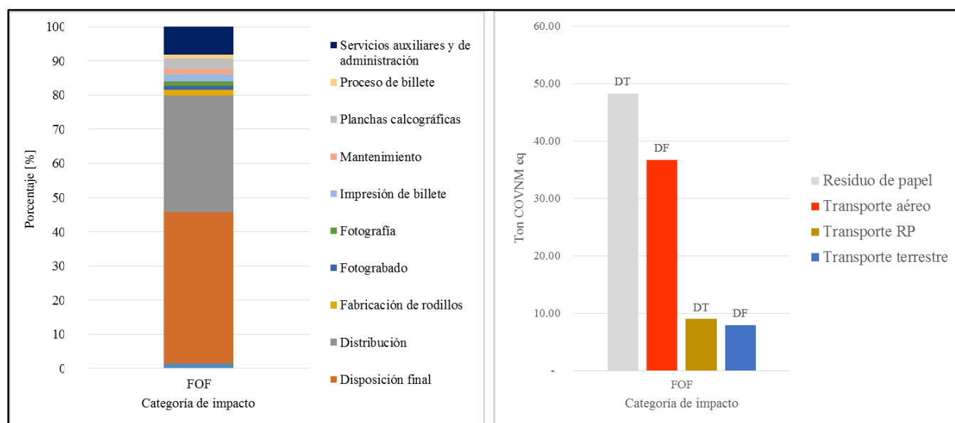
Figura 24. Resultados de impacto ambiental para la categoría de formación de oxidantes fotoquímicos.
