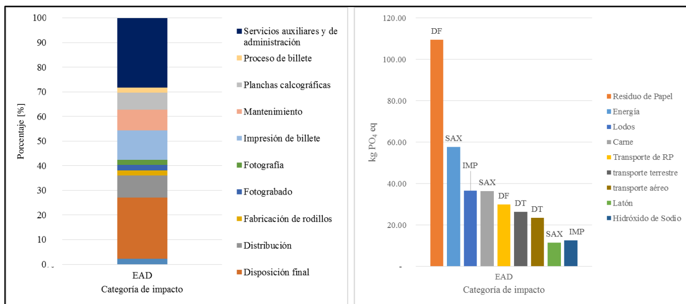
Figura 20. Resultados de impacto ambiental para la categoría de eutrofización de agua dulce.
