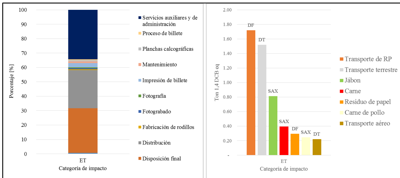
Figura 26. Resultados de impacto ambiental para la categoría de ecotoxicidad terrestre.
