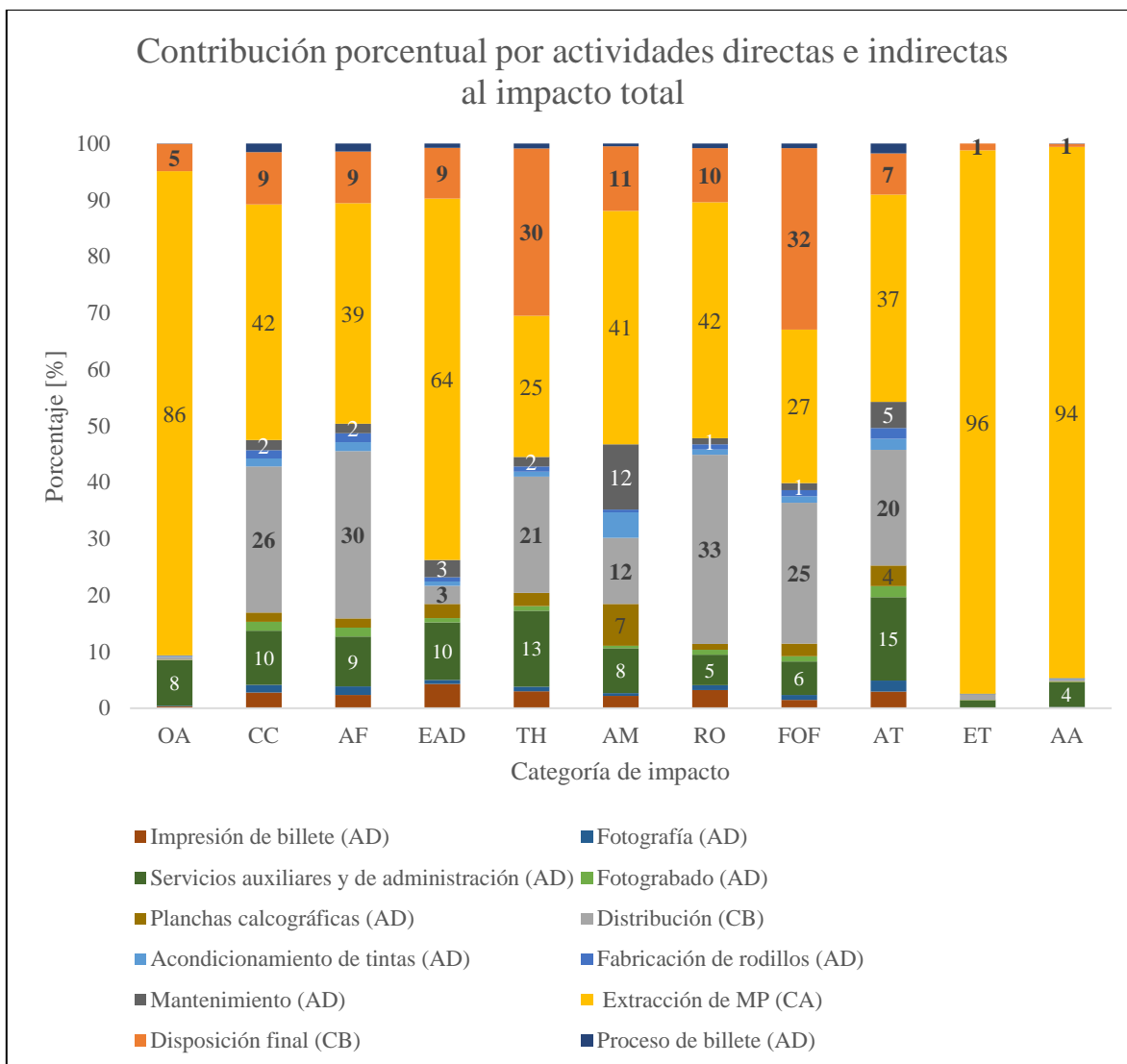
Figura 15. Impactos ambientales detallados por actividades directas e indirectas. *AD: actividades directas; CA: corriente arriba; CB: corriente abajo.
