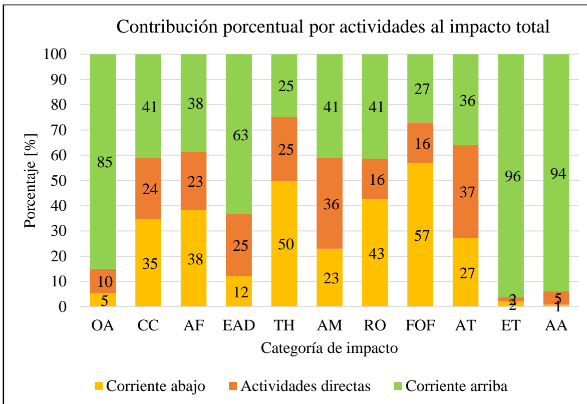
Figura 14. Impactos ambientales por actividades del Complejo Legaria.
