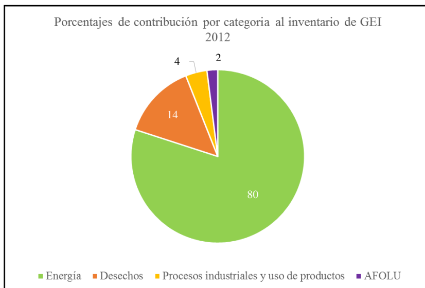
Figura 28. Contribución porcentual por categoría al inventario de GEI de la Ciudad de México en el año 2012. SEDEMA. (2012).
