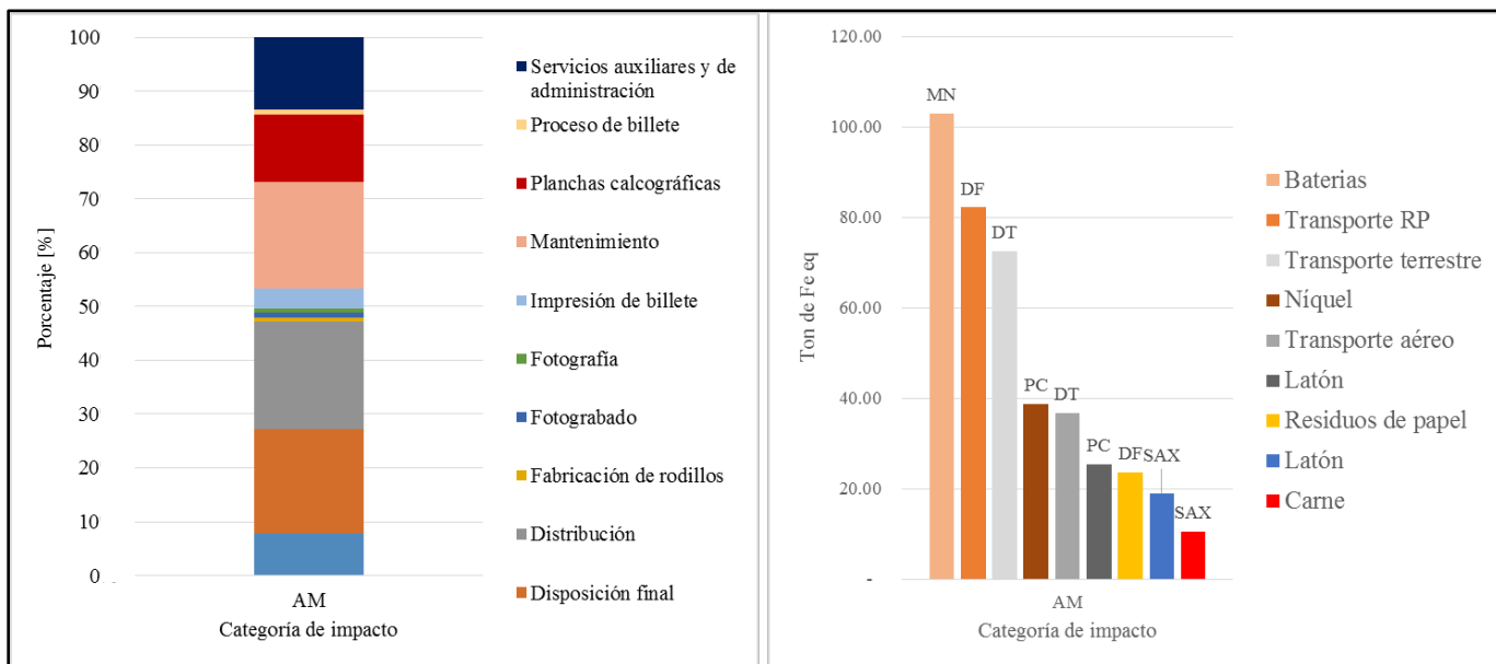
Figura 22. Resultados de impacto ambiental para la categoría de agotamiento de recursos minerales.
