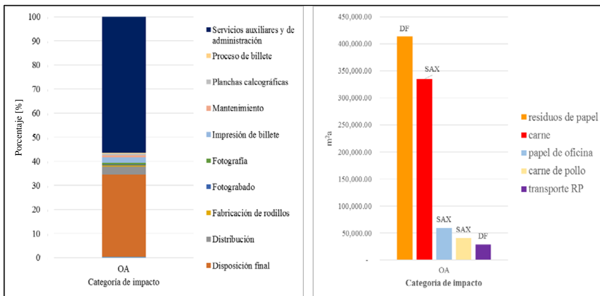
Figura 17. Resultados de impacto ambiental para la categoría de ocupación agrícola *DF: disposición final; SAX: servicios auxiliares y de administración
