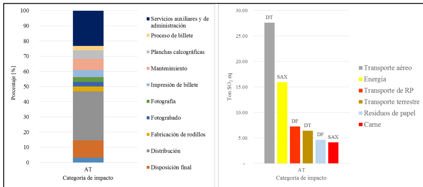
Figura 25. Resultados de impacto ambiental para la categoría de acidificación terrestre.
