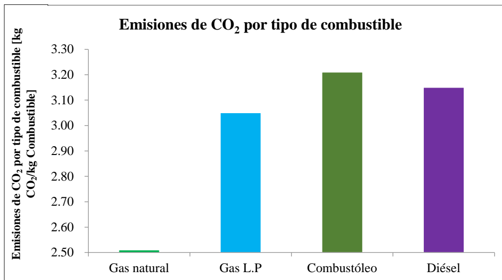
Figura 30. Emisiones expresadas en CO 2 eq generadas a partir del consumo de diferentes tipos de combustibles. ( Deloitte Touche Tohmatsu Limited, 2014).
