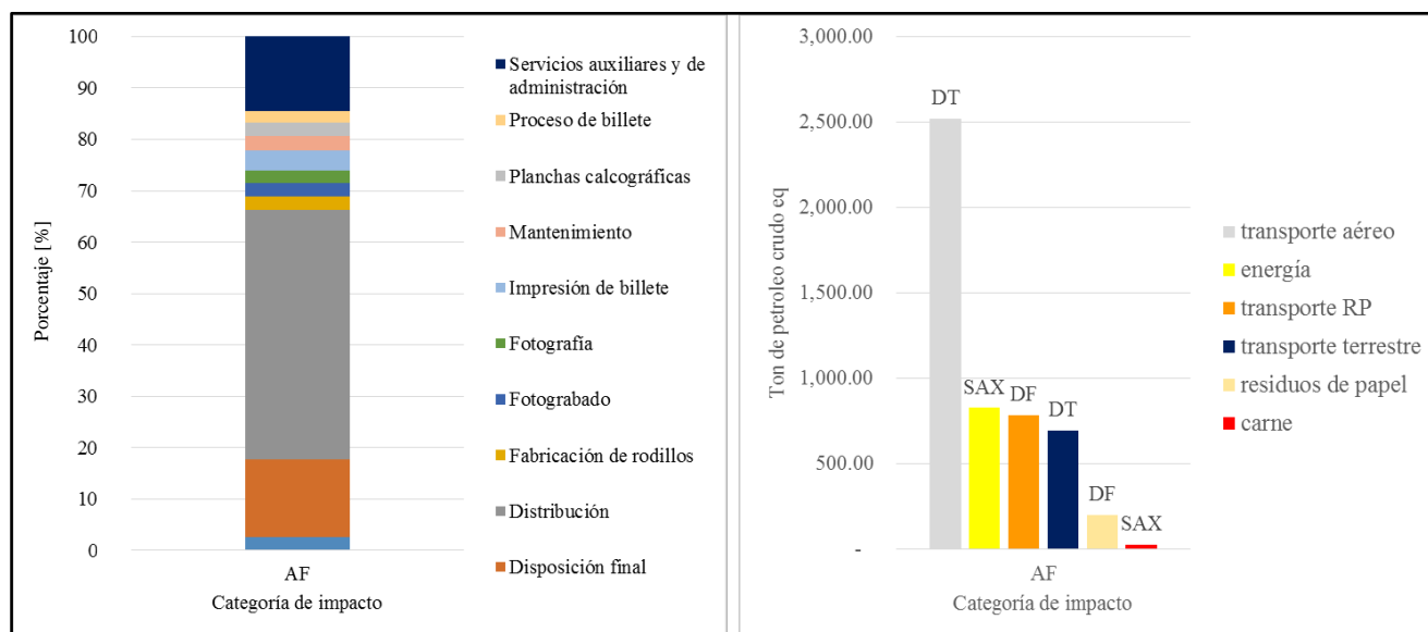
Figura 19. Resultados de impacto ambiental para la categoría de agotamiento de combustibles fósiles.
