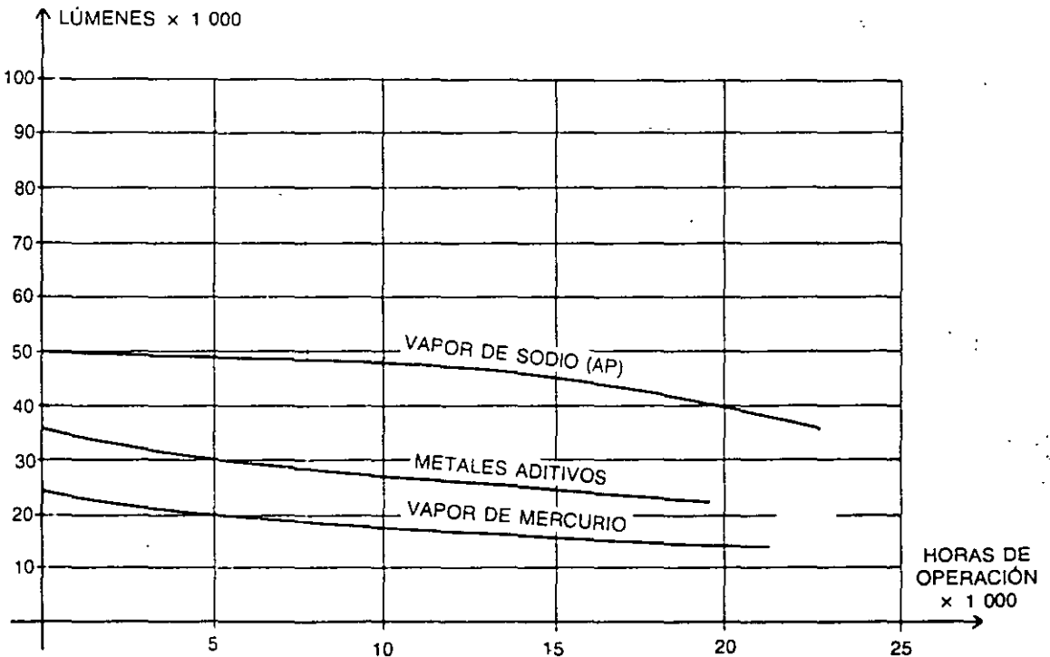
FIG. 6-4 Curvas de intensidad luminosa-tiempo
