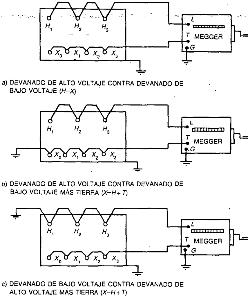
FIG. 11-2 Conexiones para las pruebas con megger.
