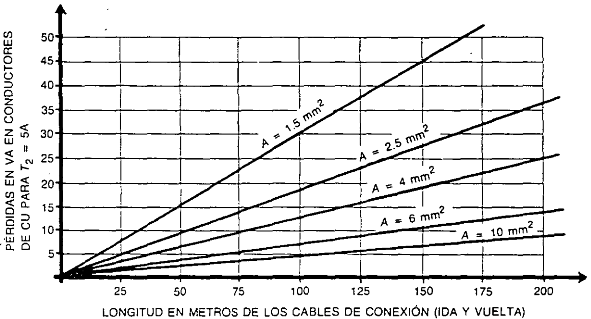
FIG. 2-8 Pérdidas en cables de control
