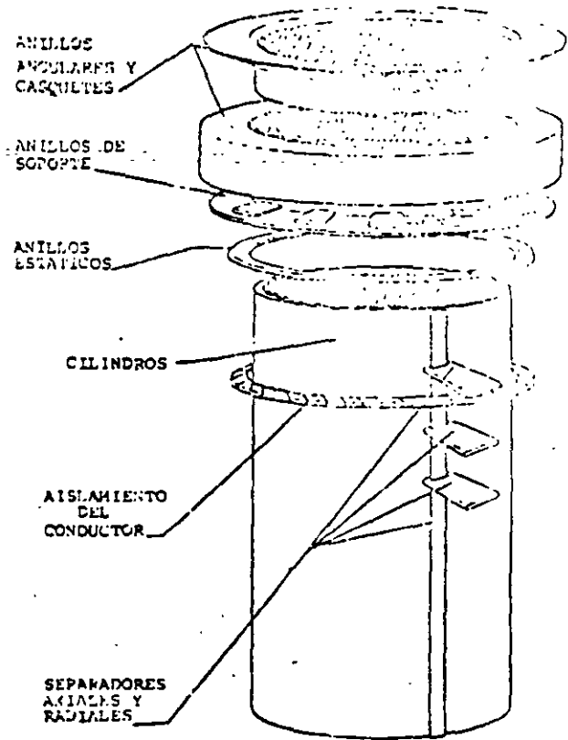
FIGURA 4 AISLAMIENTO TRANSFORMADOR TIPO COLUMNA
