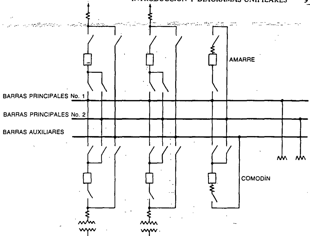
1. DIAGRAMA DE CONEXIONES CON DOBLE JUEGO DE BARRAS COLECTORAS PRINCIPALES Y UNO DE BARRAS COLECTORAS AUXILIARES
