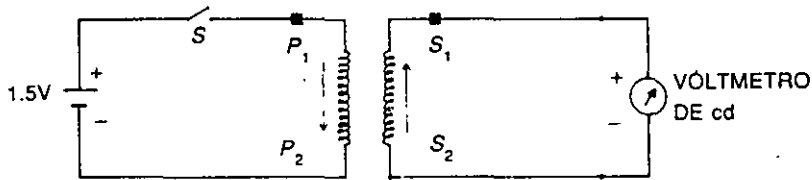
DIAGRAMA DE CONEXIONES PARA POLARIDAD ADITIVA
