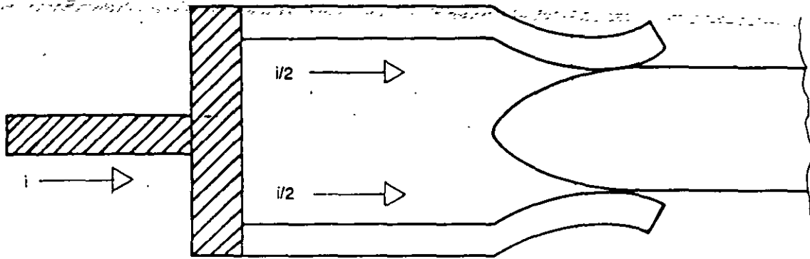
FIG. 2-24 Diferente forma de ensamble de los contactos
