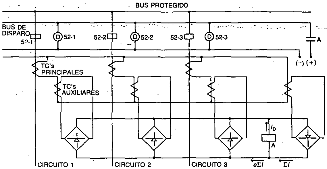
FIG. 7-25 Diagrama de protección diferencial de buses
