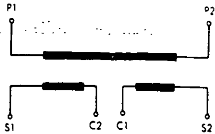
T.P. CON DOBLE RELACION DE TRANSFORMACION SOBRE EL BOBINADO SECUNDARIO POR CONEXION SERIE PARALELO.
