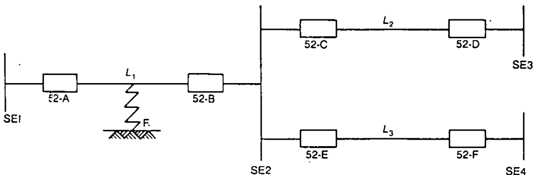
FIG. 7-12 Falla con protección de distancia
