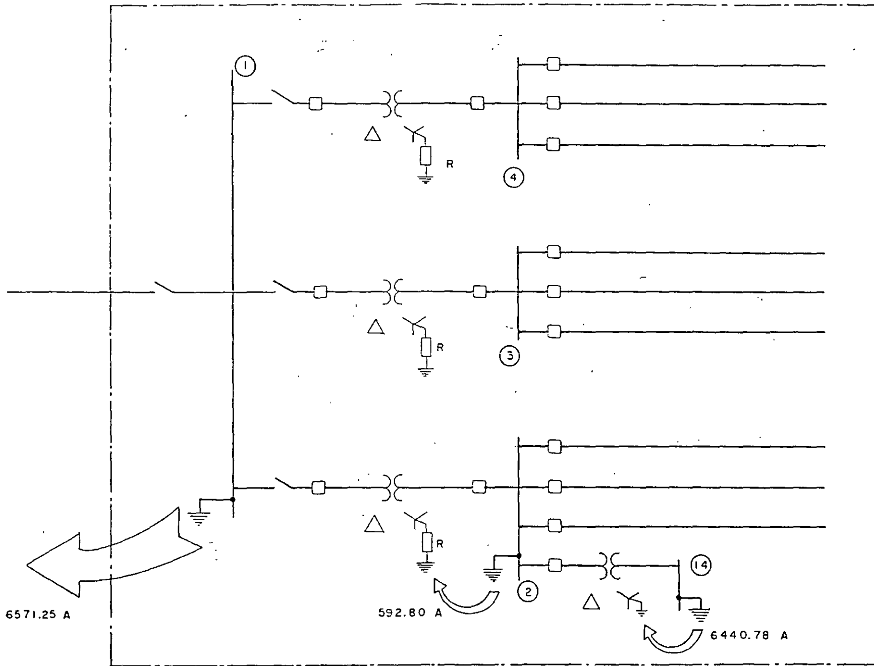
DISTRIBUCION DE CORRIENTES DE FALLA MONOFASICA EN SUBESTACION PRINCIPAL
