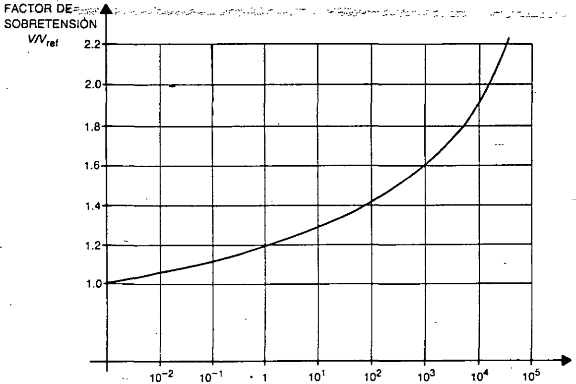
FIG. 2-18 Curva tensión-corriente en elemento de ZnO
