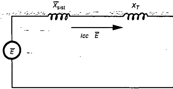
FIG. 2-5 Equivalente de Thévenin de secuencia positiva
