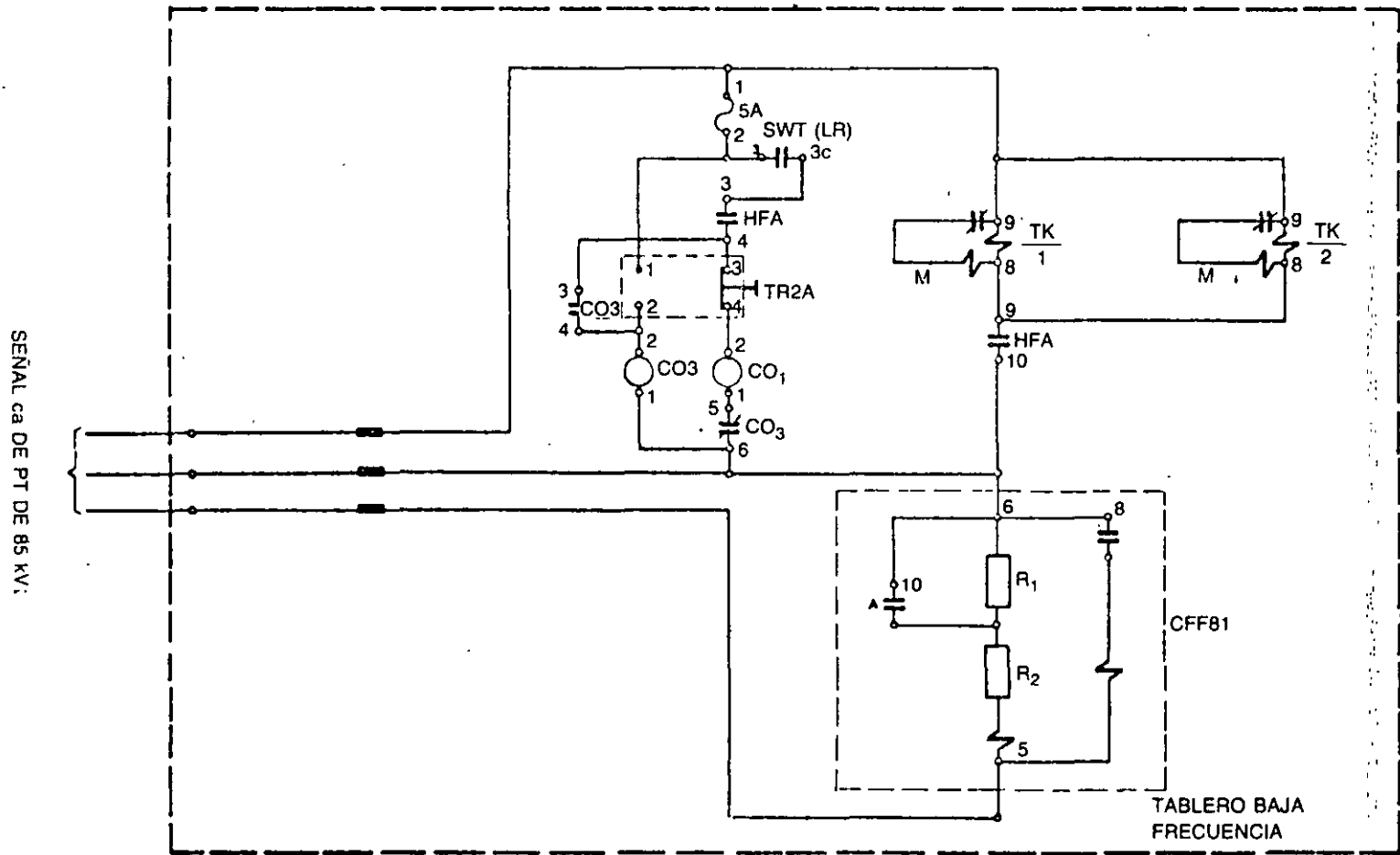
FIG. 9-7 Diagrama elemental de ca
