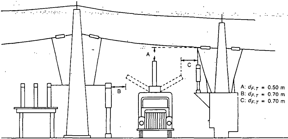
FIG. 5-26 Distancias de vehículos a partes vivas
