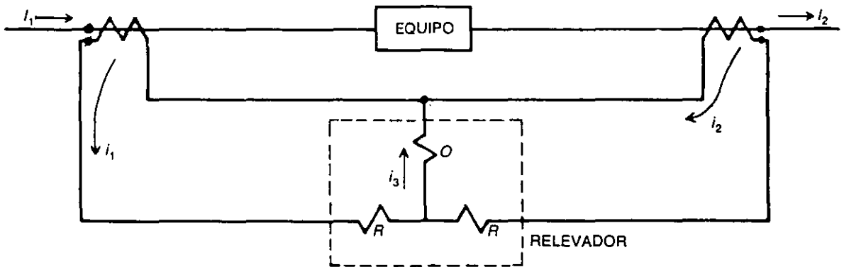
FIG. 7-7 Conexión de un relevador diferencial
