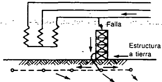
Caso 2. Falla en el local de la estación. Neutro conectado a tierra sólo en punto remoto. La corriente total de falla fluye de la red de tierra hacia la tierra.
