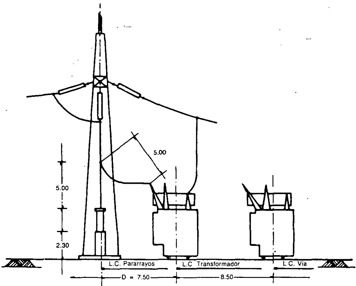
FIG. 5-9 Distancia máxima del pararrayos
