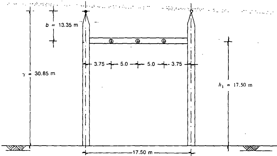
FIG. 5-16 Marco para 230 kV
