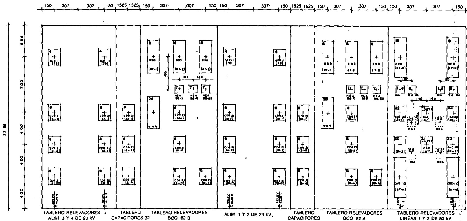
FIG. 10-1 Localización de aparatos y taladros en tableros
