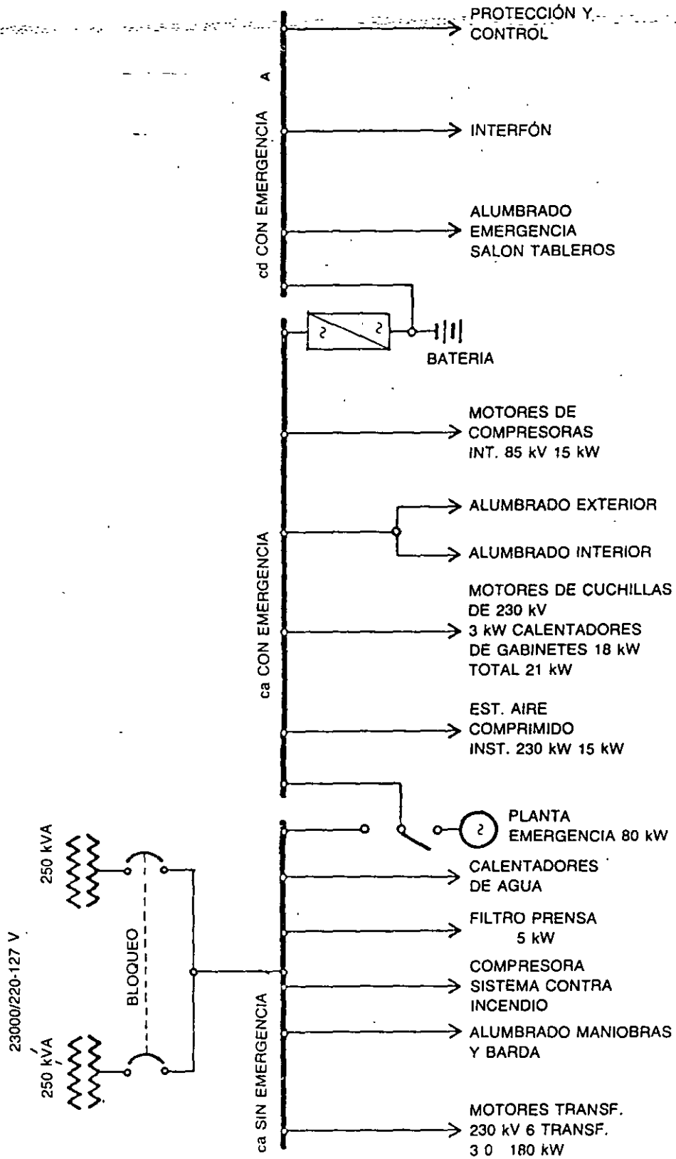
FIG. 6-2 Arreglo con planta de emergencia
