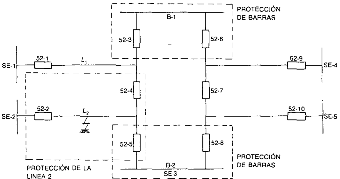
FIG. 7-13 Análisis de protecciones con falla de interruptores
