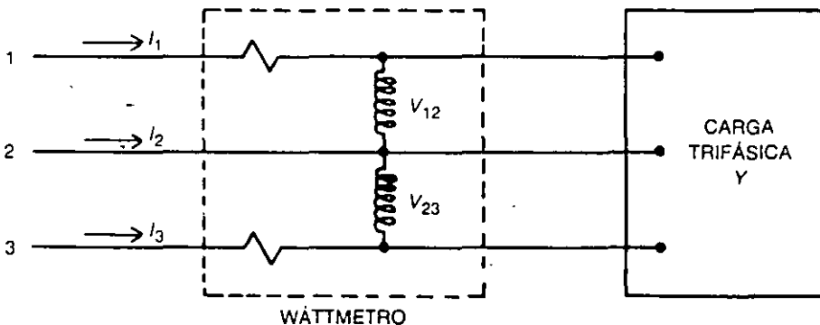
FIG. 8-2 Diagrama elemental de un wáttmetro trifásico (3 hilos)
