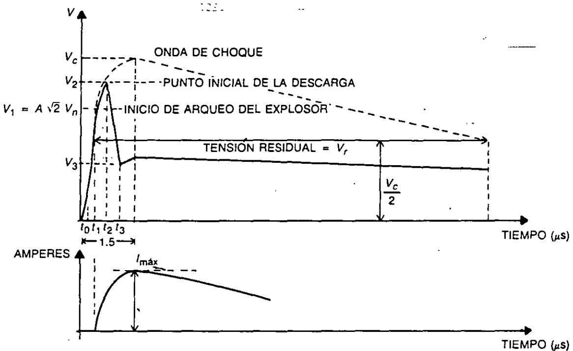
FIG. 2-16 Funcionamiento del pararrayos
