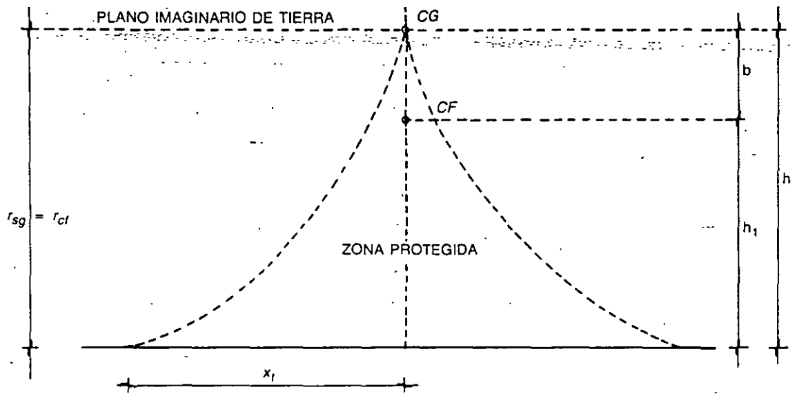
FIG. 5-11 Protección de un cable de fuerza
