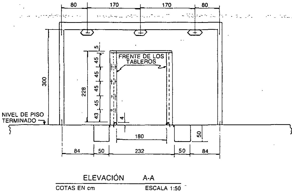
FIG. 5-35 Corte transversal de la caseta tipo
