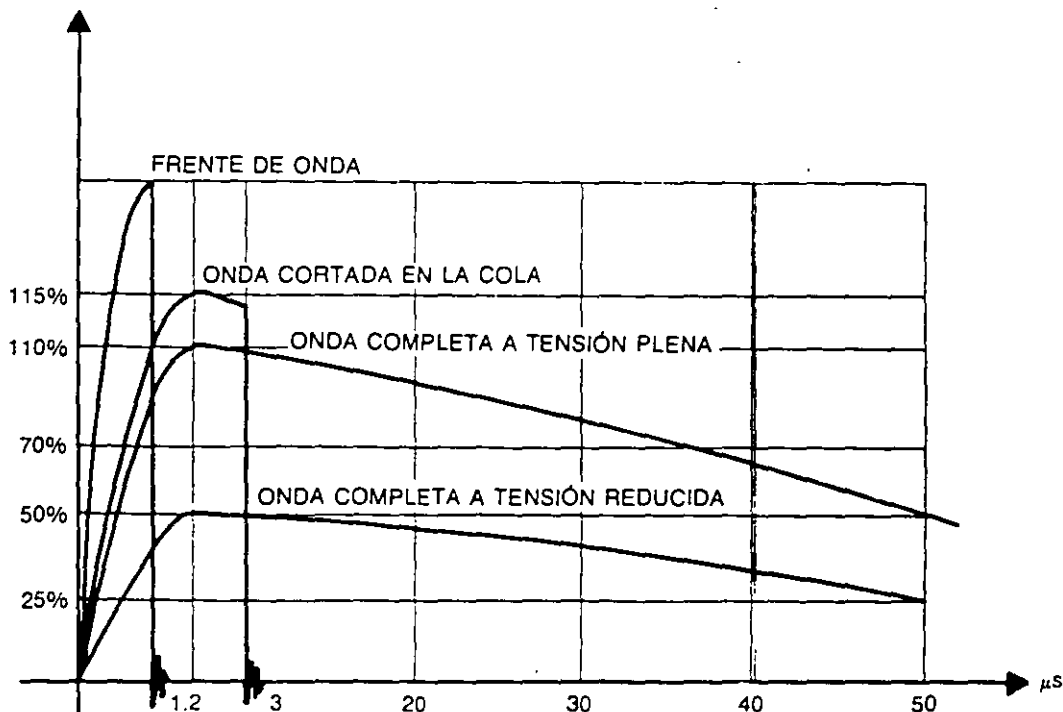
FIG. 2-7 Tipos de onda de impulso
