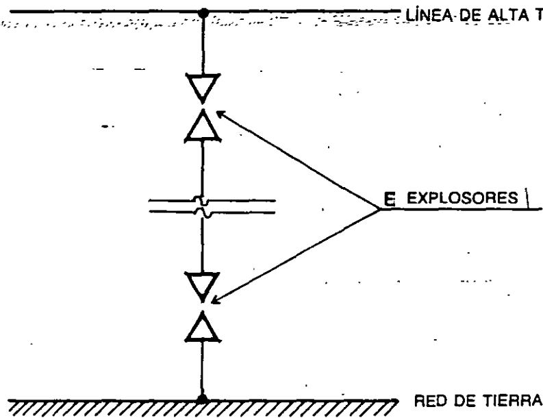
FIG. 2-13 Esquema de pararrayos primitivo
