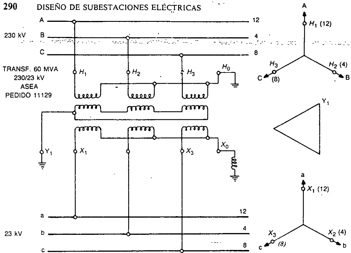
FIG. 5-31 Conexiones de transformador trifásico de 230 kV "Asea" (defasamiento de 0° entre 230 kV y 23 kV) con terciario de armónicas conectado en delta
