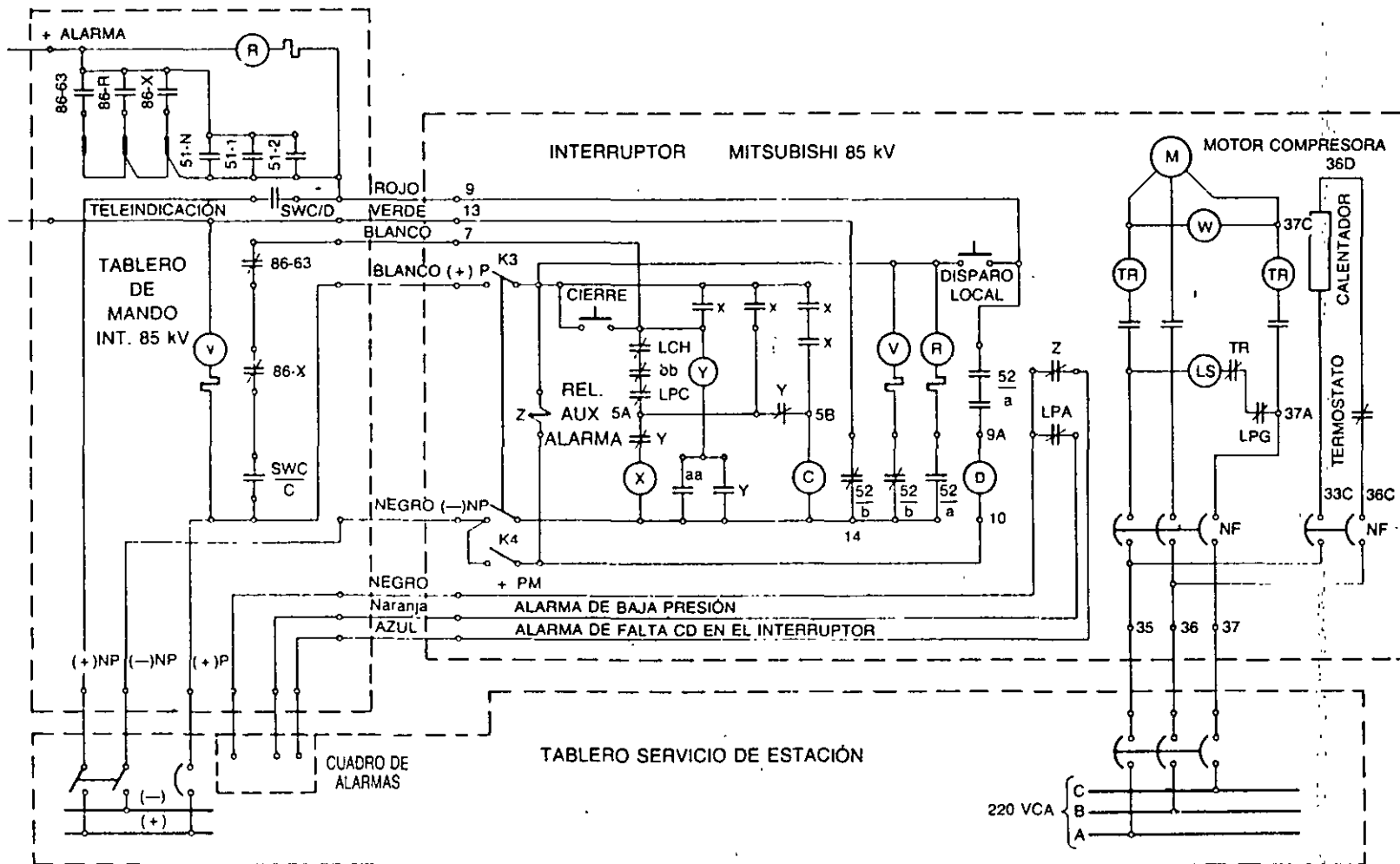
FIG 9-1 Diagrama de control de un interruptor con lámparas verde y roja
