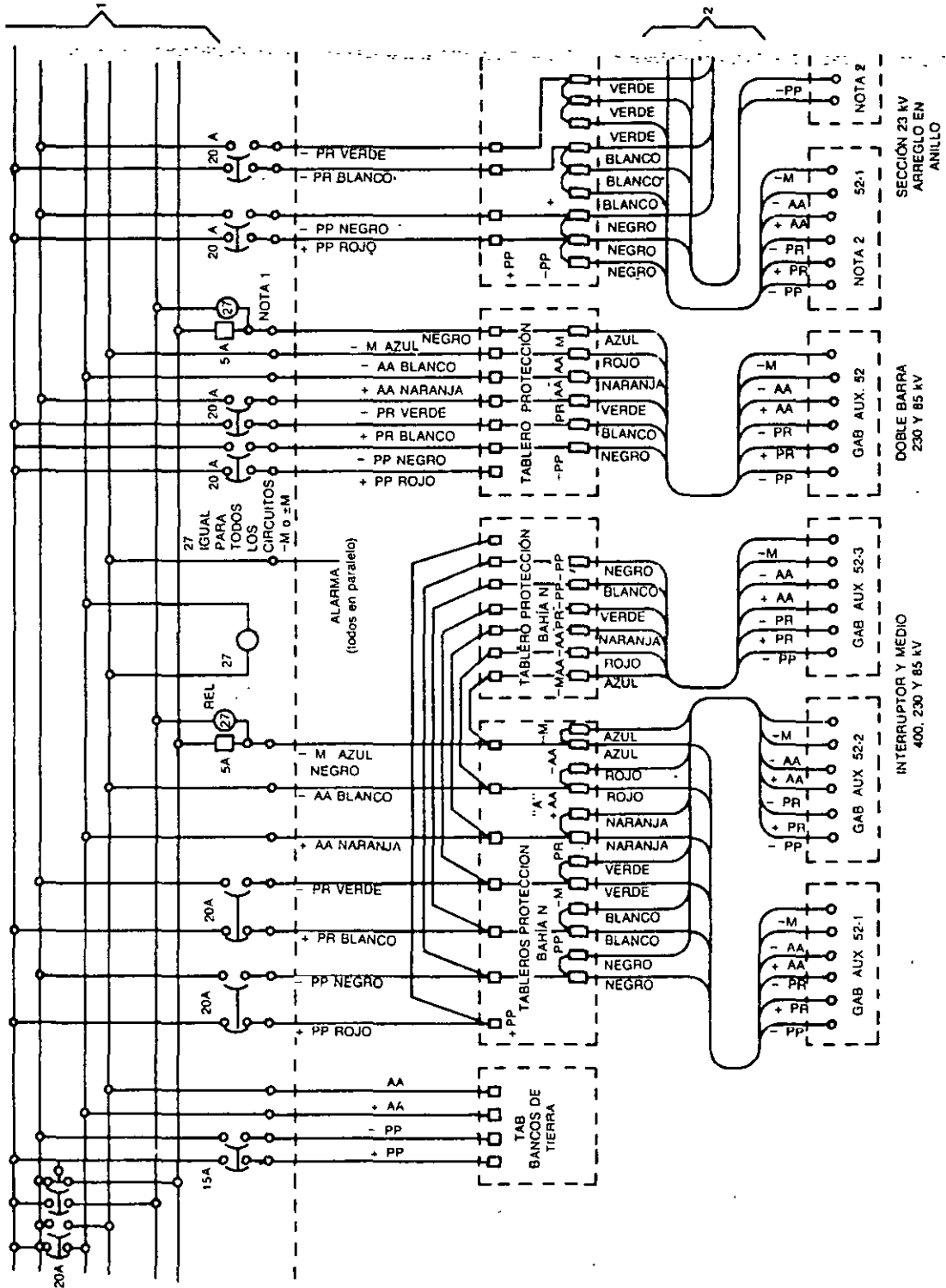
FIG. 9-16 Tablero servicio de estación
