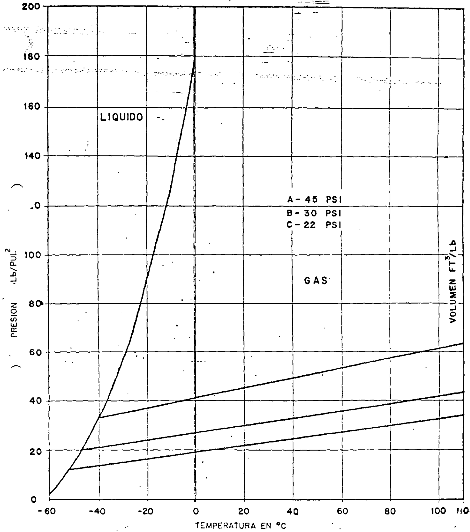
VARIACION DE PRESION Y TEMPERATURA DEL SF 6 A DENSIDAD CONSTANTE
