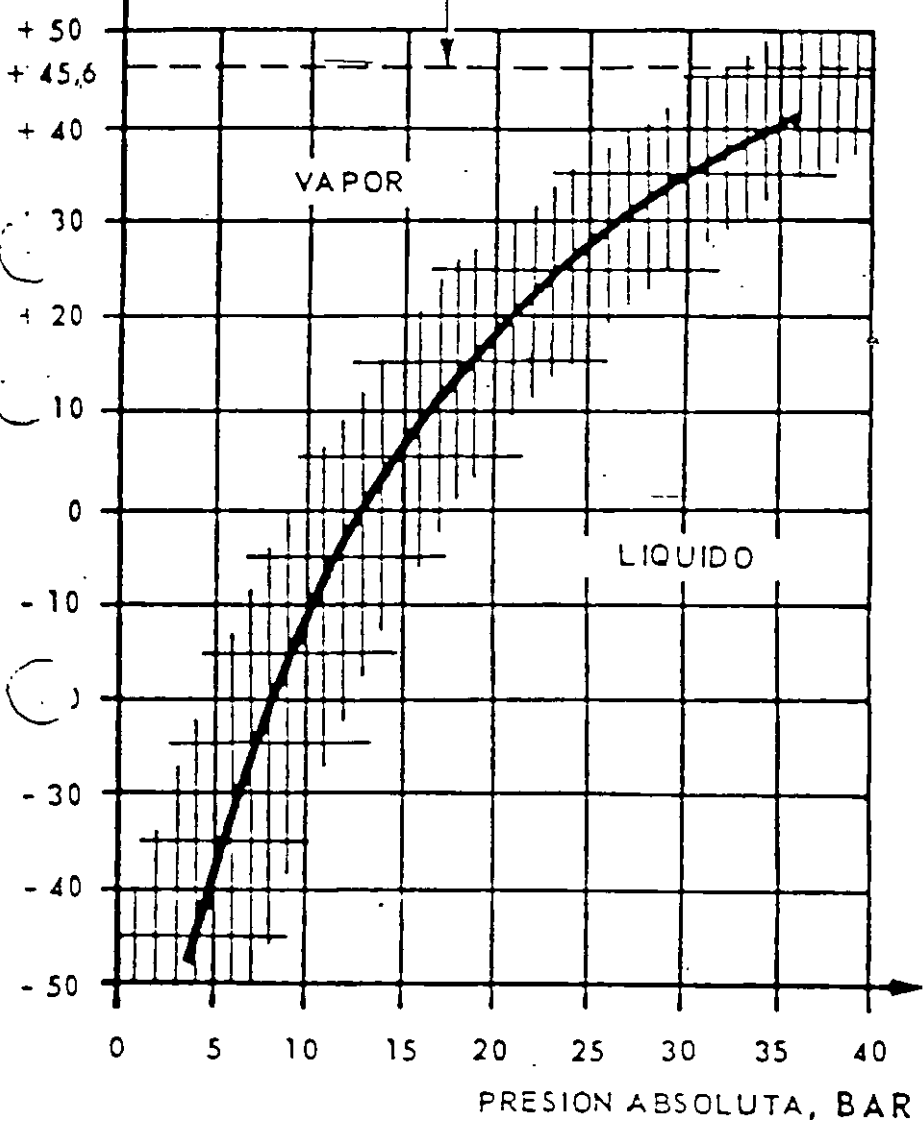
CURVA DE PRESION DE VAPOR SATURANTE DEL SF 6
