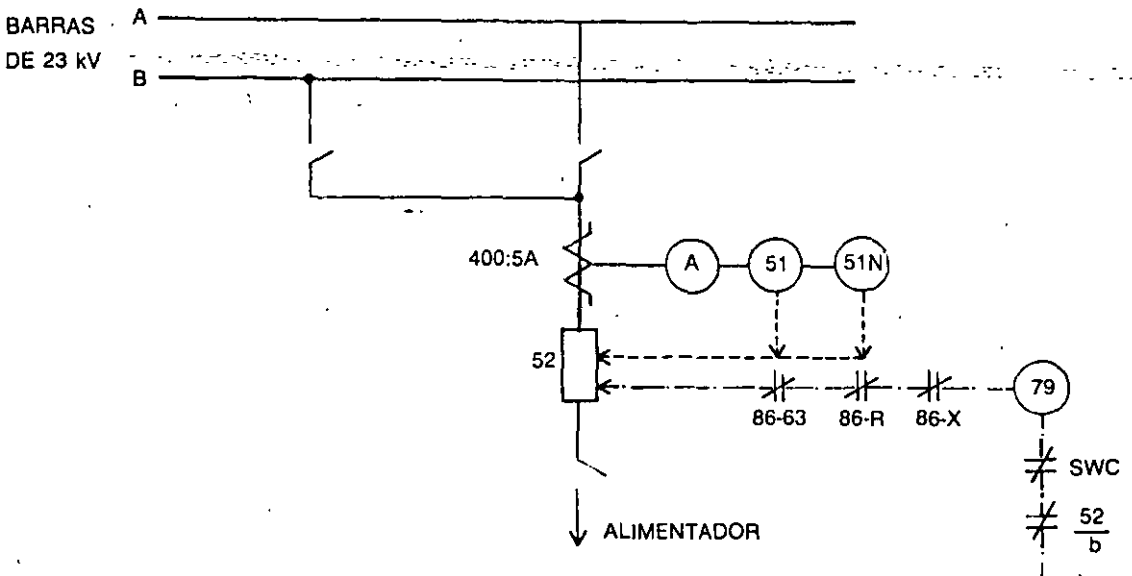
FIG. 7-28 Diagrama de protección para alimentador. Arreglo de doble barra
