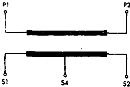
T.P. CON DOBLE RELACION DE TRANSFORMACION POR MEDIO DE "TOMA" SOBRE EL BOBINADO SECUNDARIO
