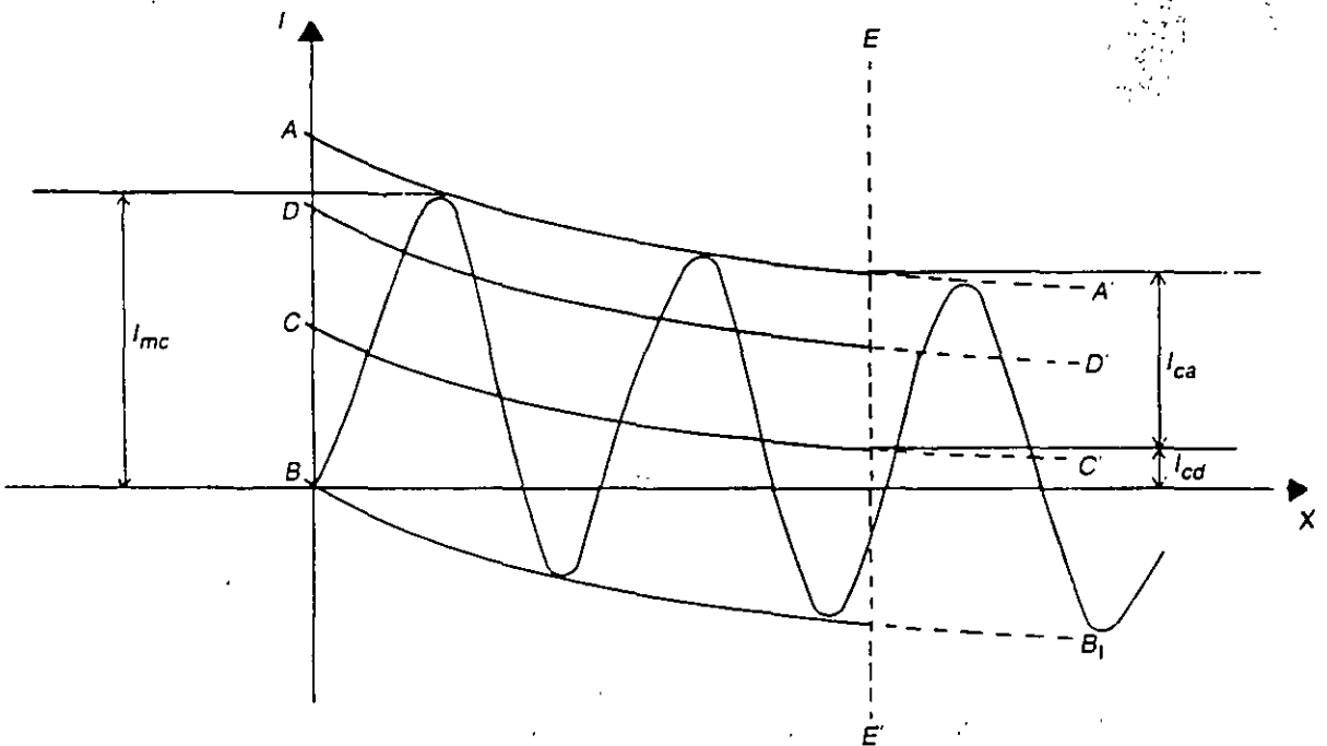
FIG. 2-22 Cortocircuito asimétrico
