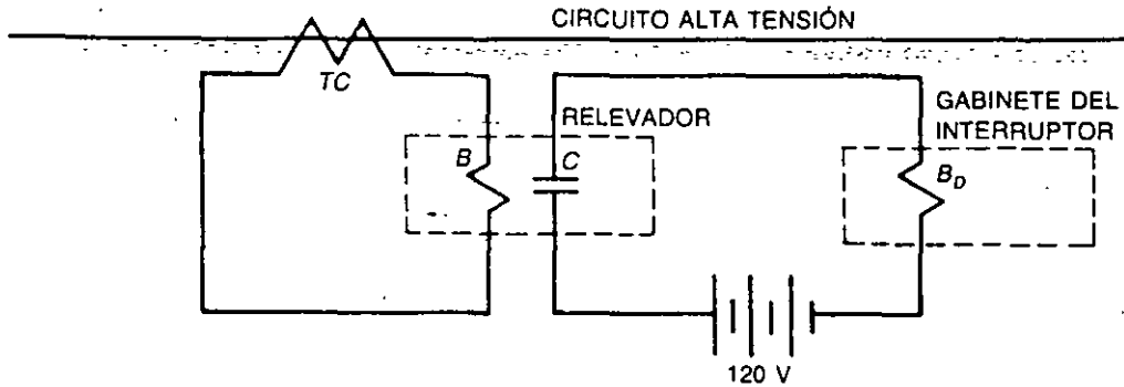
FIG. 7-1 Circuito elemental de protección por sobrecorriente
