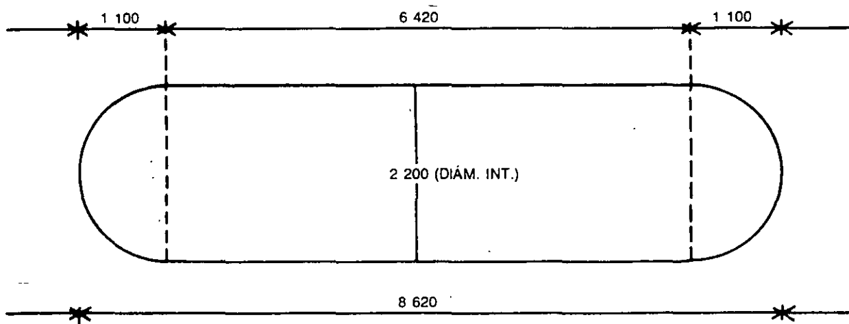
FIG. 6-18 Tanque hidroneumático
