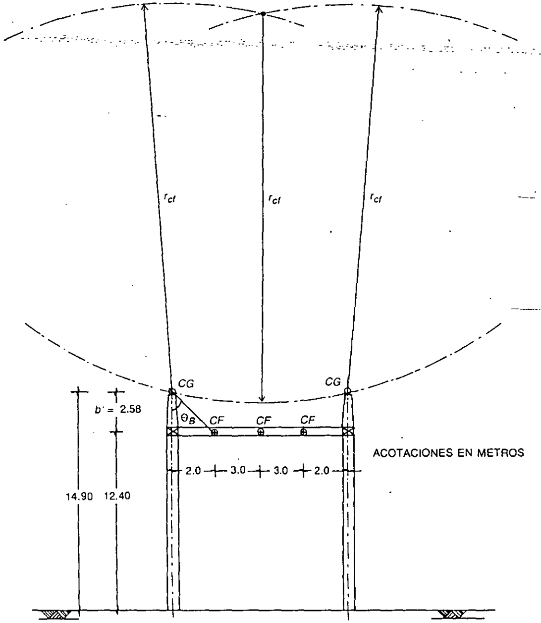
FIG. 5-15 Módulo electrogeométrico
