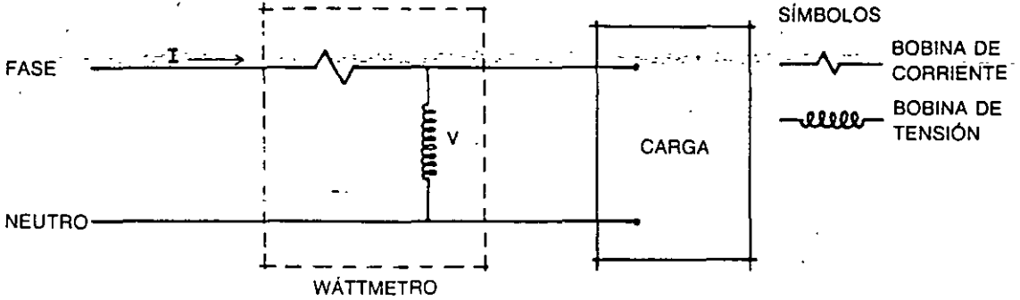
FIG. 8-1 Diagrama elemental de un wáttmetro monofásico
