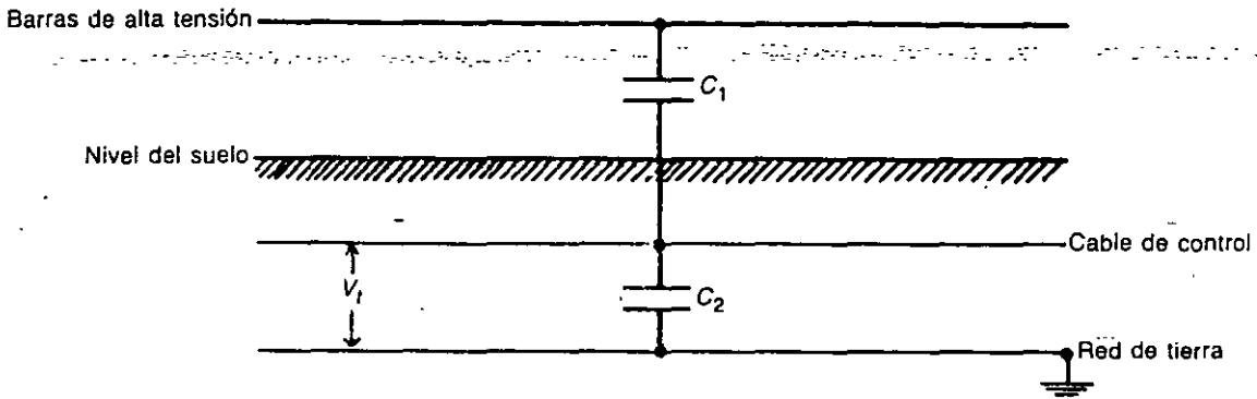
FIG. 5-38 Inducción electrostática en un conductor
