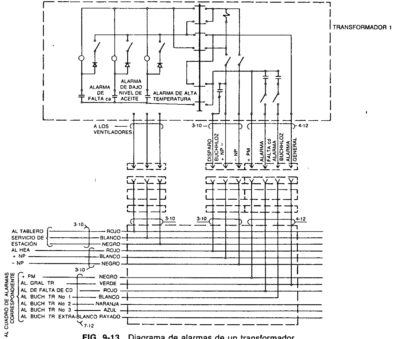
FIG. 9-13 Diagrama de alarmas de un transformador
