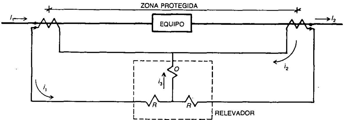
FIG. 7-16 Esquema de frotación diferencial
