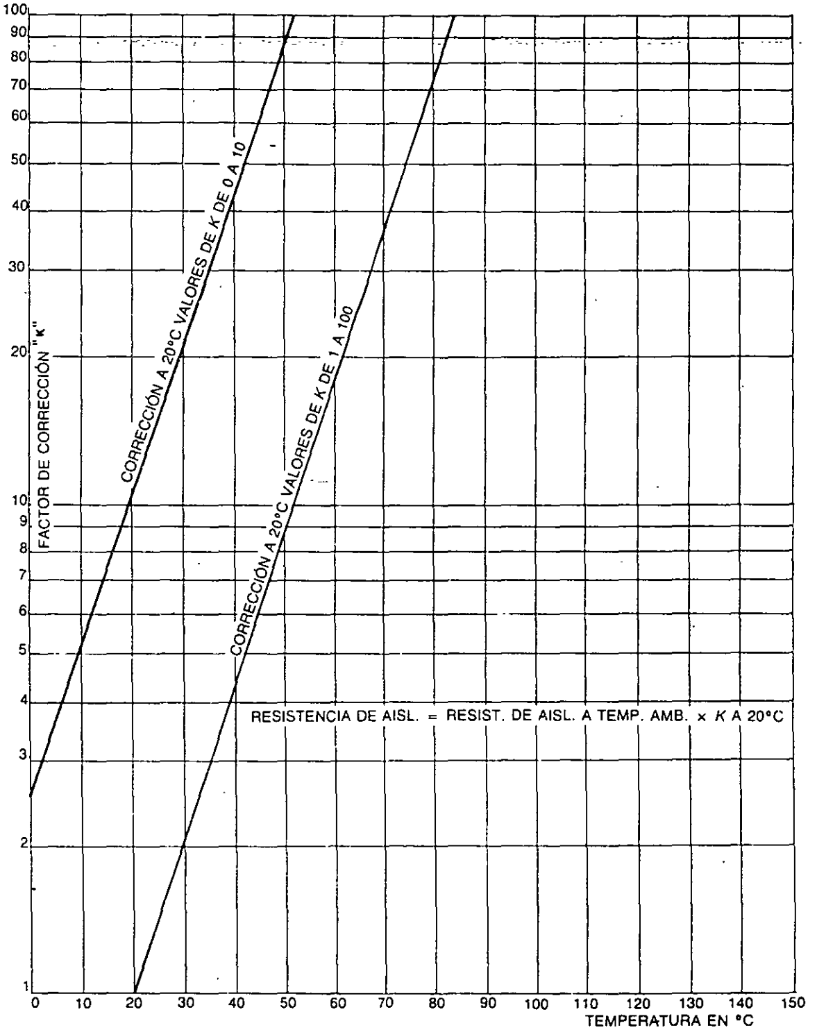
FIG. 11-1 Gráfica K-Temperatura.
