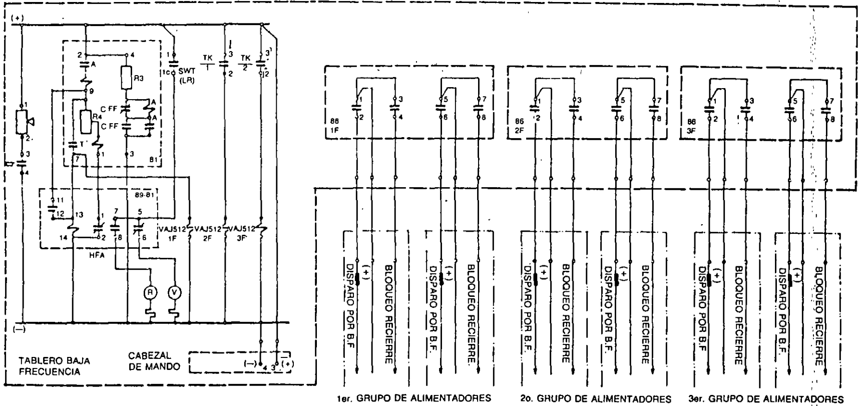
FIG. 9-8 Diagrama elemental de cd
