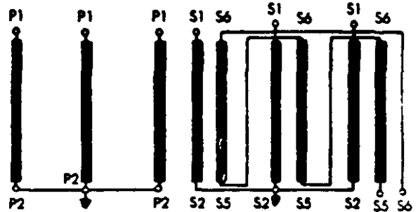
ACOPAMIENTO DE TRES TRANSFORMADORES DEL TIPO REPRESENTADO EN EL ESQUEMA SUPERIOR.
