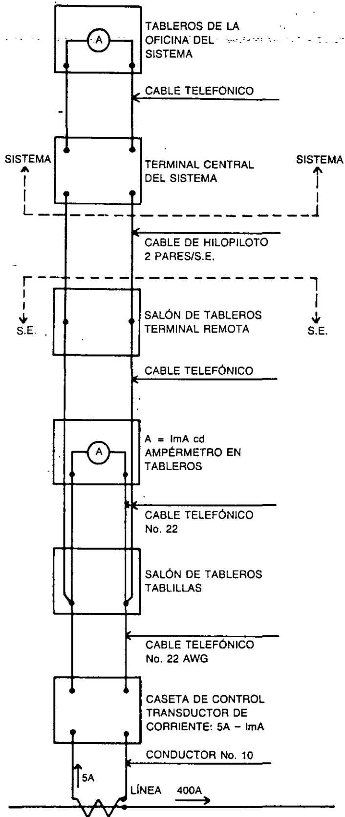
FIG. 8-6 Diagrama para la telemedición de corriente
