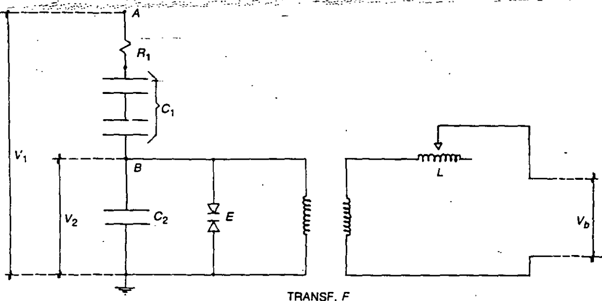
FIG. 2-9 Dispositivo de potencial
