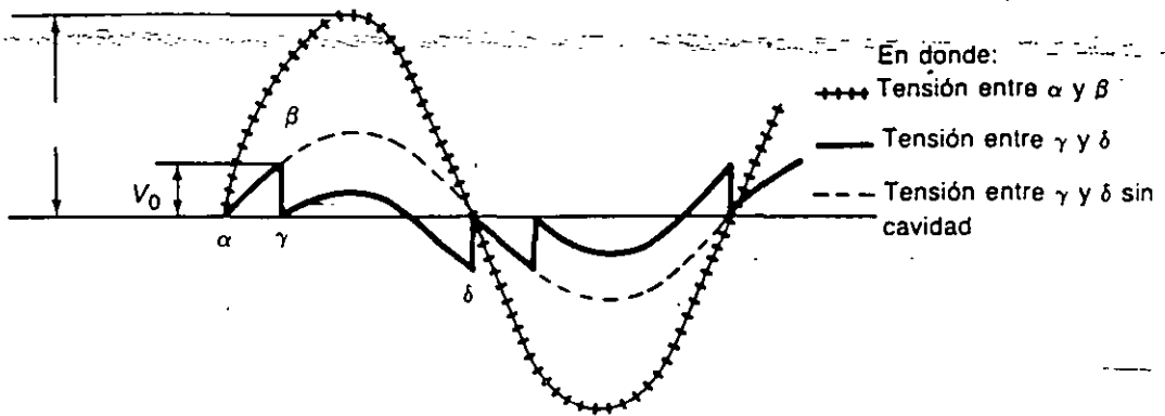
FIG. 2-4 Forma de onda de una descarga
