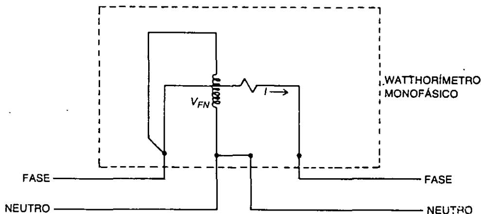
FIG. 8-4 Conexión de un wathhorímetro monofásico
