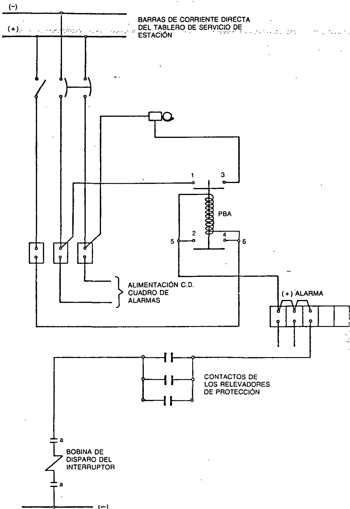
FIG. 9-12 Diagrama de un circuito de alarma
