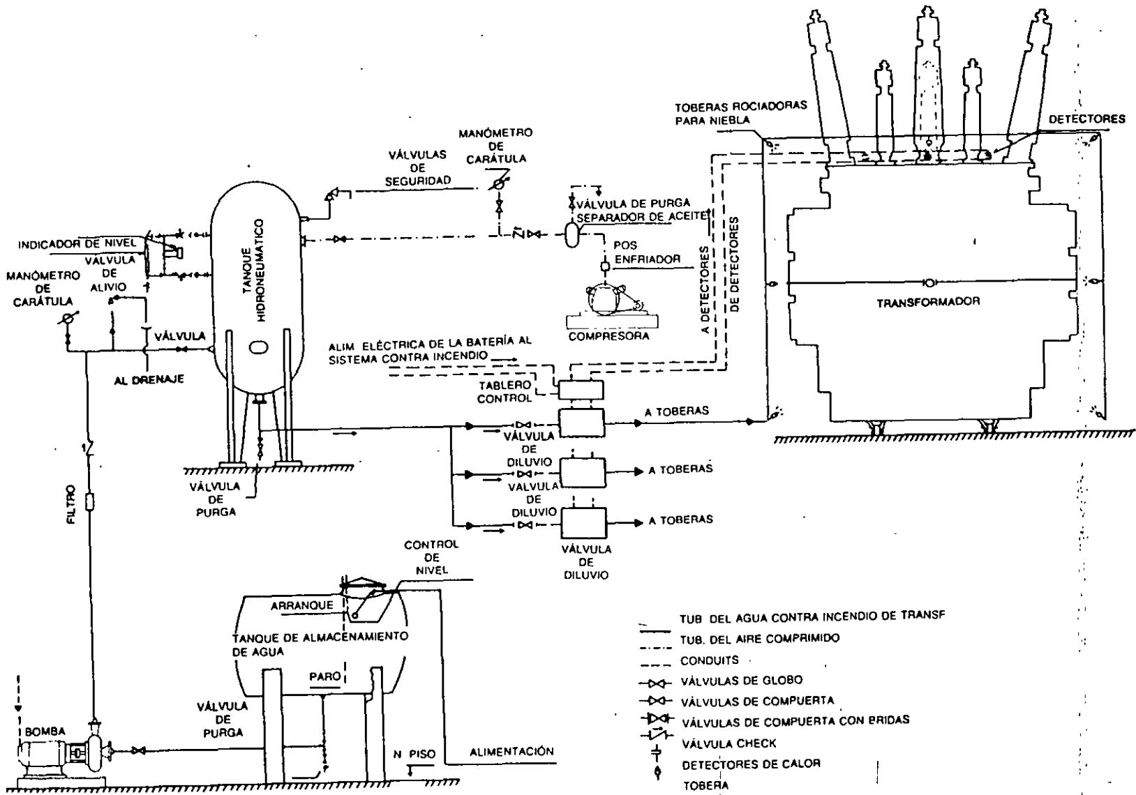
FIG. 6-16 Diagrama general del sistema automático contra incendio para
