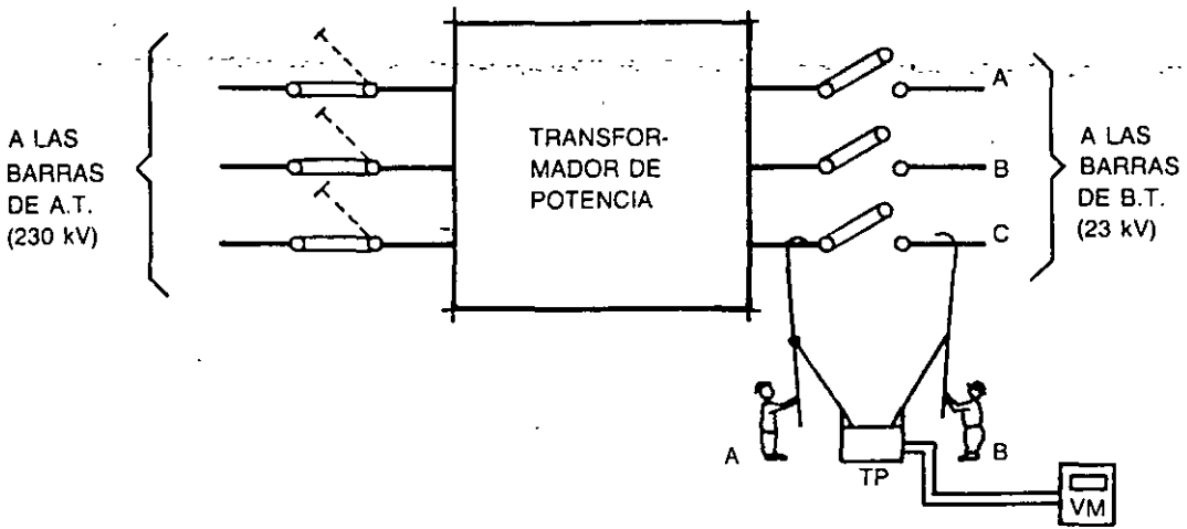
FIG. 11-8 Conexión para el faseo
