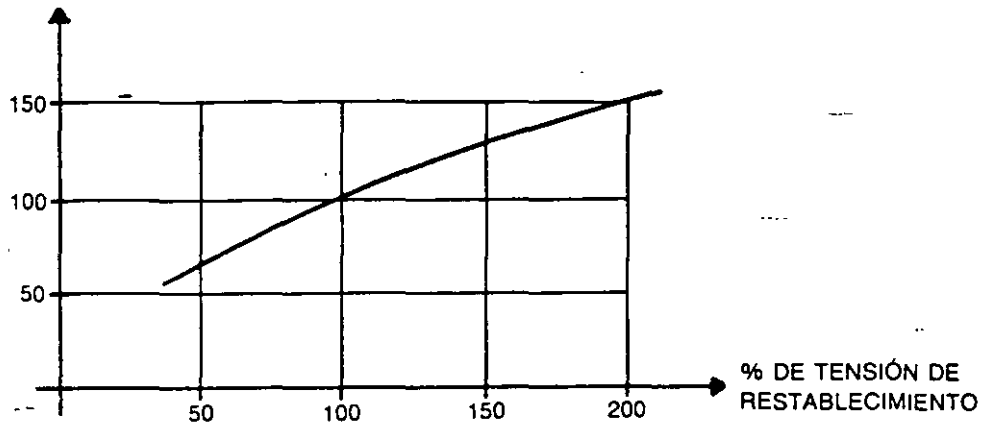
FIG. 2-19 Curvas potencia de cortocircuito-tensión de restablecimiento.
