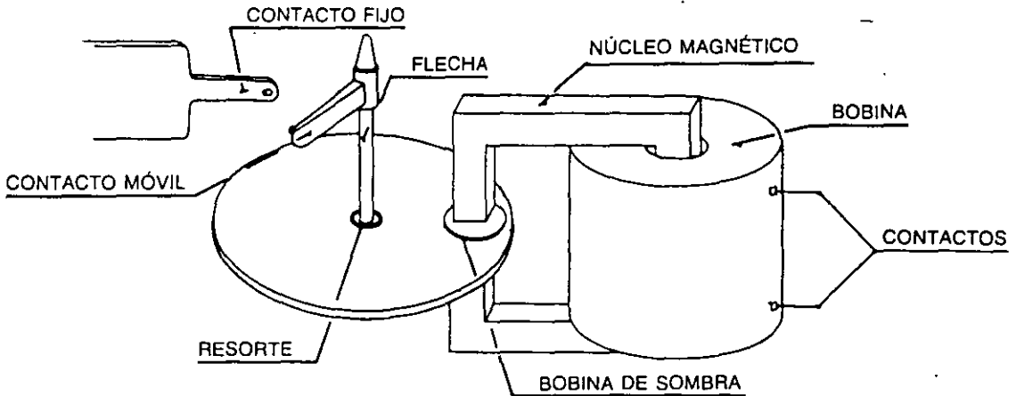
FIG. 7-5 Relevador tipo disco de inducción
