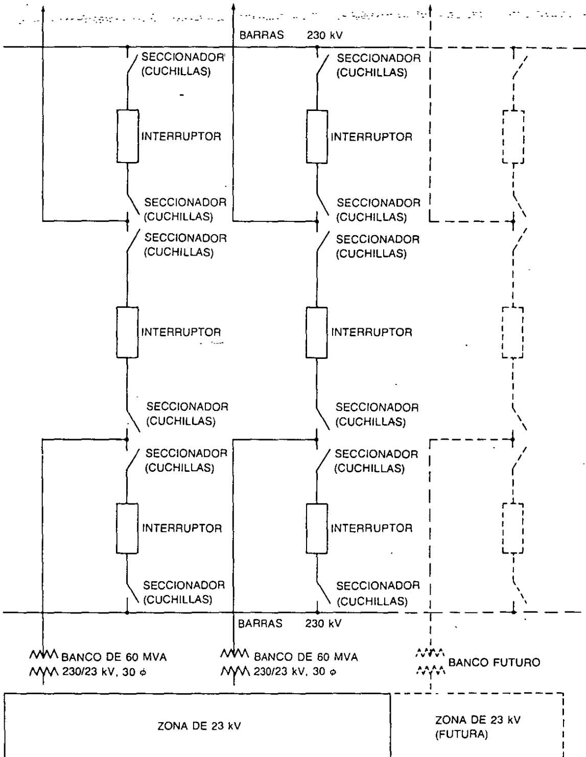
FIG. 5-2 Diagrama unifilar de subestaciones normalizadas de 230/23 kV
