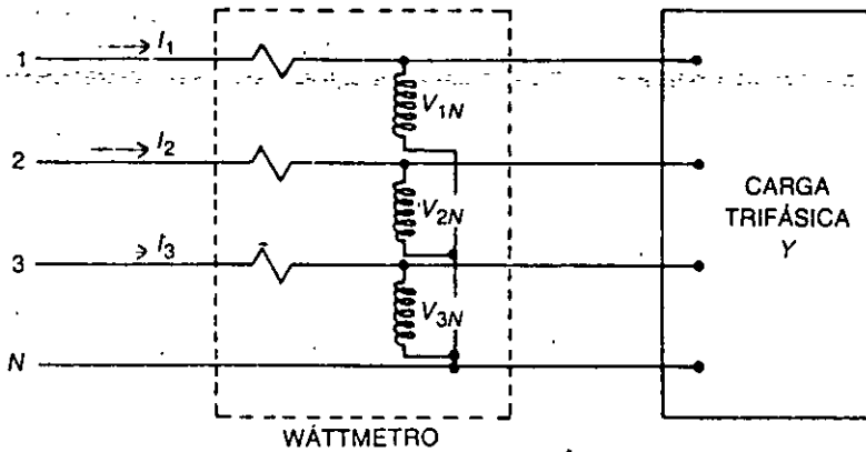
FIG. 8-3 Diagrama elemental de un wáttmetro trifásico (4 hilos)
