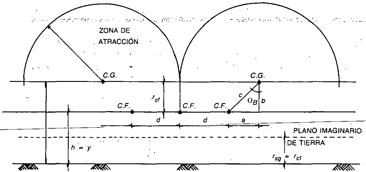
FIG. 5-12 Protección por zonas
