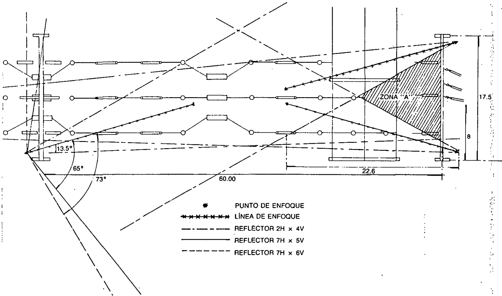
FIG. 6-7 Vista de planta de los haces horizontales de los tres reflectores (1/2 módulo de 230 kV)
