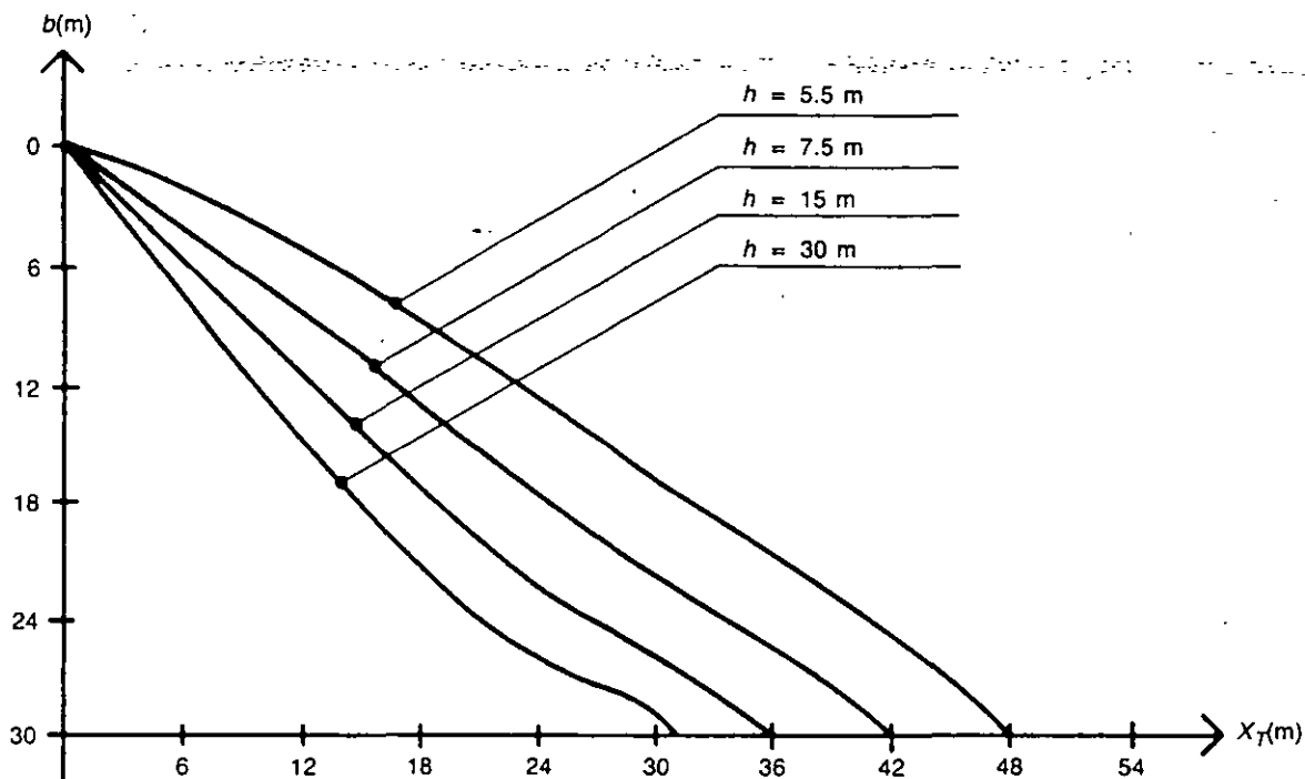
FIG. 5-19 Curvas b - X_T en función de h
