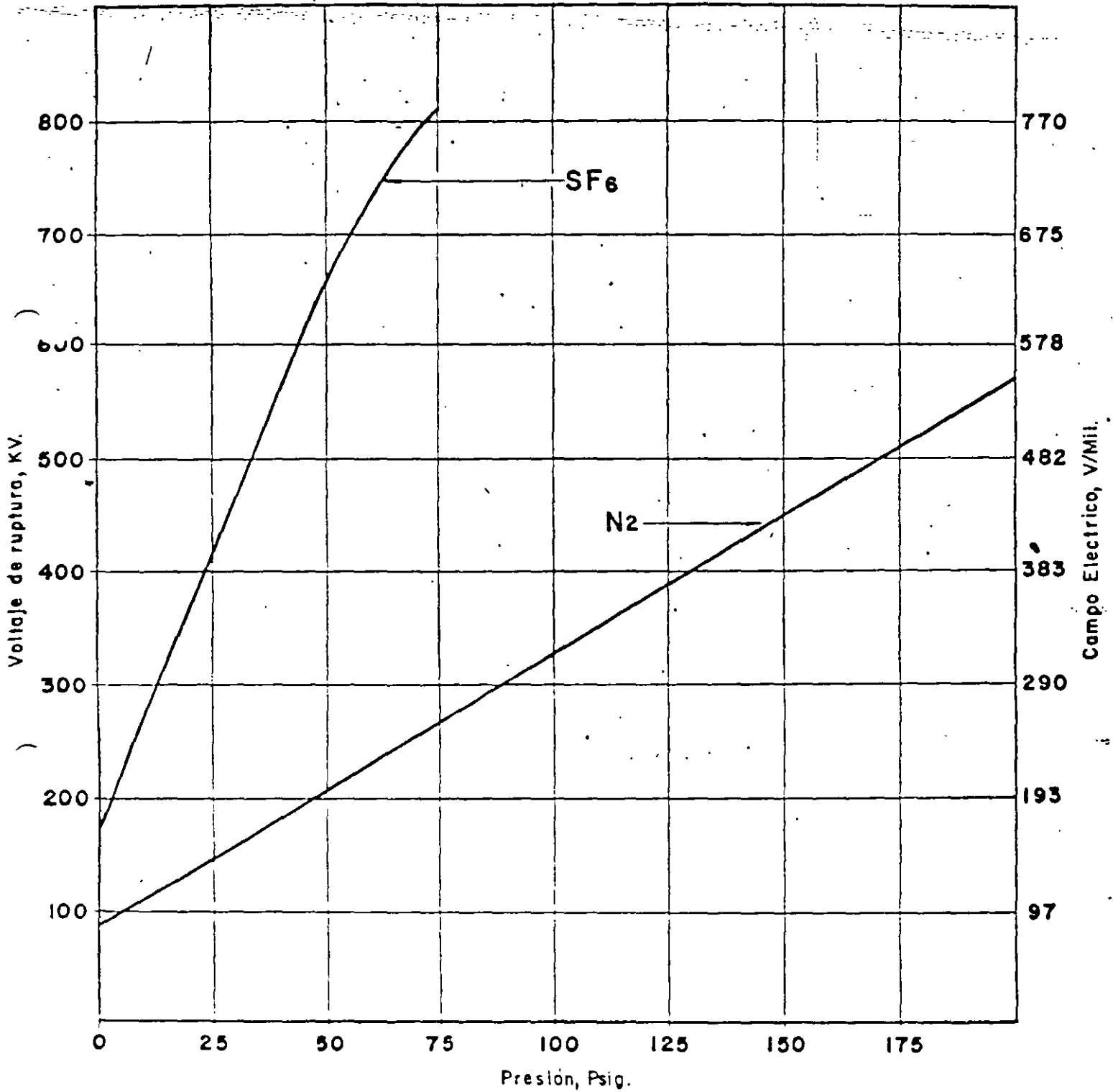
Voltaje de ruptura y campo electrico vs presión de SF 6 y N 2 .
