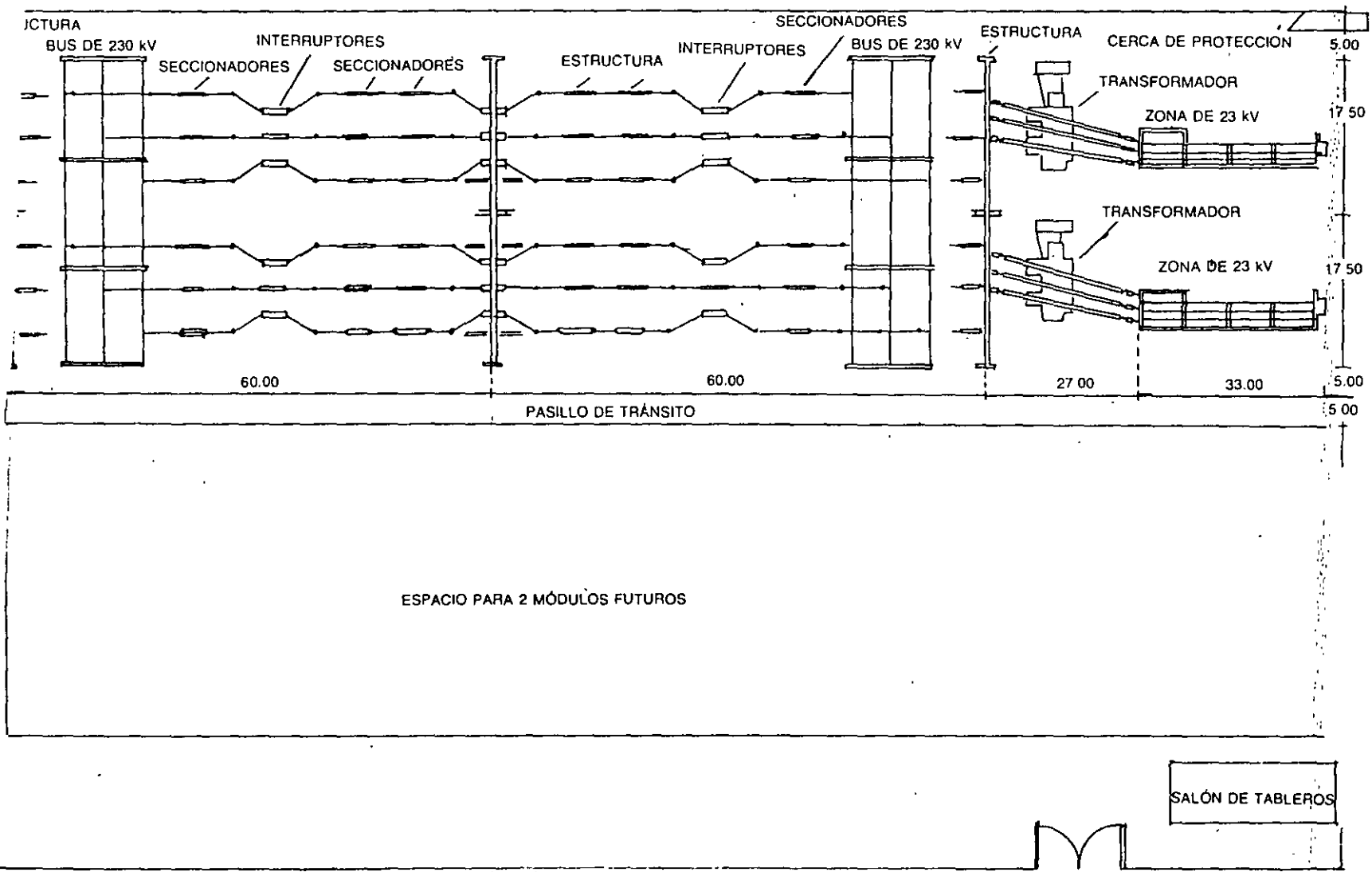
FIG. 5-4 SUBESTACIÓN AÉREA 230 000/23 000 VOLTS, VISTA DE PLANTA
