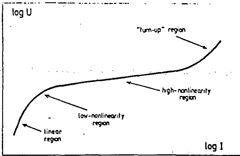
FIG. CURVA CARACTERISTICA PARA UN APARTARRAYOS DE OXIDO DE ZINC.
