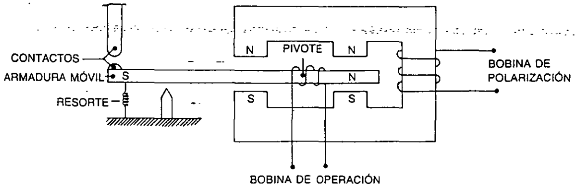
FIG. 7-9 Relevador direccional de corriente
