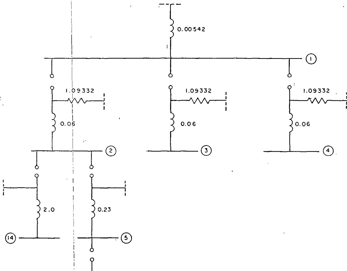
DIAGRAMA DE REACTANCIAS SECUENCIA CERO
