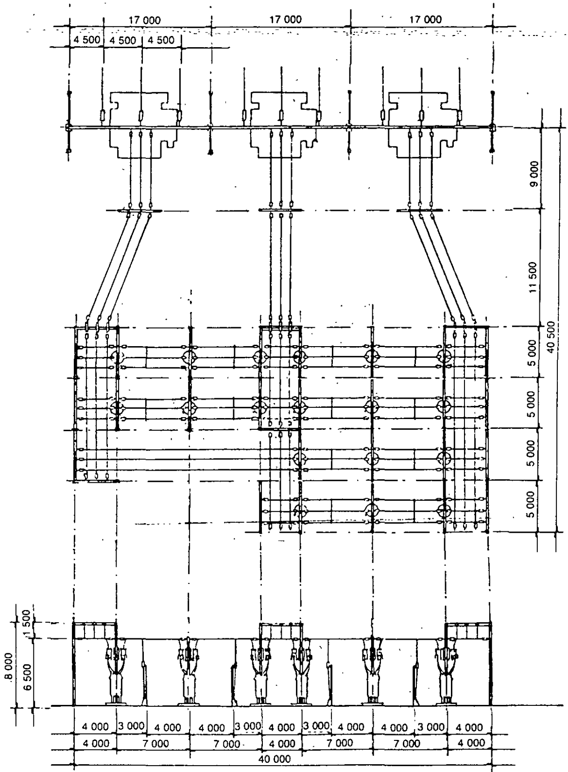
FIG. 5-33 Disposición física para el caso de tres transformadores trifásicos de 60 MVA 230/23 kV
