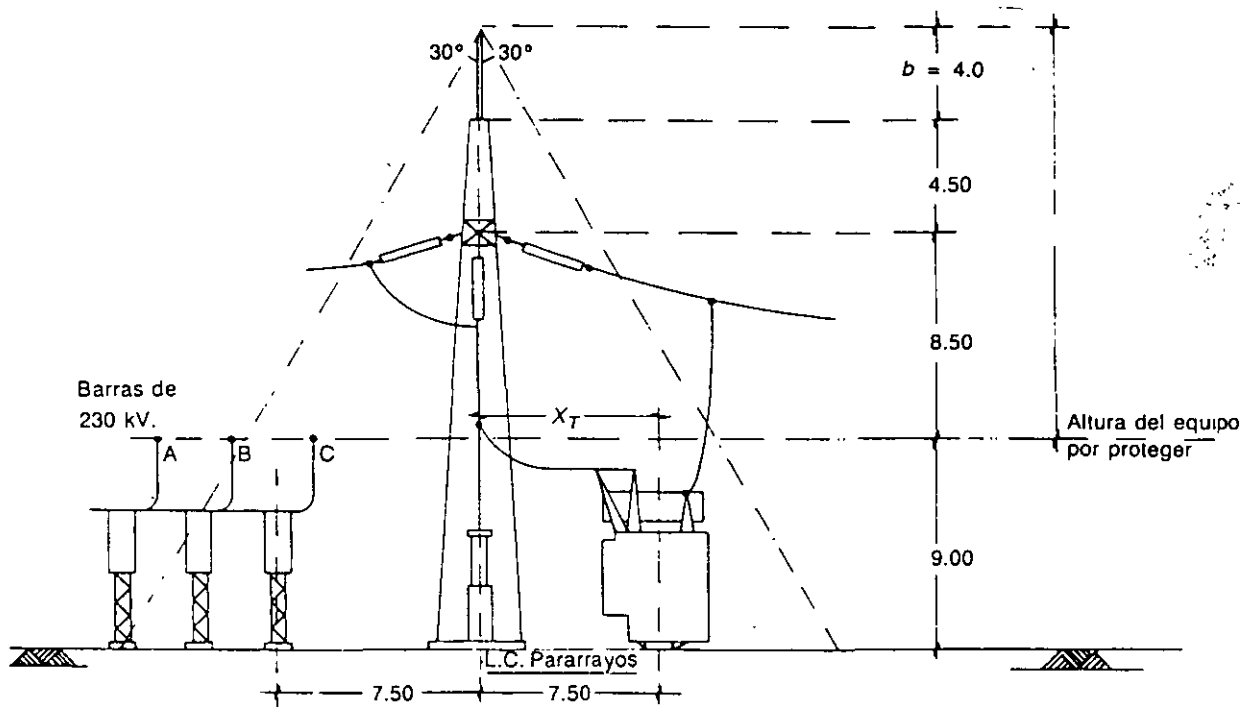
FIG. 5-20 Zona protegida de una instalación
