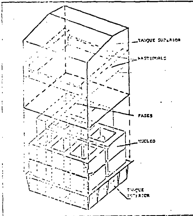
FIGURA 3 TRANSFORMADOR TIPO GORRAZADO
