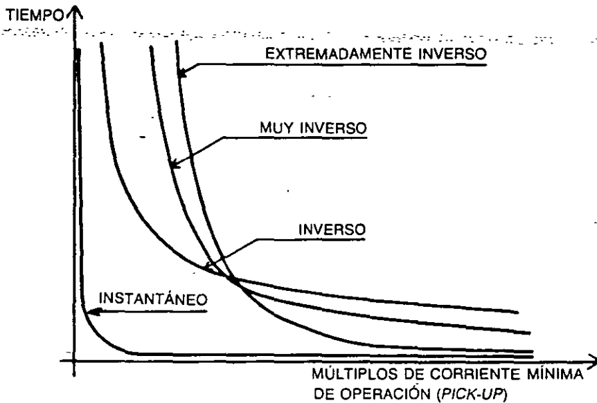
FIG. 7-6 Característica tiempo-corriente
