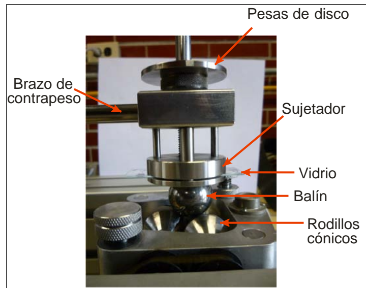
Figura 3.35 Partes del aparato de Ball Cratering
