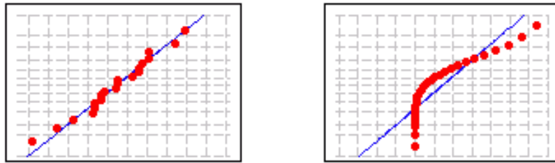
Gráfica 2.5 Gráficas de probabilidad. A la izquierda los datos se ajustan a la distribución de Weibull-3 y a la derecha los datos no se ajustan a la distribución.
