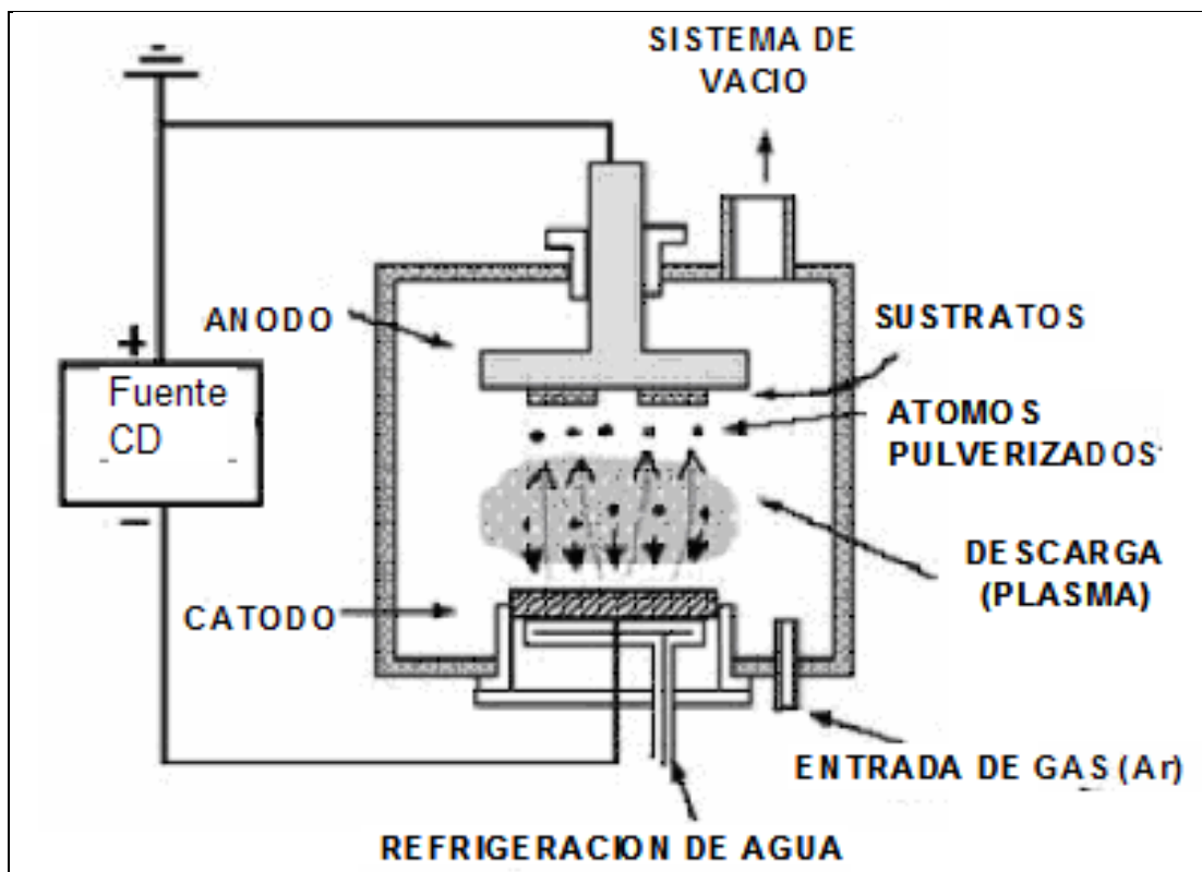
Figura 3.32 Sistema de sputtering magnético CD asistido por plasma
