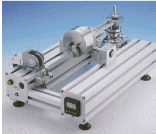
Figura 2. 2 Aparato de Ball Cratering .
