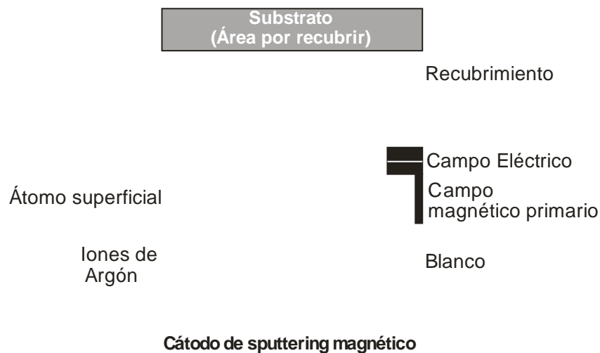
Figura 3.33 Sputtering magnético
