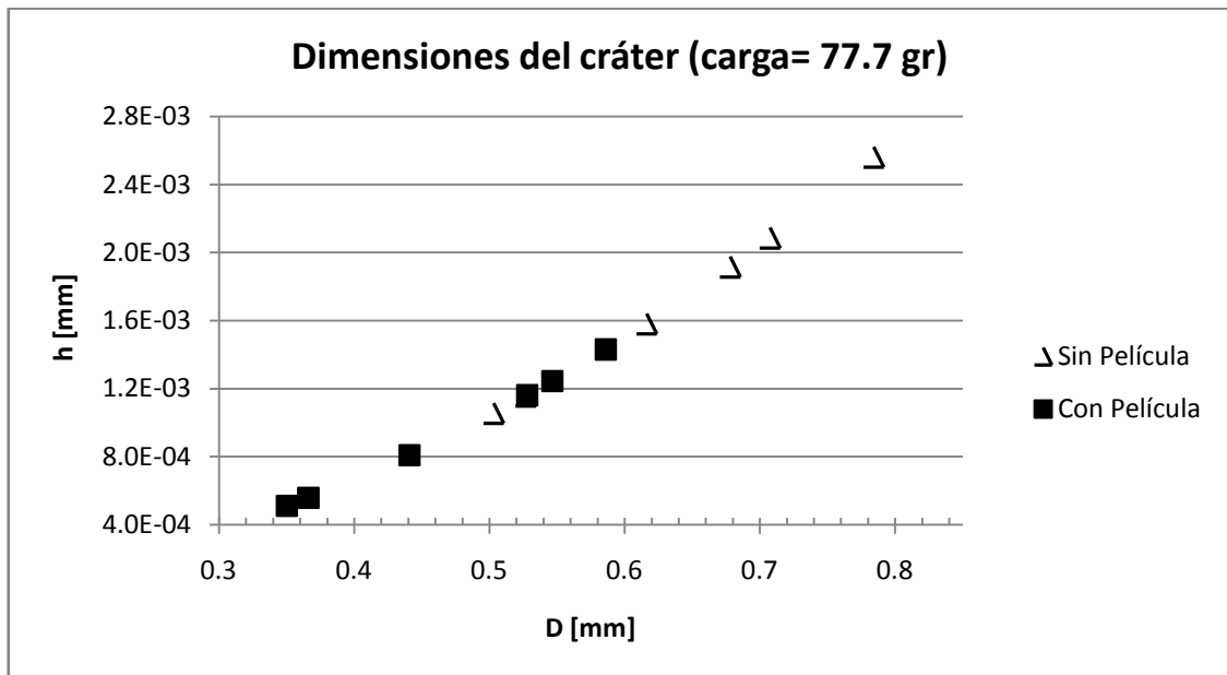
Gráfica A2.2 Relación diámetro(D) & profundidad del cráter(h) de las probetas con y sin recubrimiento, aplicando un peso de 77.7 [gr] en la prueba de Ball Cratering.
