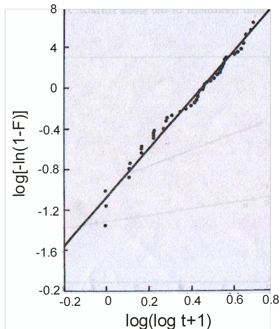
Gráfica 2. 7 Logaritmo de la probabilidad de los tiempos de falla en función de la fracción de muestras de barras Pyrex borosilicatado que fallan, para una humedad relativa de 65% y a una temperatura de 25°C [44].
