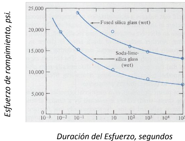
Gráfica 2. 1 Disminución en la resistencia de dos tipos de vidrio contra la respectiva duración de la carga aplicada (probetas húmedas) [43].
