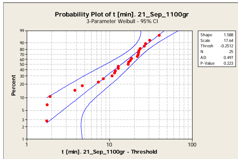
Gráfica 3.3 Gráfica de Probabilidad de Weibull-3 parámetros para los tiempos de falla de las probetas sin recubrimientos tratadas con el procedimiento del 21 de septiembre, sometidas a una carga de 1100gr en la prueba de flexión.
