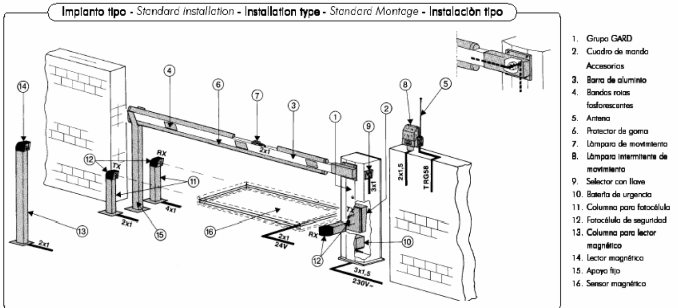
Figura 4.9. Instalación y características de la barrera vehicular a utilizar
