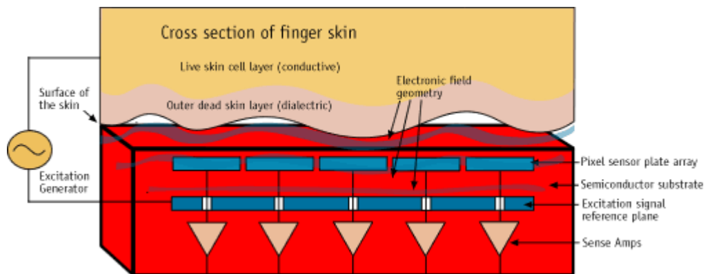
Figura 2.36.- Sensor de Matriz de Antena.
