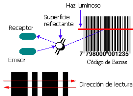
Figura 2.41.- Componentes principales en la lectura de un código de barras.
