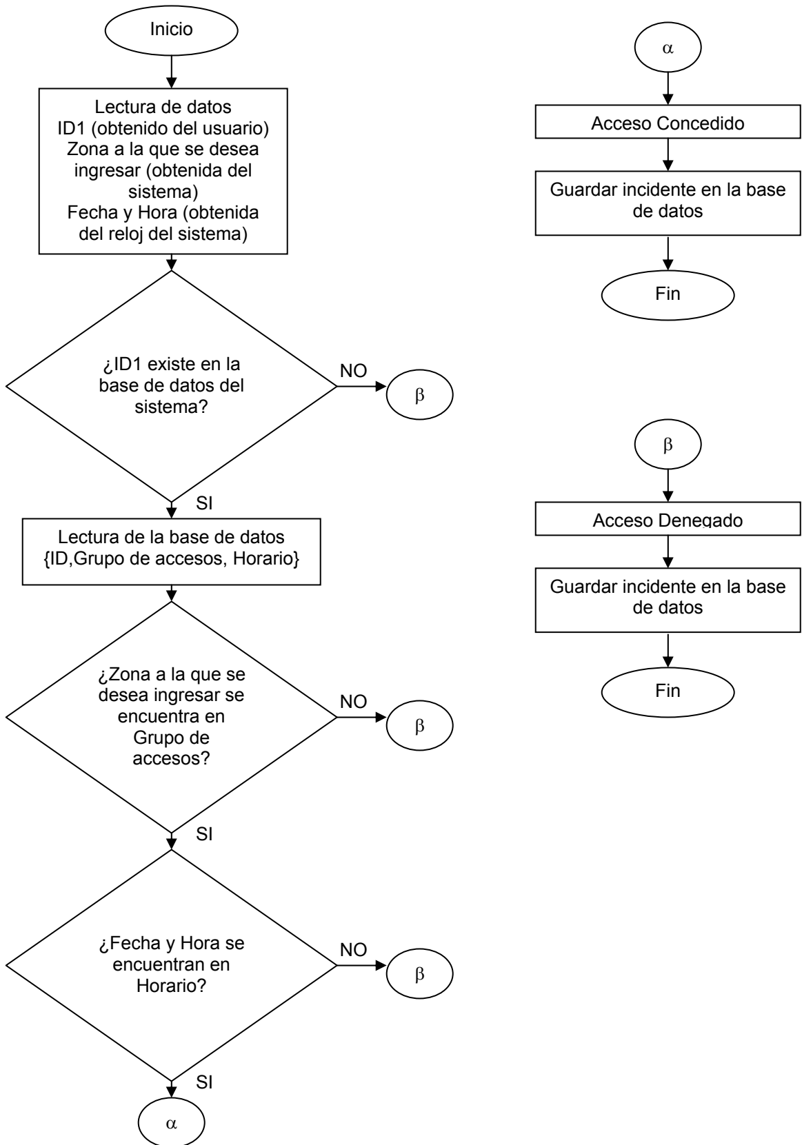
Figura 1.1.- Diagrama de Flujo del proceso de un sistema de control de acceso típico para conceder o negar un acceso
