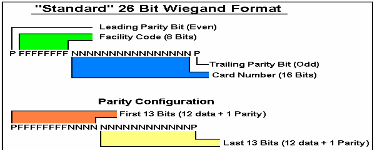
Figura 2.50.- Estructura del formato estándar Wiegand de 26 bit
