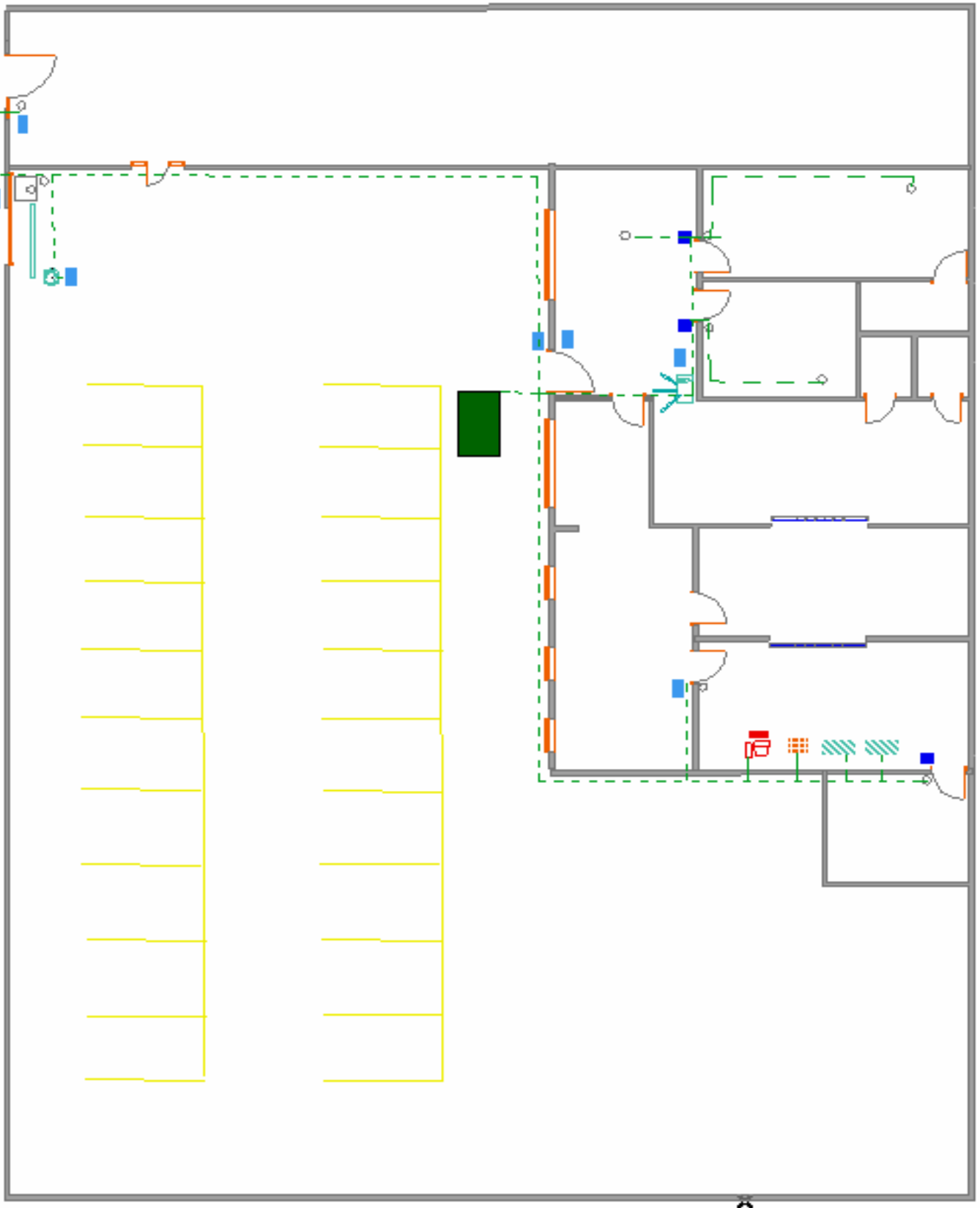
Figura 3.2.- Plano de D.S.C.A. proponiendo los elementos de sistema de control de acceso.
