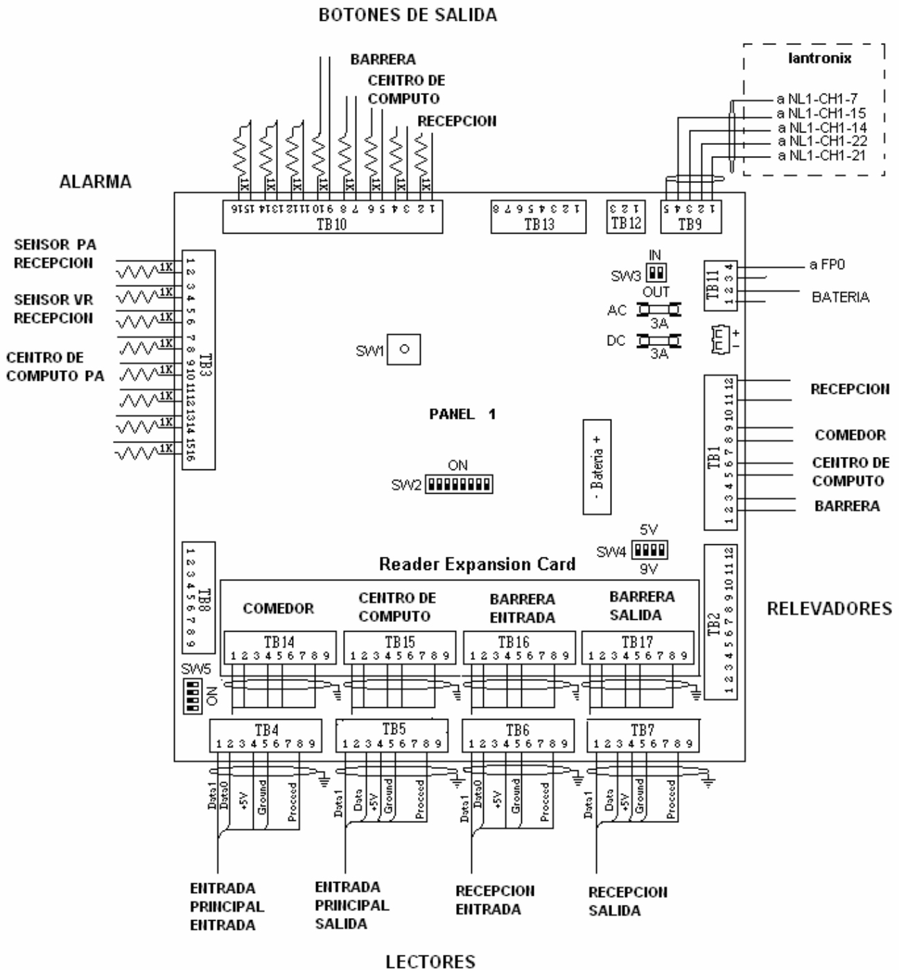
Figura 4.3. Diagrama de conexión del Panel 1
