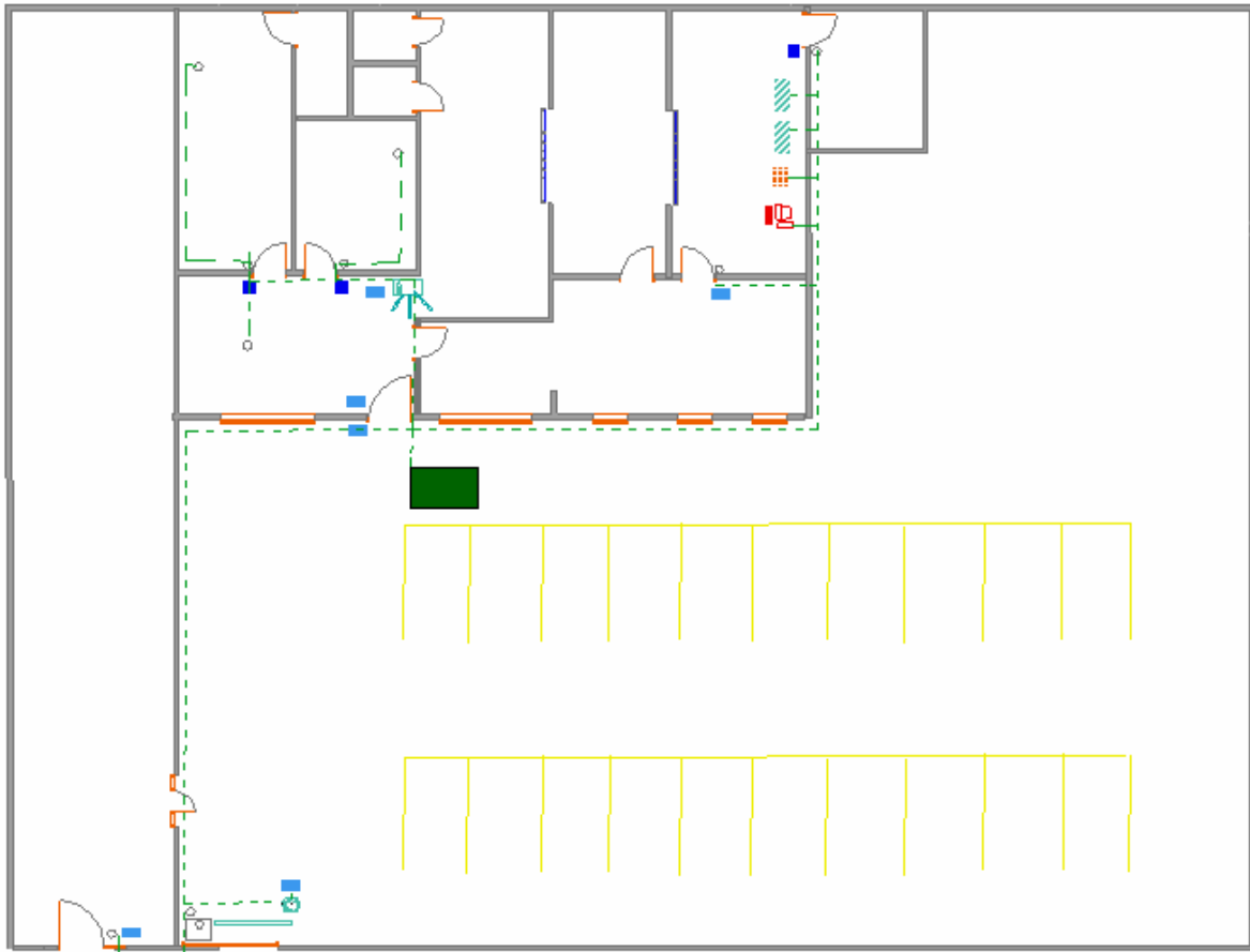
Figura 4.3. Plano de las Oficinas de D.S.C.A con cableado y dispositivos de control de acceso.
