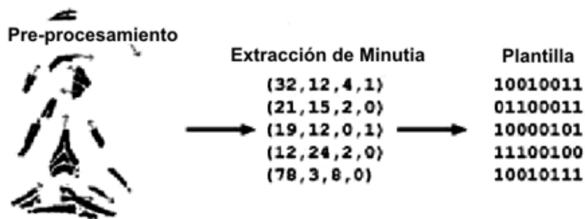
Figura 2.32.b.-Plantillas de una Huella.
