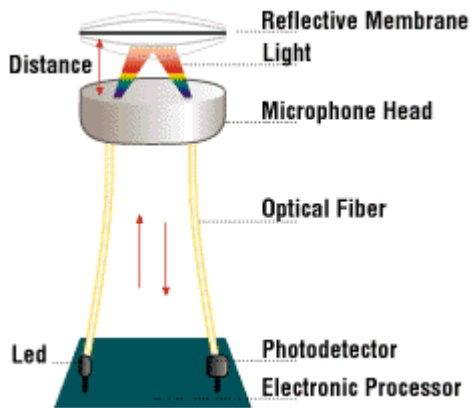
Figura 2.13.- Micrófono óptico.
