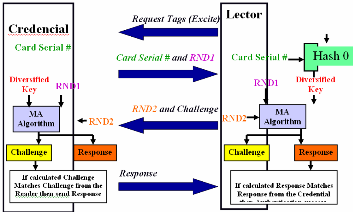
Figura 2.49.- Diagrama de Bloques del proceso de identificación.
