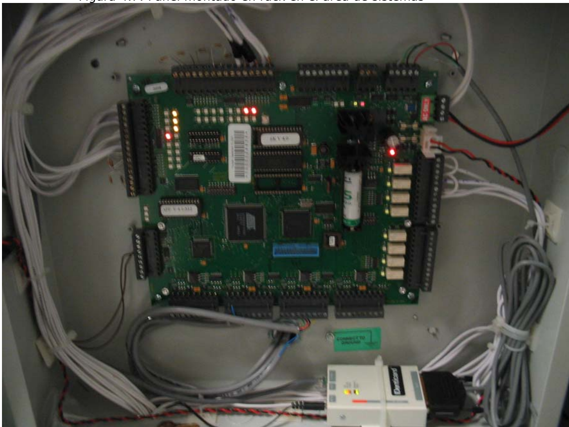
Figura 4.8 Panel 2 con todas las conexiones incluyendo el convertidor Serial/Ethernet Lantronix
