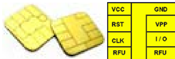
Figura 2.44.- Detalles de los chip en las tarjetas.
