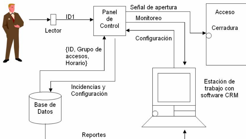
Figura 1.3.- Sistema de Control de Acceso Típico.
