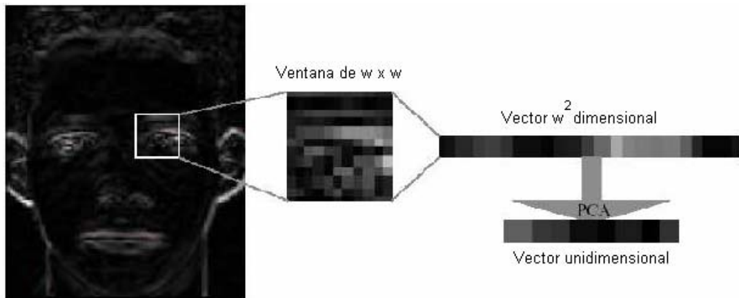
Figura 2.10- Obtención del vector unidimensional por medio del PCA.
