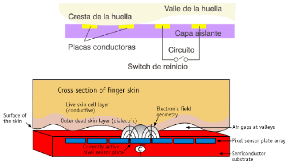
Figura 2.35.- Sensores capacitivos clásico
