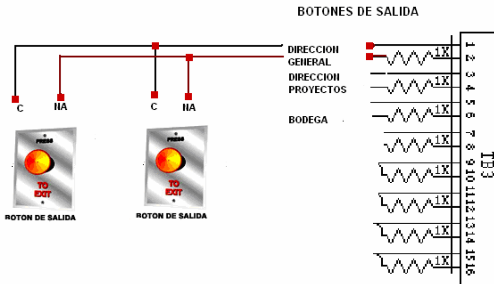
Figura 4.6. Conexión de los botones al panel
