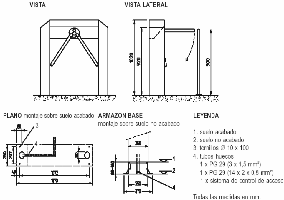
Figura 4.10. Instalación y características del torniquete.
