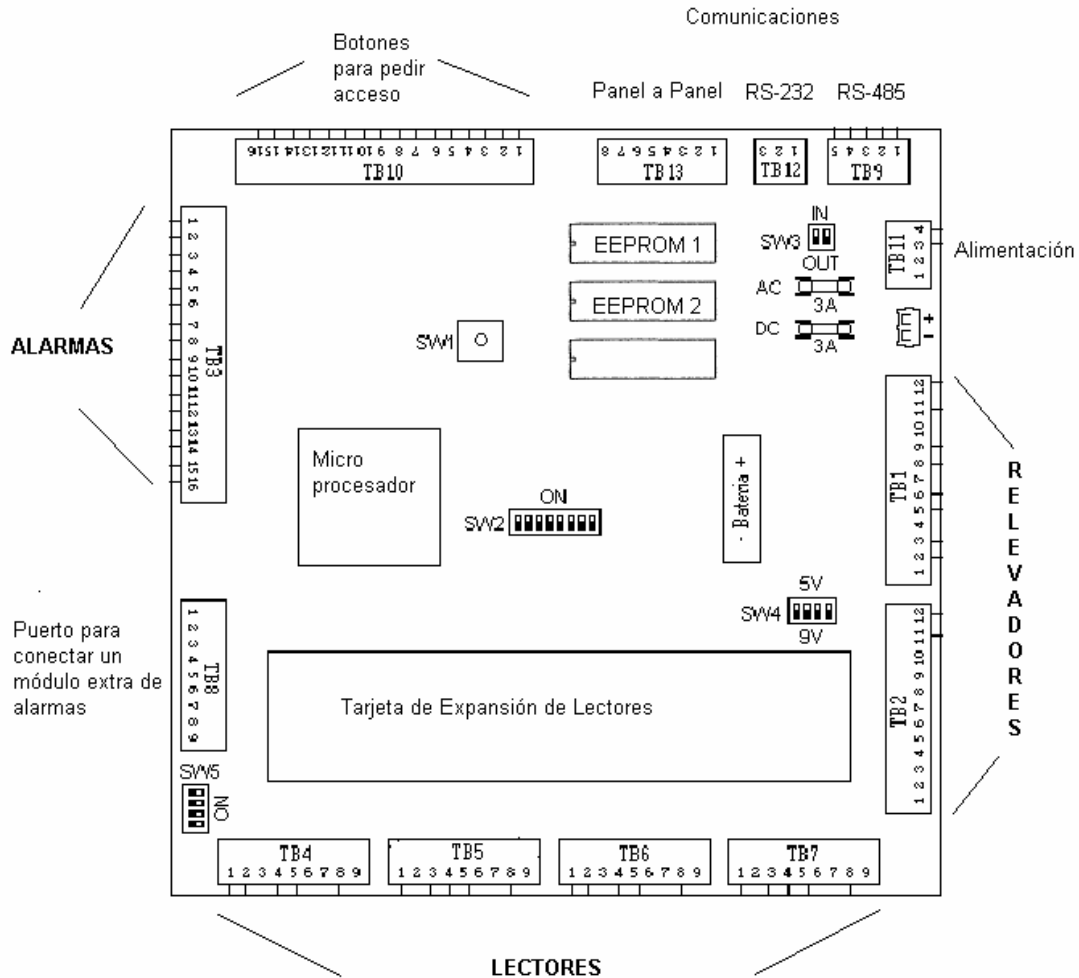
Figura 1.2- Diagrama de un panel de control comercial.
