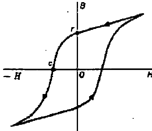
Figura 2.42.- Curva de Histéresis de los materiales ferromagnéticos.
