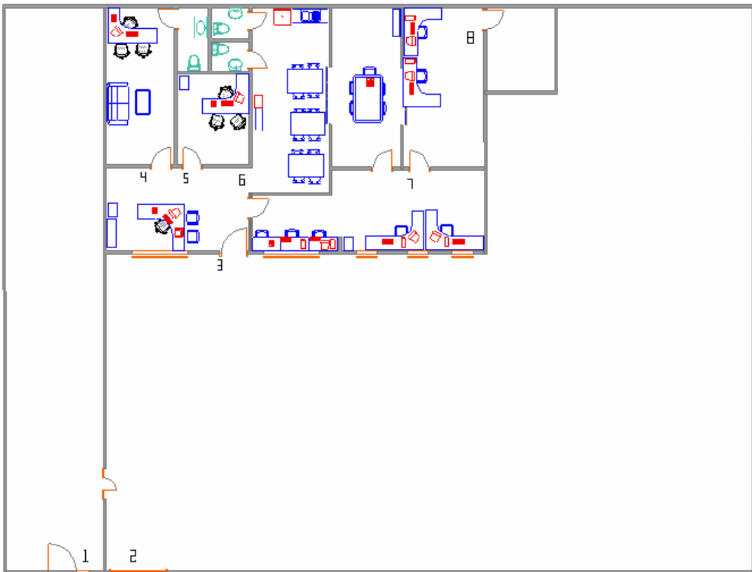
Figura 4.2. Plano arquitectónico de D.S.C.A
