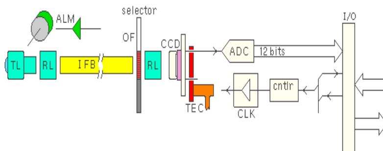
Figura 2.16.- Diagrama de bloques de la Cámara CCD.
