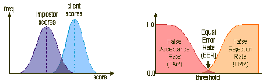
Figura 2.4.- Visualización de la unión de las dos distribuciones.
