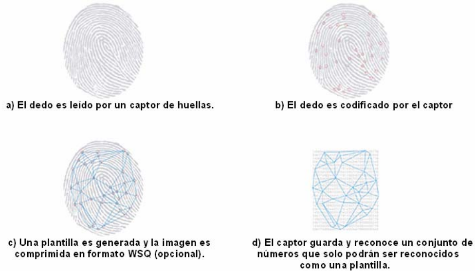
Figura 2.30.-Pasos del análisis de los puntos característicos.
