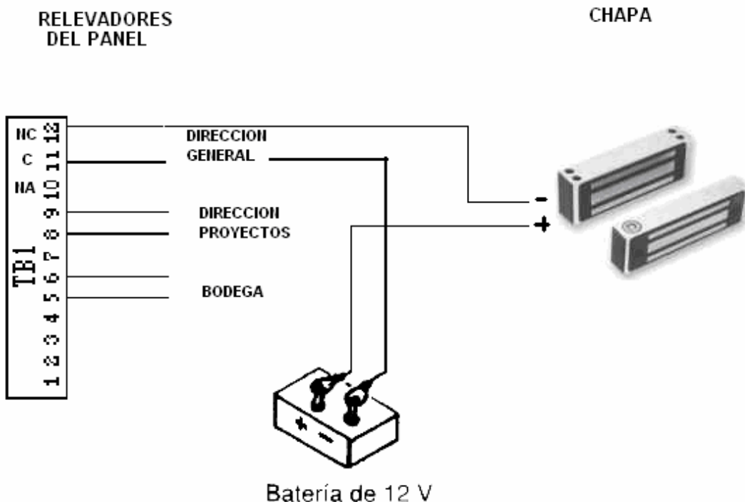
Figura 4.5. Conexión de los magnetos al panel
