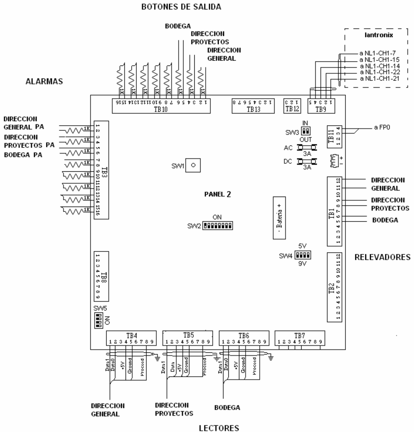
Figura 4.4. Diagrama de conexión del panel 2
