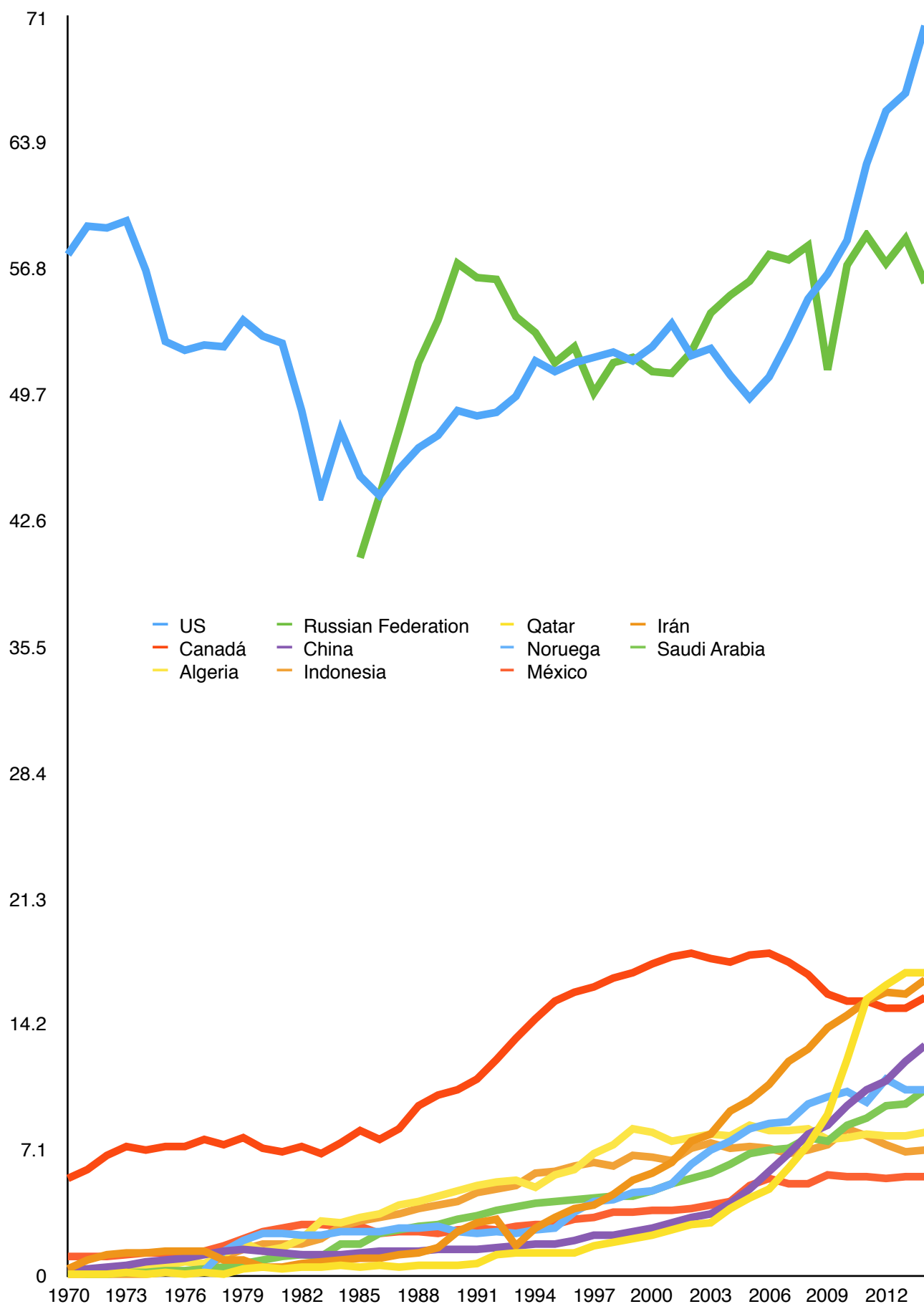
Figura 14 Producción histórica de los principales productores de gas natural (Bcf/d)
