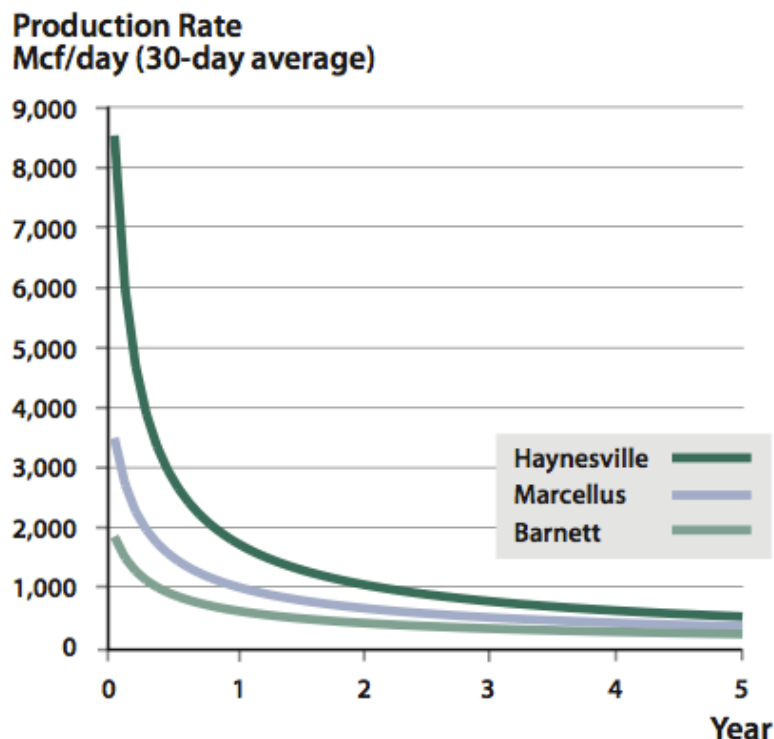
Figura 20 Perfiles de producción en Haynesville, Marcellus y Barnett
