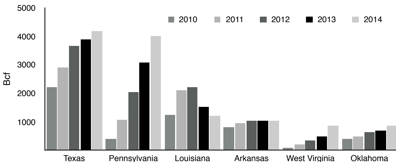
Figura 16 Distribución de la producción shale por estado
