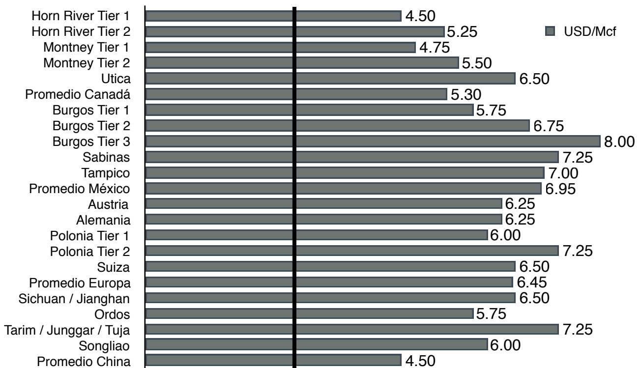
Figura 25 Break even prices alrededor del mundo
