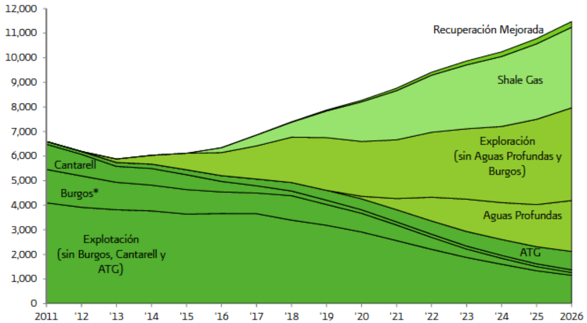
Figura 39 Producción de gas natural Escenario ENE 2012-2026 MMpc/d
