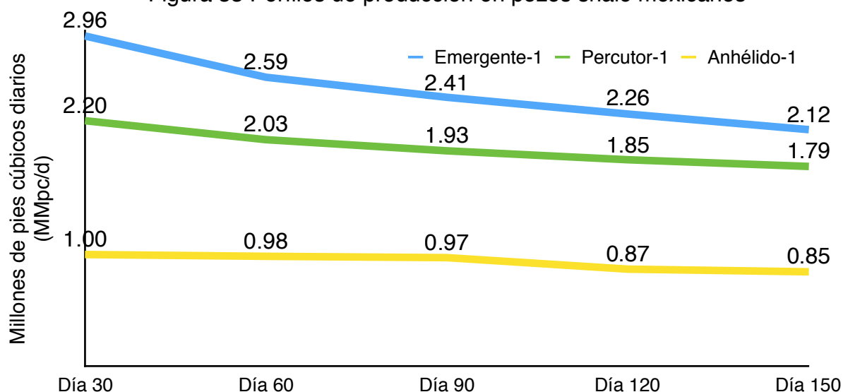
Figura 33 Perfiles de producción en pozos shale mexicanos
