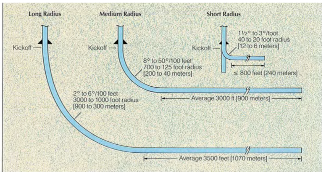
Figura 3 Tipos de pozos horizontales de acuerdo a su curvatura
