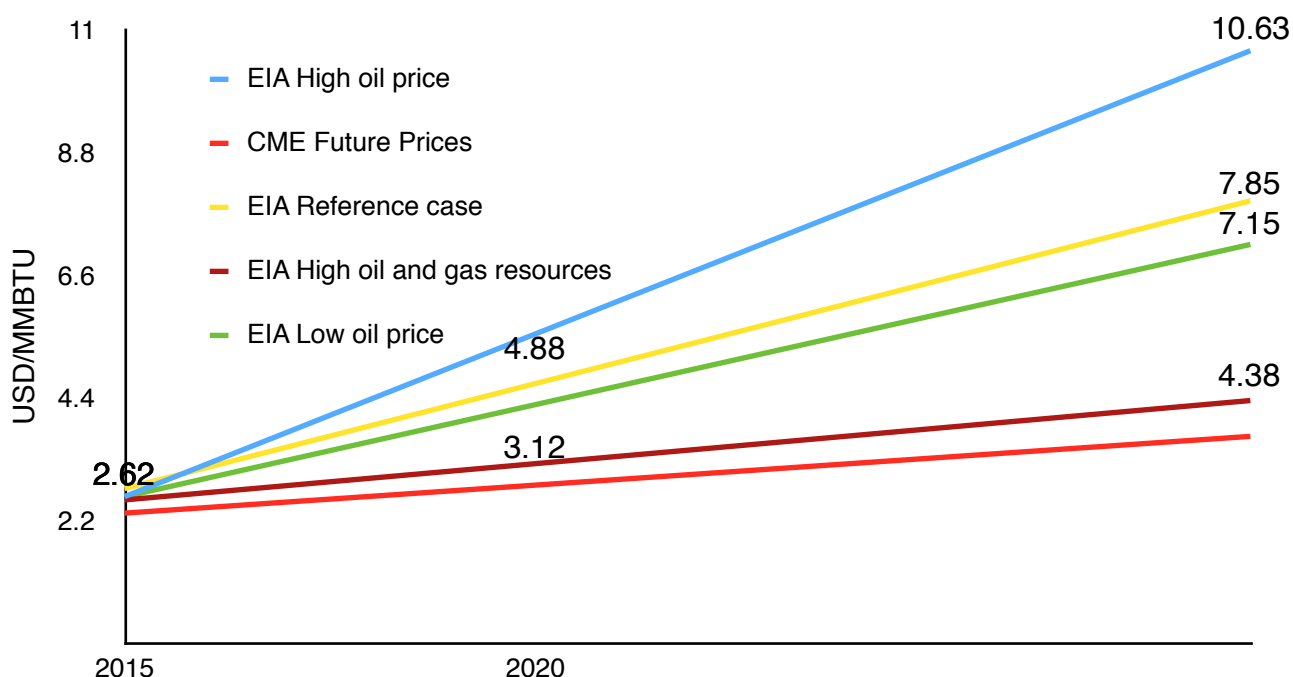
Figura 44 Evolución de los precios de gas natural en Henry Hub a)
