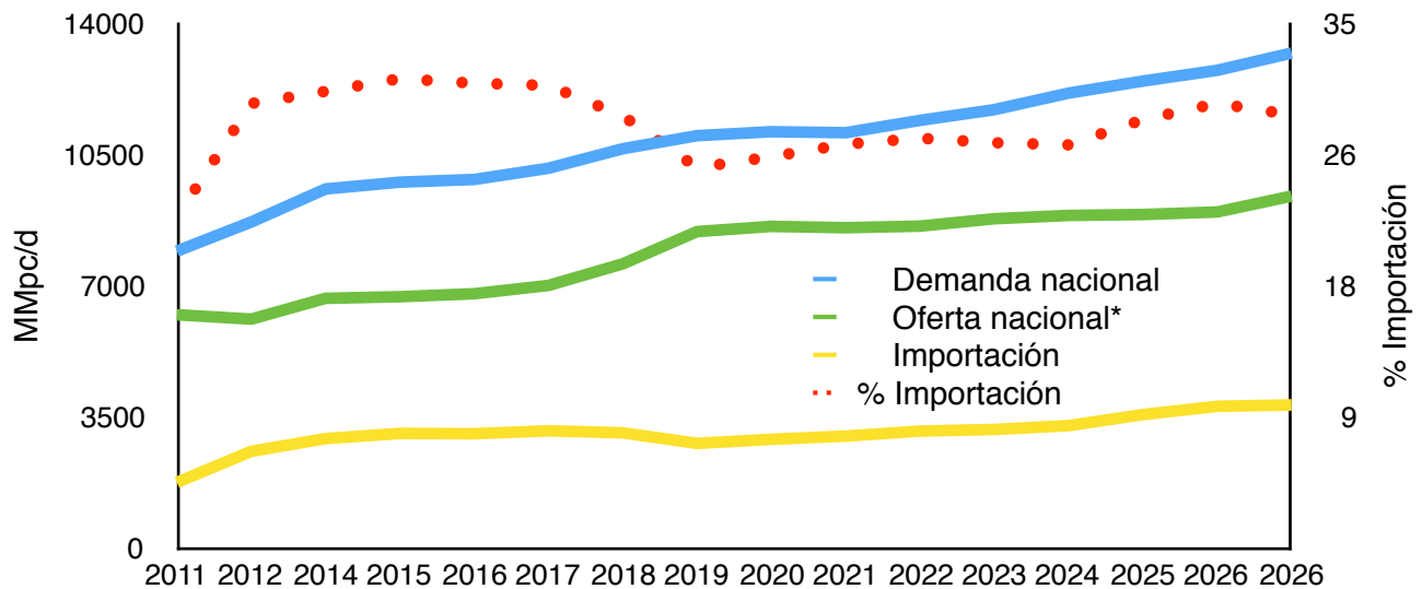
Figura 38 Balance de gas natural Escenario Inercial 2012-2026
