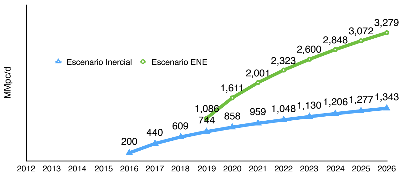
Figura 41 Escenarios de producción de gas natural shale 2012-2026
