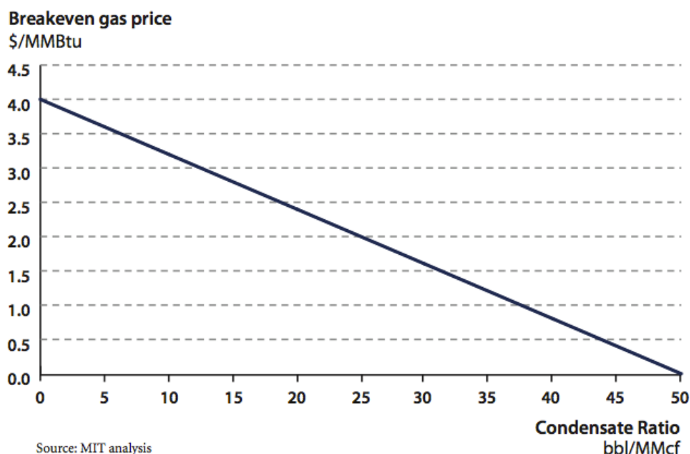
Figura 19 Influencia de los condensados en los break even prices
