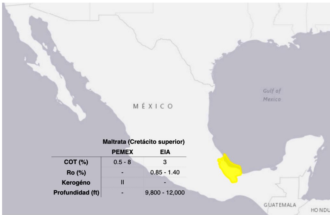
Figura 31 Ubicación y propiedades de la provincia Veracruz
