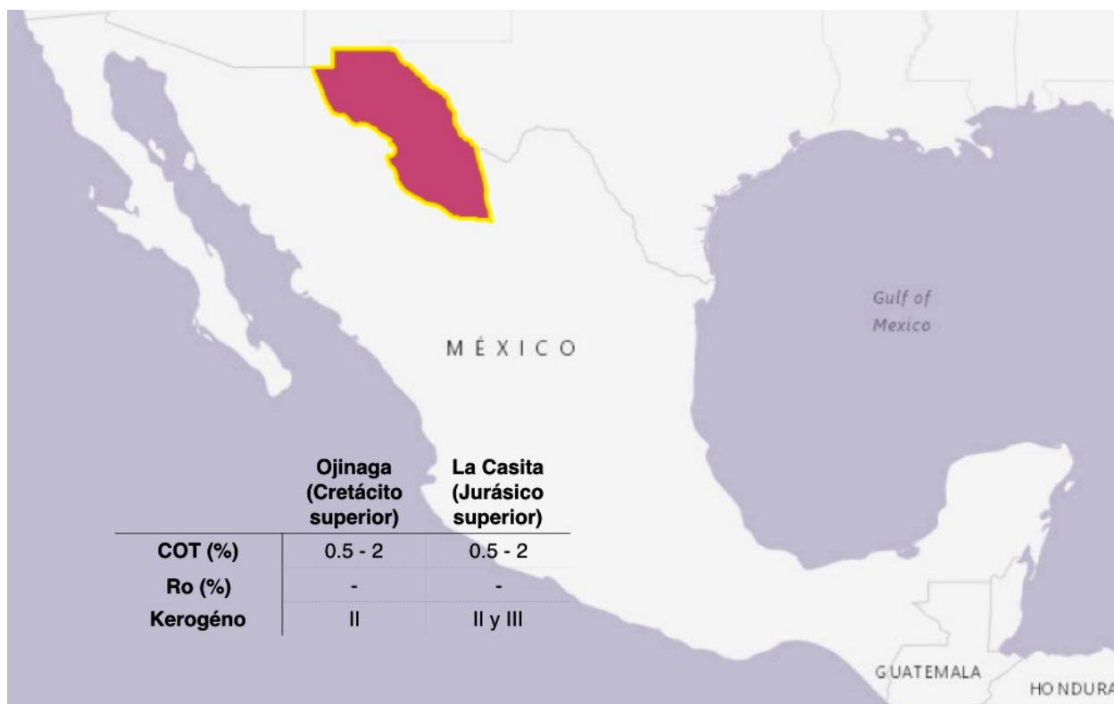
Figura 32 Ubicación y propiedades de la provincia Chihuahua
