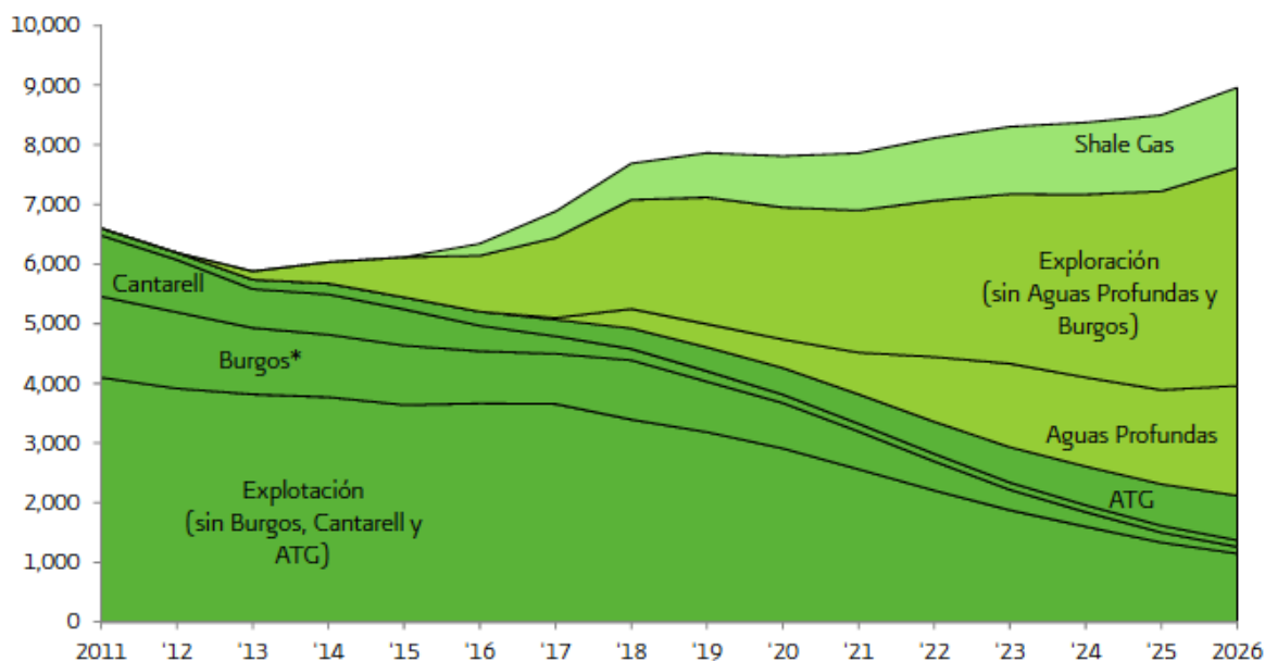
Figura 37 Producción de gas natural Escenario Inercial 2012-2026 (MMpc/d)
