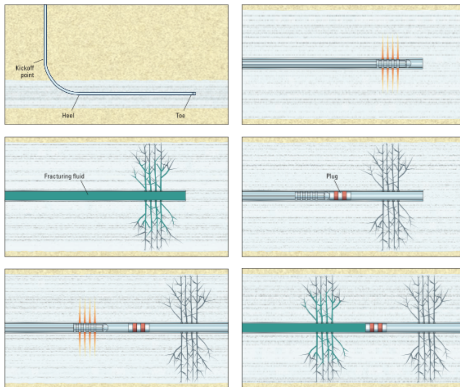
Figura 4 Técnica Plug and Peri
