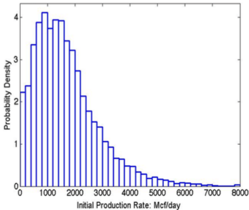
Figura 21 Distribución de probabilidad para la producción inicial de Barnett
