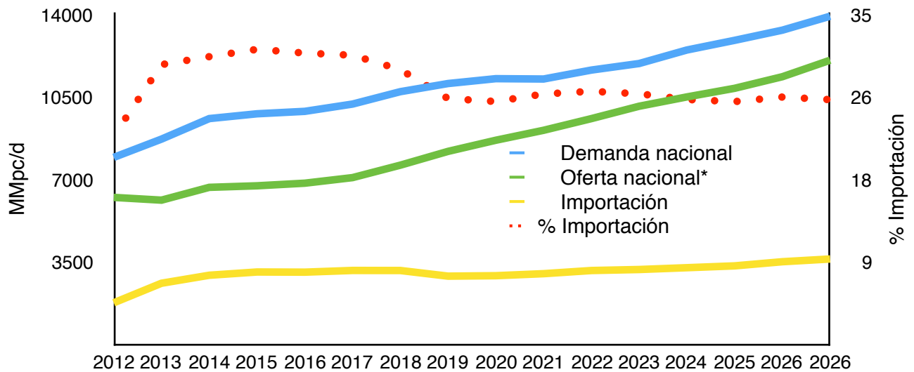
Figura 40 Balance de gas natural Escenario ENE 2012-2026
