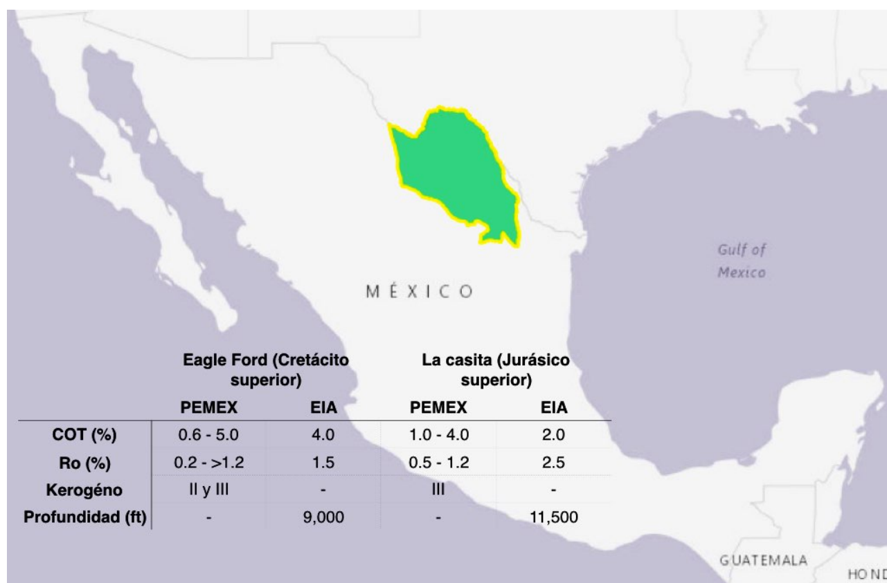
Figura 28 Ubicación y propiedades de la provincia Sabina-Burro-Picachos
