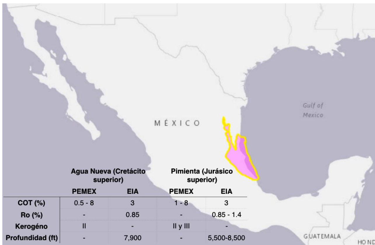
Figura 30 Ubicación y propiedades de la provincia Tampico-Misantla
