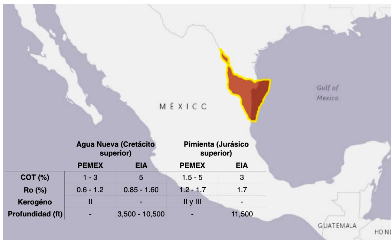
Figura 29 Ubicación y propiedades de la provincia Burgos
