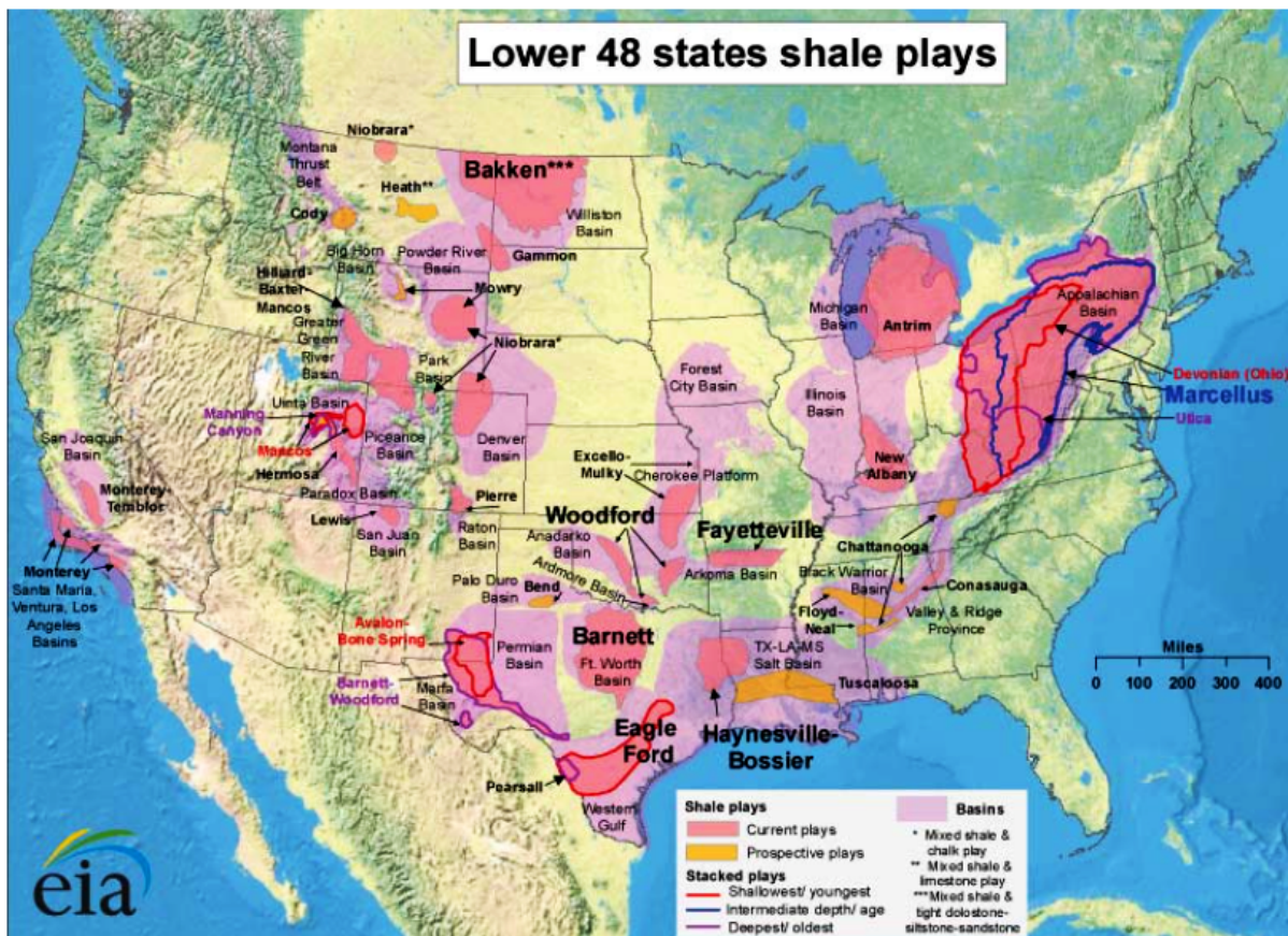
Figura 10 Distribución geográfica de las reservas shale en Estados Unidos.
