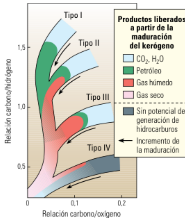
Figura 1 Diagrama de Van Krevelen
