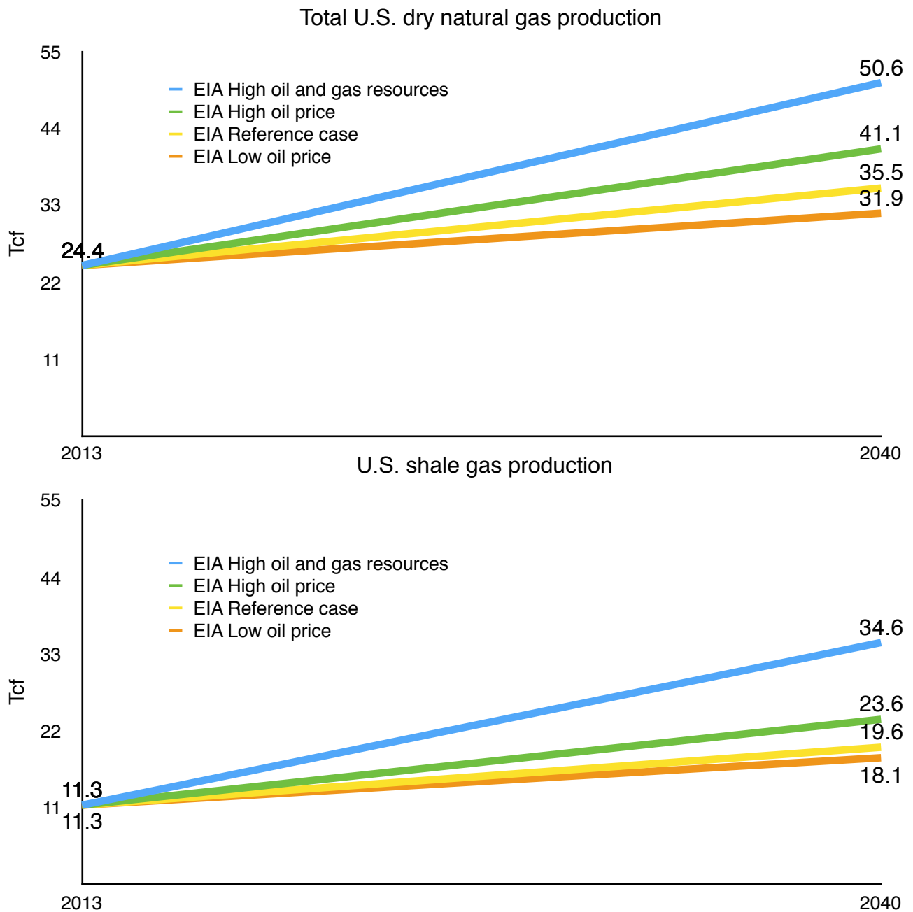
Figura 46 Escenarios de producción total y producción shale 2013-2040
