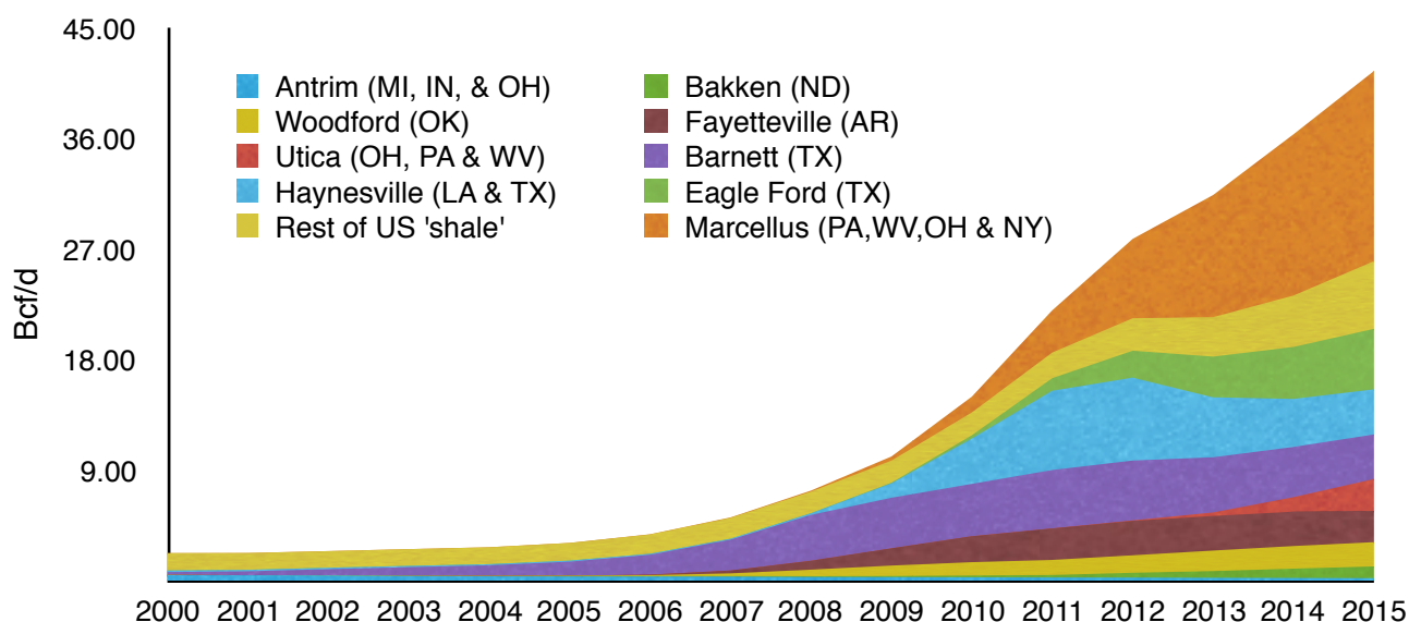
Figura 43 Producción diaria en las principales cuencas shale de EU
