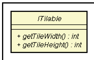
Figura 2.12: Diagrama de Clases, ITilable
