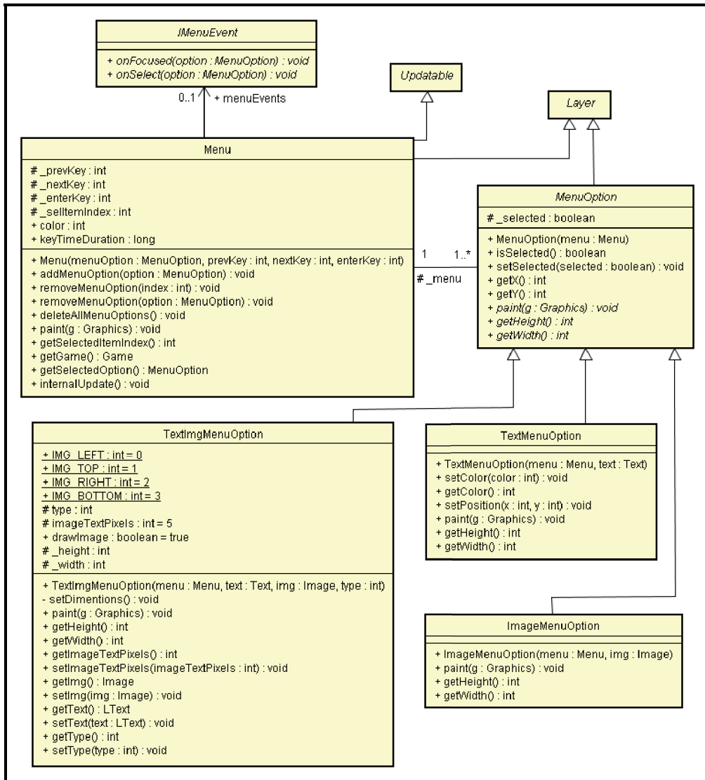
Figura 2.13: Diagrama de Clases, Menús
