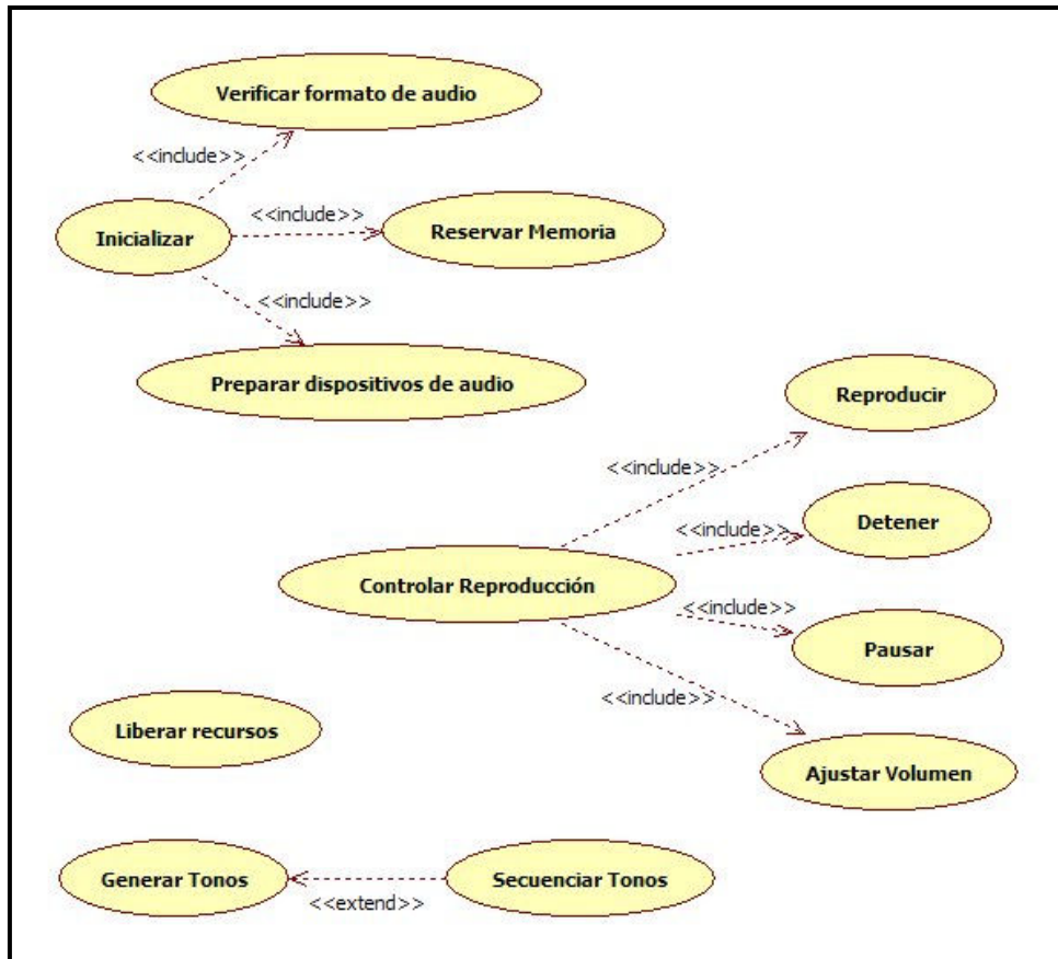
Figura 2.15: Casos de Uso, Módulo de Audio
