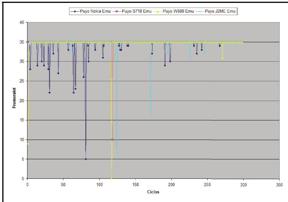
(a) Framerate limitado
