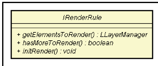
Figura 2.9: Diagrama de Clases, IRenderRule
