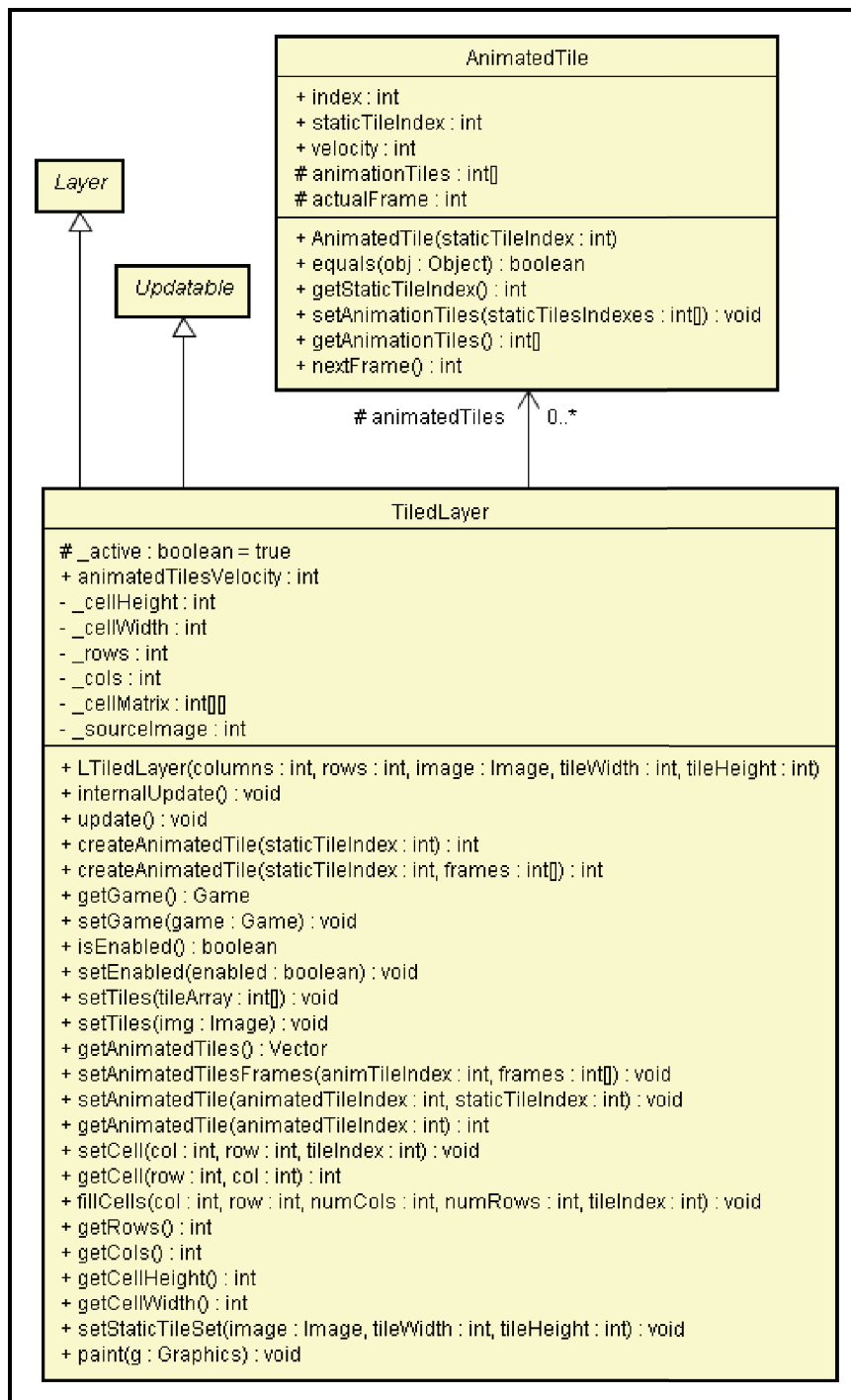
Figura 2.11: Diagrama de Clases, Tiles
