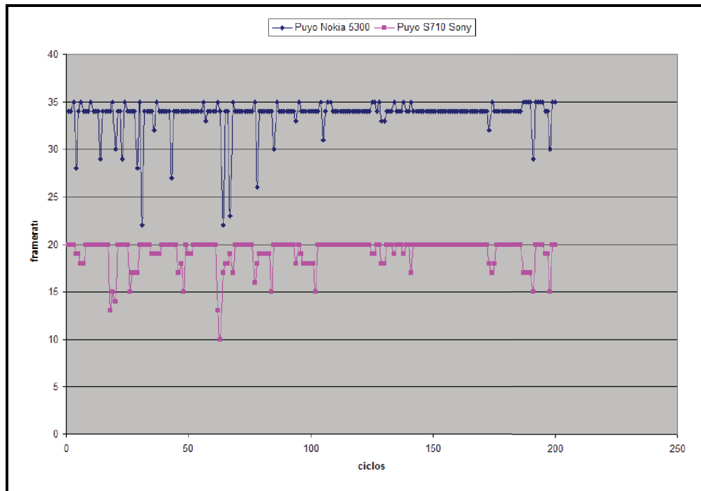
Figura 4.3: Framerates del Puyo celulares reales
