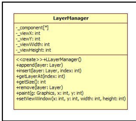
Figura 2.8: Diagrama de Clases, LayerManager
