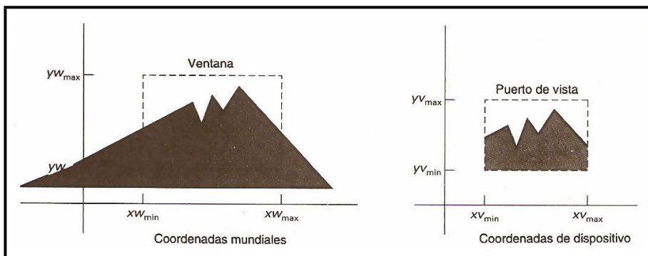
Figura 1.4: Ventana y Puerto de Vista
