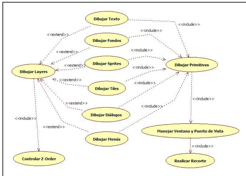
Figura 2.6: Diagrama de Casos de Uso, Módulo de Dibujo
