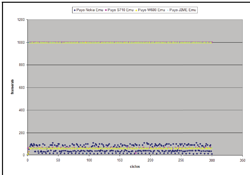
(b) Framerate libre
