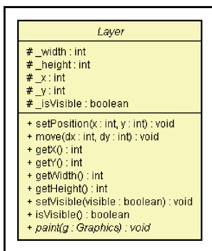
Figura 2.7: Diagrama de Clases, Layer
