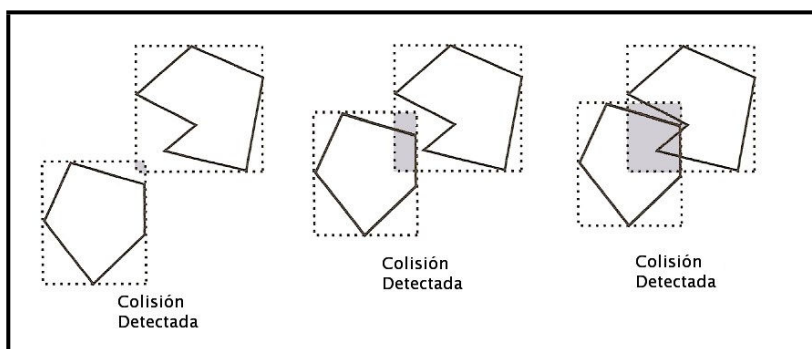
Figura 1.7: Colisión mediante rectángulos
