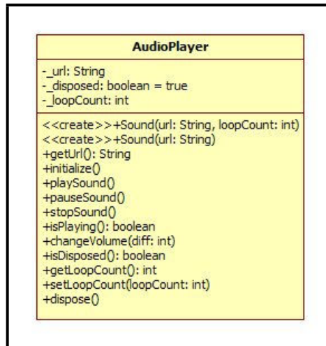
Figura 2.16: Diagrama de Clases, Módulo de Audio
