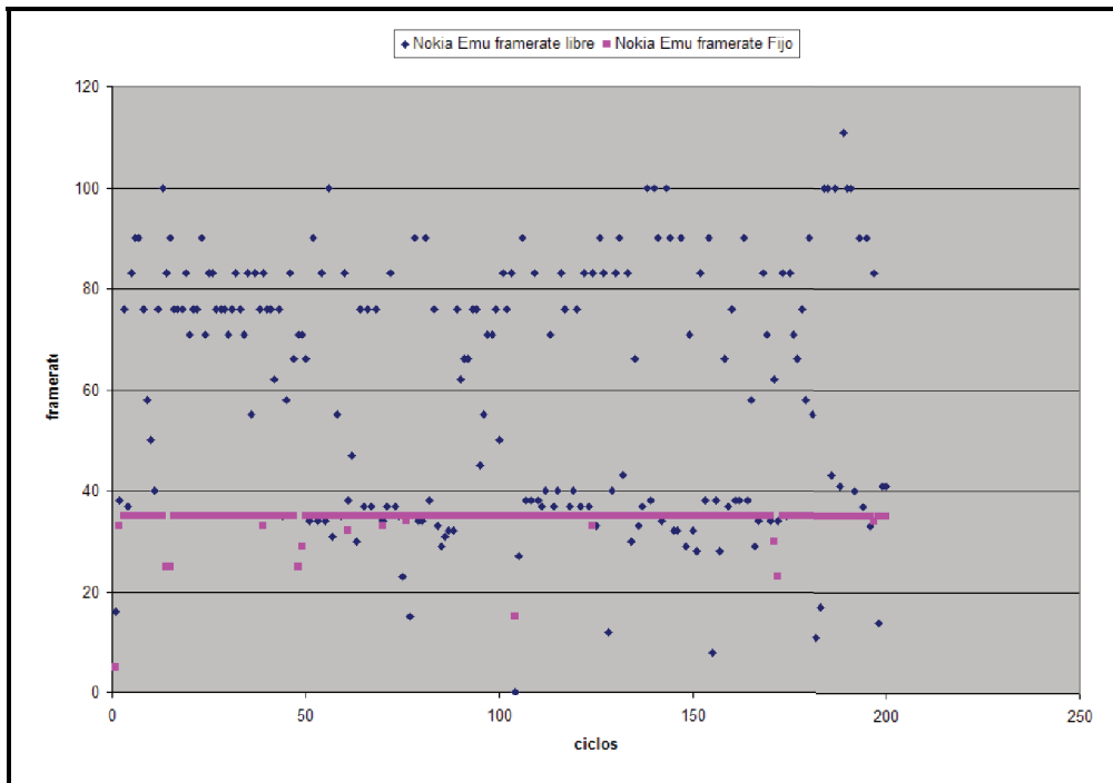
(a) Framerate Emulador de Nokia
