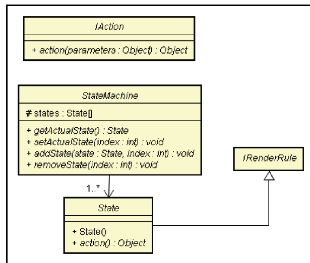
Figura 2.4: Diagrama de Clases, Paquete de Lógica
