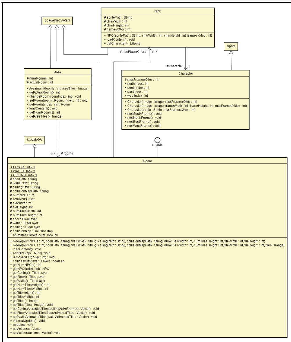
Figura 2.18: Diagrama de Clases, Paquete RPG
