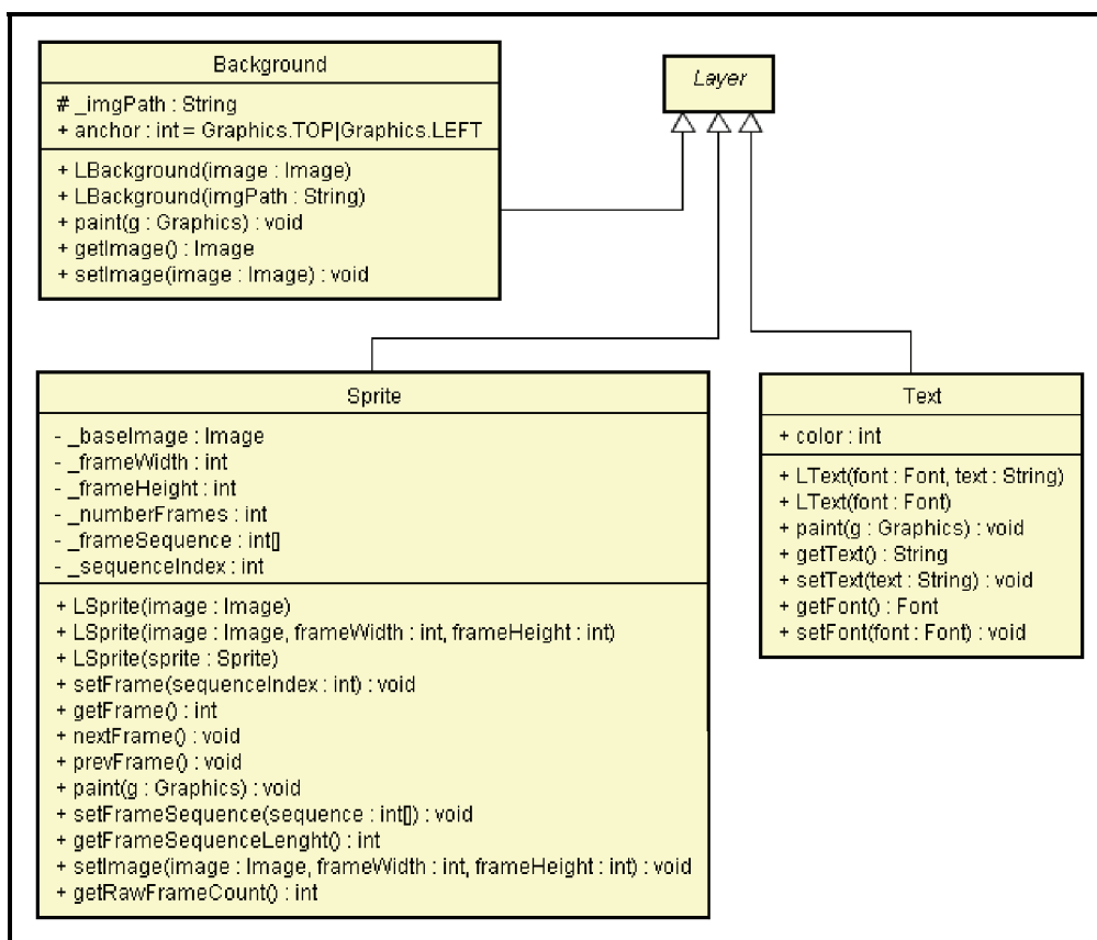
Figura 2.10: Diagrama de Clases, Elementos Gráficos Principales
