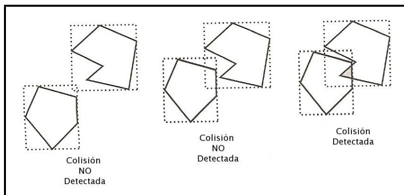
Figura 1.9: Colisión mediante verificación a nivel píxel
