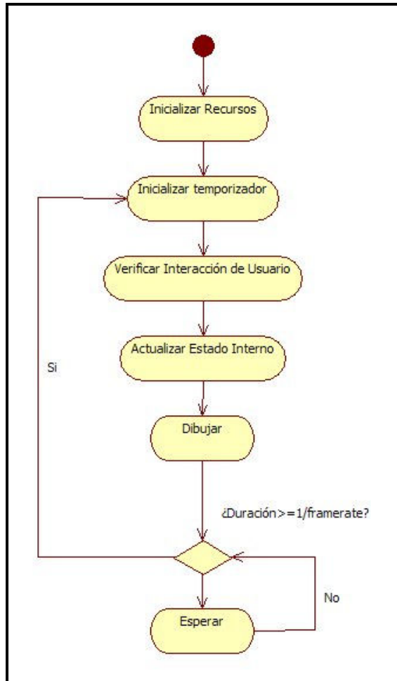
Figura 2.2: El Main Loop
