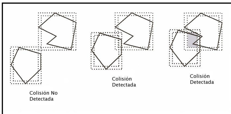
Figura 1.8: Colisión mediante rectángulos reducidos
