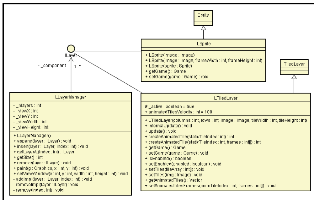
Figura 3.2: Diagrama de Clases, ILayers
