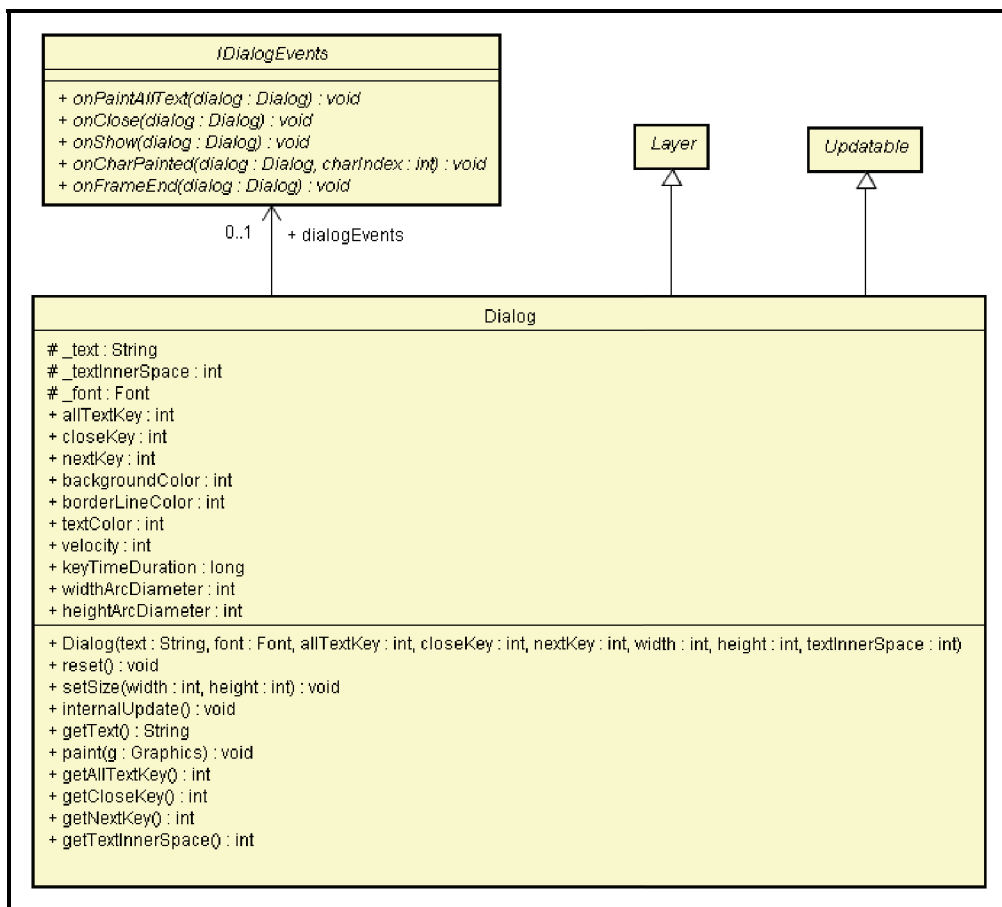
Figura 2.14: Diagrama de Clases, Diálogos
