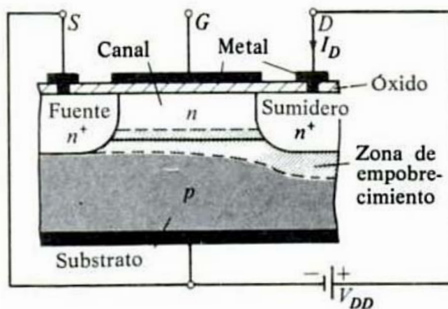
Figura II.7. La zona sombreada representa la zona de empobrecimiento entre las regiones tipo n y el sustrato.
