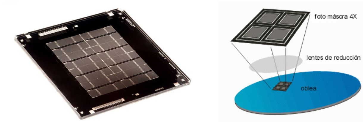
Figura III.19 Foto máscara
