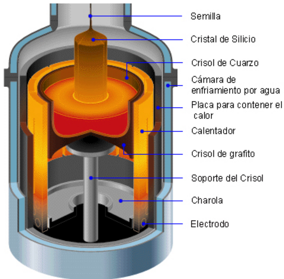
Figura III.3.10 Esquema de un Puller (2)
