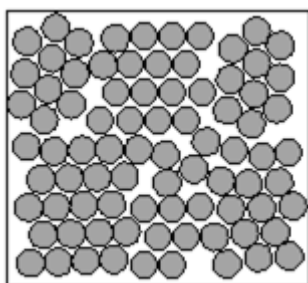
Estructura policristalina
