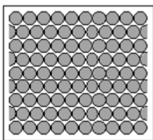
Estructura cristalina
