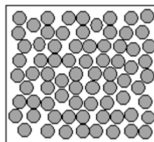
Estructura amorfa
