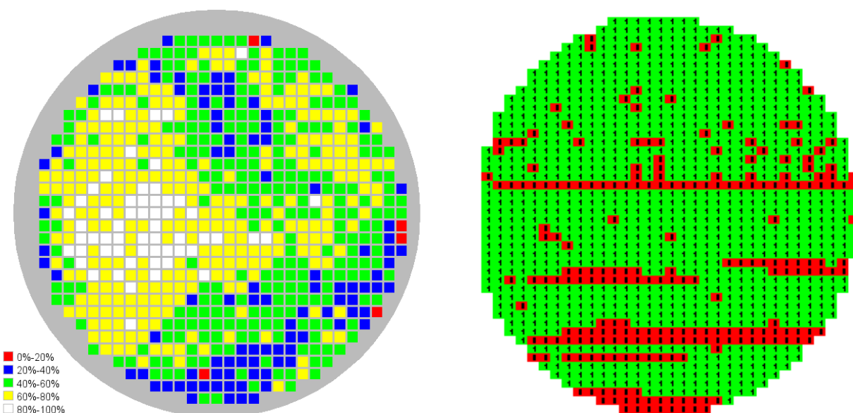
Figura III.39 Mapas de la oblea
