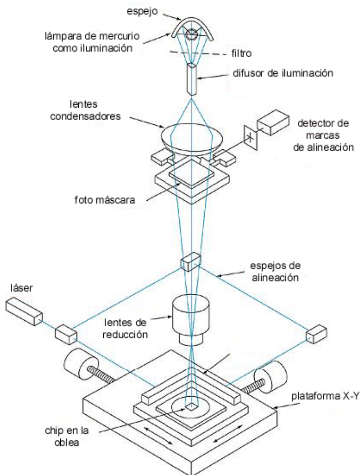
Figura III.20 Esquema de un sistema de alineamiento
