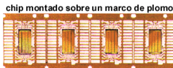
Figura III.43 Montaje de los chips en un marco de plomo
