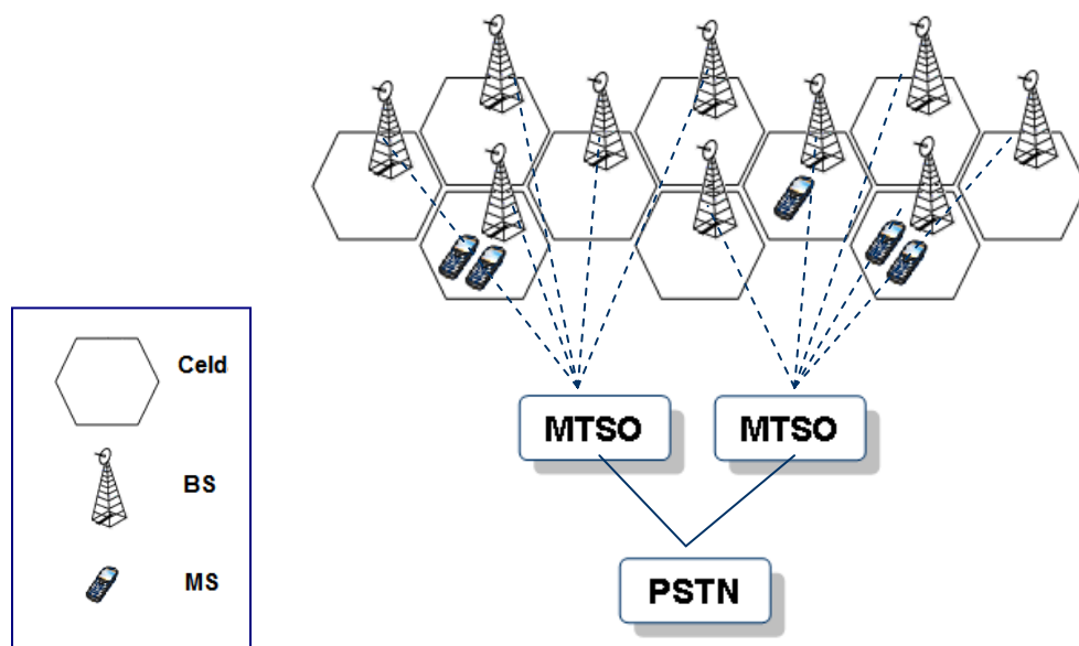
Figura IV.1. Red celular
