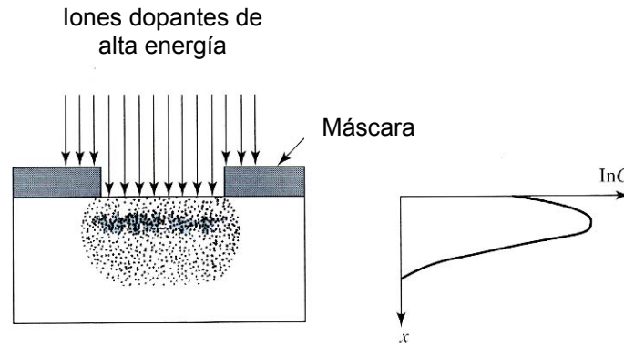
Figura III.30 Implantación Iónica
