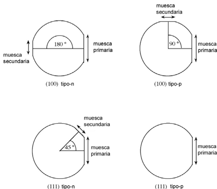
Figura III.13 Marcas para señalar la orientación del cristal.
