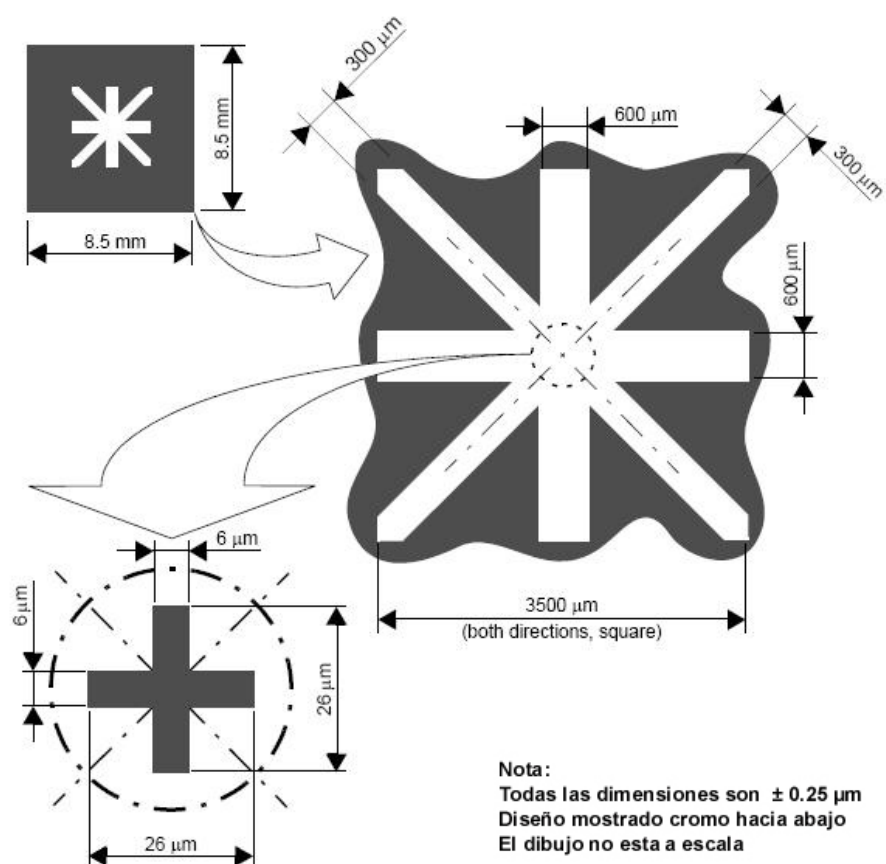
Marcas para prealineación de la mascara
