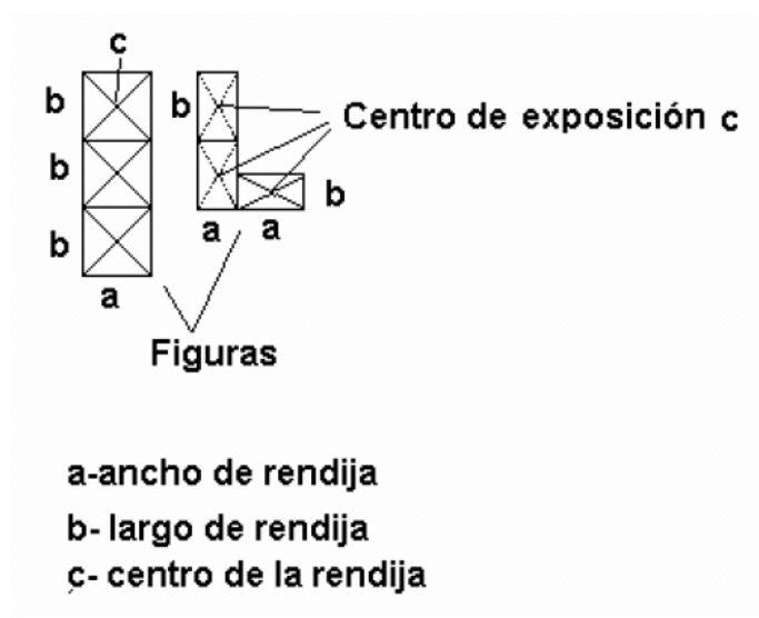
Figura III.3 Conformación de una figura por la exposición de un generador de patrones, mediante la yuxtaposición de rectángulos expuestos a través de una rendija de ancho a , largo b y centro situado en la posición c .
