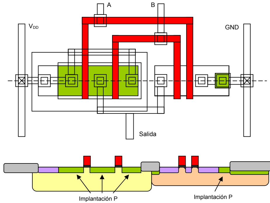
Figura II.27 Implantaciones P+
