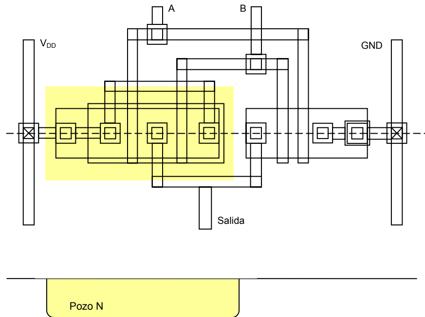
Figura II.22 Implantación de pozos N
