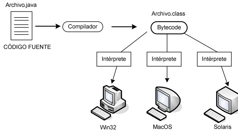
Figura 2.4 Esquema general de JAVA
