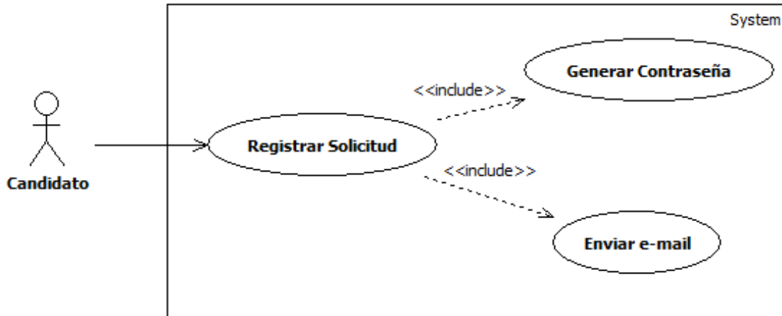
Figura 3.3 Diagrama de Casos de Uso: Registrar Solicitud
