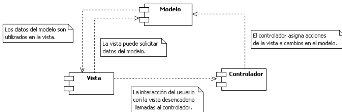
Figura 2.1 Componentes de MVC
