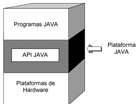
Figura 2.5 Plataforma JAVA
