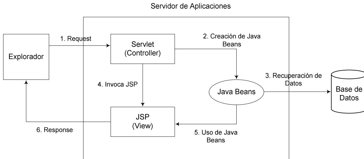
Figura 2.7 Modelo 2 de JSP
