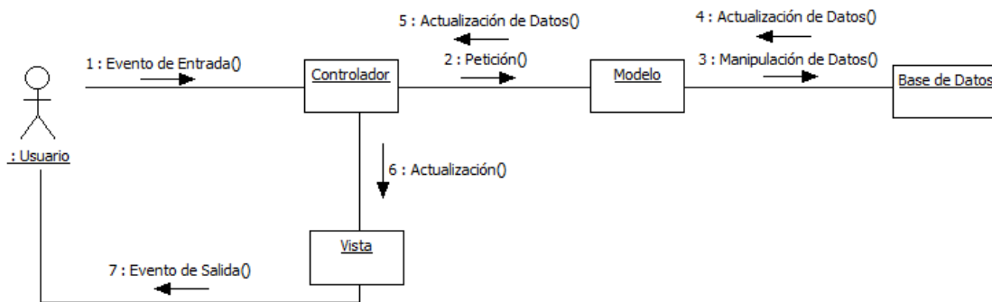
Figura 2.2 Interacción de los componentes MVC
