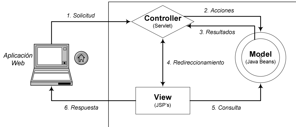
Figura 2.3 Interacción de los componentes de Struts
