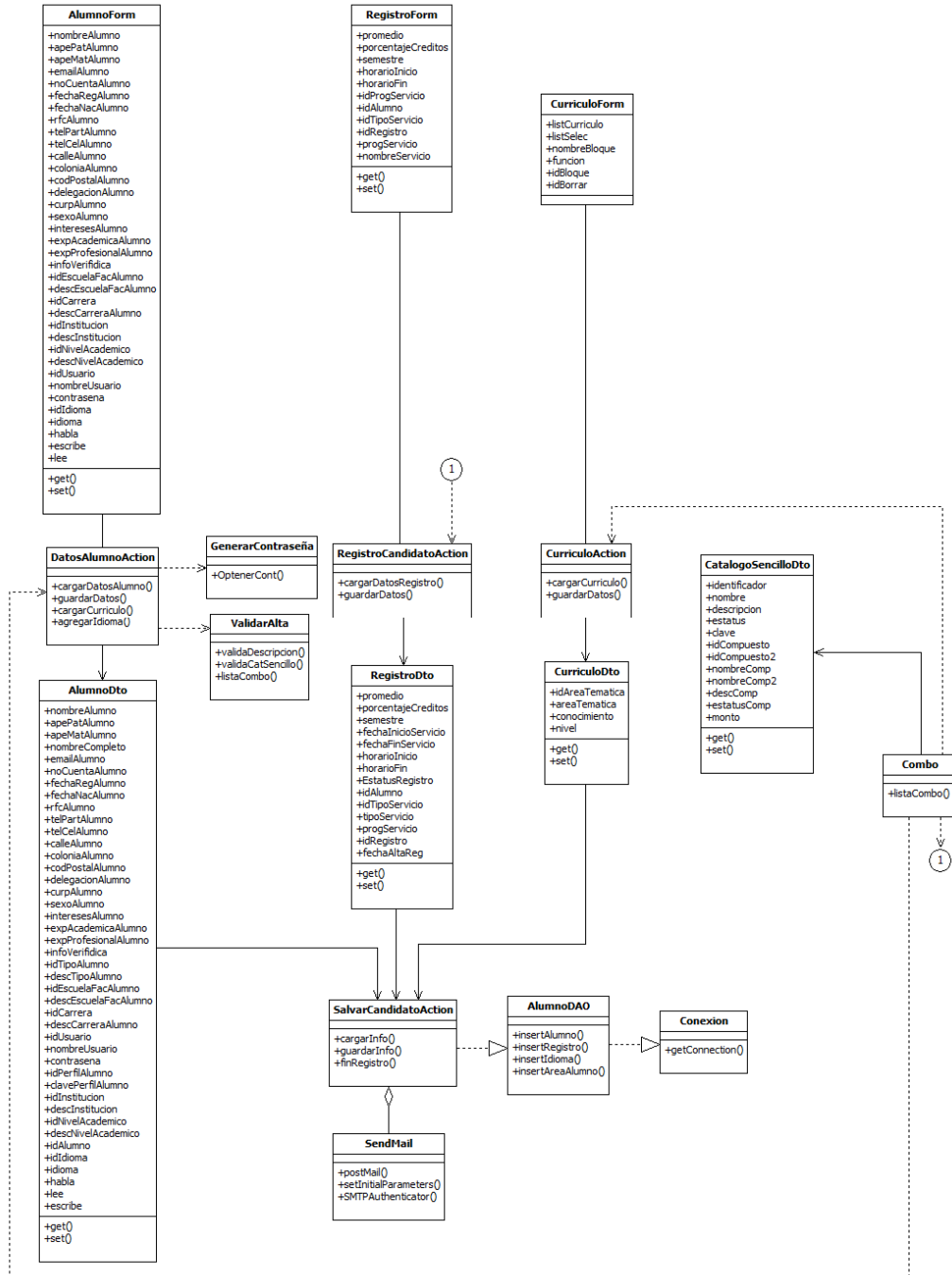
Diagrama de Clases: Registrar Solicitud
