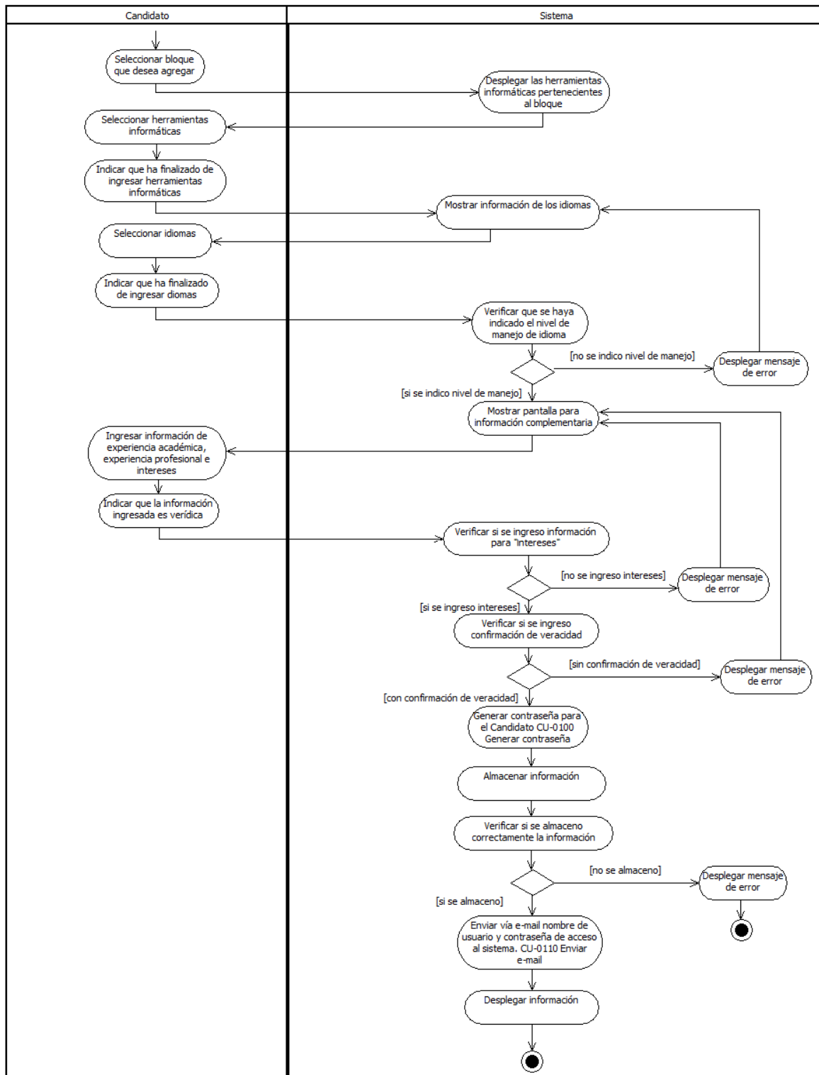
Figura 3.1 Diagrama de Actividad: Registrar Solicitud
