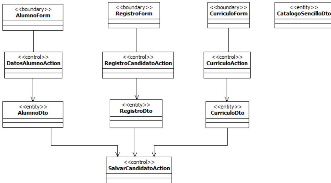
Figura 4.9 Diagrama de Clases: Registrar Solicitud
