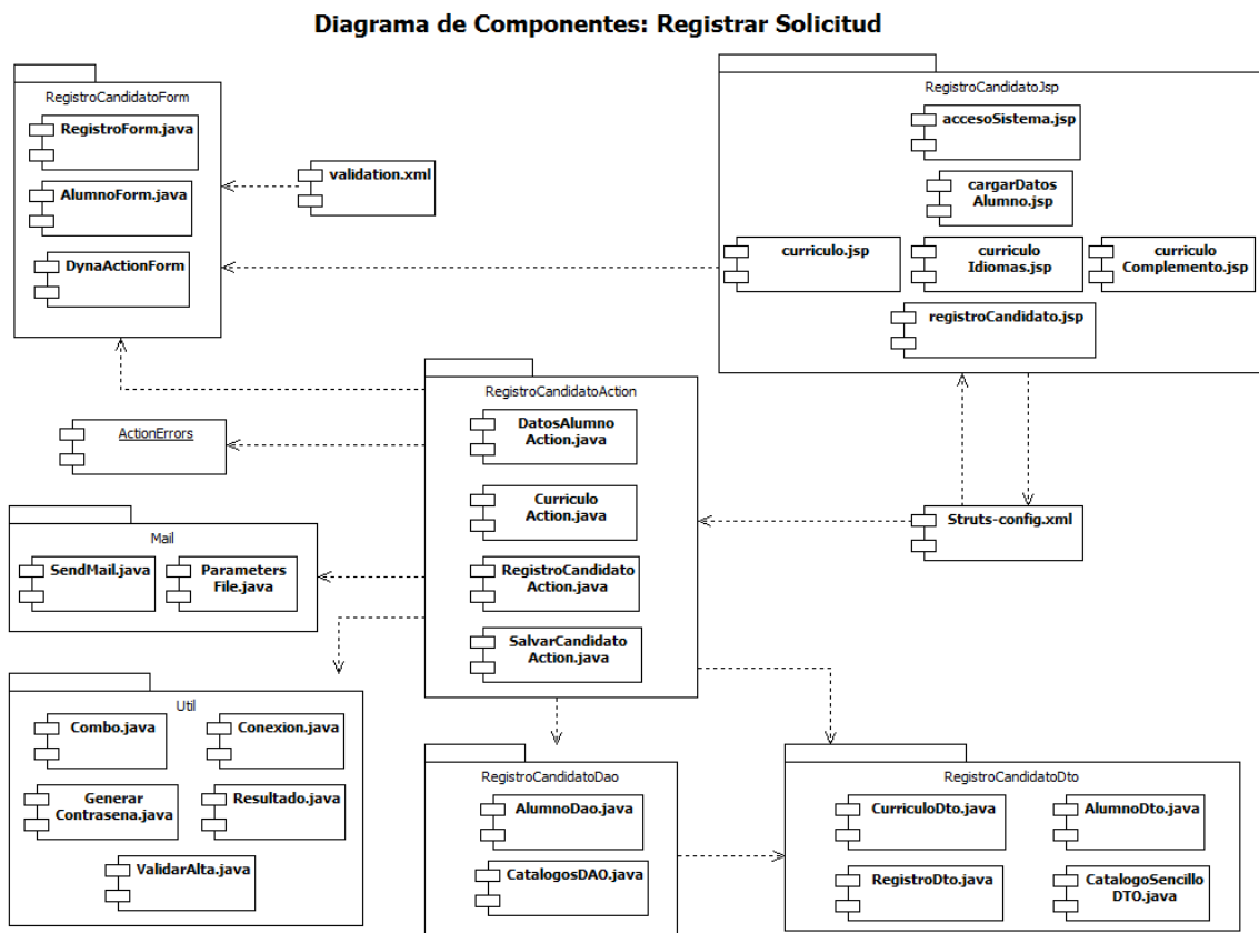
Figura 4.11 Diagrama de Componentes
