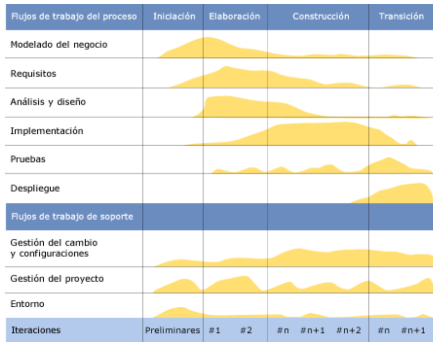
Figura 2.8 Metodología RUP
