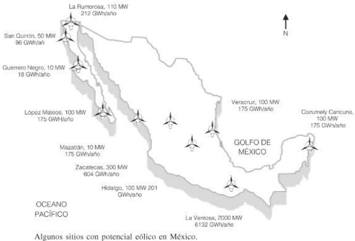
Figura 4. Fuente: Potencial de aprovechamiento de la energía eólica para la generación de energía eléctrica en zonas rurales de México Interciencia abril. Año 2006/vol. 31
