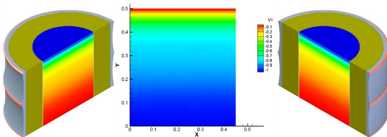
Figura 5.15: Velocidad de la fase gaseosa a través del gasificador.
