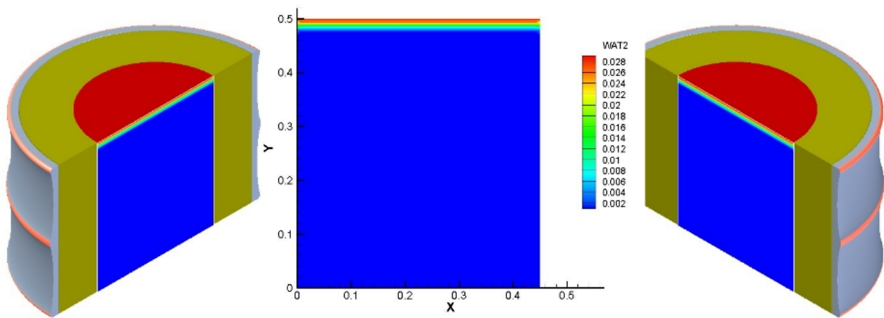
Figura 5.1: Cambio de la fracción másica de agua presente en la biomasa a lo largo del gasificador.
