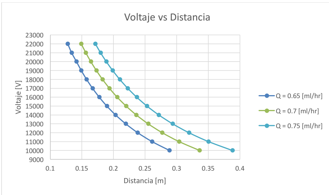
Figura 8.3 Gráfica parámetros de electrohilado con valores reales.
