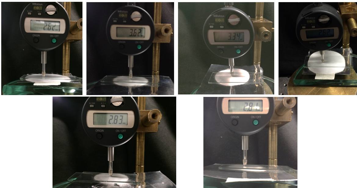
Figura 5.12 Medición de espesor de las membranas electrohiladas de PMMA.
