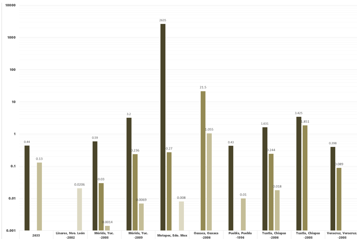
Gráfica 2. Comparativa en escala logarítmica de la presencia de 4 metales de acuerdo a las mediciones en 8 rellenos sanitarios en México.
