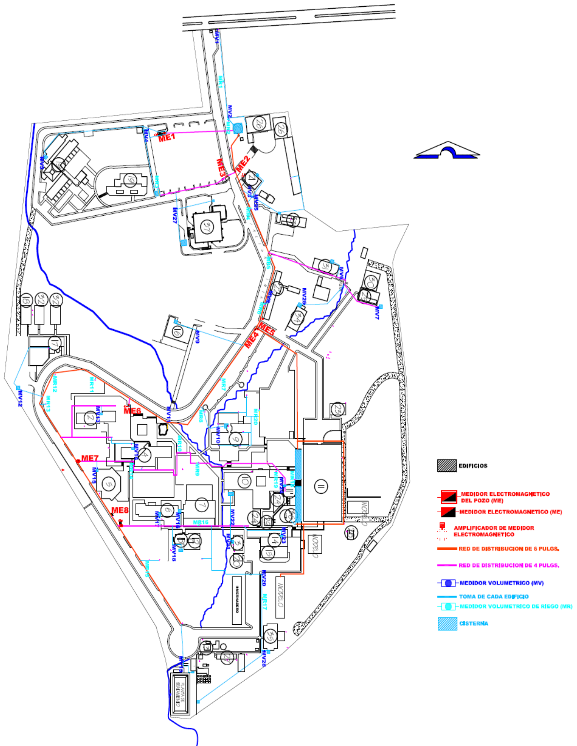
Figura 24: Localización de medidores volumétricos.
