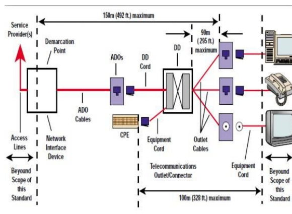
Figura 1.71: Componentes del cableado para voz, datos y video.
