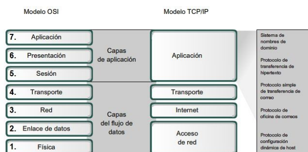
Figura 1.25: Comparativo de los modelos TCP/IP y OSI
