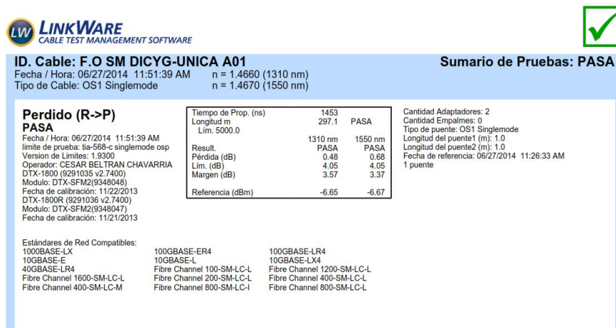
Figura 3.26: Mediciones con equipo Flike DTX-180
