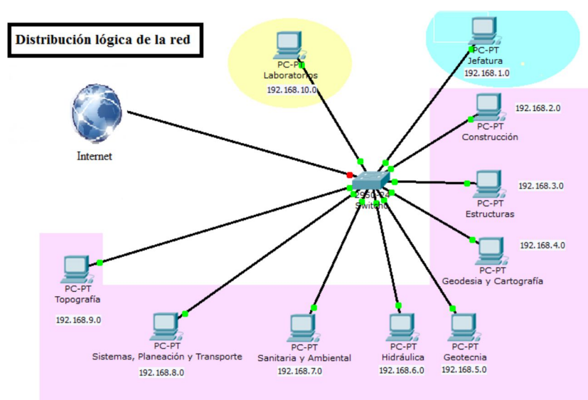
Figura 3.44: Esquema de Red por segmentos.
