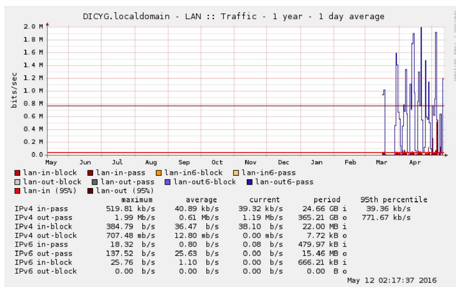
Figura 4.3: Tráfico de red por año
