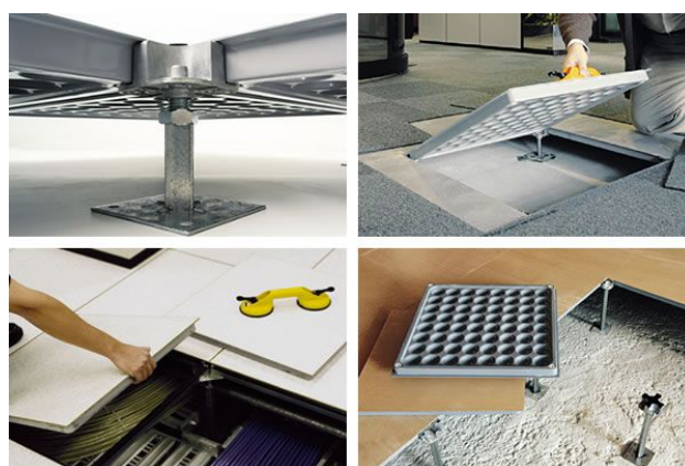
Figura 1.68: Suelo técnico.
