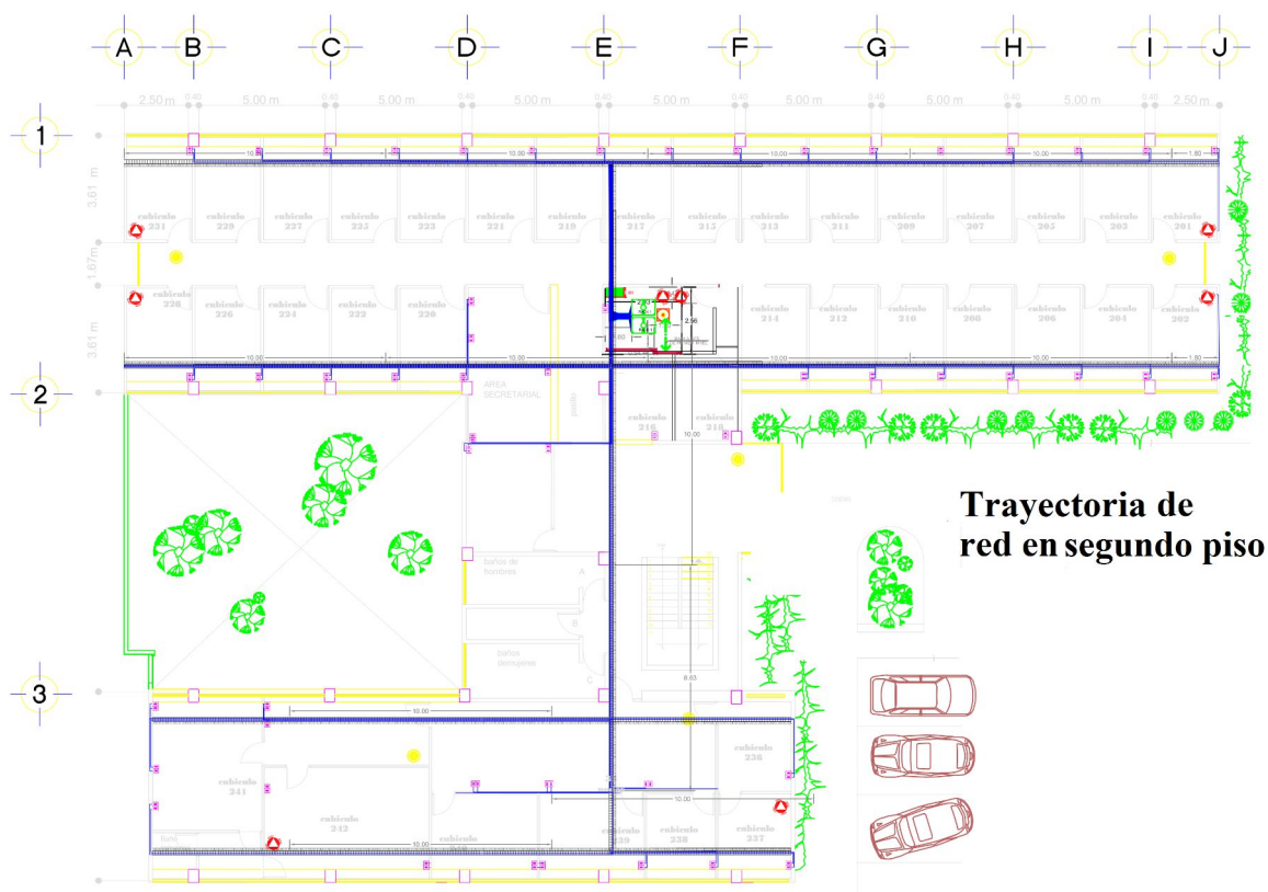
Figura 3.11: Trayectoria de red en segundo piso
