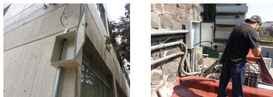
Figura 3.21: Canalización con tubería conduit y paneles liu
