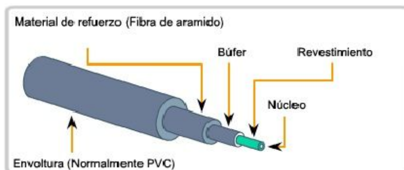
Figura 1.34: Fibra Óptica
