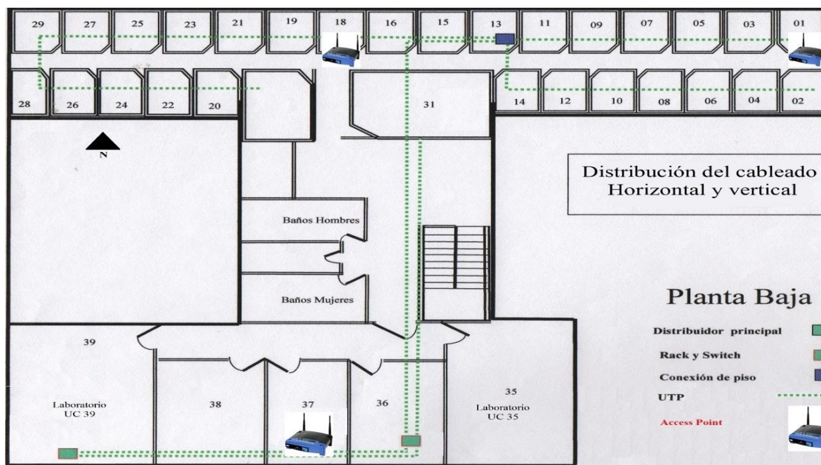
Figura 2.40: Distribución de puntos de acceso inalámbricos
