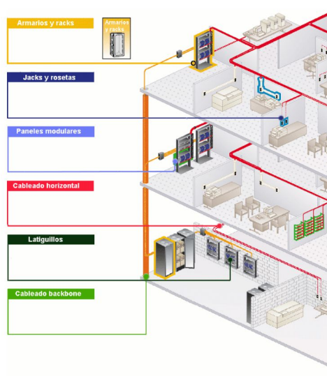
Figura 1.79: Identificación por código de colores
