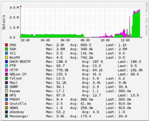
Figura 4.6: Gráfica de vista histórica de los tipos de tráficos (protocolos).
