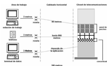
Figura 1.84: Cableado Horizontal
