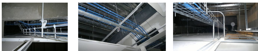
Figura 3.4: Canalizaciones horizontales en segundo piso
