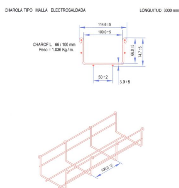
Figura 3.7: Charola tipo malla de 100 mm de ancho.
