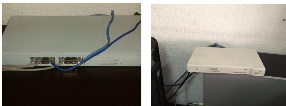
Figura 2.22: Switch improvisados.
