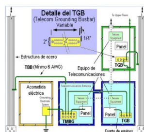
Figura 1.83: Diagrama del Sistema de Puesta a Tierra.
