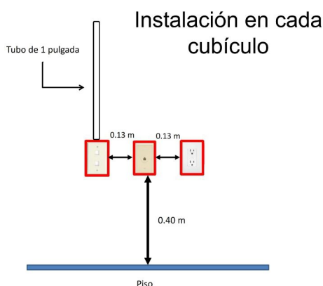
Figura 3.16: Especificaciones de rosetas de red y telefónica
