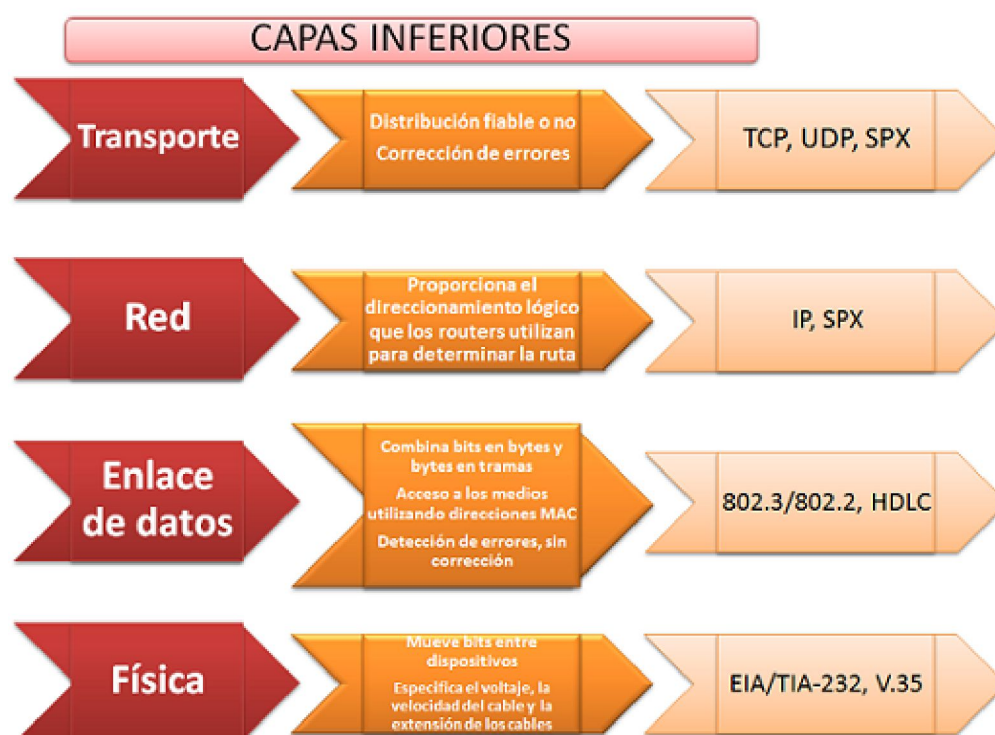
Figura 1.22: Capas Inferiores del modelo OSI
