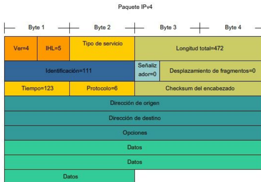
Figura 1.28: Paquete IPv4
