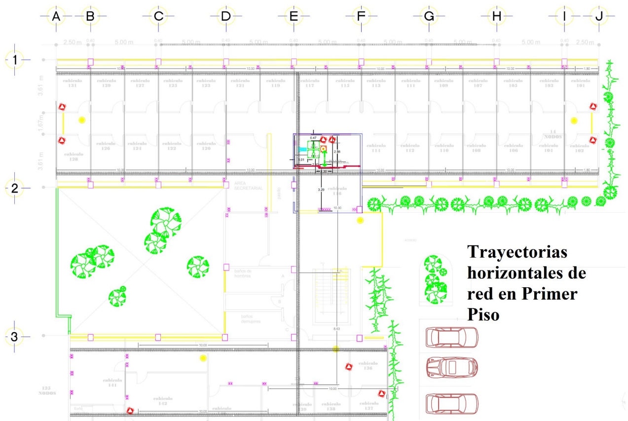
Figura 3.10: Trayectoria de red en primer piso
