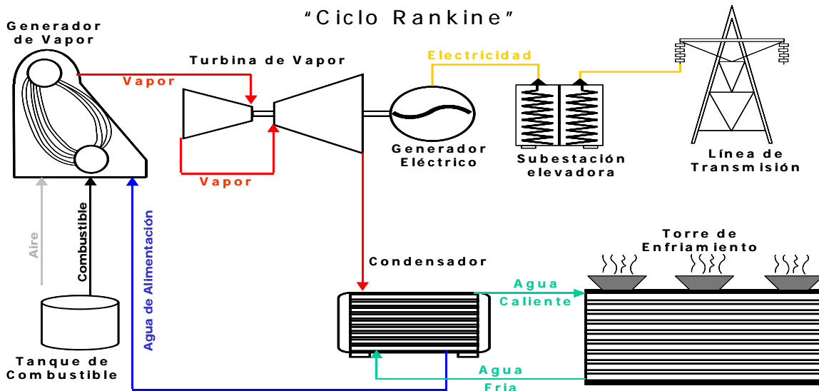
Figura 3. Diagrama de una Central Termoeléctrica Convencional
