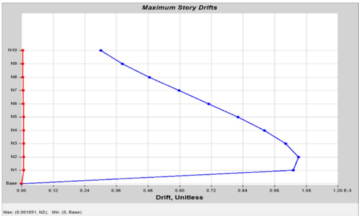
Figura 3.11 Distorsiones, edificio aislado
