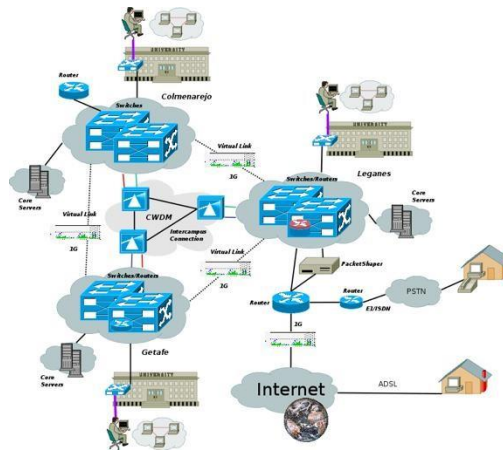
Figura 8 Red de Área Local por campus o complejo, CAN.
