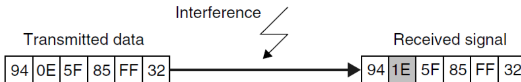
Fig. 3.22 La interferencia durante la transmisión causa errores. [8]
