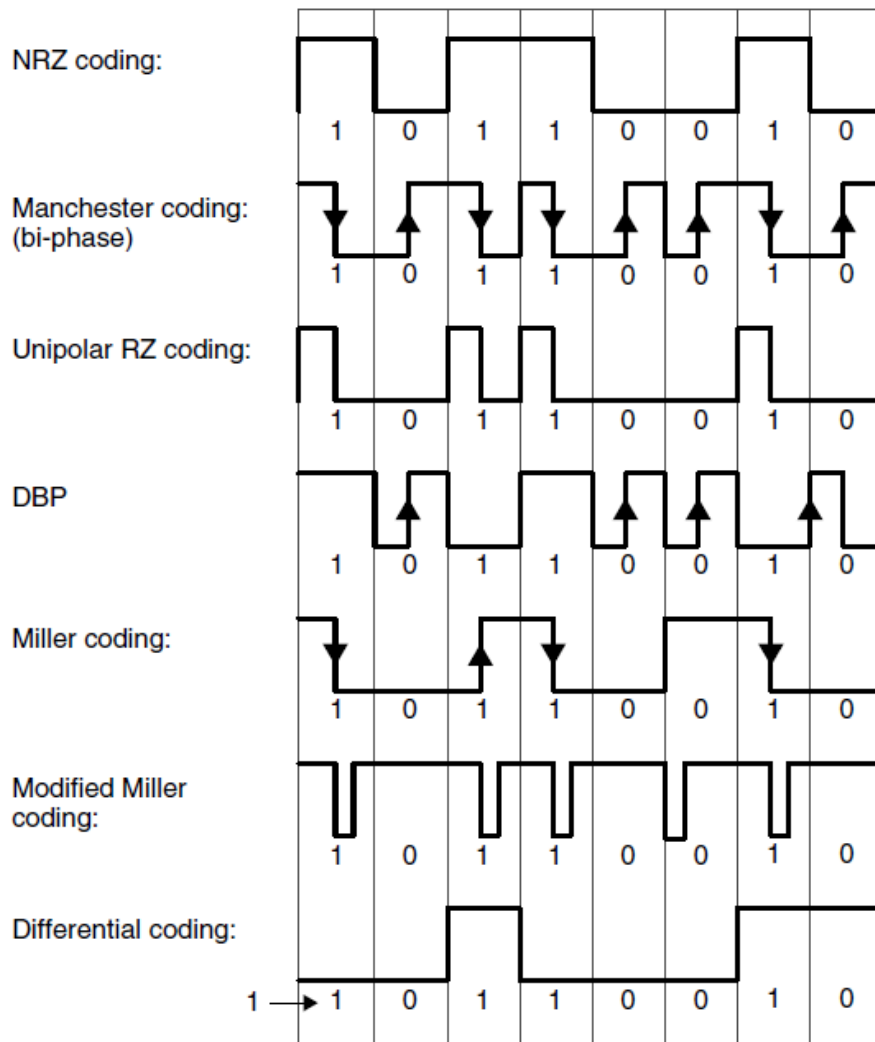
Fig. 3.18 Códigos utilizados en los sistemas RFID. [8]
