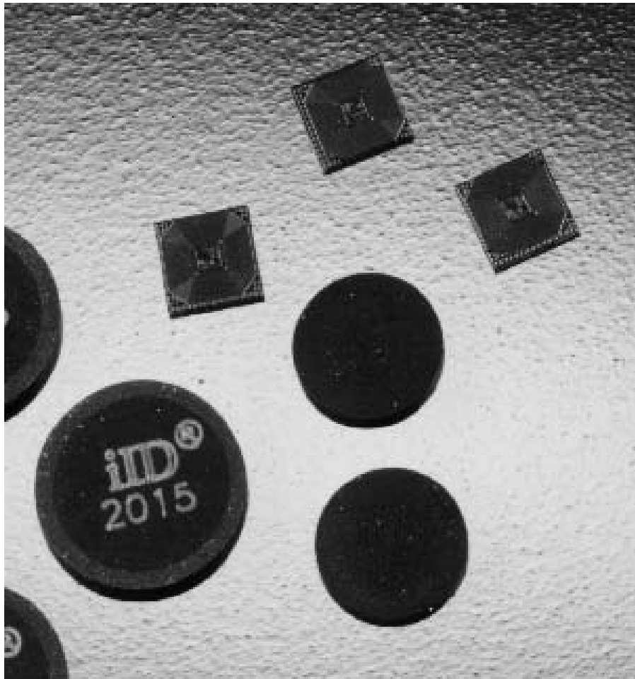
Fig. 3.12 Tag miniatura bobina en chip ( coil-on-chip ). [Propiedad de Micro Sensys, Erfurt] [8]
