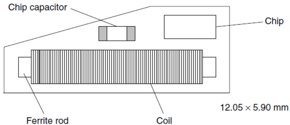
Fig. 3.6 Diseño mecánico de una cápsula de plástico. [8]
