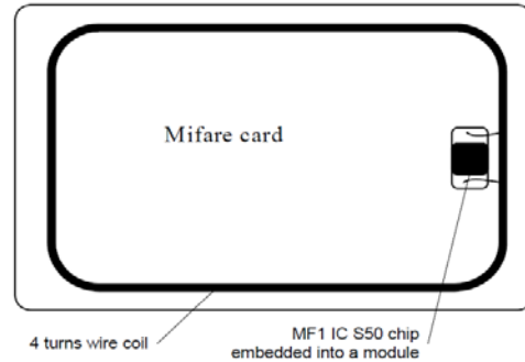
Fig. 3.33 Elementos dentro de una tarjeta MiFare
