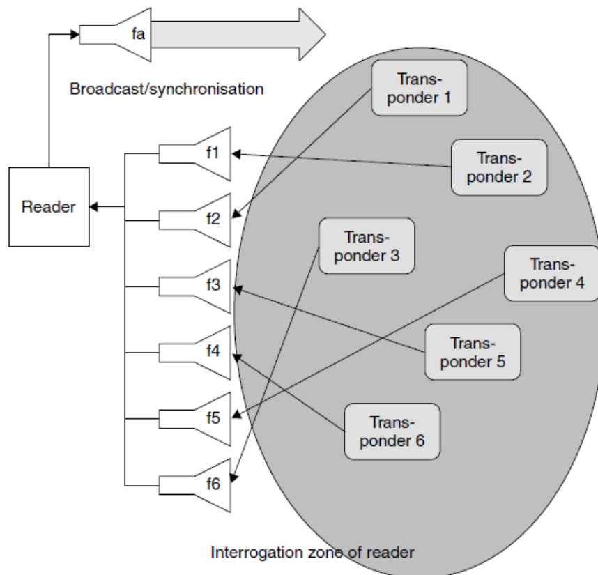
Fig. 3.30 En FDMA varios canales de frecuencia están disponibles para la transferencia de datos [8]
