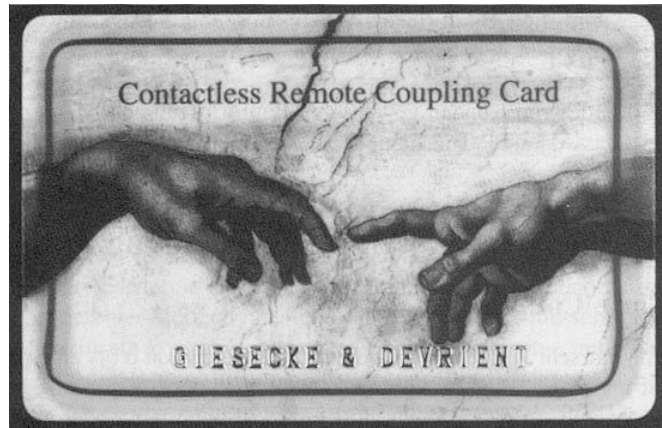
Fig. 3.10 Smart Card semitransparente. La antena puede verse claramente alrededor del borde de la tarjeta. [Propiedad de Giesecke & Devrient, Munich] [8]
