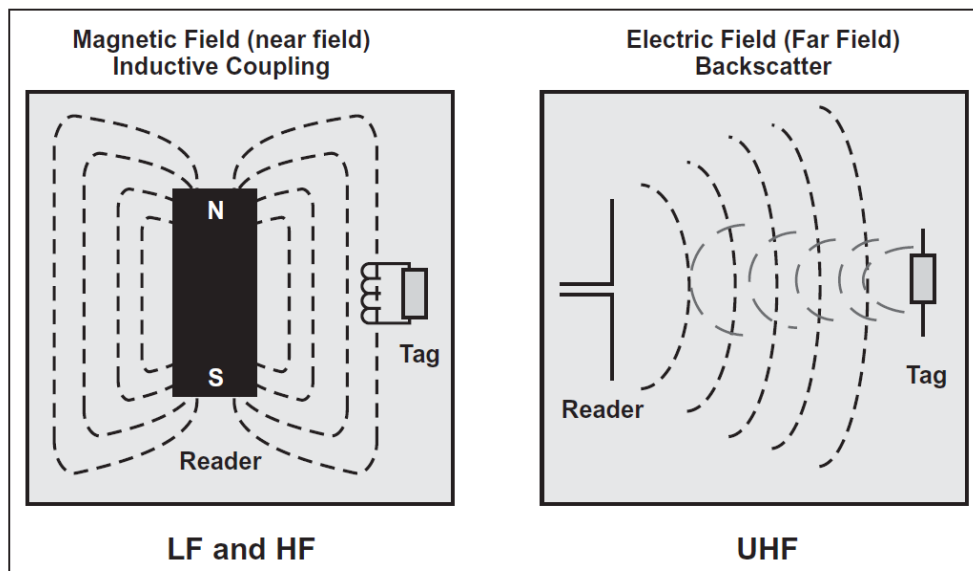
Fig. 3.16 Dos tipos diferentes de acoplamientos de Antenas/Tags. [7]
