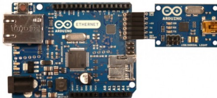
Fig. 4.14 Conexión del Arduino Ethernet Board y el USB Serial
