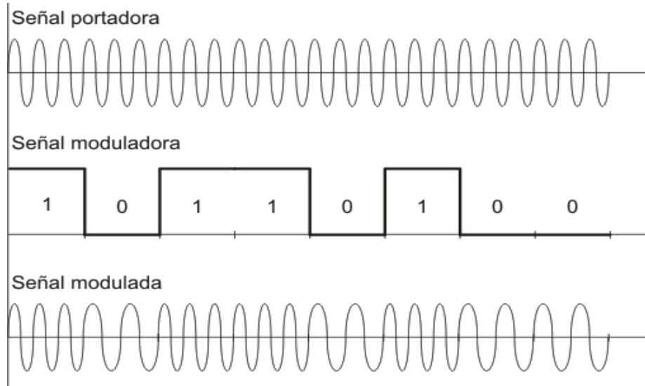
Fig. 3.20 Ejemplo de Modulación FSK [F]
