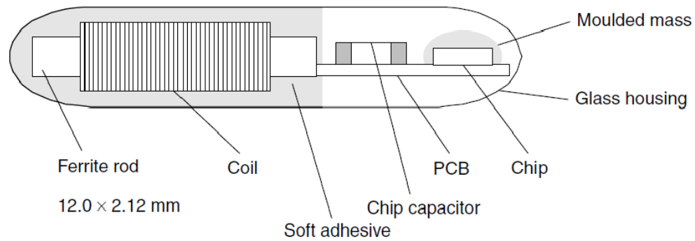
Fig. 3.4 Diseño mecánico de un Tag de vidrio [8]
