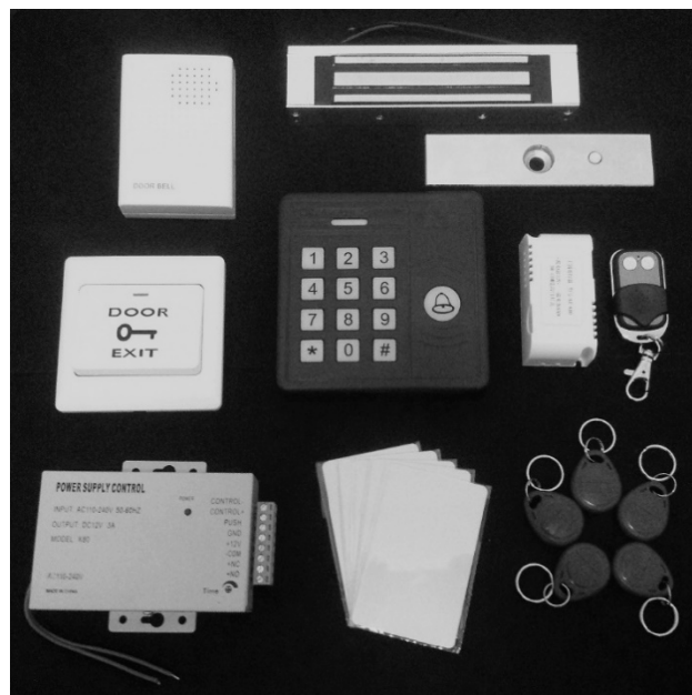
Fig. 3.15 Sistema de Acceso RFID [Propiedad de OEM] [8]
