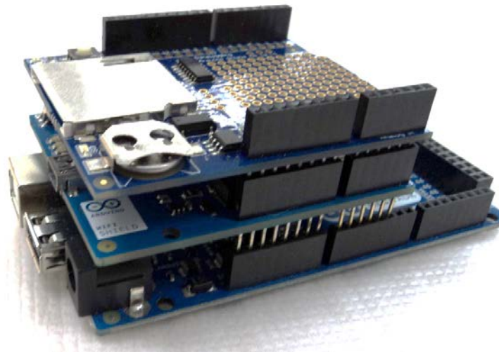
Fig. 4.10 Arduino Mega ADK + Arduino Wi-Fi Shield + Data Logger
