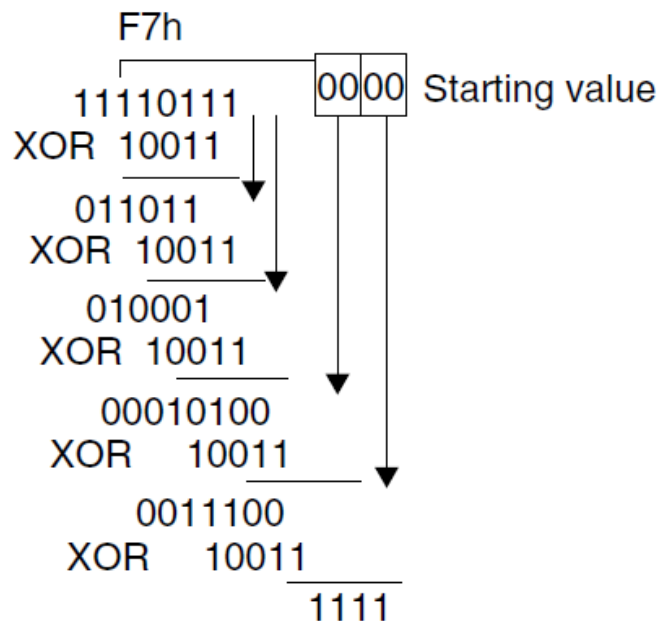
Fig. 3.25 Cálculo de la verificación CRC paso a paso. [8]
