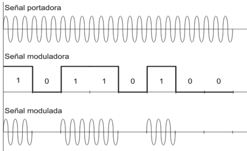
Fig. 3.19 Ejemplo de Modulación ASK [F]
