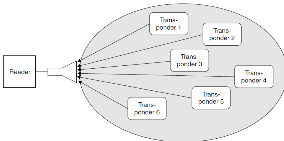
Fig. 3.28 Modo de transmisión tipo Multi-Access. [8]
