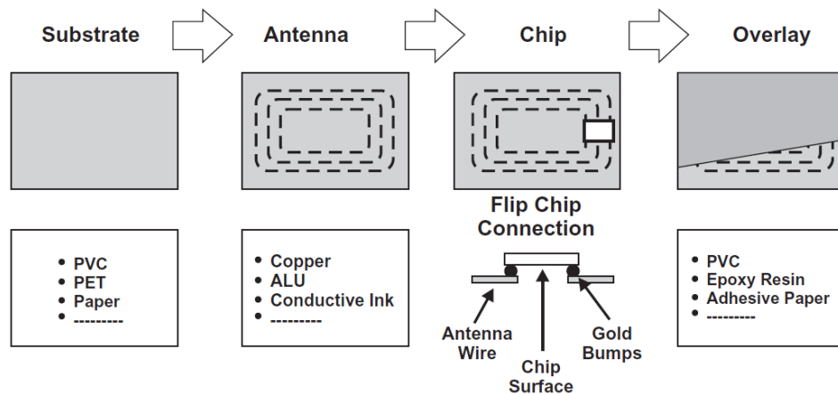
Fig. 3.2 Componentes de un Tag RFID [7]
