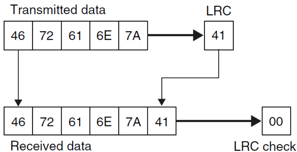
Fig. 3.24 Ejemplo de la verificación por medio del Procedimiento LRC. La suma será cero. [8]
