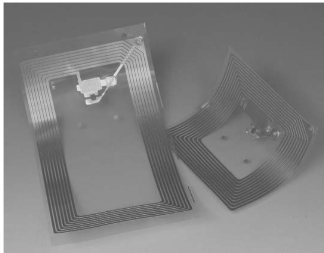
Fig. 3.11 Tag Smart Label (Etiqueta Inteligente). [Propiedad de Texas Instruments, Friesing] [8]
