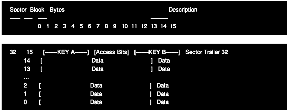
Fig. 3.35 Ejemplo de un sector de 16 Bloques
