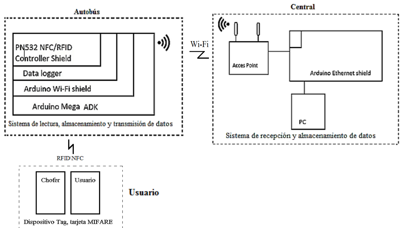
Fig. 4.1 Esquema de solución
