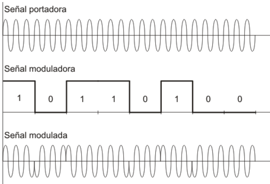
Fig. 3.21 Ejemplo de Modulación PSK [F]
