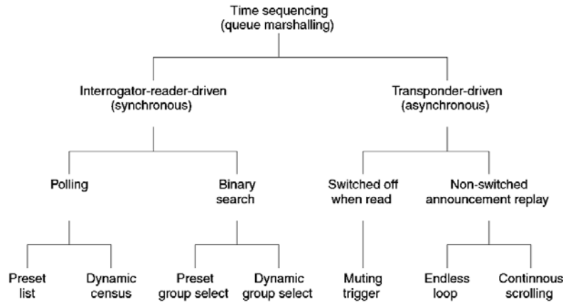
Fig 3.31 Clasificación de TDMA de acuerdo a Hawkes (1997) [8]
