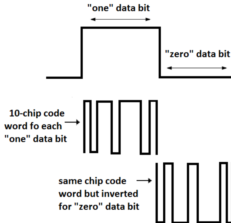
Fig. 2.5 Funcionamiento de DSSS [5]
