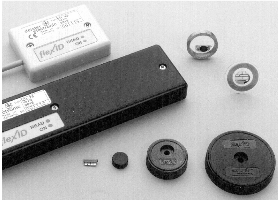
Fig. 3.3 Diferentes tipos de Tags Coin/Disk (moneda o disco). [Propiedad de Deister Electronic, Barsinghausen] [8]
