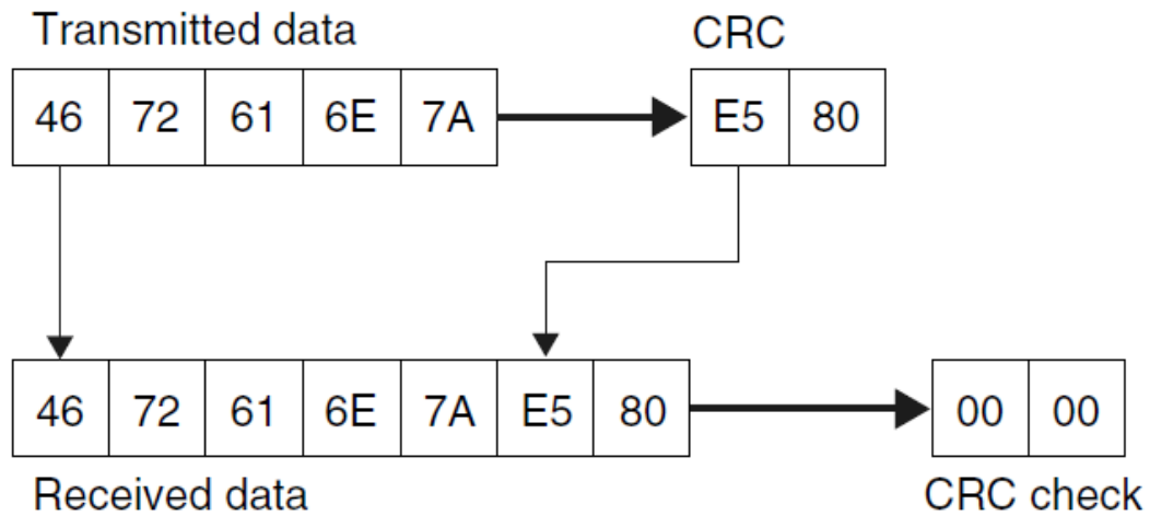
Fig. 3.26 Cálculo del CRC y la suma de comprobación. [8]
