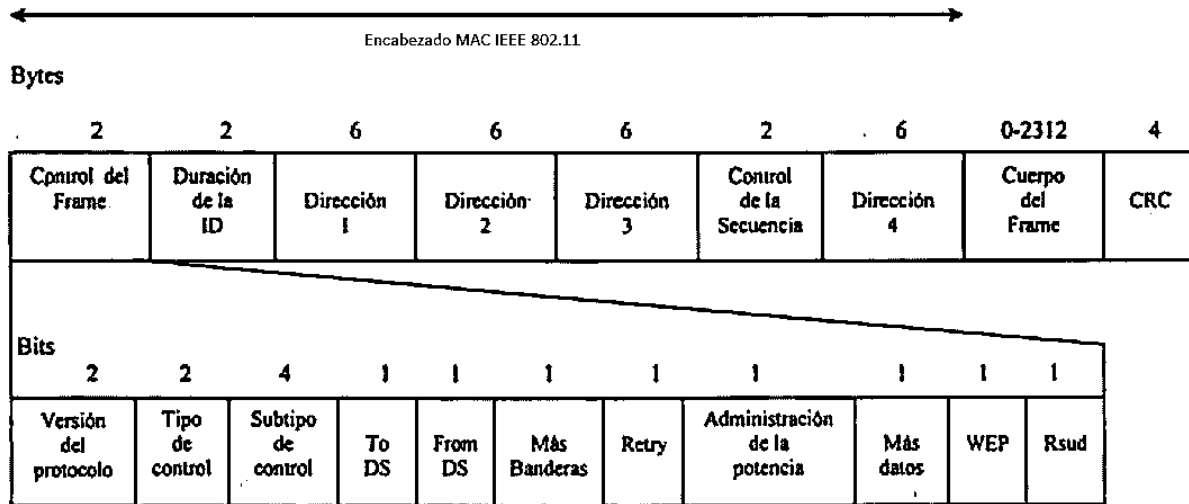
Fig. 2.6 Trama MAC IEEE 802.11 [5]
