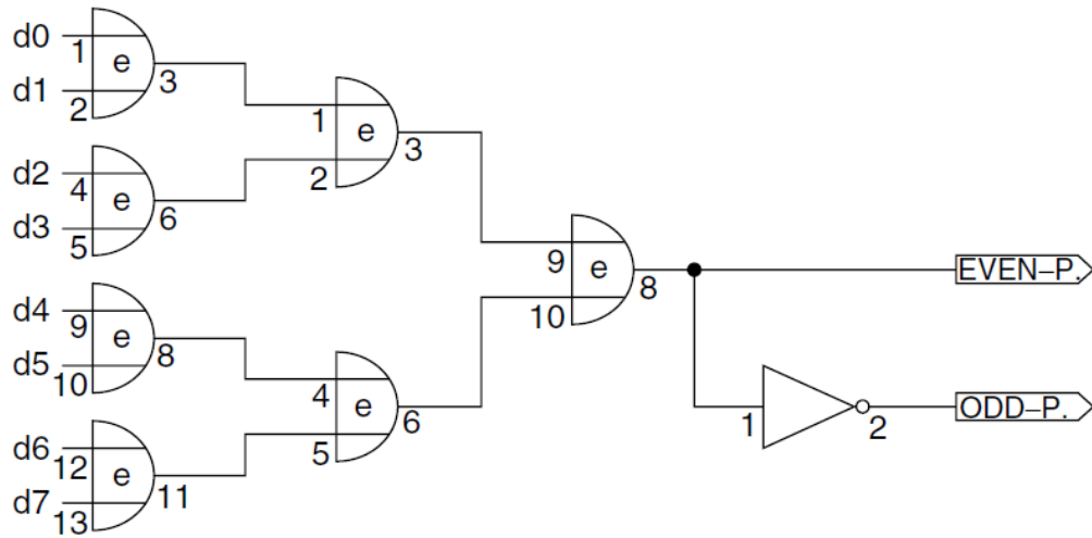
Fig. 3.23 El Bit de Paridad puede ser determinado bajo una serie de Compuertas Lógicas OR. [8]
