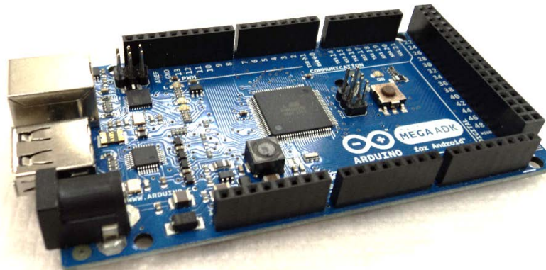
Fig. 4.8 Arduino Mega ADK
