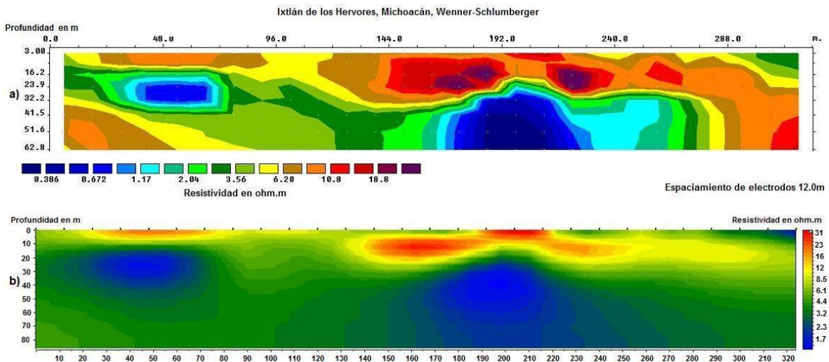
Figura 5.11. Modelos de inversión de uno de los perfiles realizados en Ixtlán de los Hervores, Michoacán. (a) Modelo de Inversión realizado con el programa RES2DINV. (b) Modelo de Inversión realizado con el programa ZONDRES2D.
