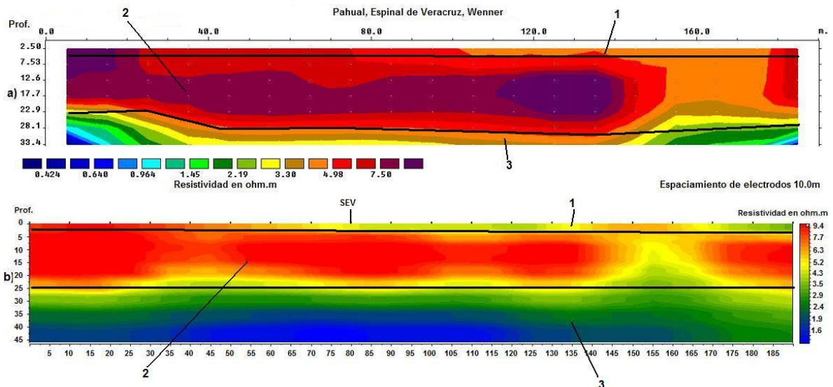
Figura 5.14. Modelos de inversión del perfil realizado en Pahuatl. (a) Modelo de Inversión realizado con el programa RES2DINV. (b) Modelo de Inversión realizado con el programa ZONDRES2D.
