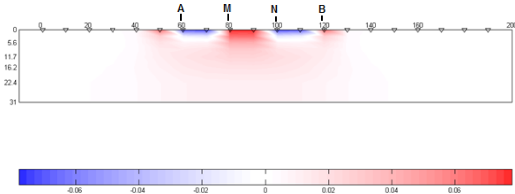
Figura 4.1. Gráfica de la función de sensibilidad de la modalidad Wenner
