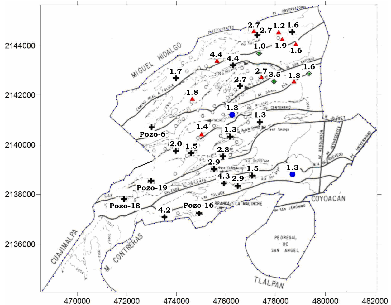
Figura 5.5 Mapa de frecuencias fundamentales (adaptado de Hubp-Lugo et al 1995), cada punto muestra el valor de la frecuencia fundamental en los terrenos de la DAO, los puntos que carecen de valor solo se han señalado con su nombre.
