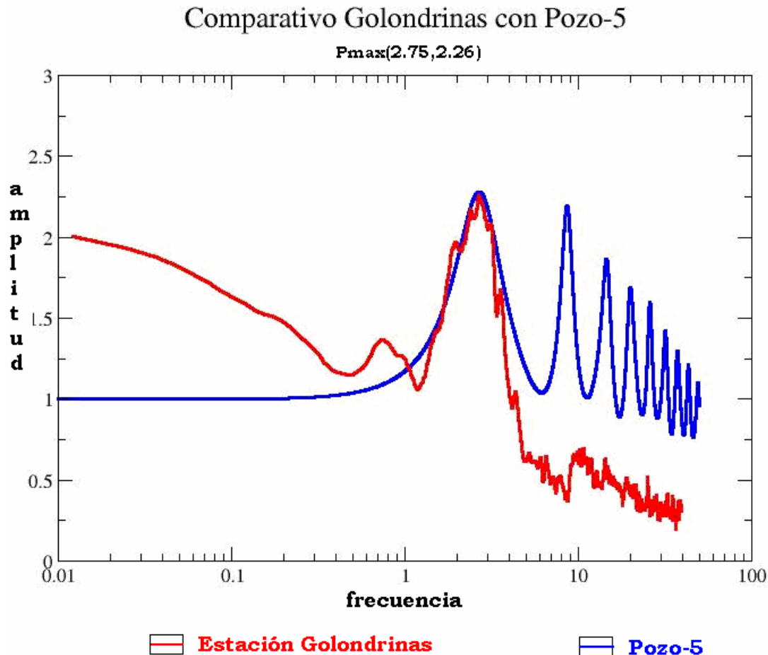
Figura 5.3 Ajuste de modelos, entre el medido (estación Golondrinas) y el pozo 5 que es el más cercano a esta)
