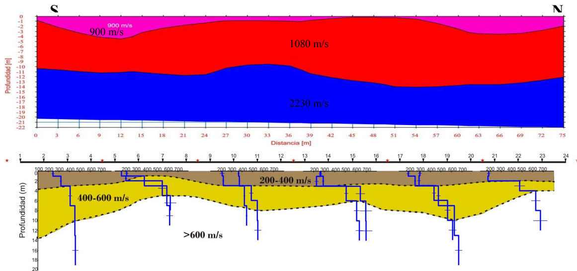
Figura 5.2 El modelo de velocidades de ondas P y S se obtuvo del estudio de refracción realizado por Cardenas et al. ; 2009. La velocidad de la onda S fué obtenida a partir de ondas superficiales generadas durante la toma de datos. El eje horizontal corresponde a la distancia a lo largo del perfil en el modelo de la onda P, y el eje vertical es la profundidad dada en metros.
