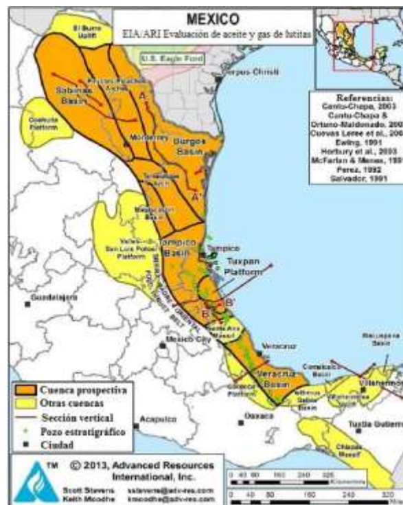
Figura 3. Ubicación de las cuencas con recursos de aceite y gas en lutitas, fuente EIA 2015.
