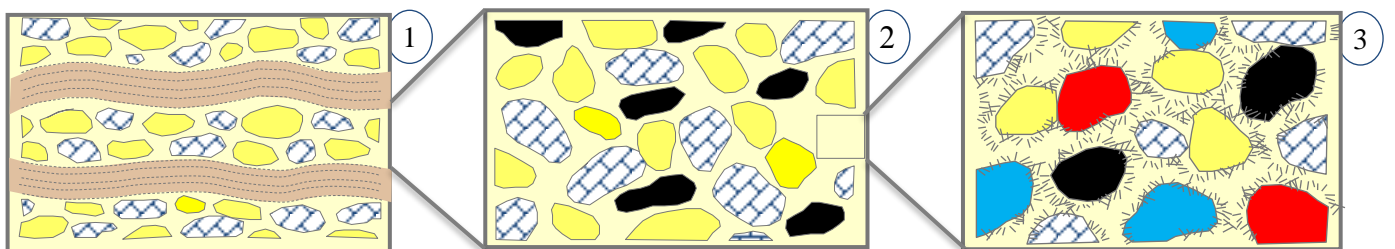
Figura 11. Segundo modelo de clásticos utilizado para inversión.
