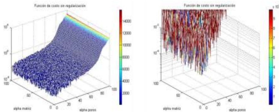
Figura 28. Representación de la función de costo sin regularización.
