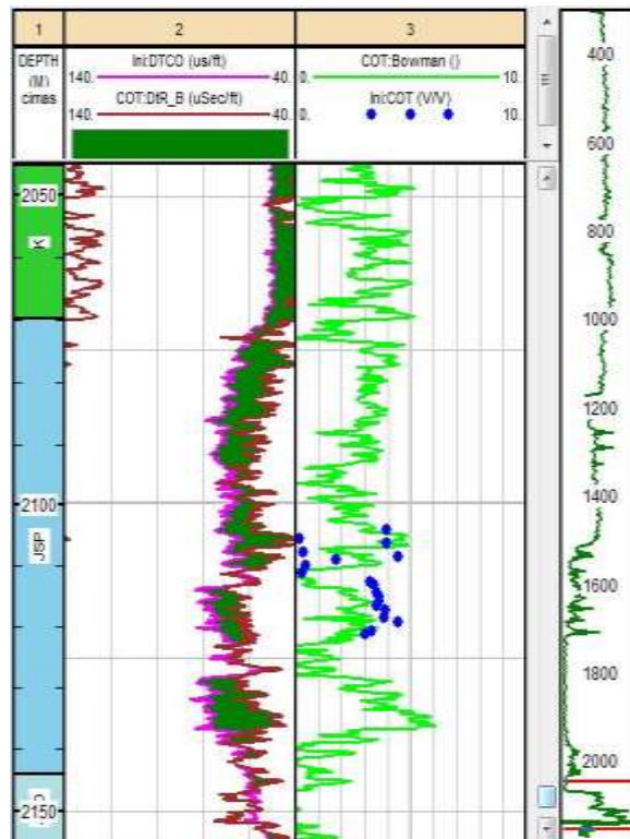
Figura 25. Aplicación de la metodología de Bowman en la estimación de COT, carril 1-zonificación, carril 2-cálculo de \Delta \log R con las curvas DTCO y \Delta tR , carril 3- COT calculado con el método de Bowman. (línea continua) y en color azul los datos puntuales de COT medidos con núcleos, último carril-registro de rayos gamma total en la columna completa del pozo.
