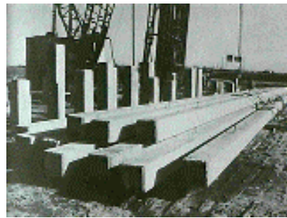
Pilotes prefabricados
