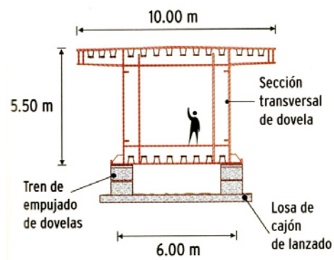
Corte transversal superestructura
