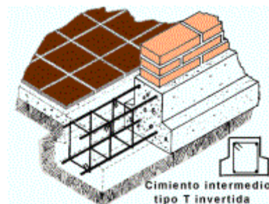
i.2) Zapata Corrida de Concreto Reforzado
