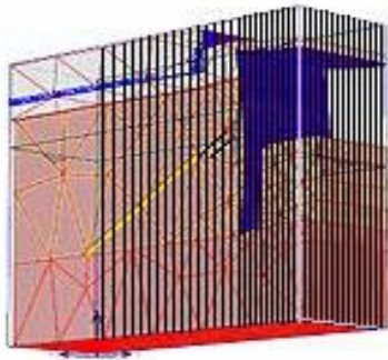
Fig. 9. Suelo con pilotes de 1mm.
