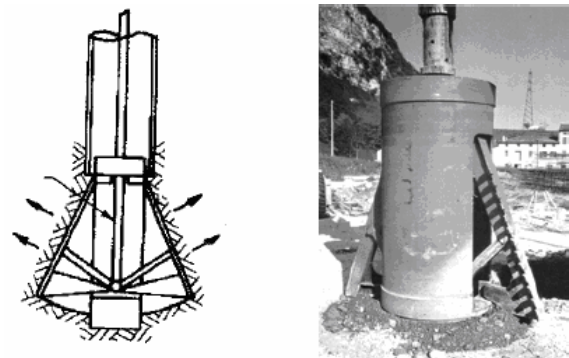
Fig. 1. Bote campana
