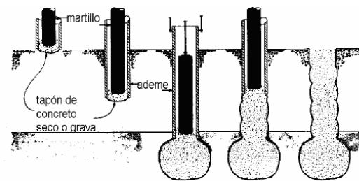
inicio de la instalación hincado de ademe hasta estrato resistente base formada en el estrato resistente formación de fuste de pila pila terminada
