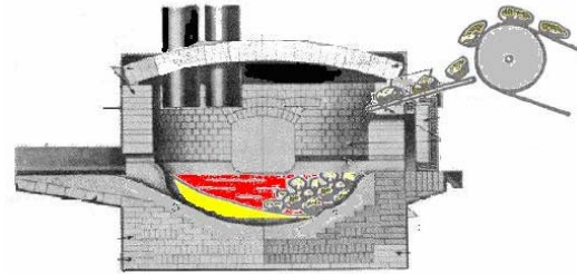
Dibujo del corte de un horno
