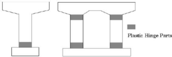
Fig. 3.2.8. Ubicación de la articulación plástica
