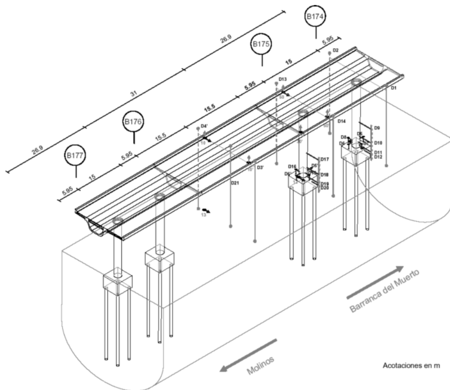
Fig. 4.1.16. Distribución de los acelerómetros y de los transductores de desplazamiento para las pruebas con cargas vehiculares de Barranca del Muerto (IINGEN 2005)
