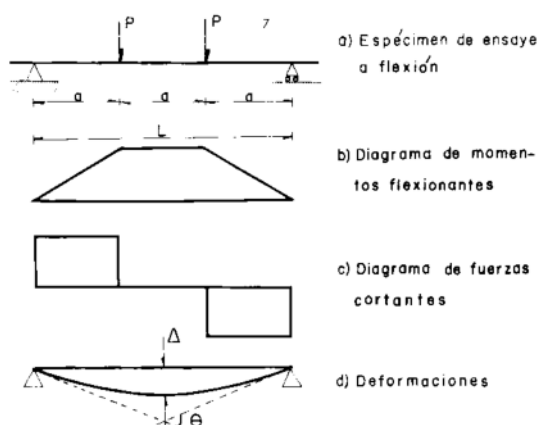
Fig. 3.1.1. Ensaye de flexión típico
