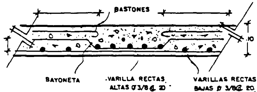
SECCION DE LOSA
