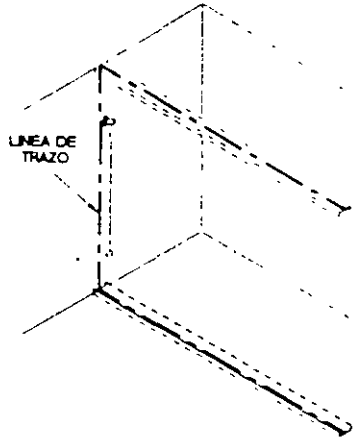
1.- Trazado del muro interior verificando su correcta alineacion a plomo.
