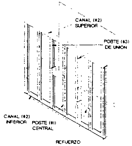
3.- Colocacion y fijacion a cada 61 cm de postes centrales y de union para los tableros PLYCEM, y colocacion de refuerzos para instalaciones, puertas y ventanas
