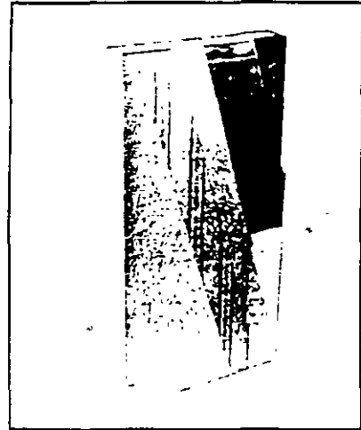
Muestra de muro divisorio ilustrando los componentes: perfiles galvanizados, paneles de vado y aislamiento termo-acústico, en su superficie lisa se logran magníficos acabados
