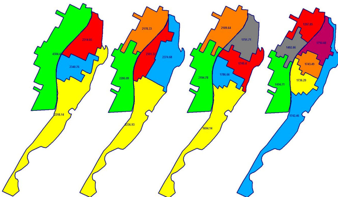
Figura 33 Partición regional para 4, 5, 6 y 7 distritos, respectivamente. Elaboración propia.
