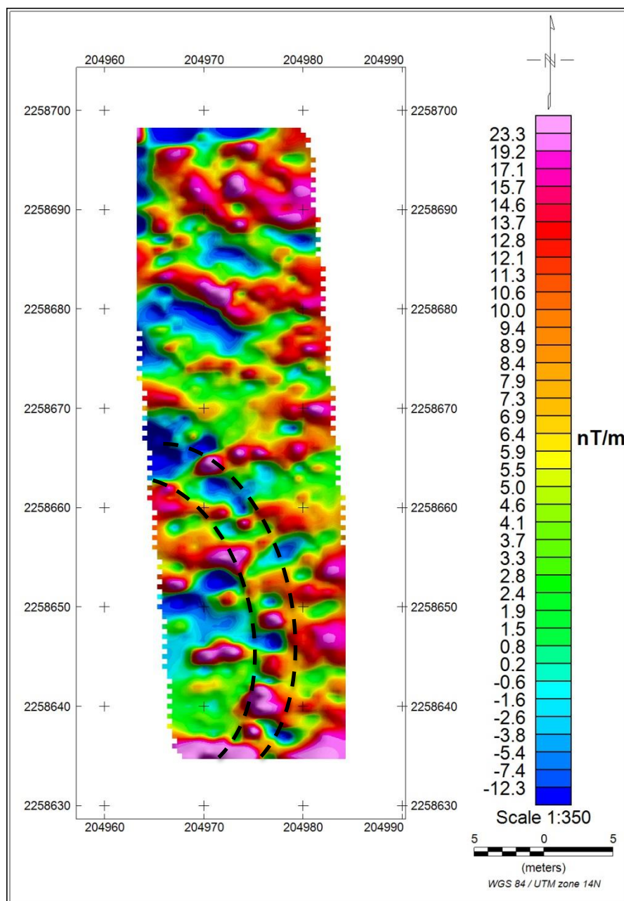
Figura 25. Gradiente vertical del JP
