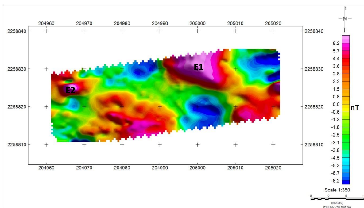
Figura 43. Campo residual del sensor superior para la T4.
