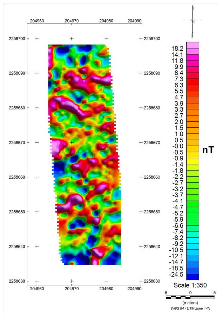
Figura 26. Resta de la reducción al polo del sensor inferior menos el sensor superior del JP
