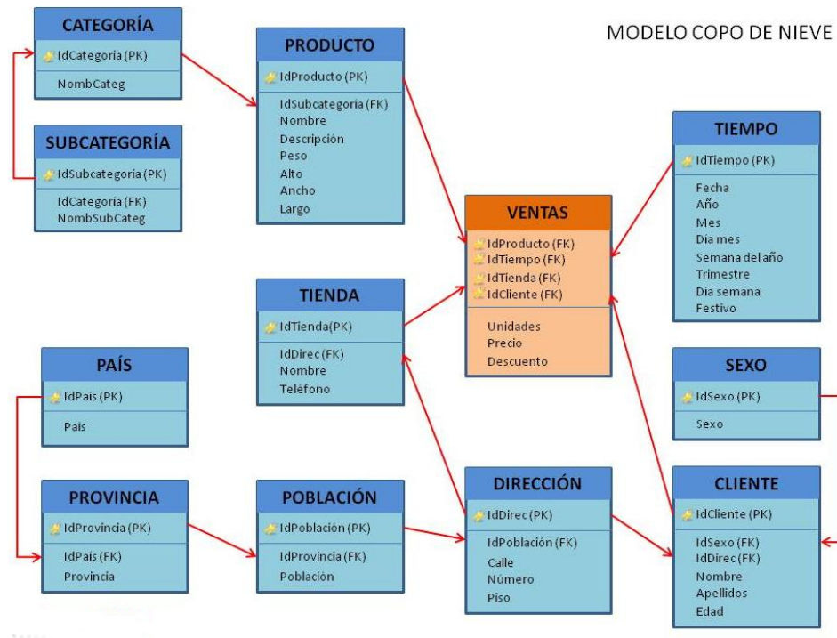
Figura 3.3. Ejemplo de un data mart con esquema de copo de nieve. Tomado de: García (2013)
