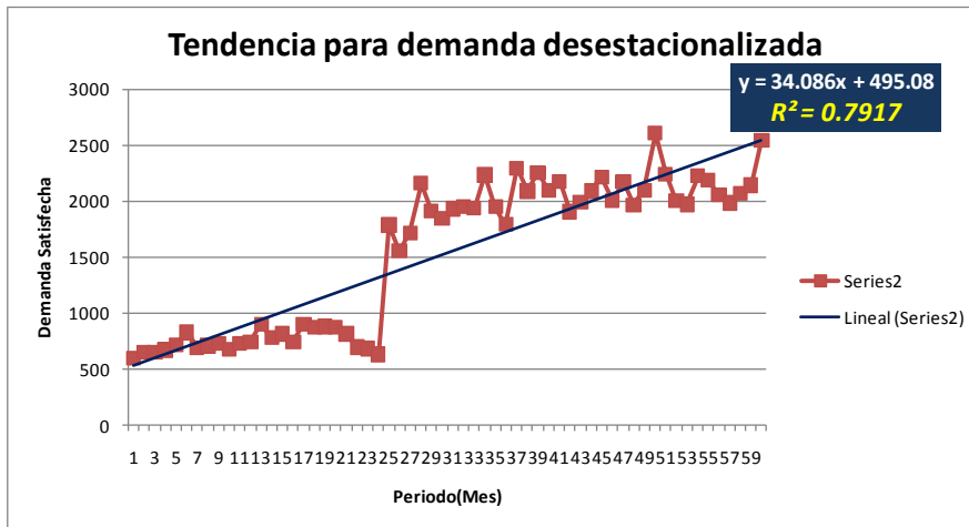
Gráfico 9 Modelo para la demanda satisfecha desestacionalizada
