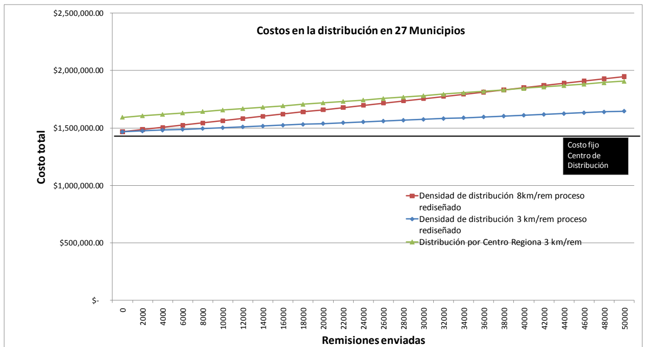
Gráfico 15 Costo de distribución de la demanda Total
