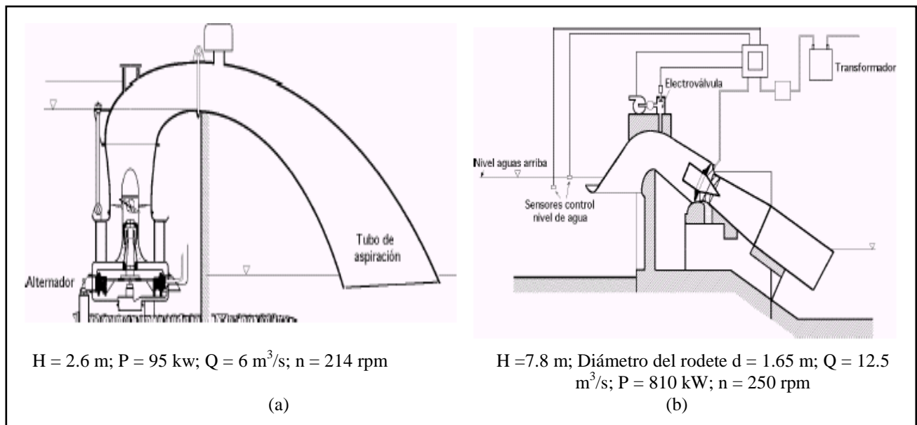
Figura 3.19: a) Sistema Bulbo con sifón-aspirador a la salida; b) Sistema de Bulbo con depósito de agua y sifón aguas arriba. [94]
