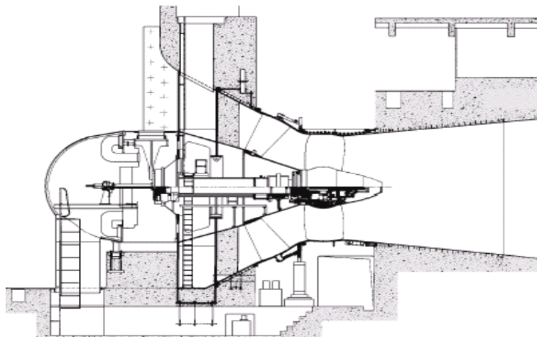
Figura 3.14: Turbina Bulbo y tubo de aspiración. [94]
