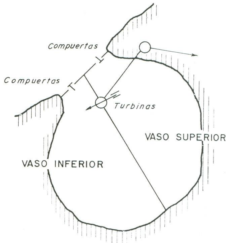
Figura 3.6: Disposición de obras mediante vasos conjugados. [28]
