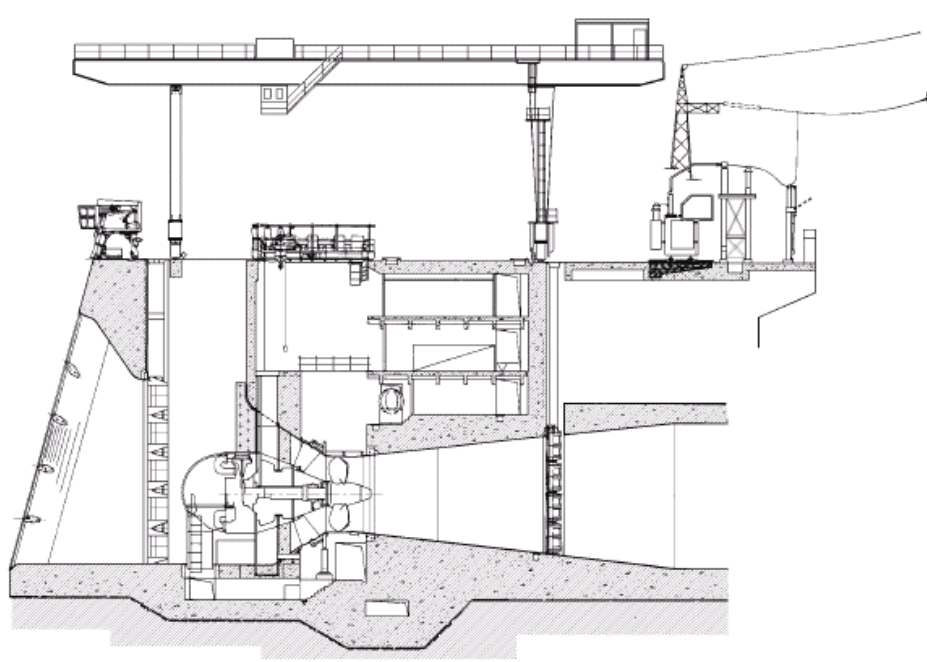
Figura 3.15: Turbina Bulbo instalada en el dique. [94]
