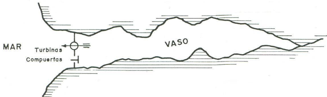
Figura 3.1: Disposición de obras mediante un solo vaso.[24]
