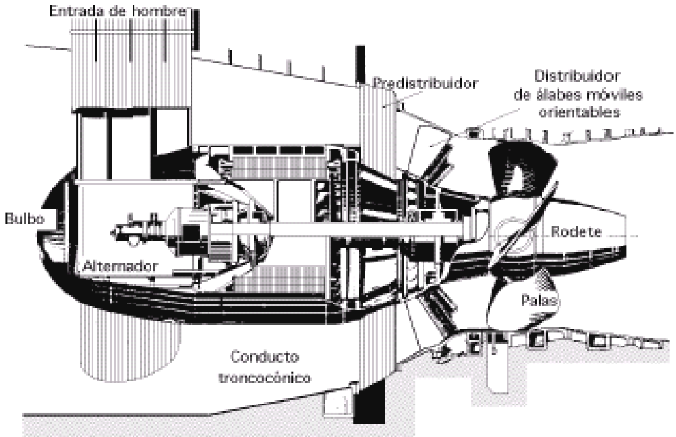
Figura 3.25: Grupo Bulbo de Beaumont-Monteux. [94]
