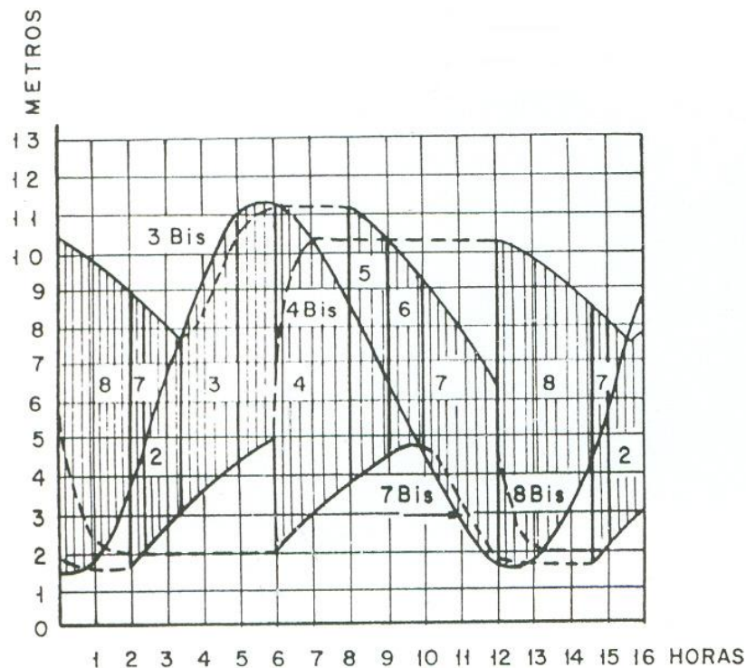
Figura 3.9: Funcionamiento y operación mediante vasos múltiples. [24]
