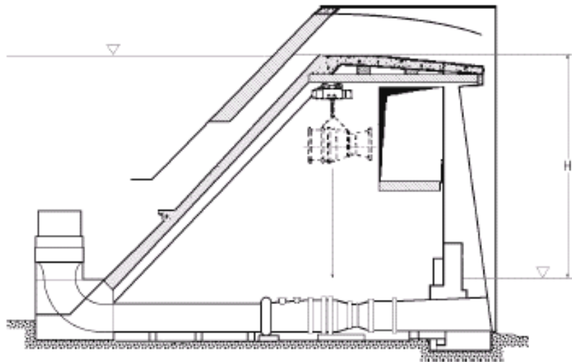
Figura 3.21: Sistema de Bulbo en conducción. [94]
