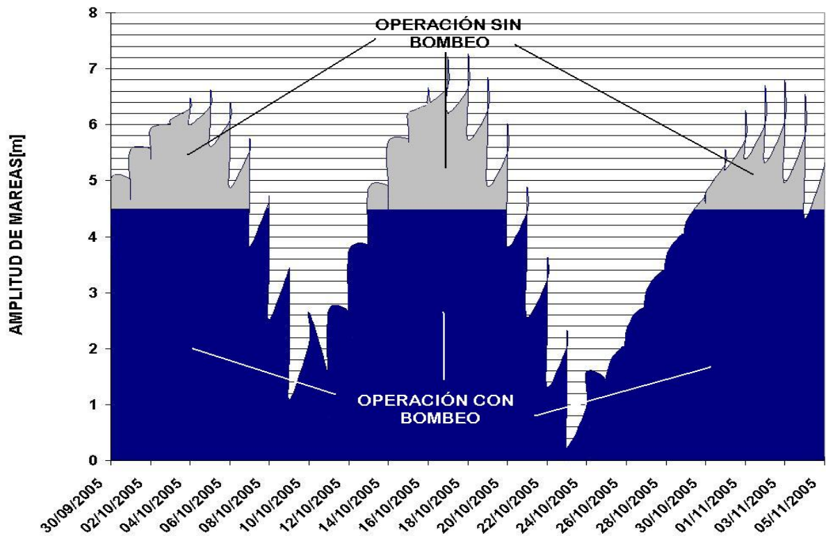
Figura 5.15: Operación de la planta considerando el comportamiento de las mareas en el Golfo de Santa Clara, Sonora.
