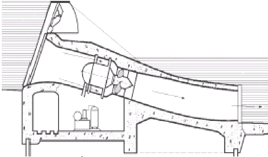
Figura 3.13: Grupo Bulbo de Röstin, 1936. [94]
