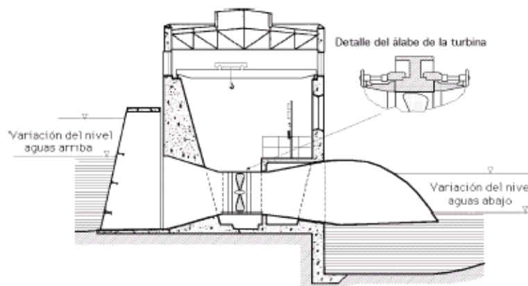
Figura 3.16: Grupo con alternador periférico (Harza). [94]
