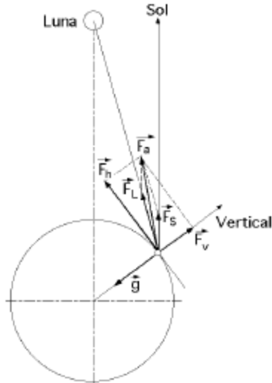
Figura 4.4: Fuerza generadora de la marea. [94]
