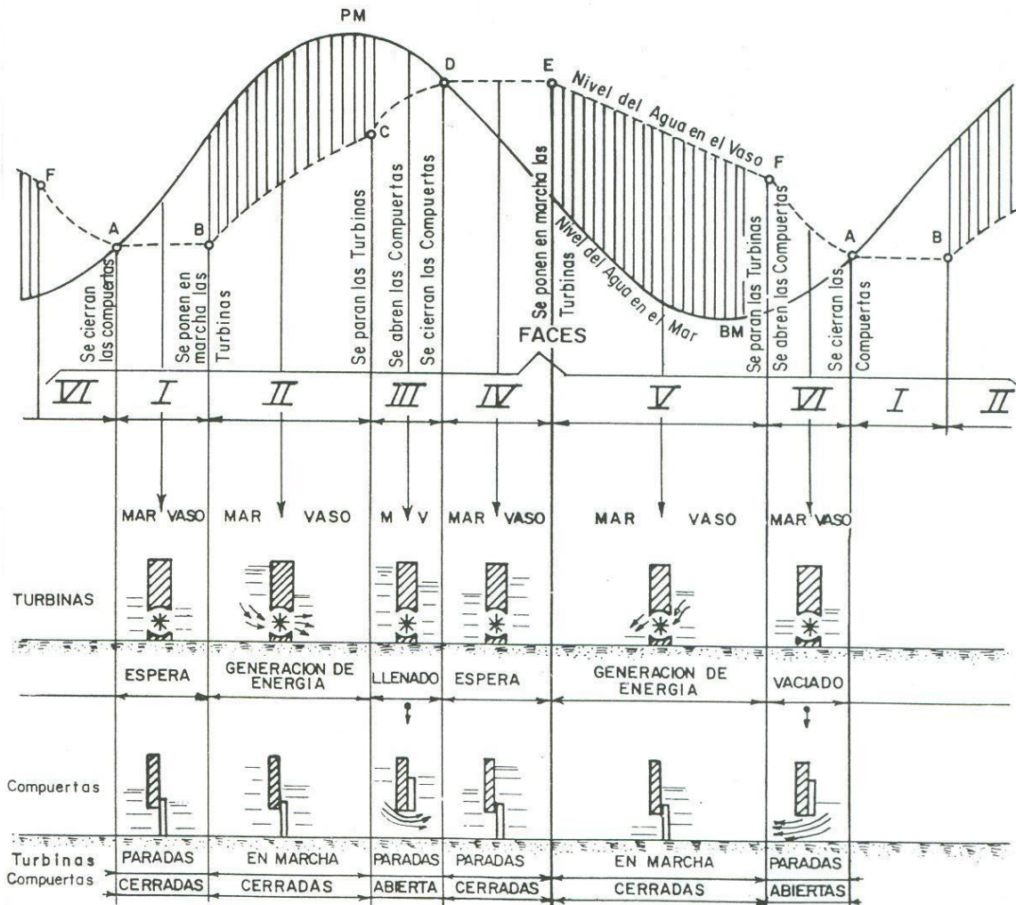
Figura 3.3: Funcionamiento y operación del ciclo al doble efecto. [24]
