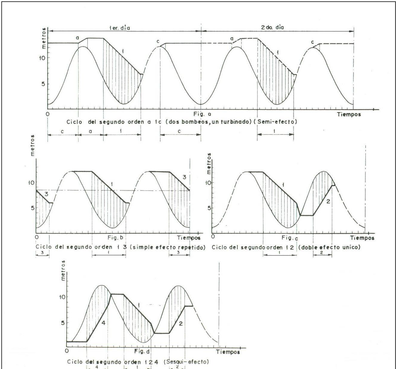
Figura 3.12: Ciclos de bombeo de segundo orden. [24]
