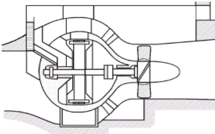
Diámetro del rodete = 8 m; diámetro del Bulbo = 12 m Figura 3.18: El primer proyecto de grupo Bulbo para el Rance, 1943. [94]
