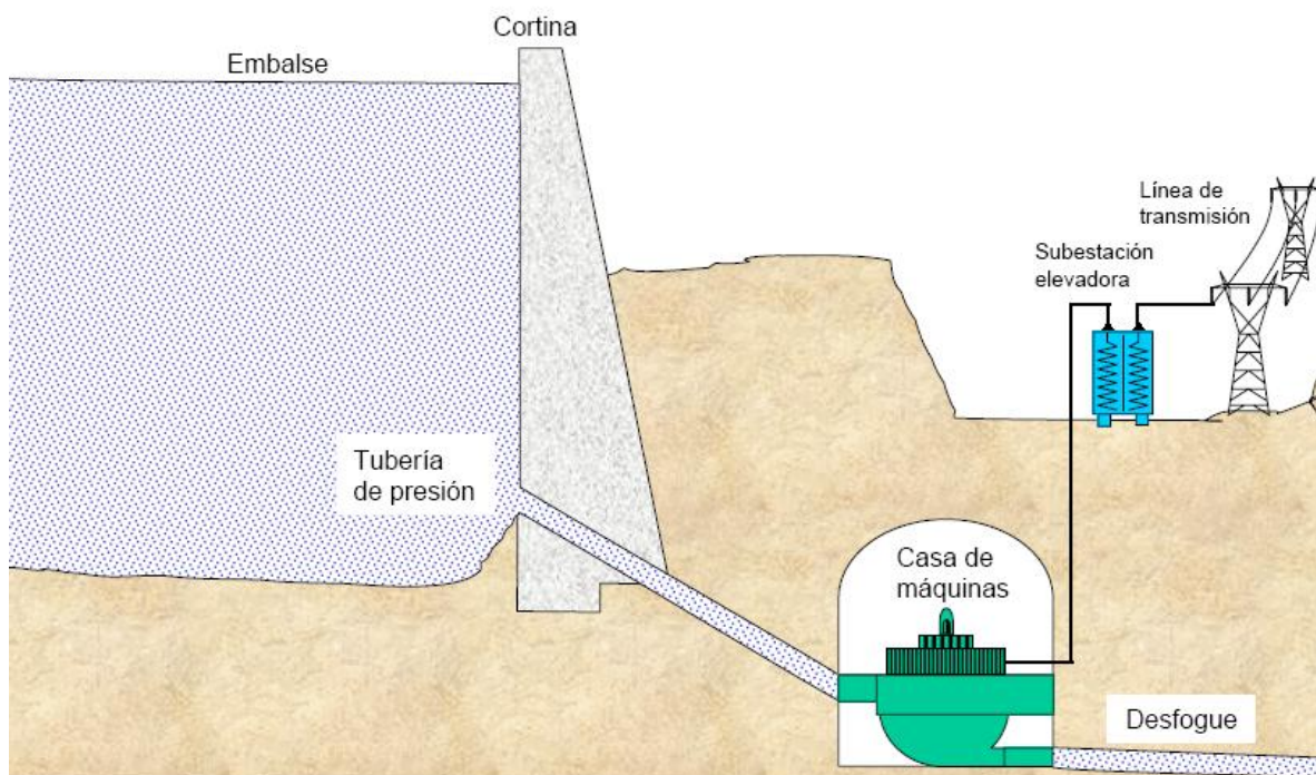
Figura 2.1: Central hidroeléctrica. [10]
