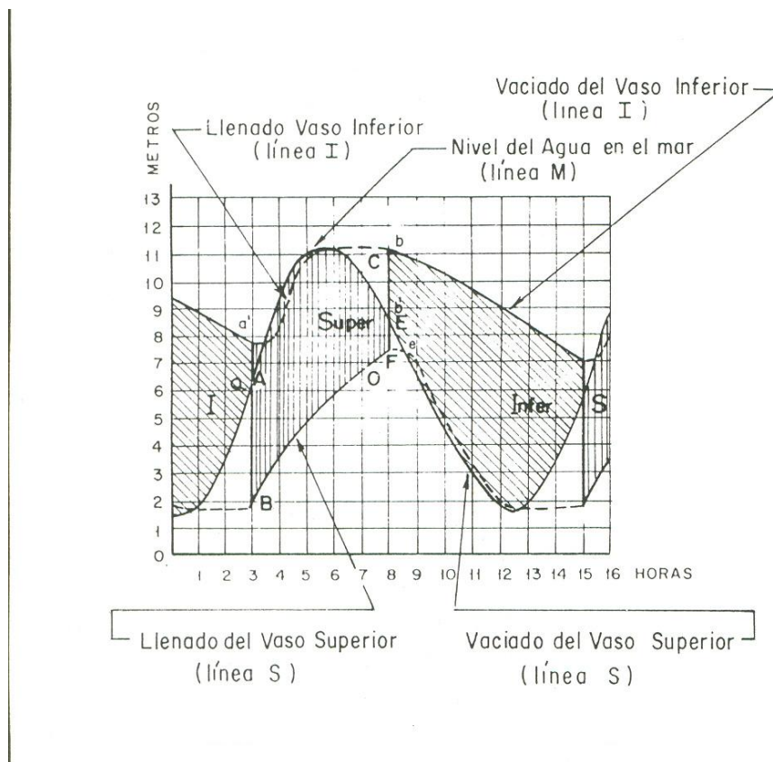
Figura 3.5: Funcionamiento y operación mediante vasos asociados. [24]
