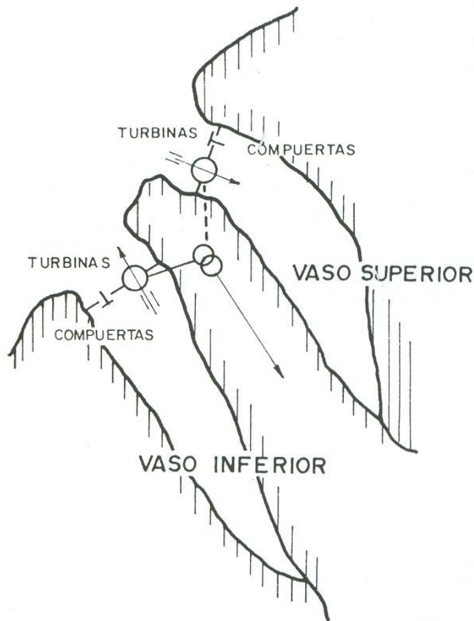
Figura 3.4: Disposición de obras mediante vasos asociados. [24]
