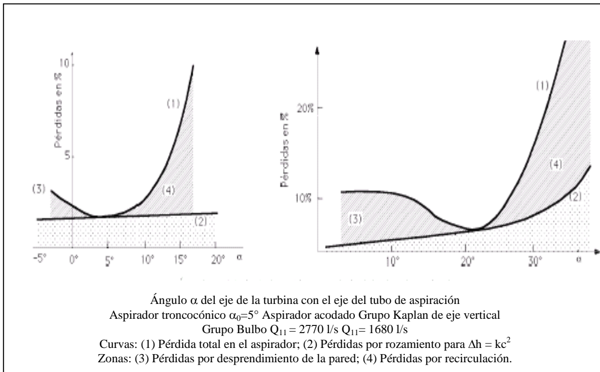
Figura 3.24: Pérdida de carga en algunos tipos de tubo de aspiración de turbinas Bulbo y Kaplan. [94]
