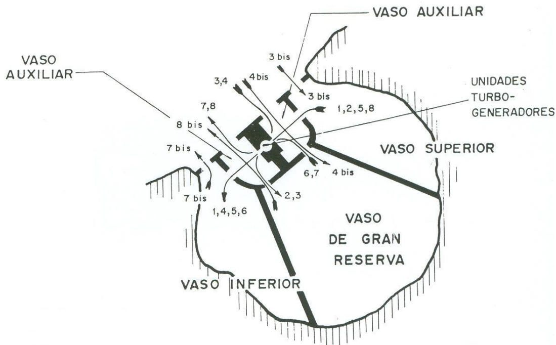
Figura 3.8: Disposición de obras mediante vasos múltiples. [28]
