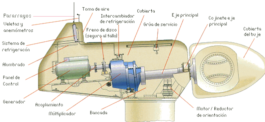
Figura 2.4: Partes constitutivas del chasis de un aerogenerador. [128]
