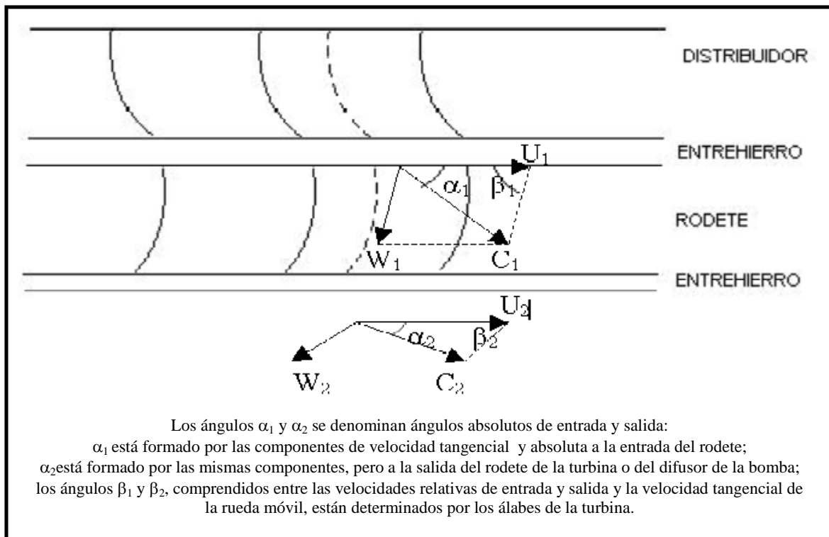
Figura 3.23: Diagrama de velocidad de una turbina axial. [53]
