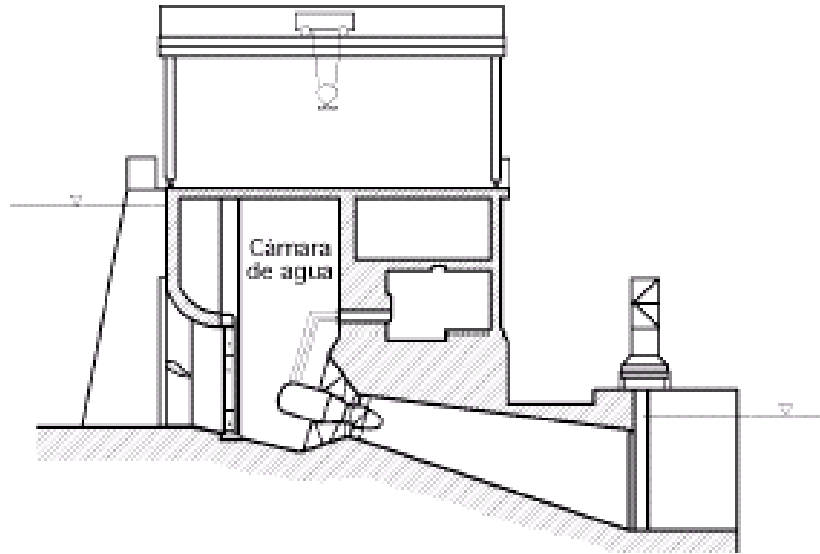
Q = 7.5 \text{ m}^3/\text{s} ; H = 15.5 \text{ m} ; P = 0.8 \text{ MW} ; n = 500 \text{ rpm} ; Diámetro del rodete d = 1.12 \text{ m} Figura 3.20: Sistema de grupo Bulbo instalado en cámara de agua (Castet), 1954. [94]
