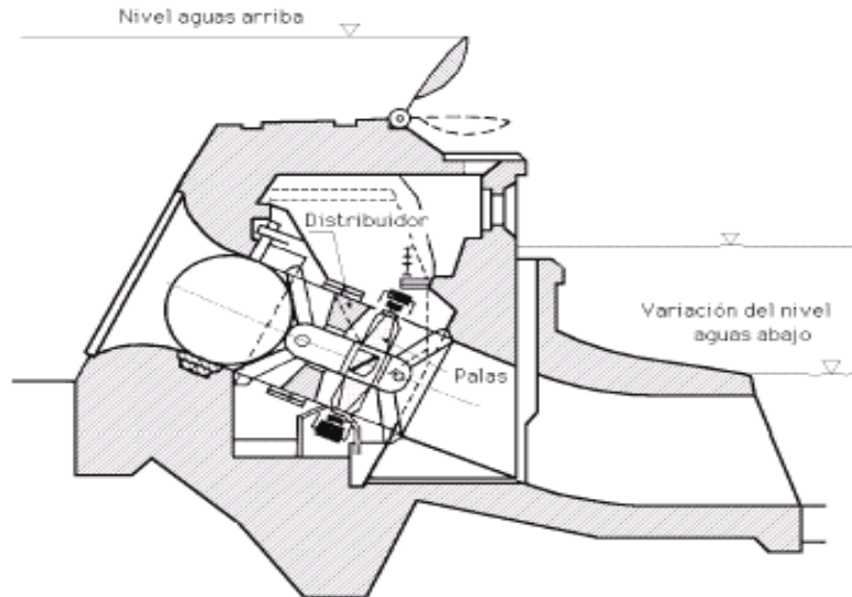
H = 9 \text{ m} ; Q = 25 \text{ m}^3/\text{s} ; P = 1.75 \text{ MW} ; n = 214 \text{ rpm} ; Diámetro del rodete d = 2.15 \text{ m} Figura 3.17: Grupo con alternador periférico de Steinbach (Baviera). [94]
