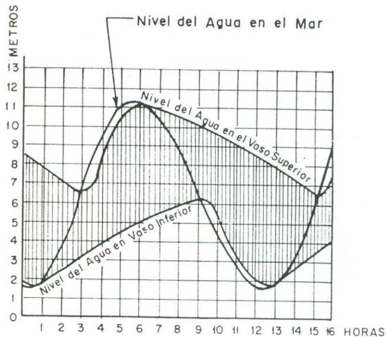
Figura 3.7: Funcionamiento y operación mediante vasos conjugados. [24]
