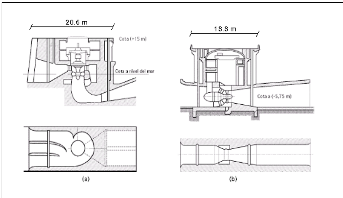
Figura 3.22: Conductos hidráulicos requeridos por una turbina Kaplan y un grupo Bulbo. [94]
