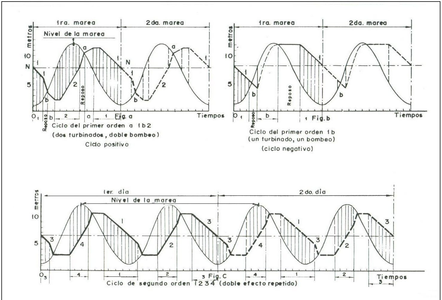
Figura 3.11: Ciclos de bombeo. [24]
