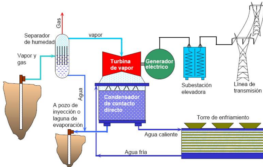
Figura 2.6: Central Geotermoeléctrica. [10]
