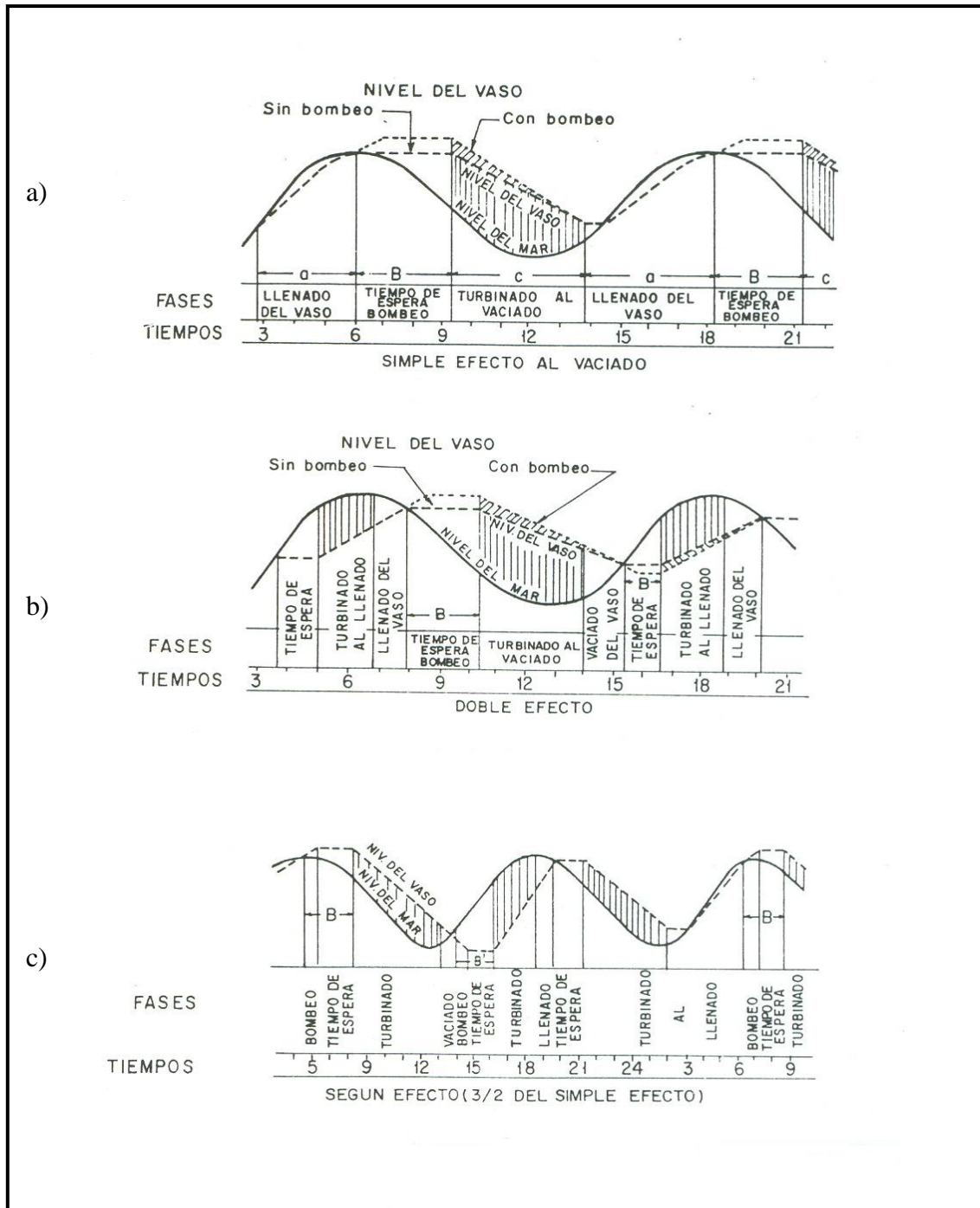
Figura 3.10: Operaciones con bombeo a) Simple efecto al vaciado, b) Doble efecto c) 3/2 del simple efecto. [24]
