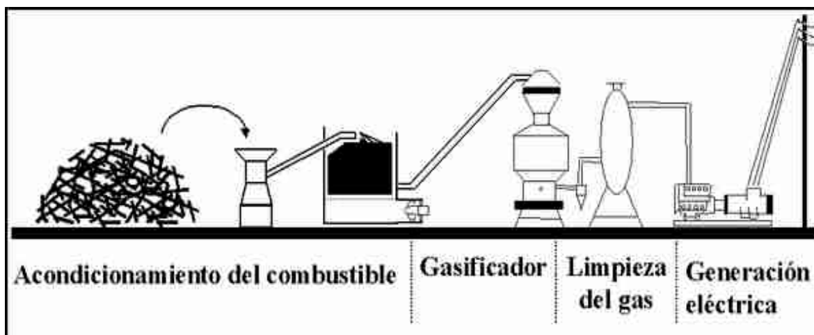
Figura 2.7: Esquema de aprovechamiento de la Biomasa. [117]
