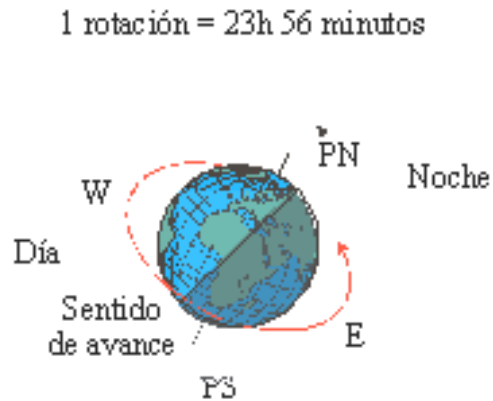
Figura 4.1: Movimiento de rotación Terrestre. [94]
