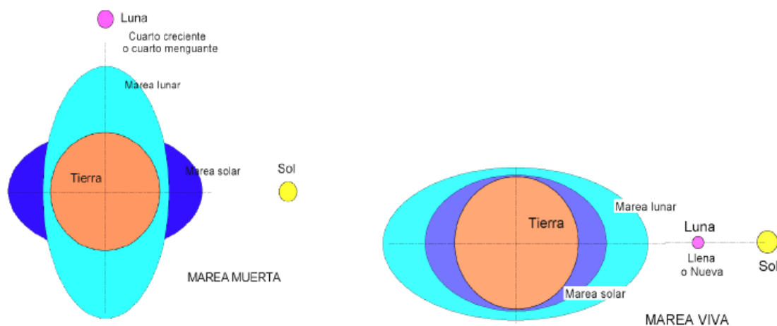
Figura 4.6: Mareas vivas y mareas muertas. [94]
