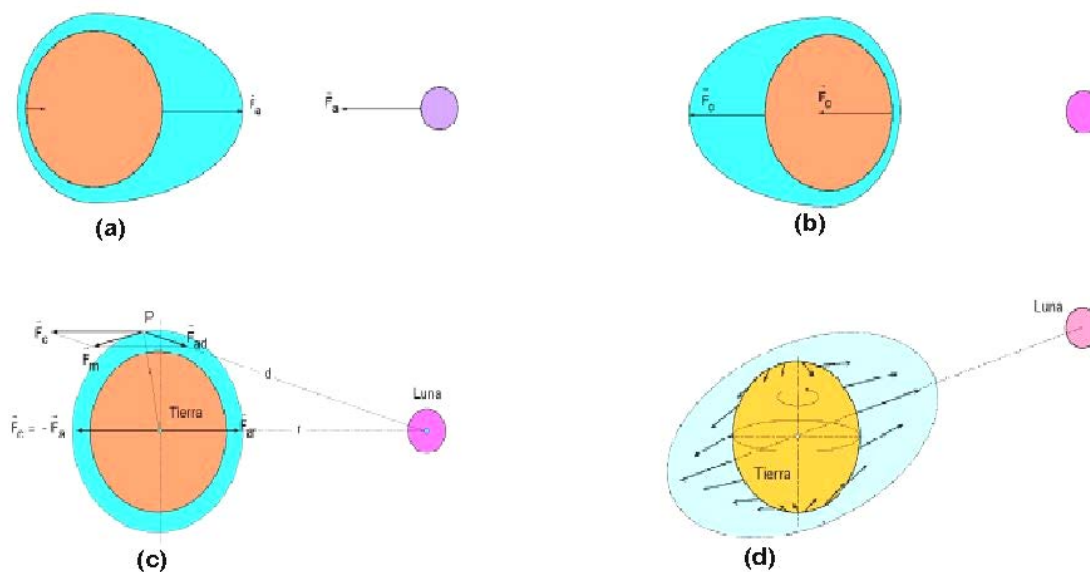
Figura 4.5: (a)Efecto de la fuerza atractiva sobre las masas de agua; (b) efecto de la fuerza centrífuga sobre las masas de agua; (c) y (d),efecto combinado de las fuerza centrífuga y atractiva sobre las masas de agua. [94]
