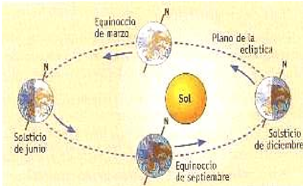
Figura 4.2: Movimiento de traslación terrestre. [94]
