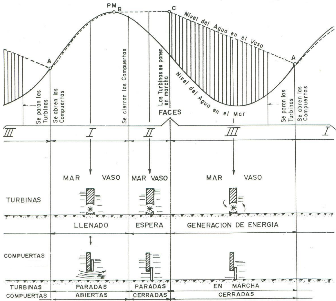
Figura 3.2: Funcionamiento del ciclo al simple efecto de vaciado. [24]
