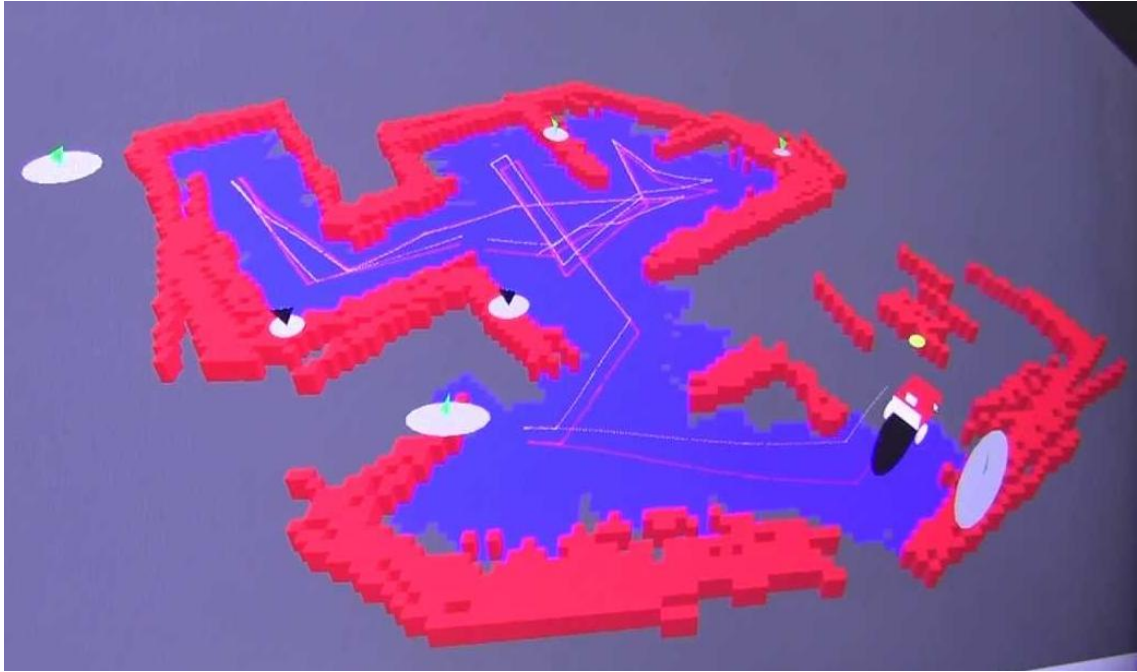
Figura 78. Aplicación del SLAM para la ubicación de un robot. [79]
