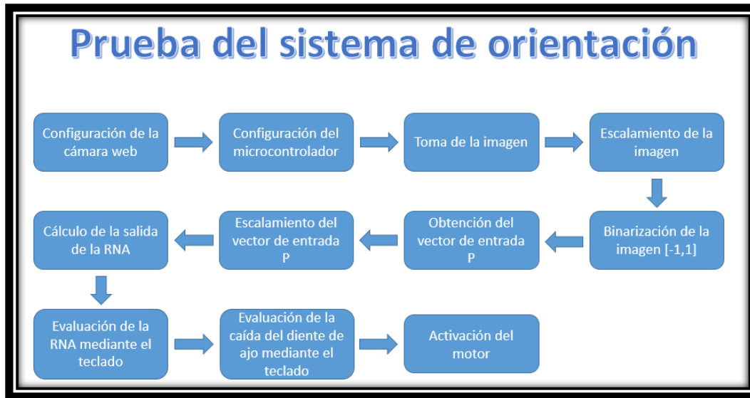
Figura 3.7 Diagrama de bloques del programa de prueba del sistema de orientación
