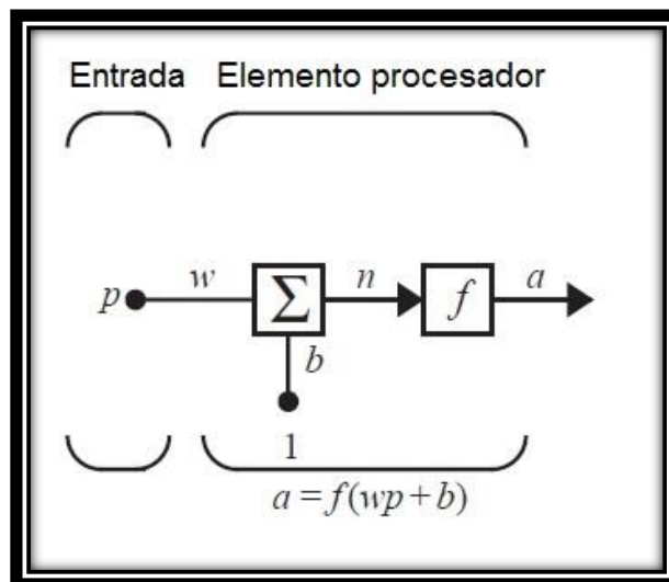
Figura 2.2 Modelo general de un elemento procesador
